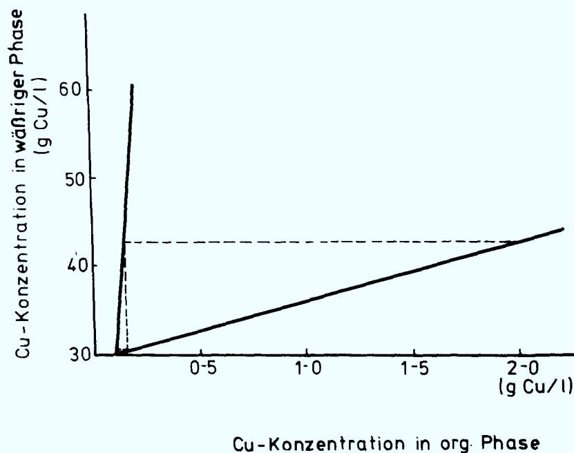
Abb. 26: McCabe-Thiele-Diagramm zur Rückextraktion von Kupfer - 2 Stufen Basis: Org. Phase: 11 % v/v LIX 64 N in Shellsol T mit 2,1 g \text{Cu}^{2+} /l Wäßrige Phase: 30 g \text{Cu}^{2+} /l; 170 g \text{H}_2\text{SO}_4 /l nach [26]
