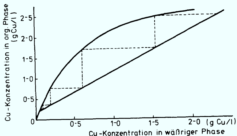
Abb. 25: McCabe-Thiele-Diagramm zur Extraktion von Kupfer - 5 Extraktionsstufen Basis: Wäßrige Phase: 2,35 g \text{Cu}^{2+} /l; 1,04 g \text{Fe}^{3+} /l; pH 2,0 Org. Phase: 11 % v/v LIX 64 N in Shellsol T nach [26]
