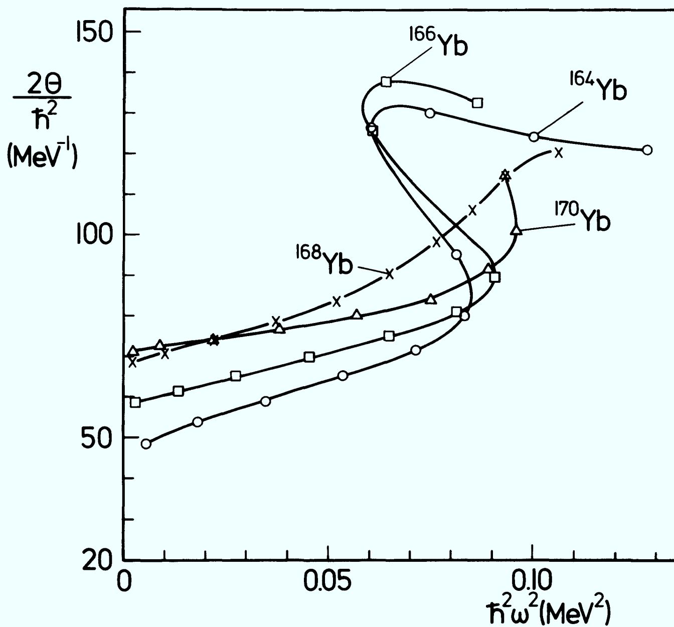
Fig. 9: Darstellung des Backbending-Verhaltens der GRB in ^{164}, ^{166}, ^{168}, ^{170}\text{Yb} .
