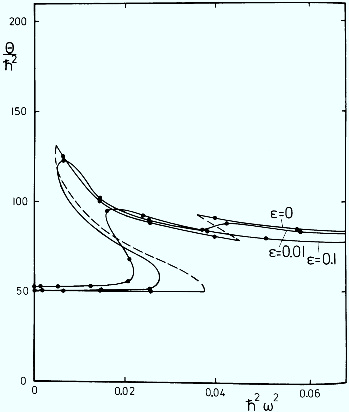
Fig.20: Darstellung des Backbending-Verhaltens der Yrastbande im Vierniveau-Modell für verschiedene Niveauabstände \epsilon .
