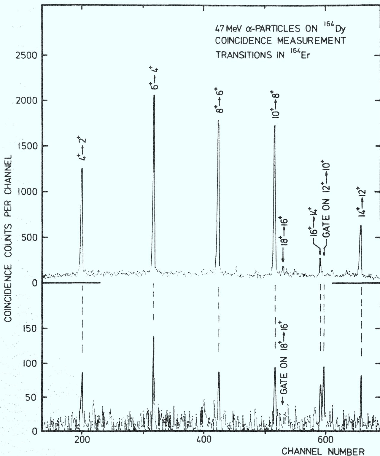
Fig. 4: Zwei \gamma - \gamma Koinzidenzspektren, in denen Fenster auf die 12^+ \rightarrow 10^+ und 18^+ \rightarrow 16^+ Übergänge in ^{164}\text{Er} gesetzt worden sind.
