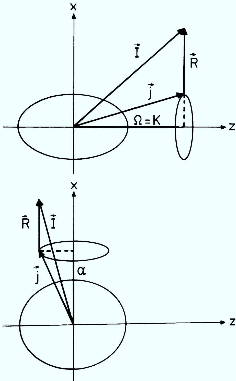
Fig.23: Schematische Vektordiagramme für das starke Kopplungsschema (oben) und das RAL-Kopplungsschema (unten). Die Ellipsen um den Ursprung charakterisieren den Potentialtopf der deformierten Kerne.
