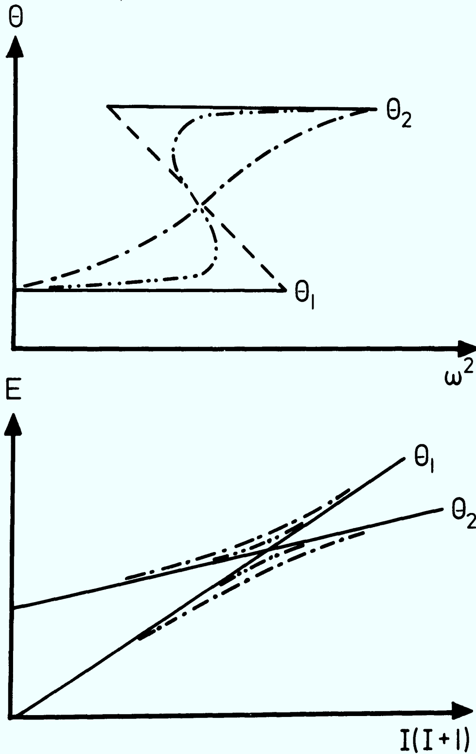
Fig.17: Schematische Darstellung des Backbending-Verhaltens zweier sich kreuzender Banden von unterschiedlichem Trägheitsmoment.
