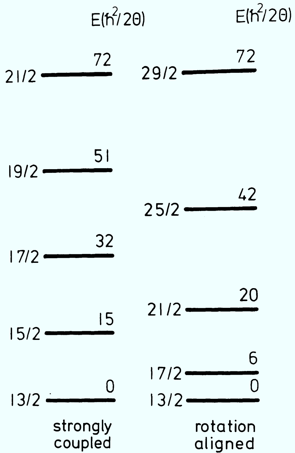
Fig.28: Darstellung der Anregungsenergien von i_{13/2} Banden in ungeraden Kernen für das starke Kopplungsschema (links) und das RAL-Kopplungsschema (rechts).
