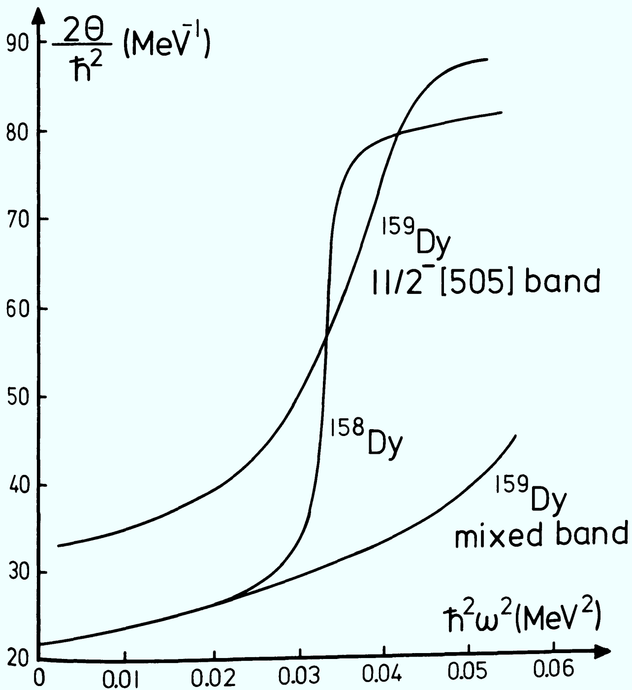
Fig.31: Darstellung des Backbending-Verhaltens der gemischten i_{13/2} Neutronenbande und der 11/2^- [505] Bande in ^{159}\text{Dy} sowie der GRB in ^{158}\text{Dy} berechnet im Rahmen der HFB-Cranking-Theorie.
