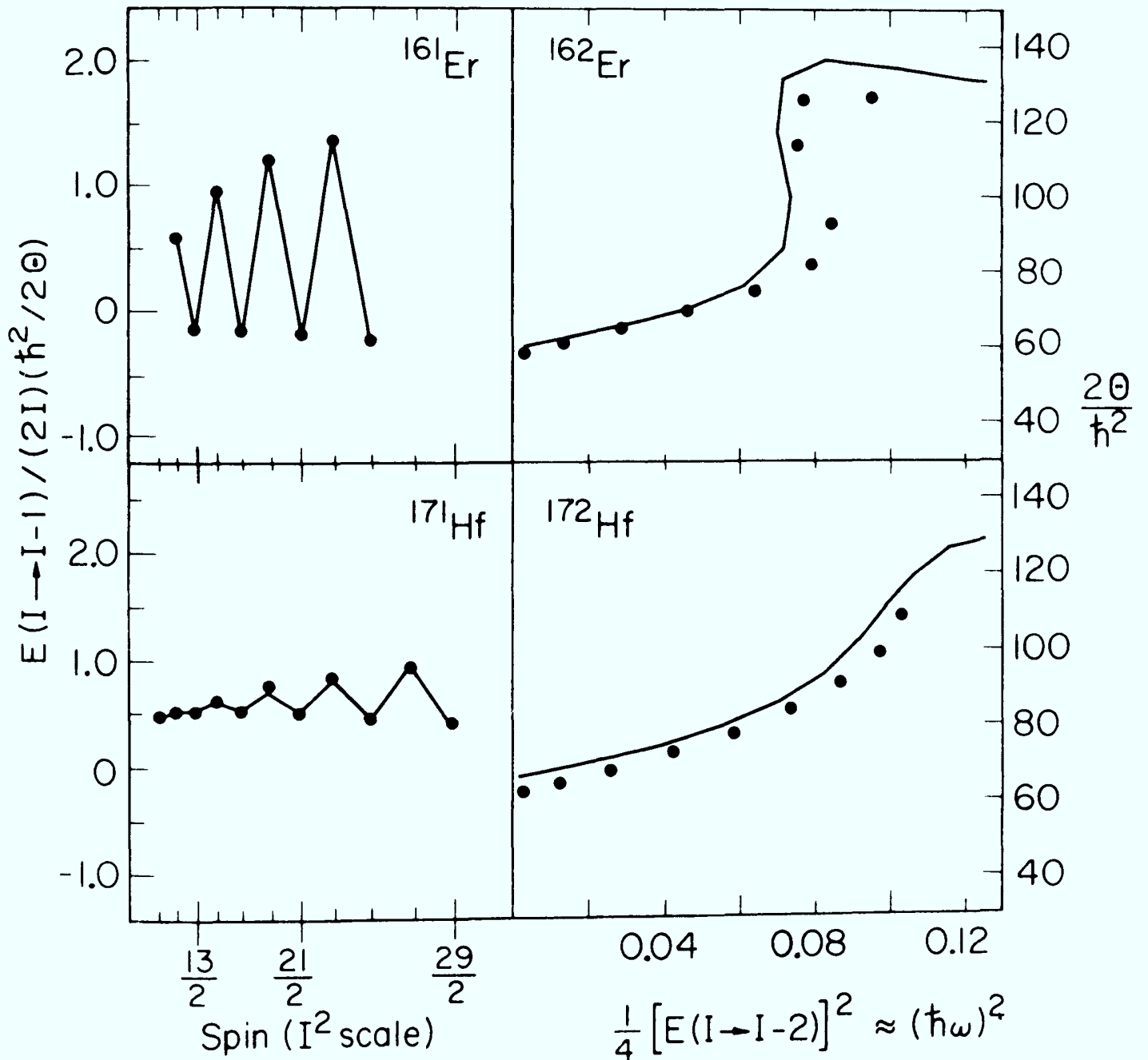
Fig.19: Vergleich der experimentellen (Punkte) und der im Rahmen des RAL-Modells berechneten (ausgezogene Linien) Eigenschaften von Zuständen in den Kernen ^{161,162}\text{Er} und ^{171,172}\text{Hf} . Für die gemischten i_{13/2} Neutronenbänden in ^{161}\text{Er} und ^{171}\text{Hf} ist die Energie der Kaskadenübergänge normiert auf 2I gegen I^2 aufgetragen worden. Für die GRB in ^{162}\text{Er} und ^{172}\text{Hf} ist das Backbending-Verhalten zu sehen.
