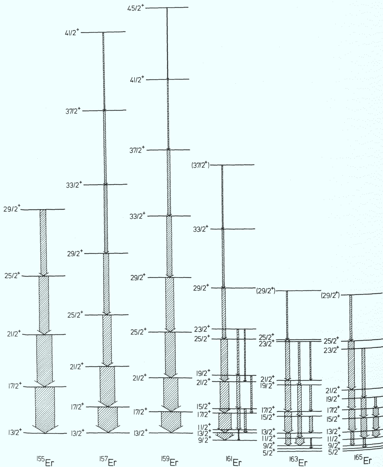
Fig.25: Niveauschemata der i_{13/2} Neutronenbanden in ungeraden Er-Kernen.
