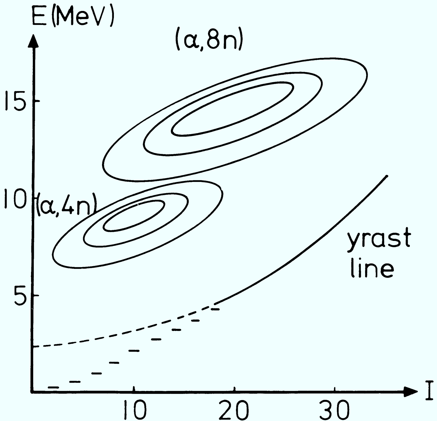
Fig. 1: Darstellung der gerechneten Bevölkerungsverteilung für die Endkerne ^{164,168}\text{Yb} , die durch (\alpha, 8n) bzw. (\alpha, 4n) Reaktionen erzeugt worden sind. Die Konturlinien geben die Wahrscheinlichkeit dafür an, daß sich ein Endkern in einem Zustand bestimmter Anregungsenergie und bestimmten Drehimpulses befindet.
