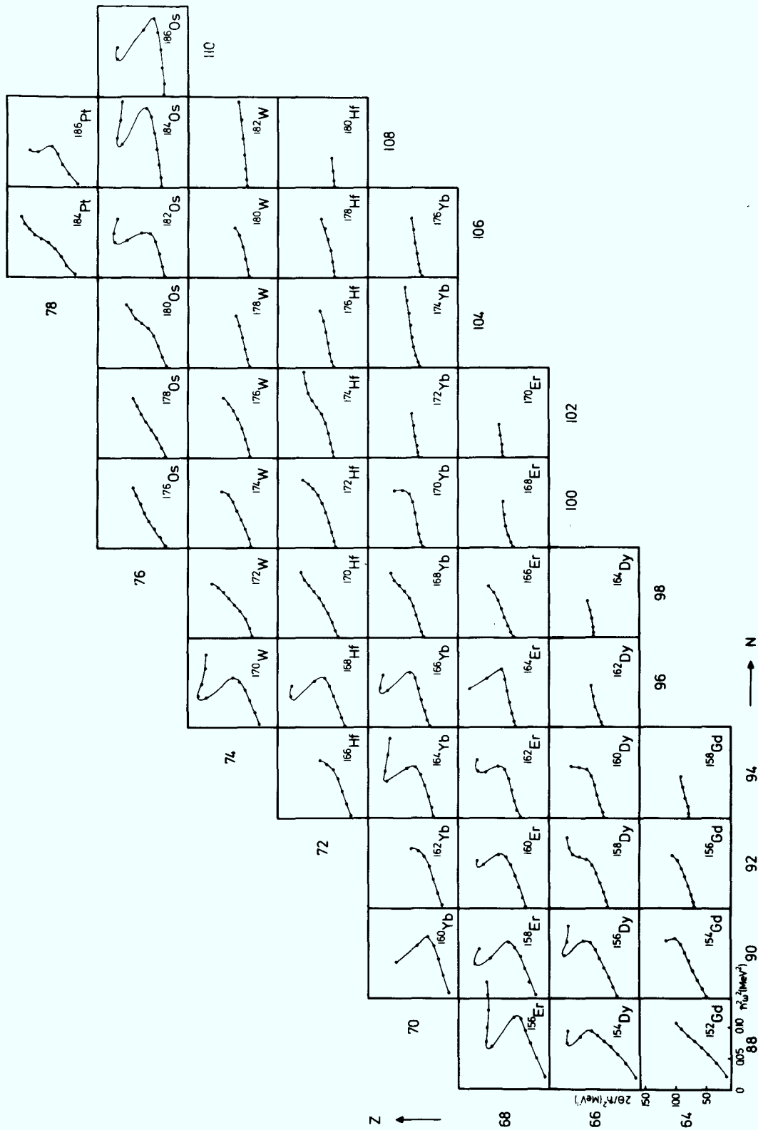
Fig. 8: Zusammenfassende Darstellung des Backbending-Verhaltens der in den Kernen der Seltenen Erden beobachteten Yrast-banden.
