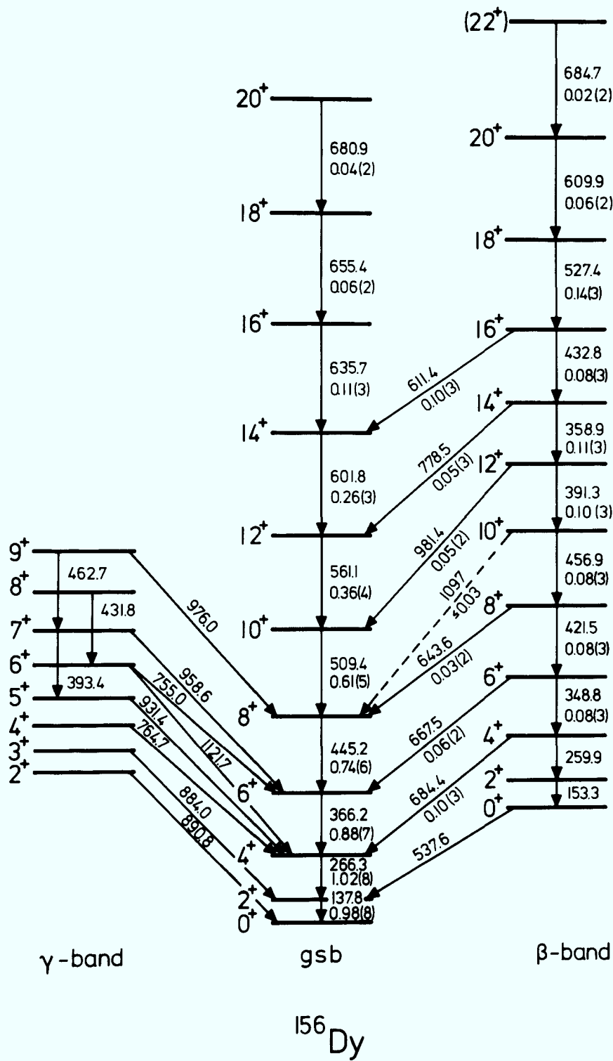
Fig.12: Niveauschema von ^{156}\text{Dy} .
