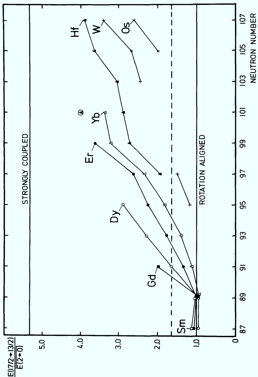
Fig.29: Darstellung des Energieverhältnisses E(17/2 \rightarrow 13/2)/E(2 \rightarrow 0) gegen die Neutronenzahl für 1_{13/2} Neutronenbanden von ungeraden deformierten Kernen und für die 5/2^- [512] Bande in ^{175}\text{Hf} (im Kreis). Die Grenzwerte für das starke bzw. RAL-Kopplungsschema sind eingezeichnet.
