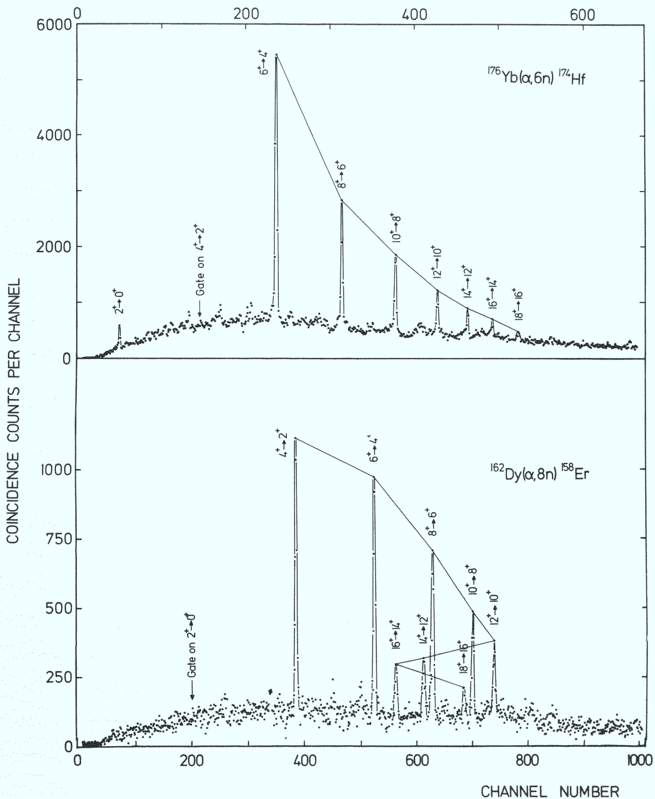
Fig. 2: Zwei \gamma - \gamma Koinzidenzspektren, in denen ein Fenster auf den 4^+ \rightarrow 2^+ Übergang in ^{174}\text{Hf} bzw. auf den 2^+ \rightarrow 0^+ Übergang in ^{158}\text{Er} gesetzt worden ist.
