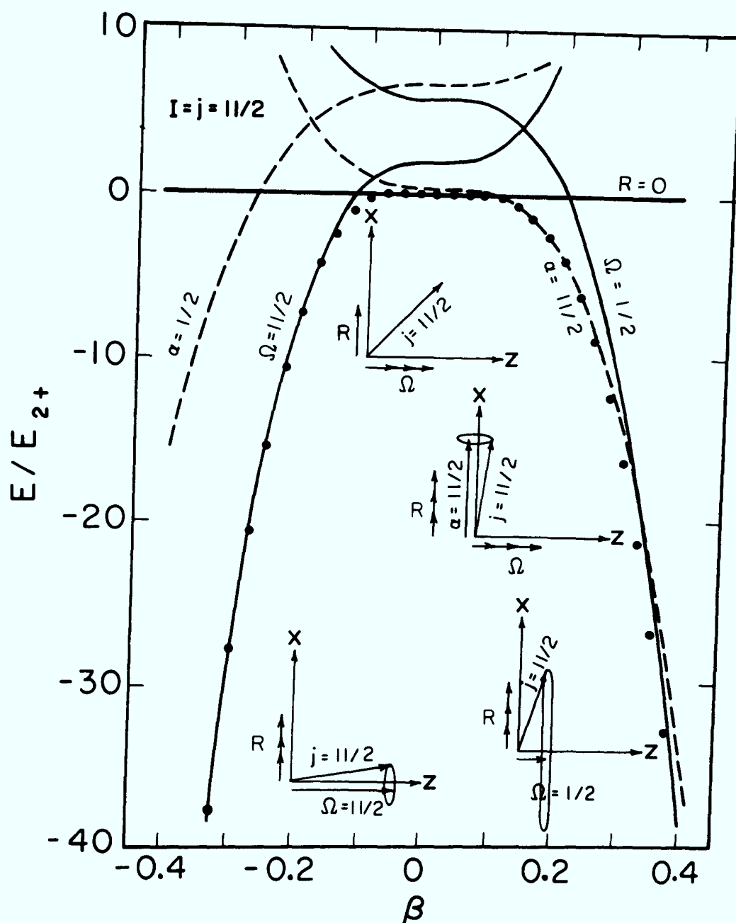
Fig.26: Darstellung der Energie des I=j=11/2 Zustands normiert auf die Energie des 2^+ Rump fzustands gegen den Deformationsparameter \beta für das schwache-, RAL- und starke Kopplungsschema (Linien) und für das Ergebnis der exakten Diagonalisierung des axialsymmetrischen Rotor-plus-Teilchen-Hamiltonoperators (Punkte). Die jeweils gültigen Kopplungsschemata sind angedeutet.
