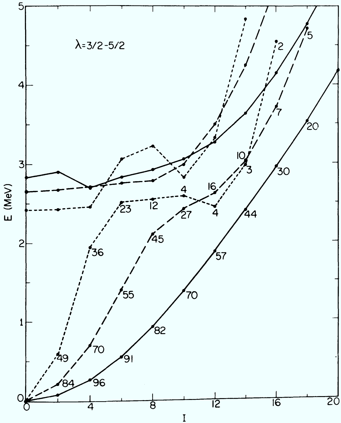
Fig.18: Darstellung der Anregungsenergie gegen I für die Yrast- und Yrarebanden im RAL-Modell für die Deformationsparameter \beta=0,3 (ausgezogene Linien), \beta=0,2 (gestrichelte Linien) und \beta=0,1 (gepunktete Linien). Die Zahlen geben die Intensitäten der Übergänge an.
