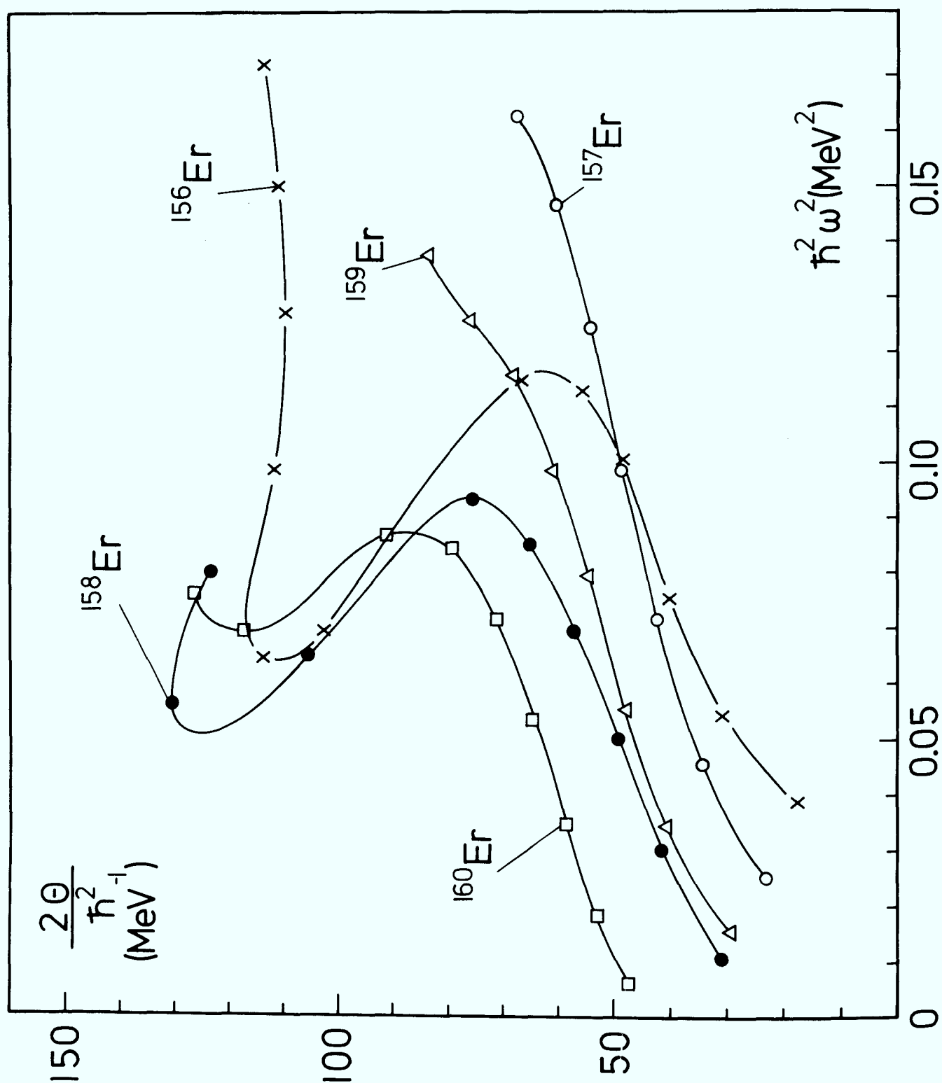
Fig.30: Vergleich des Backbending-Verhaltens der entkoppelten i_{13/2} Neutronenbanden in ^{157,159}\text{Er} und der GRB in ^{156,158,160}\text{Er} .
