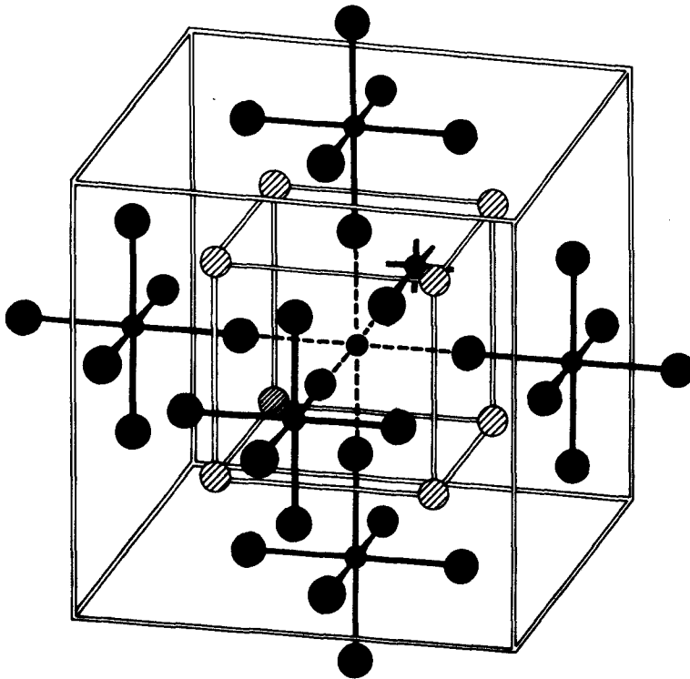
Abb. 43 Projektion auf der Oktaederlage (1/2, 1/2, 1/2) in der K_2MX_6 -Einheitszelle
