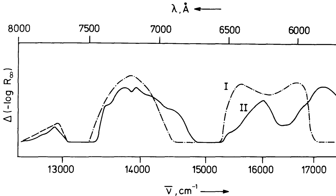
Abb. 22 Differenz zwischen dem relativen Reflexionsvermögen von bestrahltem und unbestrahltem polykristallines K_2ReCl_6 als Funktion der Temperatur I. Messung bei 296 K II. Messung bei 5 K
