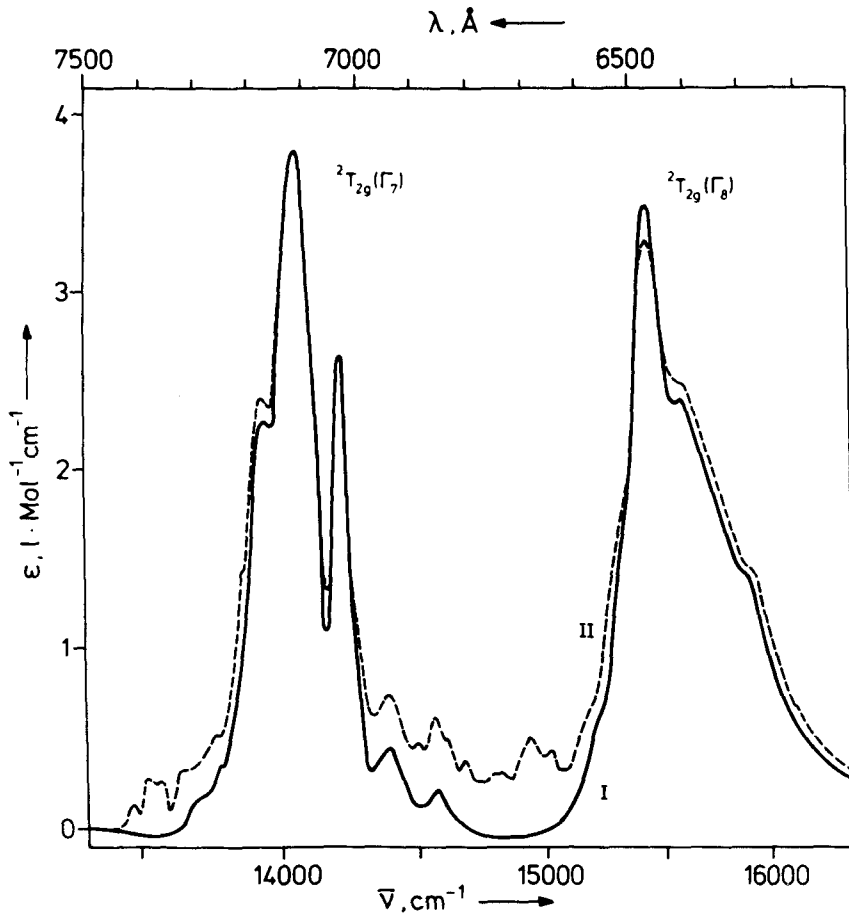
Abb. 16 Absorptionsspektrum eines K_2ReCl_6 -Einkristalls im sichtbaren Bereich vor (I) und nach (II) einer Bestrahlung mit 0,1 Cb \text{ cm}^{-2} 3 MeV-Elektronen bei 5 K, Messung bei 5 K
