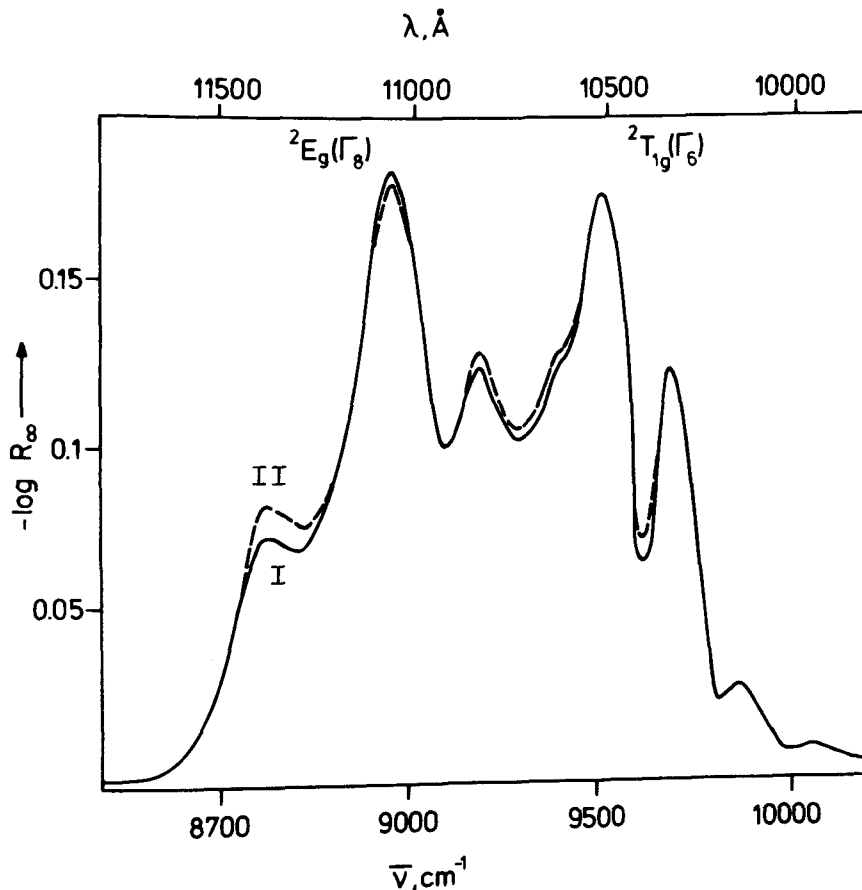
Abb. 18 Diffuse Reflexionsspektren (naher IR-Bereich) von polykristallinem K_2ReCl_6 vor (I) und nach (II) Implantation mit 0,2 \text{ mCb cm}^{-2} 40 keV Ar^+ -Ionen; Bestrahlung und Messung bei 5 K
