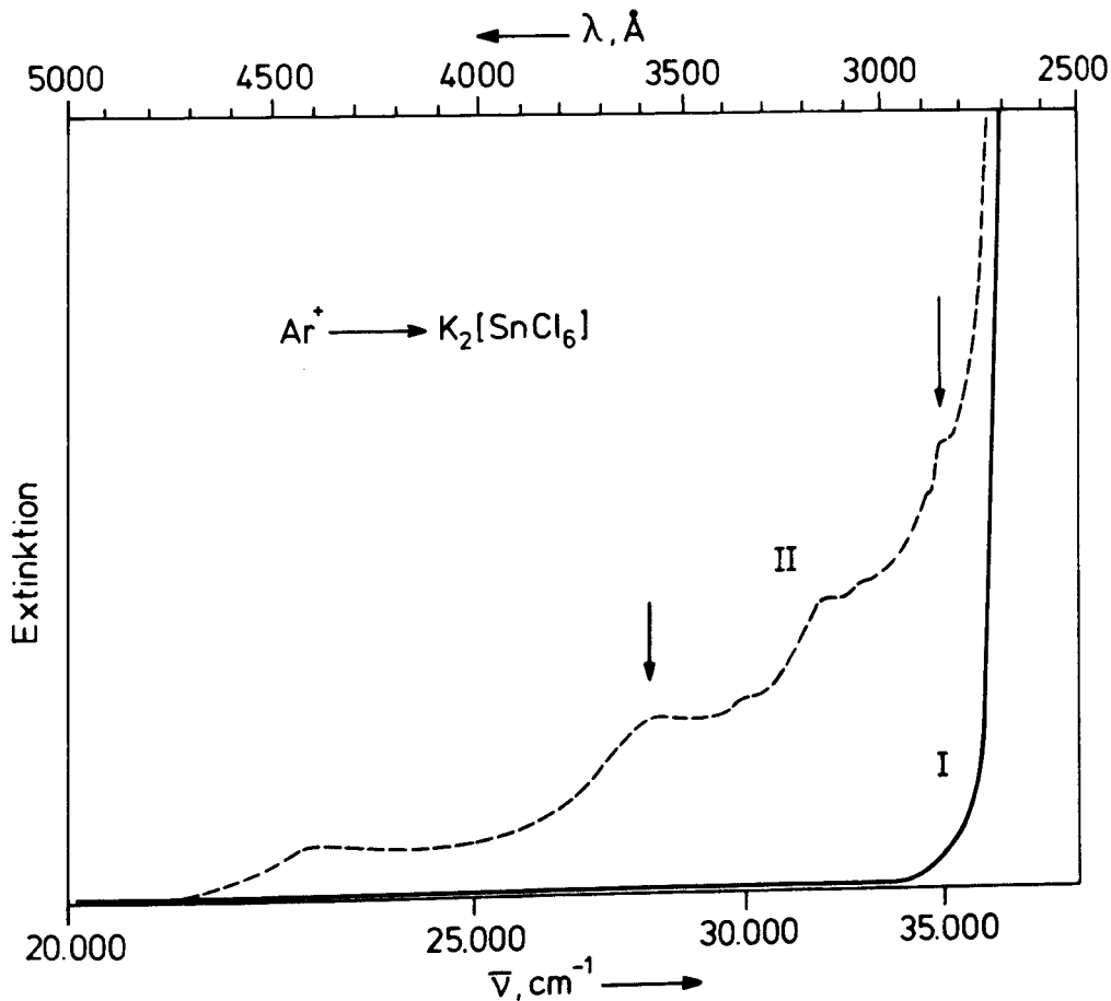
Abb. 26 Absorptionsspektren eines K_2SnCl_6 -Einkristalls (UV-Bereich) vor (I) und nach (II) Implantation von 0,3 \text{ mCb cm}^{-2} 40 keV Ar^+ -Ionen; Bestrahlung und Messung bei 5 K
