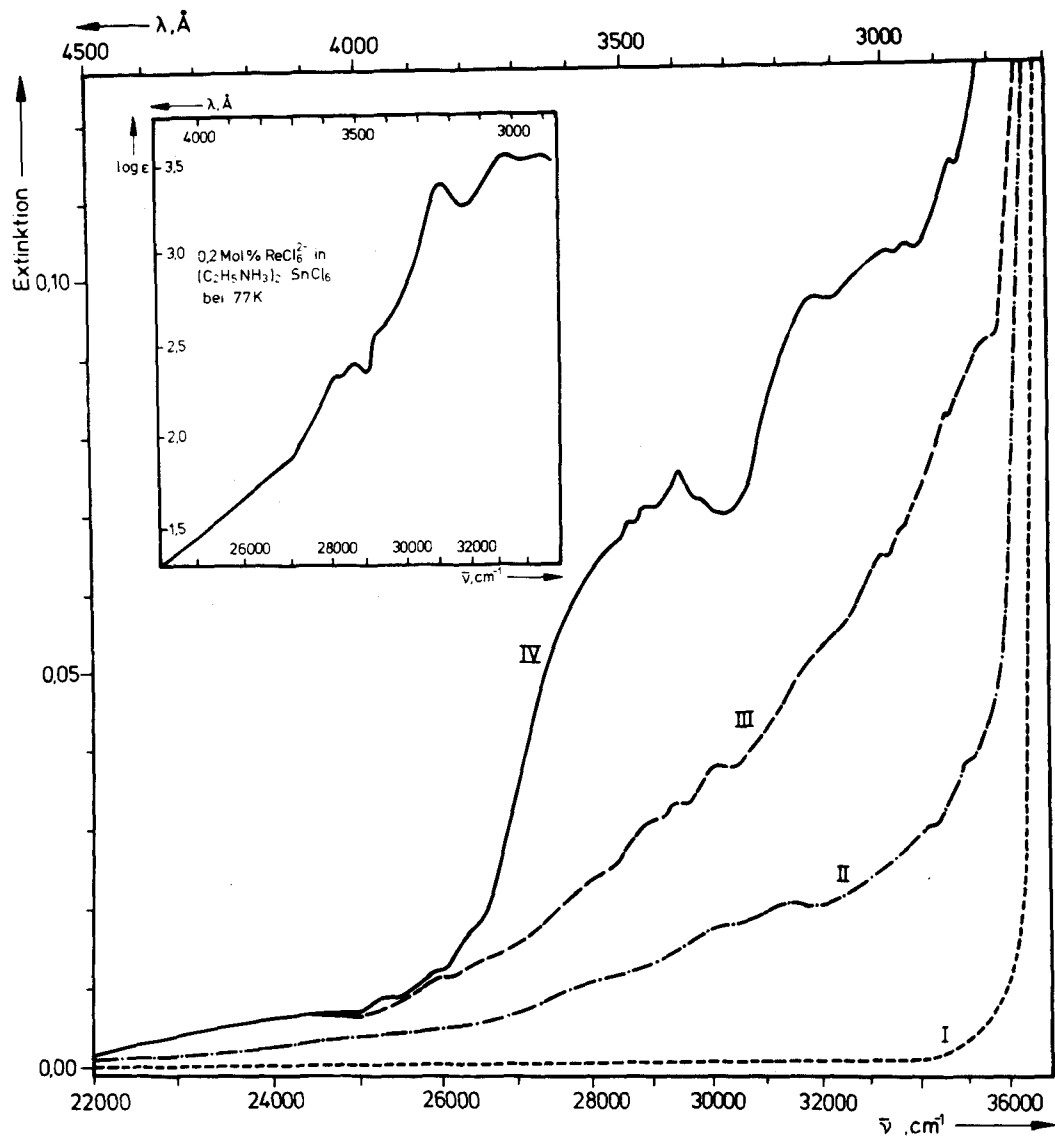
Abb. 31 Tieftemperaturabsorptionsspektren von K_2SnCl_6 im Bereich von 22000 bis 36000 cm^{-1} vor und nach Ionenbestrahlung
