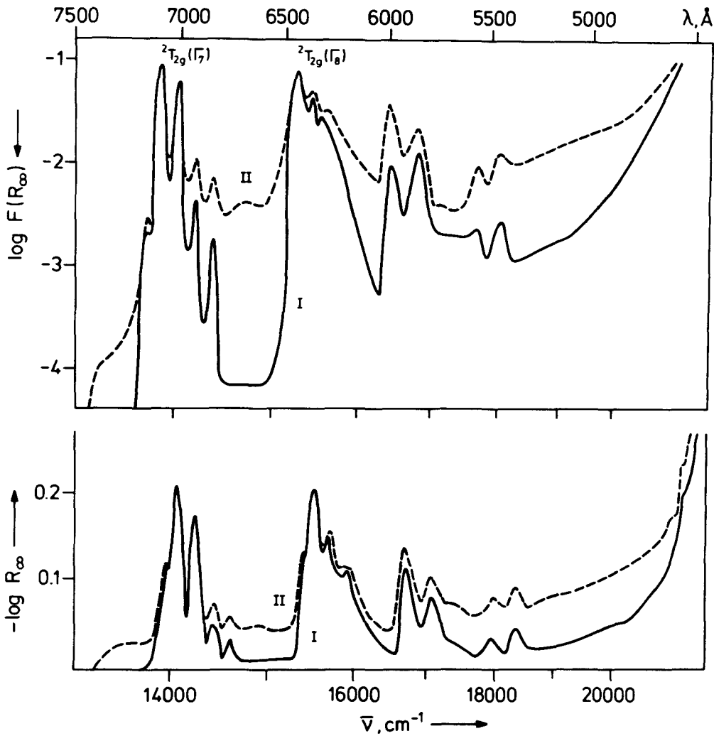
Abb. 20 Diffuse Reflexionsspektren (sichtbarer Bereich) von grob-polykristallinem \text{K}_2\text{ReCl}_6 vor (I) und nach (II) Implantation von 2 \text{ mCb cm}^{-2} 40 \text{ keV Ar}^+ -Ionen; Bestrahlung bei 293 \text{ K} und Messung bei 5 \text{ K}
