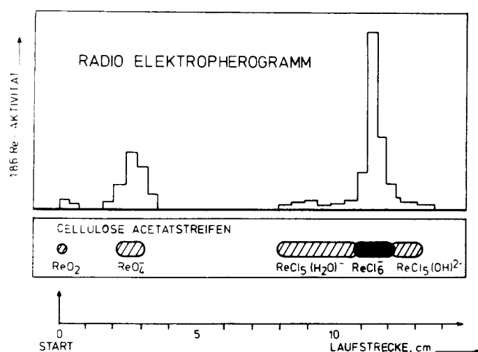
Abb. 7 Elektropherogramm von neutronenbestrahltem K_2ReCl_6 auf Celluloseacetat-Streifen
