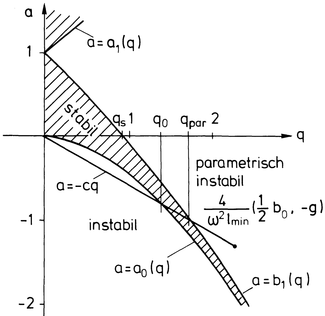
Fig. 4: Mathieusche Stabilitätskarte
