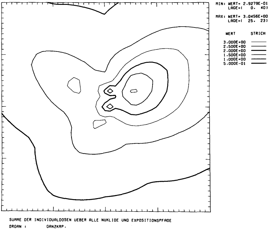
Abb. 5.2.2b : Isodosislينien der Ganzkörperdosis durch Block A und B
