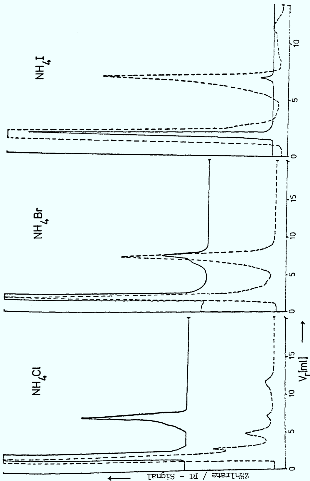
Abb. 9 Typische HPLC-Chromatogramme der Anionenaustauscher-Trennung auf Aminex A25; Trennbedingungen s. Abschnitt 2.6.
