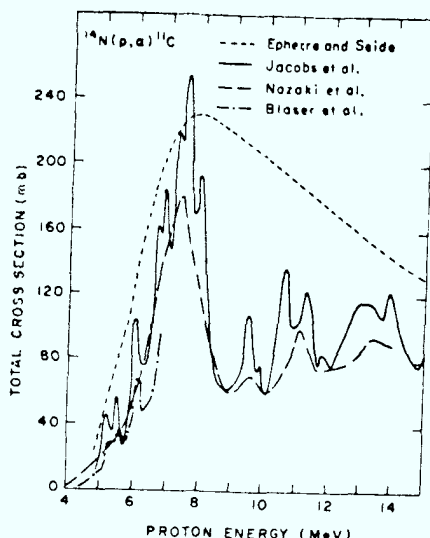
Abb. 1 Abhängigkeit des Wirkungsquerschnittes der Reaktion ^{14}\text{N}(p,\alpha)^{11}\text{C} von der Protonenenergie, nach [5]
