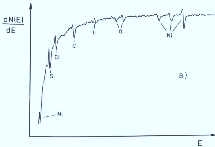
Abb. 15: Auger-Elektronen-Spektren, aufgenommen an einer Ni(001)-Fläche a) Starke Kontamination durch Fremdatome ( \geq 0,1 Monolage), b) Entfernung der Verunrei- nigungen ( \leq 0,01 Monolage) nach längerem Reinigungs- prozeß
