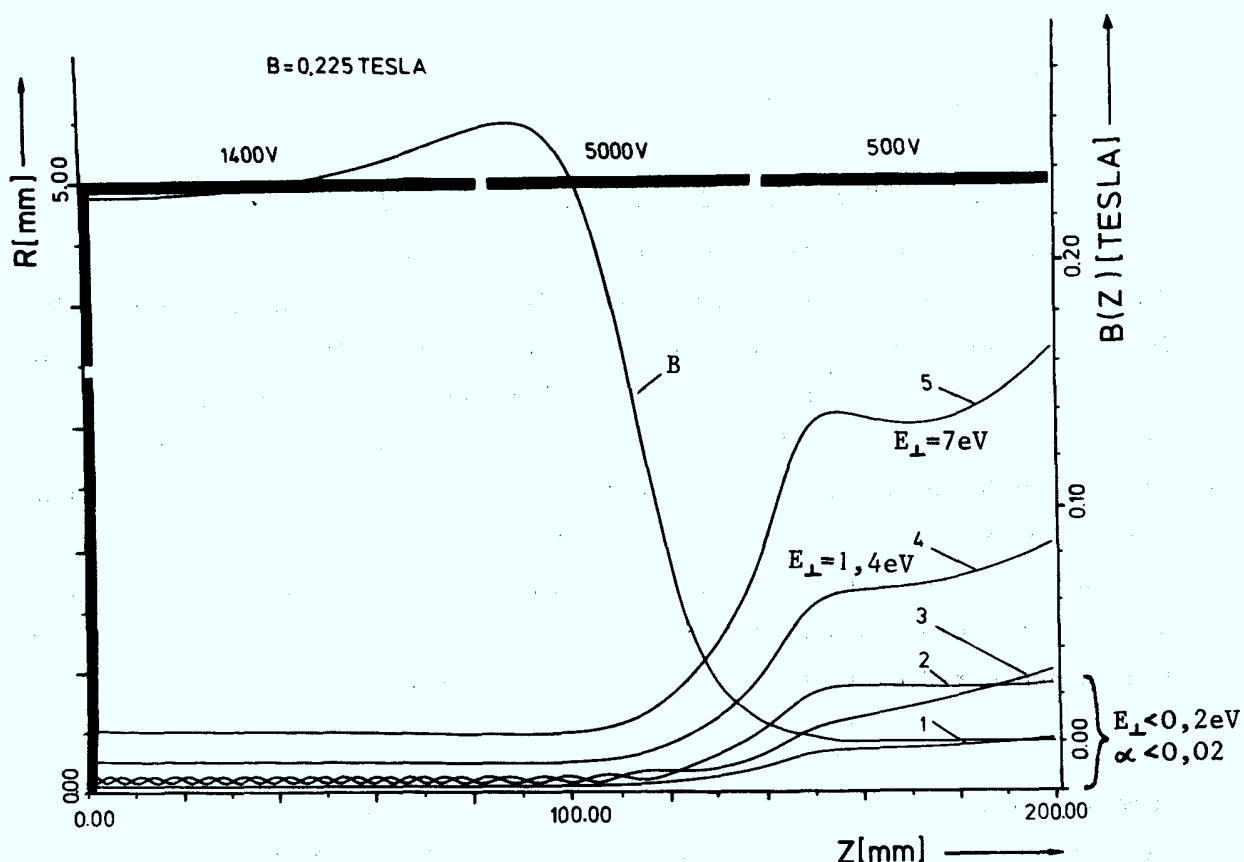
Abb. 9: Computer-Zeichnung von diskreten Elektronenbahnen und von der magnetischen Induktion B des Elektromagneten. Die angegebenen Potentiale der elektrostatischen Linsen sind auf die Probe bezogen. E_{\perp} ist die transversale Elektronen-Energie. Die Anfangsenergie der Elektronen beträgt einige eV
