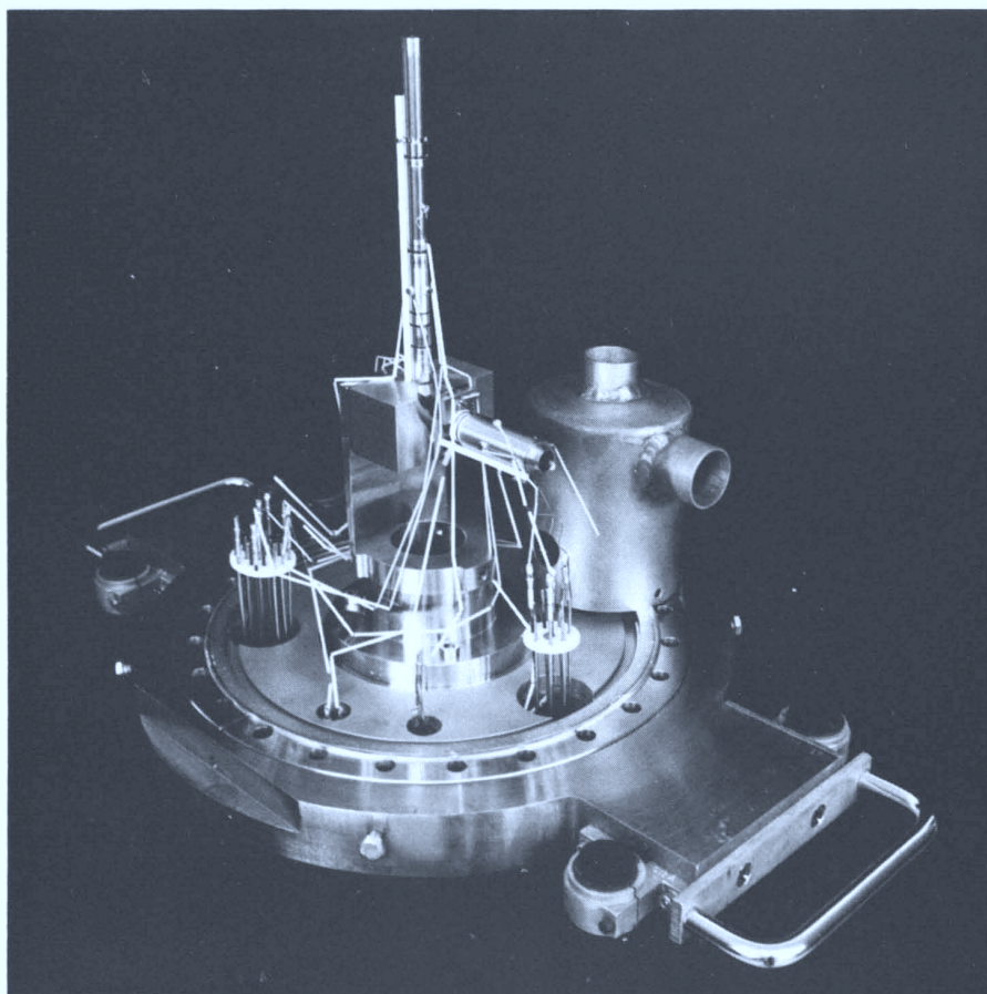
Abb. 12: Elektronenoptik aus elektrostatischen Rohrlinsen, Quadrupol-Ablenksystemen und einer 90^\circ -Umlenkeinheit (Kugulkondensator-Segment). Die magnetische Abschirmung aus \mu -Metall ist seitlich danebengestellt.
