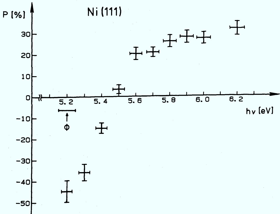
Abbn. 18 und 19 : ESP- Messungen an Ni(110) und Ni(111)
