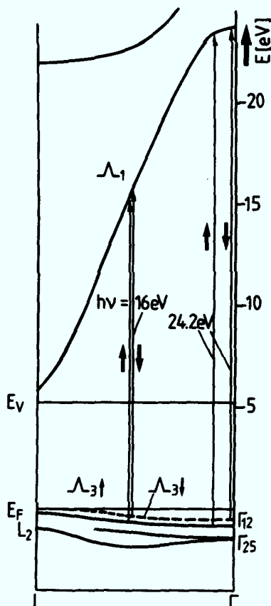
Abb. 25: Ni-Bandstruktur entlang der \Delta -Linie der fcc-Brillouin- Zone. Die direkten Übergänge aus dem obersten aufge= spaltenen \Delta_3 -Band bei h\nu = 16 und 24,2 eV sind mit Angabe der jeweiligen Spinrichtung eingezeichnet
