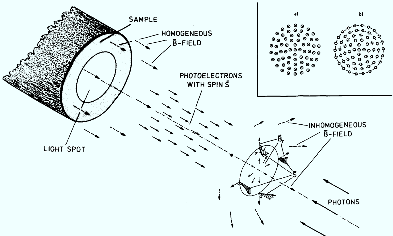
Abb. 10: Präzession des Elektronenspins \vec{S} durch radiale Magnetfeldkomponenten B_r . Rechts oben: Querschnitt durch einen polarisierten Elektronenstrahl vor (a) und nach der Spin-Präzession (b) (Blick von vorne auf die Spitzen der "Spin-Pfeile": \odot )
