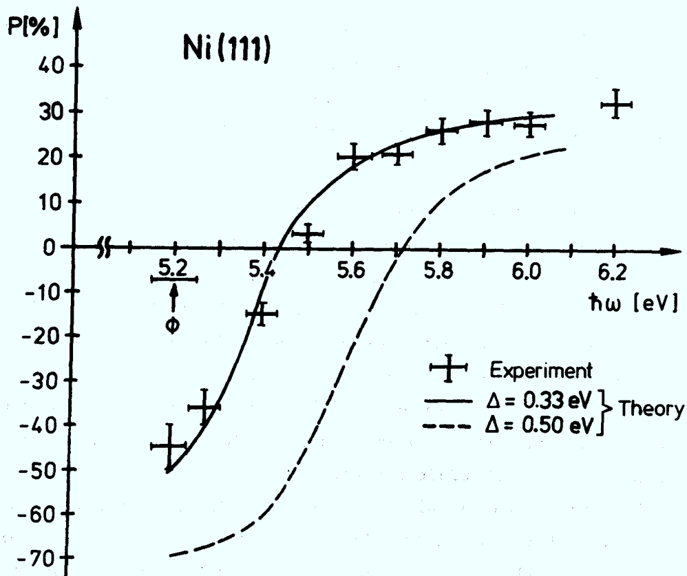
Abb. 27: Gemessene und berechnete Elektronen-Polarisation der Photo-Ausbeute an Ni(111) (aus Ref.52)
