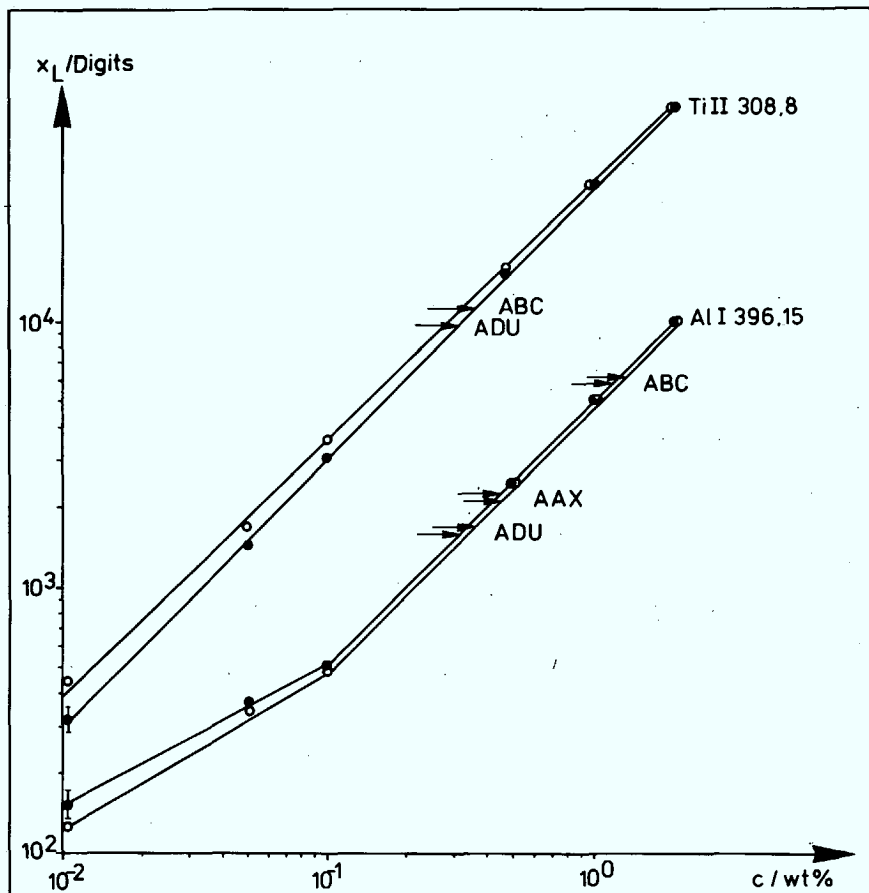
Abb. 57: Eichkurven zur Bestimmung von Ti und Al in Hochtemperaturlegierungen ( N_2 /Ar-Plasma, R = 0 , Beobachtungshöhe 15 mm, \circ reine H_2O Lösungen, \bullet Lösungen mit Zugabe von 200 \mu g \text{ ml}^{-1} Cr + 400 \mu g \text{ ml}^{-1} Fe und Ni)
