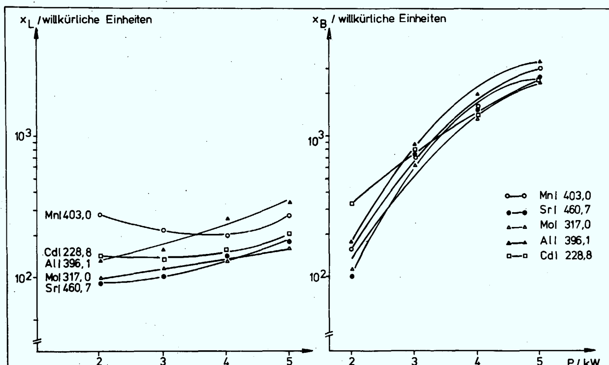
Abb. 23: Nettolinien- und Untergrundintensitäten von Atomlinien im N_2/Ar -Plasma als Funktion der Leistung (Konzentration der Elemente 1 \mu g \text{ ml}^{-1} , Beobachtungshöhe 15 mm, Integrationszeit 10 s, Wellenlänge in nm)
