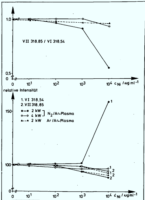
Abb. 53: Einfluß von Na (a), Cr (b), Ni (c) und Fe (d) auf die Emissionsintensität von 10 \mu\text{g ml}^{-1} V und daraus berechnete Linienintensitätsverhältnisse VII/VI (Wellenlänge ausgedrückt in nm)
