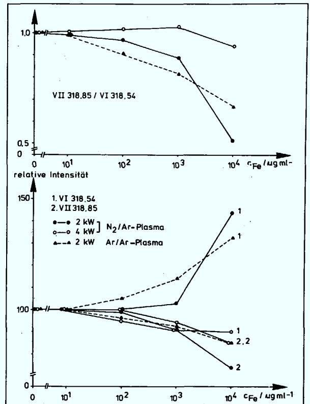
Abb. 53: Einfluß von Na (a), Cr (b), Ni (c) und Fe (d) auf die Emissionsintensität von 10 \mu\text{g ml}^{-1} V und daraus berechnete Linienintensitätsverhältnisse VII/VI (Wellenlänge ausgedrückt in nm)
