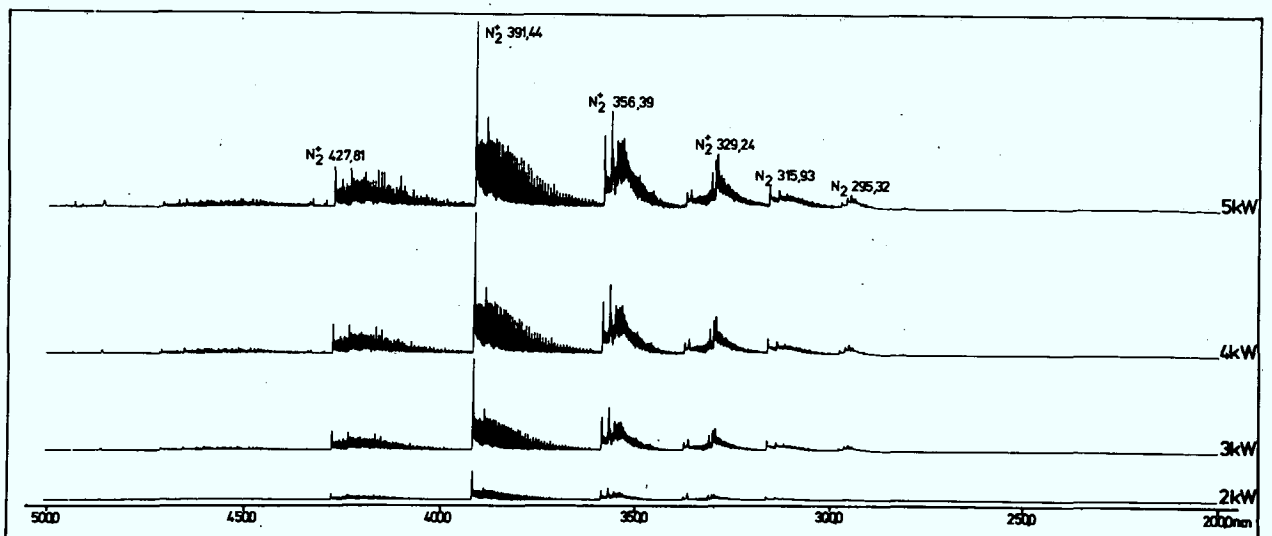
Abb. 17: Emissionsspektren des N_2/Ar -Plasmas bei verschiedenen Leistungen
