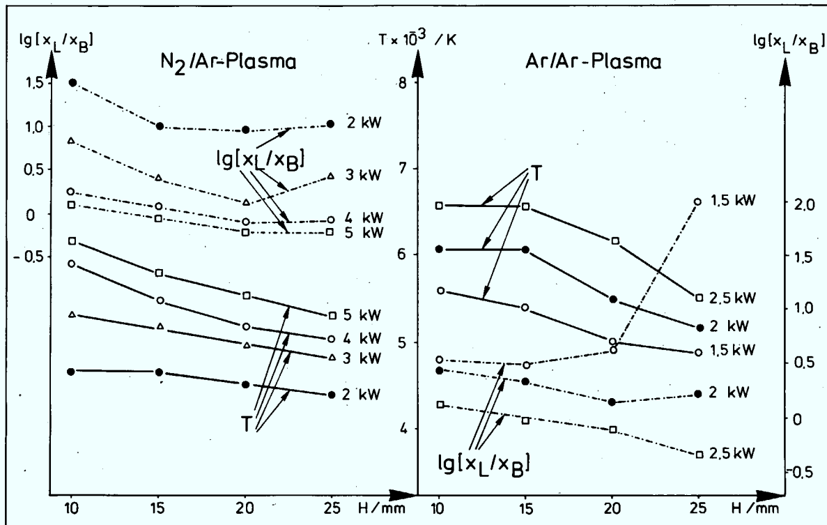
Abb. 45: Fe-Anregungstemperatur und Verhältnis Linien-/ Untergrundintensität der zur Temperaturbestimmung verwendeten FeI-Linie 373,49 nm in Abhängigkeit von der Beobachtungshöhe und der Leistung in N 2 /Ar- und Ar/Ar-Plasmen (R = 0, FeI 371,99nm/FeI 373,49nm)
