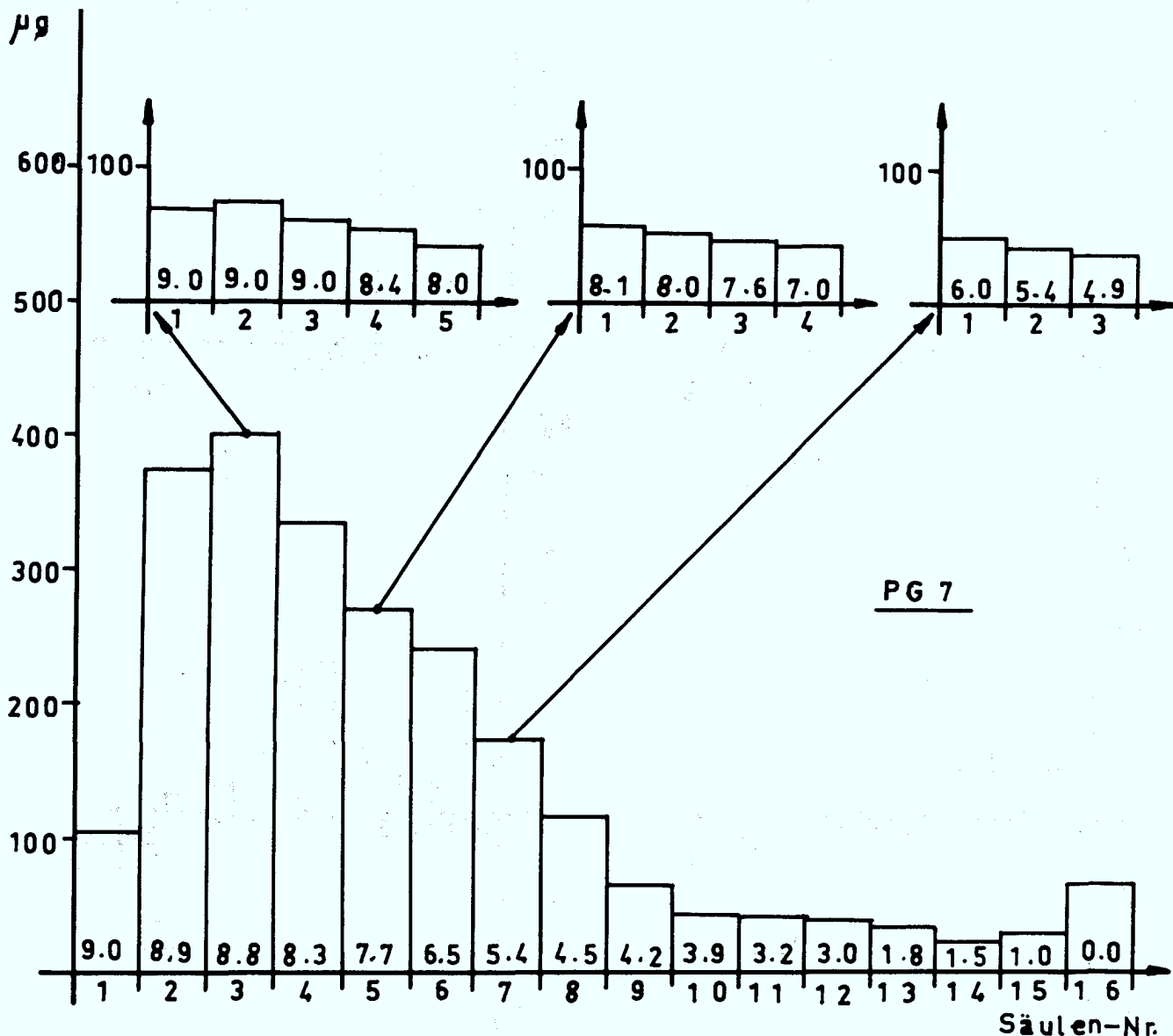
Abb. 16 Auftrennung einer Rhodopsin-Probe mit dem Durchschnitts-P.-Grad 7 P/Rh in Fraktionen mit verschiedenen P.-Graden auf der Ecteola-Säulen-Kaskade. Die Zahlen unter der x-Achse geben die Säulen-Nr. an, die Zahlen über der x-Achse den P.-Grad der zugehörigen Rhodopsin-Fraktion. Die Fraktionen von den Säulen Nr. 3, 5 und 7 wurden nach Reinigung auf einer Concanavalin-A-Sepharose-Säule einer weiteren Auftrennung auf 3 weiteren Ecteola-Säulen-Kaskaden unterzogen (inset). Einzelheiten s. Text.
