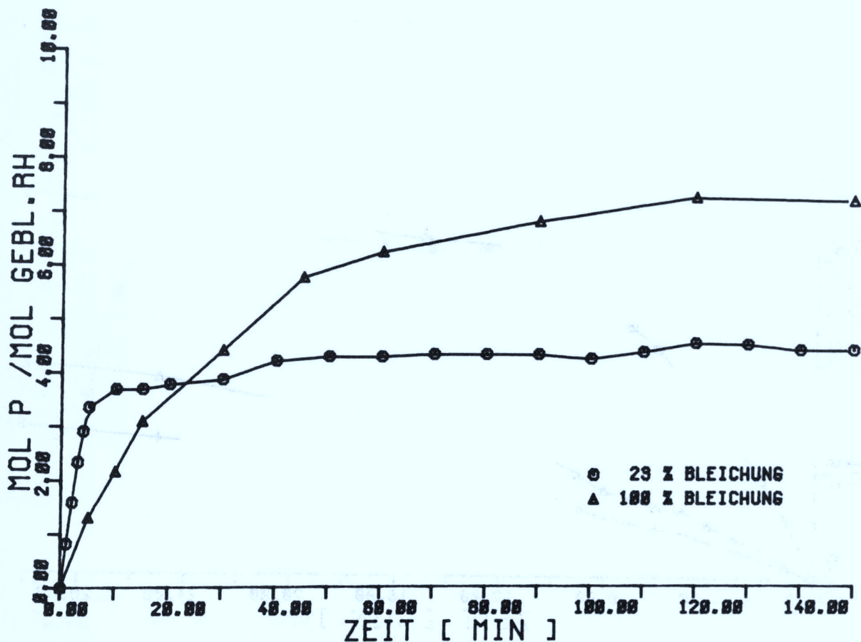
Abb. 18 Zeitverlauf der Phosphorylierung mit der gleichen Rinder-ROS-Präparation bei 23 % und 100 % Bleichung. Inkubationsmedium: 100 mM NaPP, 3 mM ATP, 1 mM \text{MgCl}_2 , pH 7,4.
