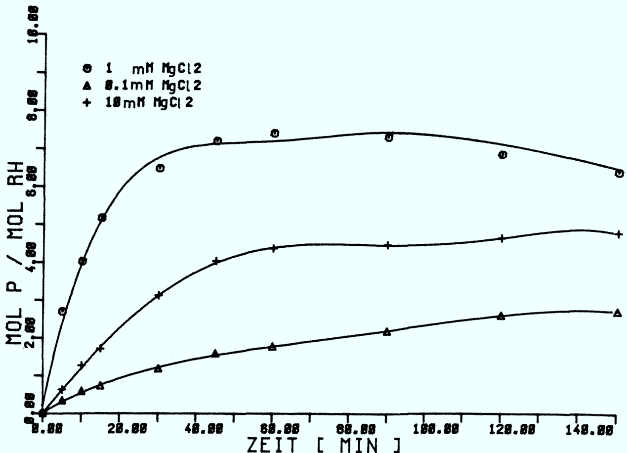
Abb. 9 Einfluß der Mg^{2+} -Konzentration auf Initialgeschwindigkeit und Endwert der Phosphorylierung. Inkubationsmedium: 100 mM Tris-HCl, 3 mM ATP, pH 7,4.
