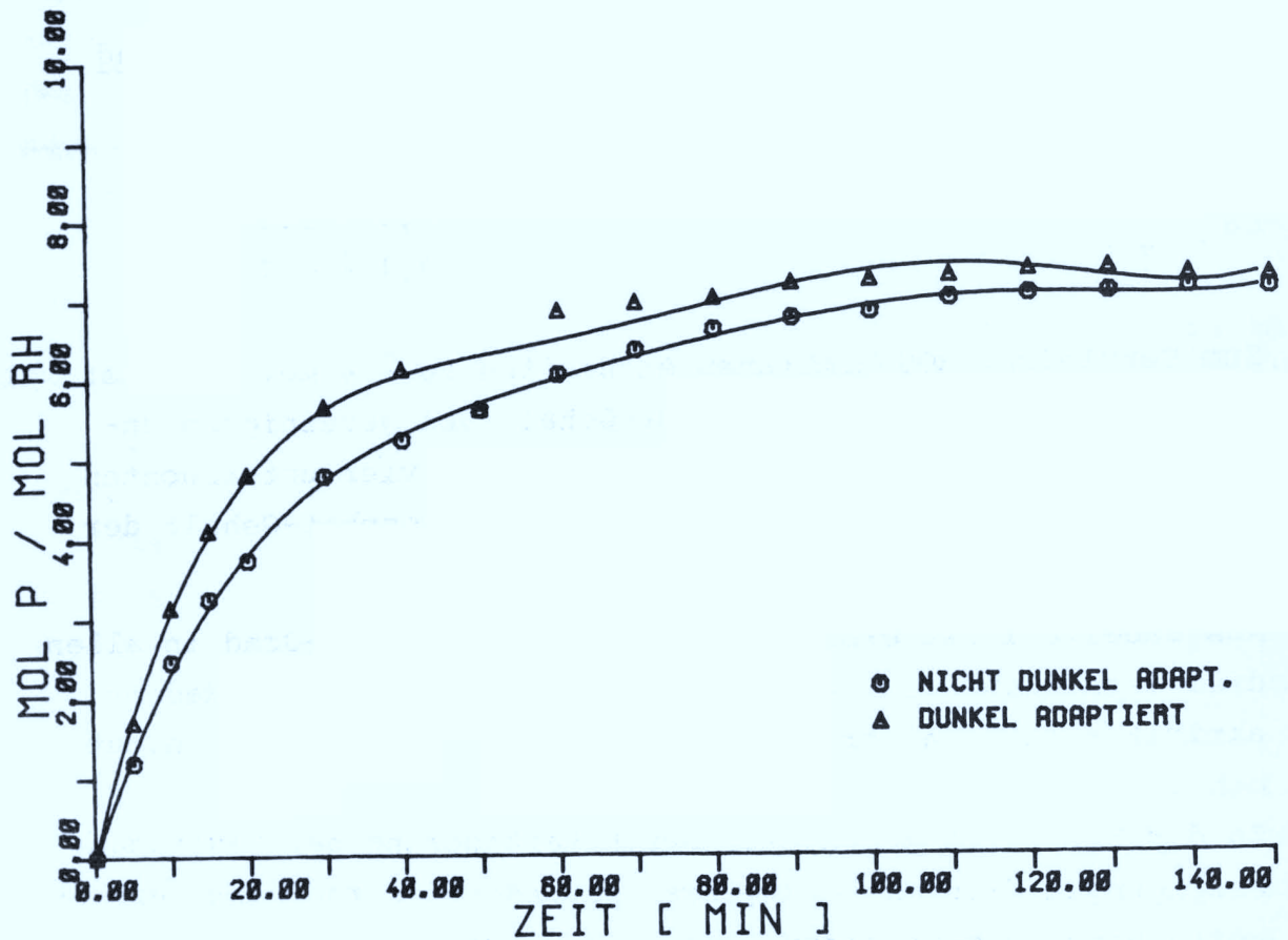
Abb. 5 Zeitverlauf der Phosphorylierung mit einer dunkeladaptierten und einer nicht-dunkeladaptierten ROS-Präparation. Inkubationsmedium: 100 mM NaPP, 3 mM ATP, 1 mM \text{MgCl}_2 , pH 7,4.
