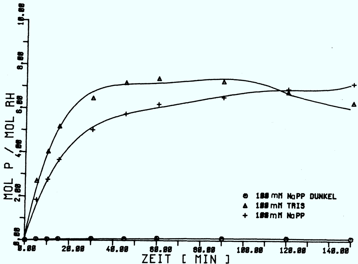
Abb. 2 Vergleich des Zeitverlaufs der Phosphorylierung mit der gleichen ROS-Präparation in Tris-HCl und NaPP bei kontinuierlicher Belichtung und im Dunkeln in NaPP. ATP-Konzentration jeweils 3 mM, MgCl_2 1 mM, pH 7,4 (=optimale Bedingungen)
