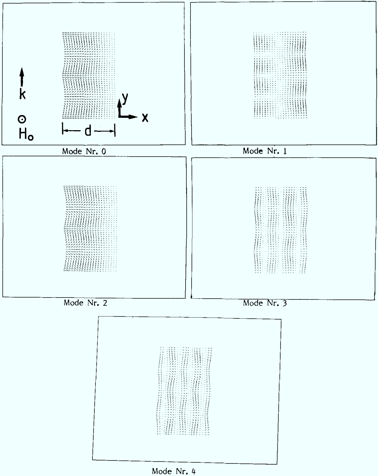
Bild 1.5: Wie Bild 1.4, aber für eine 50 nm dicke Fe-Schicht
