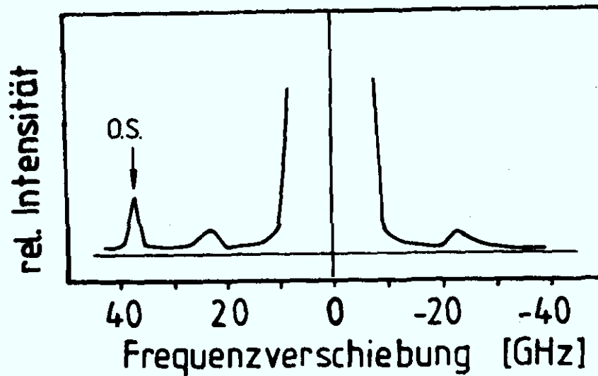
Bild 3.4: Streuspektrum von einer 300 nm dicken Fe-Schicht. B_0 = 0,23 T Es ist die elastische Linie und die zugehörigen inelastischen Linien von der Oberflächenspinwelle (O.S.) und den Volumenspinwellen dargestellt.
