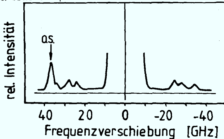
Bild 3.5: Streuspektrum von einer 100 nm dicken Fe-Schicht. B_0 = 0,23 T Die Volumenspinwellen spalten in stehende Spinwellen auf.
