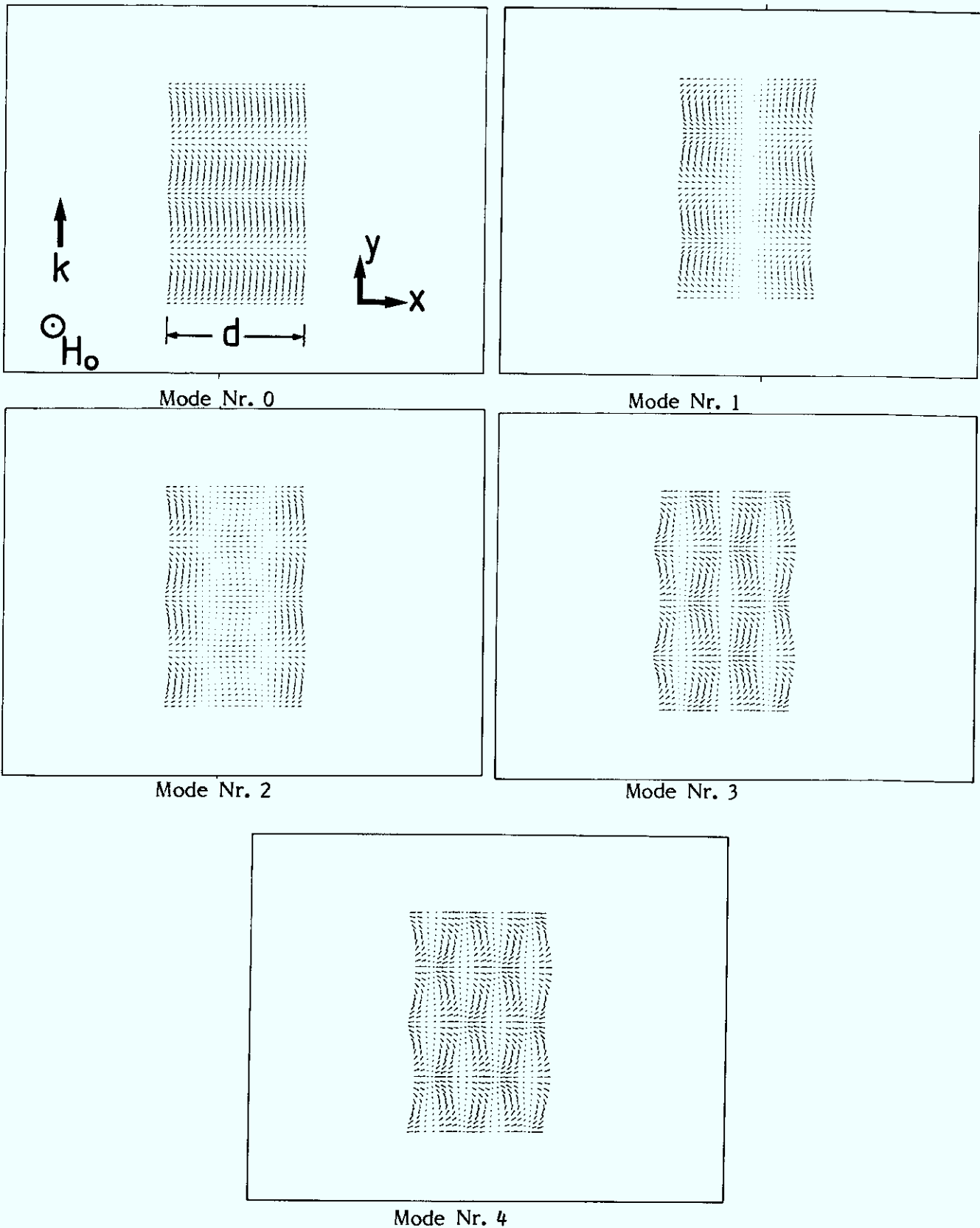
Bild 1.4: Verlauf der Querkomponente der Magnetisierung für verschiedene Spinwellenmoden in einer 15 nm dicken Fe-Schicht bei einem äußeren Feld von B_0 = 0,05 T. In y-Richtung sind zwei Wellenlängen der Spinwellen dargestellt. Die Mode Nr. 0 ist die Oberflächenspinwelle und die anderen Moden sind die stehenden Spinwellen mit der entsprechenden Anzahl von Wellenknoten senkrecht zur Schicht.
