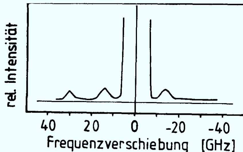
Bild 3.14: Streuspektrum einer Doppelschicht Fe/SiO 2 /Fe; d_1 = 150 nm/ d_0=10 nm/ d_2=15 nm; B_0=0.05 T
