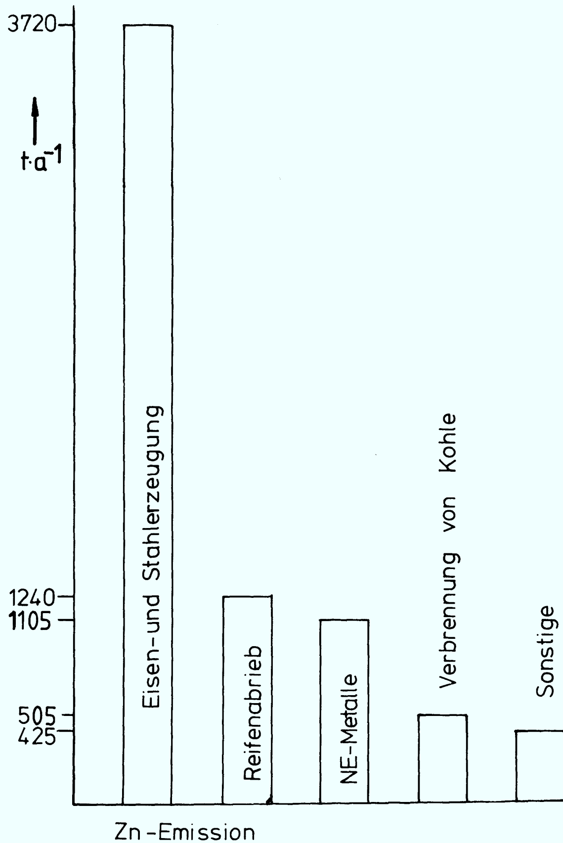
Abb. 16 Verteilung der Zn-Gesamtemission für die Bundesrepublik auf Emittentengruppen
