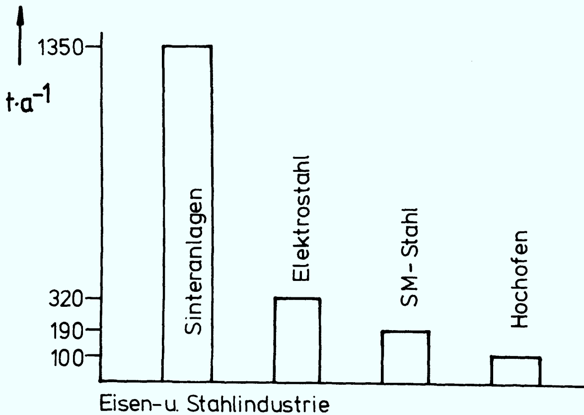
Abb. 4 Staubförmige Pb-Emission der Metallindustrie
