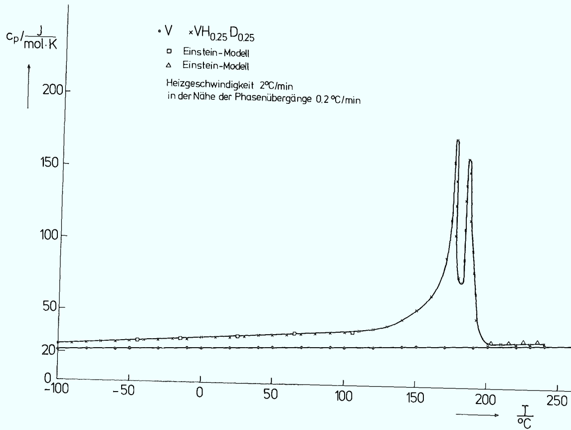
Abb. 18: Messung der spezifischen Wärme an \text{VH}_{0.25}\text{D}_{0.25} (Aufheizen)
