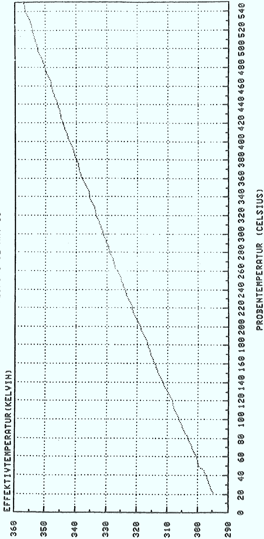
Abb. 9: Bestimmung der Effektivtemperatur des Probenvolumens
