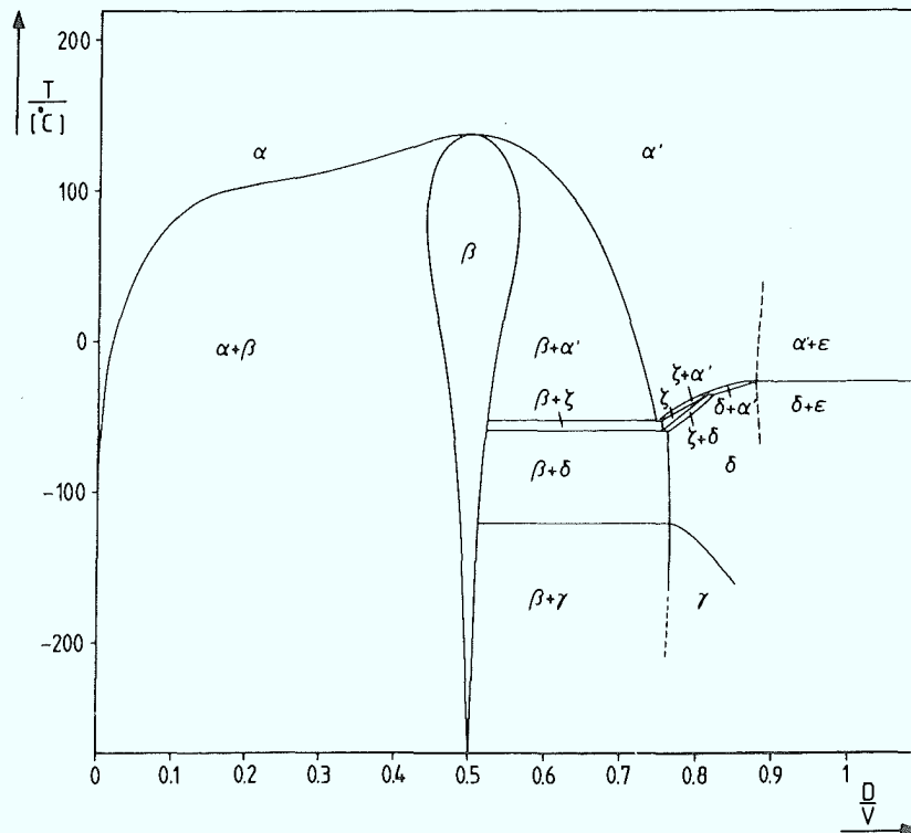
Abb. 1: V-H-Phasendiagramm nach /34/
