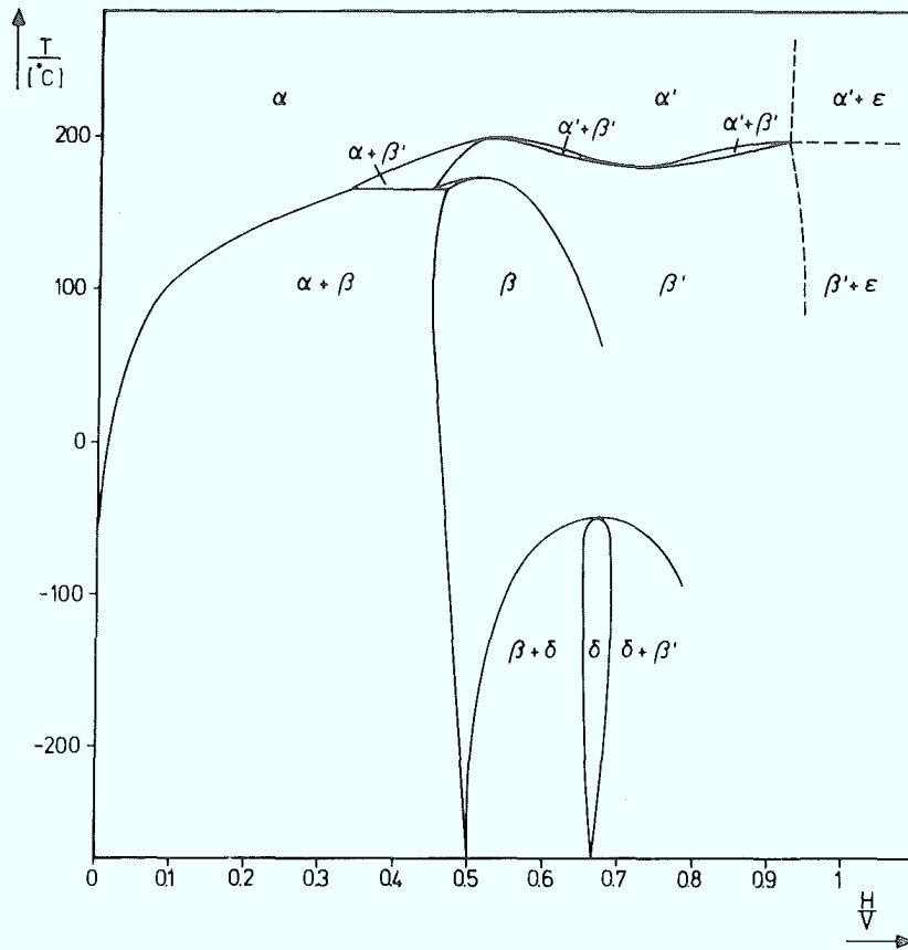
Abb. 1: V-H-Phasendiagramm nach /34/
