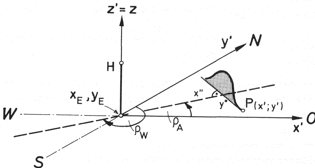
Abb. 3.2.1: Überblick der verwendeten Koordinatensysteme
