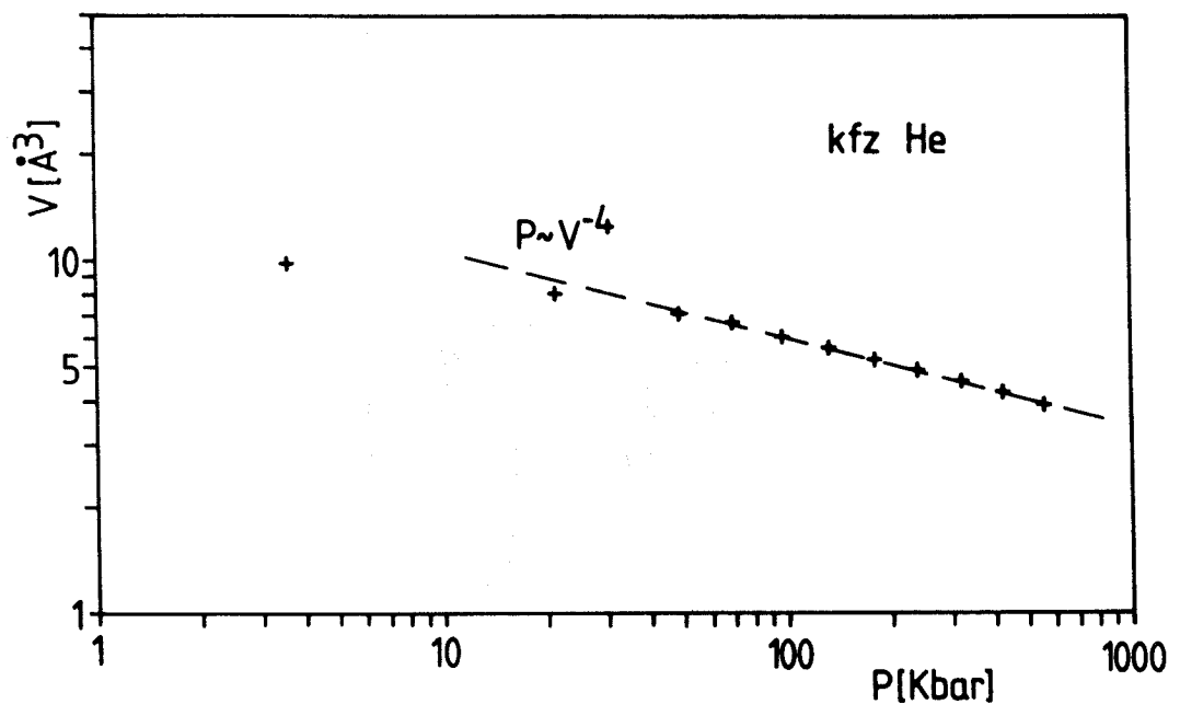
Fig. 4.9 Aus der totalen Energie des Grundzustandes für kfz He berechnete Abhängigkeit des He-Atomvolumens V von dem Elektronengasdruck P /4.16/. Die Gerade gibt ein V \propto P^{-1/4} -Verhalten wieder.
