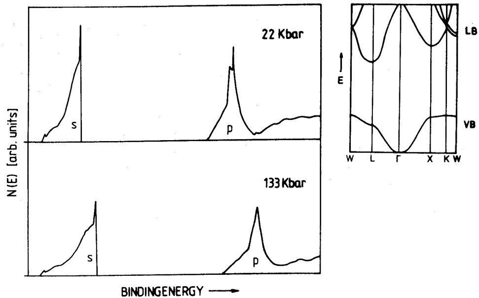
Fig. 4.8 Links: Zustandsdichte N(E) als Funktion der Bindungsenergie für kfz He für zwei Elektronengasdrücke /4.16/. p(s) bedeutet, daß die Zustände überwiegend p(s)-Charakter besitzen. Rechts: Bandstruktur von kfz He unter einem Elektronengasdruck von 600 Kbar. LB = Leitungsband, VB = Valenzband.
