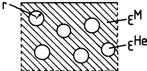
Fig. 2.3 Modell eines Metalls mit der dielektrischen Funktion \epsilon^M und eingebettete, kugelförmige He-Blasen mit der dielektrischen Funktion \epsilon^{He} . r = Blasenradius.
