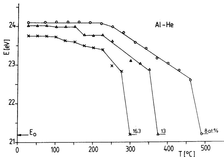
Fig. 4.13 Temperaturabhängigkeit der He 1^1S_0 - 2^1P_1 -Übergangsenergie von 1000 Å-dicken Al-Schichten für verschiedene He-Konzentrationen. E_0 = 21.23 eV = atomare Übergangsenergie. Die Temperzeit pro Meßpunkt betrug immer 20 min.
