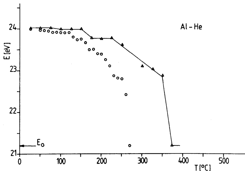
Fig. 4.14 Temperaturabhängigkeit der He 1^1S_0 - 2^1P_1 -Übergangsenergie von 1000 Å-dicken Al-Schichten mit C_{\text{He}} = 13 at.-% für Temperschnitte von \Delta T = 25^\circ\text{C} ( \Delta ) und \Delta T = 10^\circ\text{C} (o).
