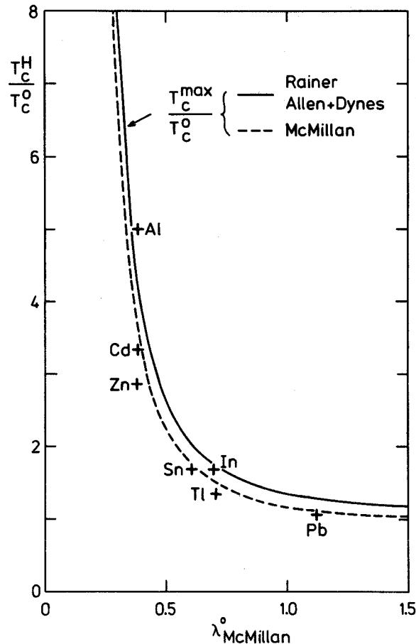
Abb. 15 Experimentell ermittelte Werte von T_C^H/T_C^0 als Funktion von \lambda_{McMillan}^0 des Ausgangsmaterials im Vergleich mit T_C^{max}/T_C^0 nach den Gleichungen von McMillan bzw. Rainer und Allen und Dynes
