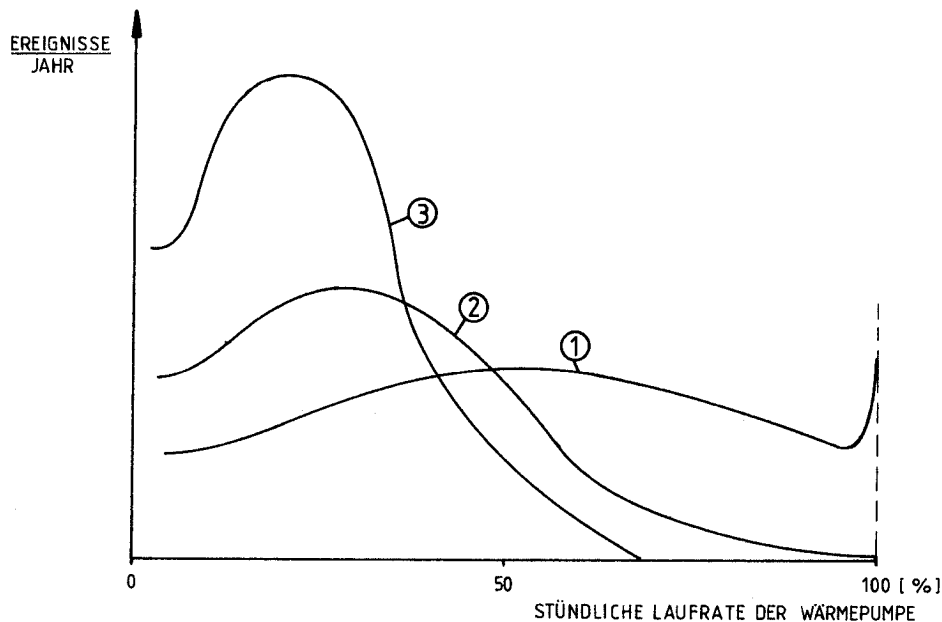
Abb. 4.31: Qualitative Häufigkeitsverteilung der Wärmepumpenlaufzeiten für Stundenintervalle verschiedener Auslegungsfälle.
