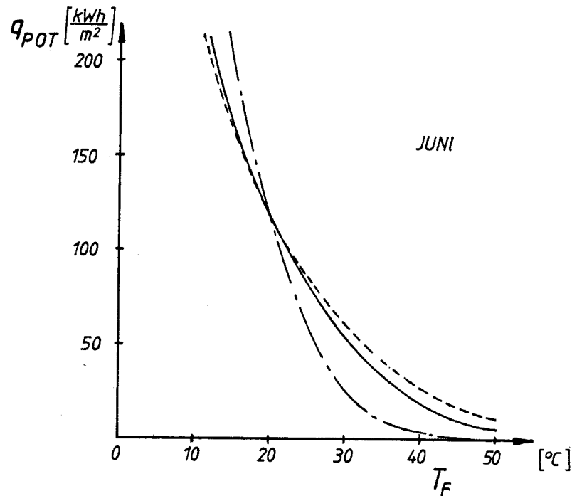
Abb. 3.8: Energiepotential verschiedener Energieabsorber in Abhängigkeit des nutzbaren Temperaturniveaus ( Datenbasis: Hamburg, Juni 1973 ). ————— integrierter Energieabsorber, nicht selektiv - - - - - integrierter Energieabsorber, selektiv - · - · - hinterlüfteter Energieabsorber, nicht selektiv
