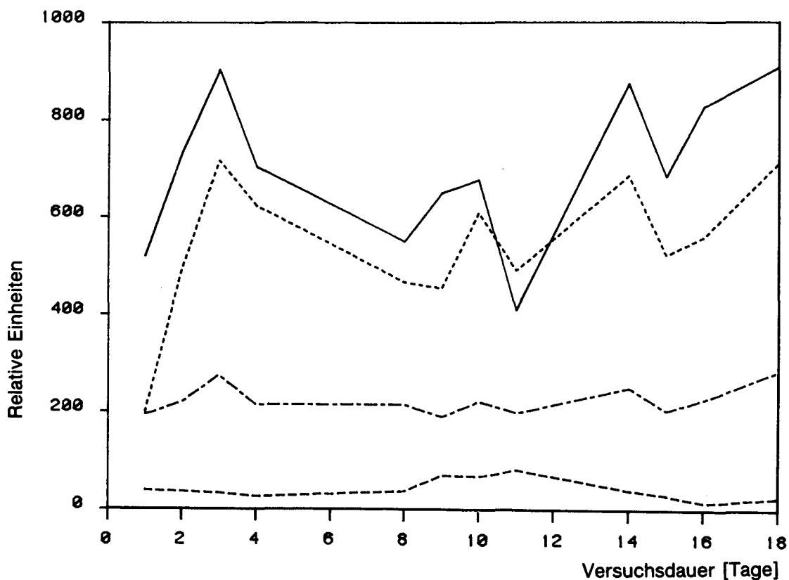
Abb. 32: Licht-limitierte Algenkultur
