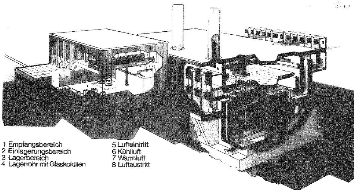
Bild 10-1: Perspektivische Darstellung des Glasblocklagers der DWK /10-1/
