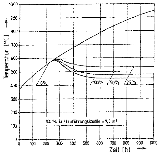
Bild 7-9: Maximale Glastemperatur bei um 240 h verzögerter Inbetriebnahme der Naturkonvektionskühlung mit unterschiedlich großen Zuströmquerschnitten: 100% = 9,3 m 2 , Thermische Leistung = 1100 kW
