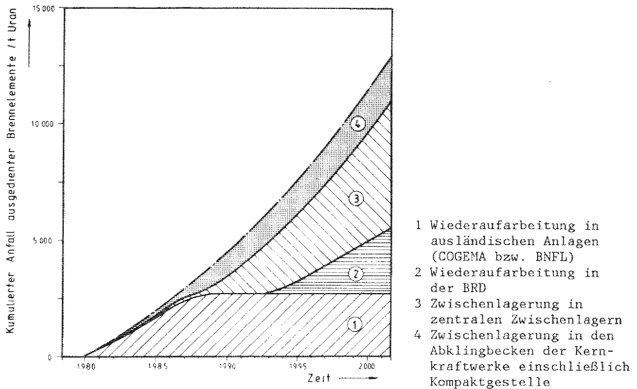
Bild 2-1: Anfall ausgedienter LWR-Brennelemente für installierte Kernkraftwerksleistung von 30 GW(e) bis zum Jahre 2000
