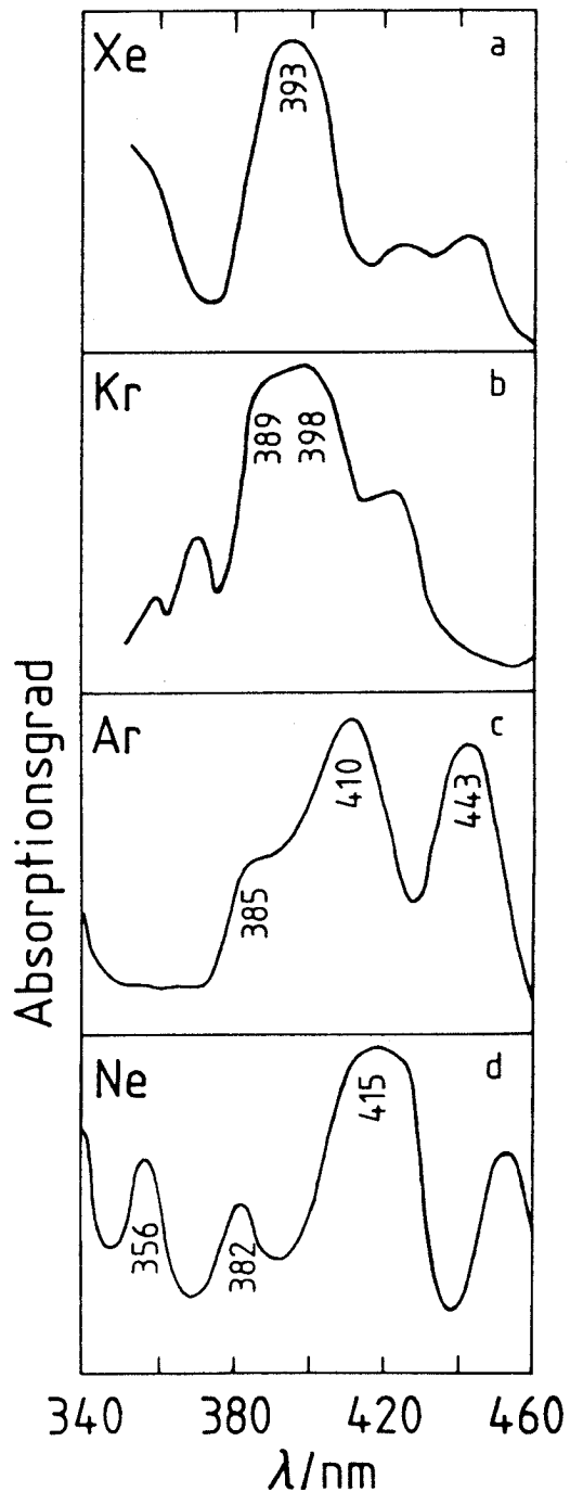
Abb. 4.2: Absorptionsspektren von Silberdimeren isoliert in festen Edelgasen. Die Lagen der Absorptionsbanden ( \lambda/\text{nm} ) sind angegeben. Nicht gekennzeichnete Banden werden höheren Clustern zuge- schrieben. Sie werden später behandelt. Die Zuordnung der Banden bei 443nm in Ar- und bei 356nm in Ne-Matrizen zu \text{Ag}_2 ist in der Literatur umstritten /41,45/.
