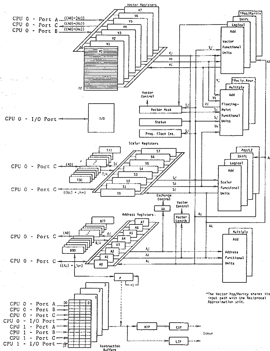
Abb.5.1 eine CPU des Doppelprozessorsystems CRAY X-MP [CRA 82] (Zahlenangaben oktal)
