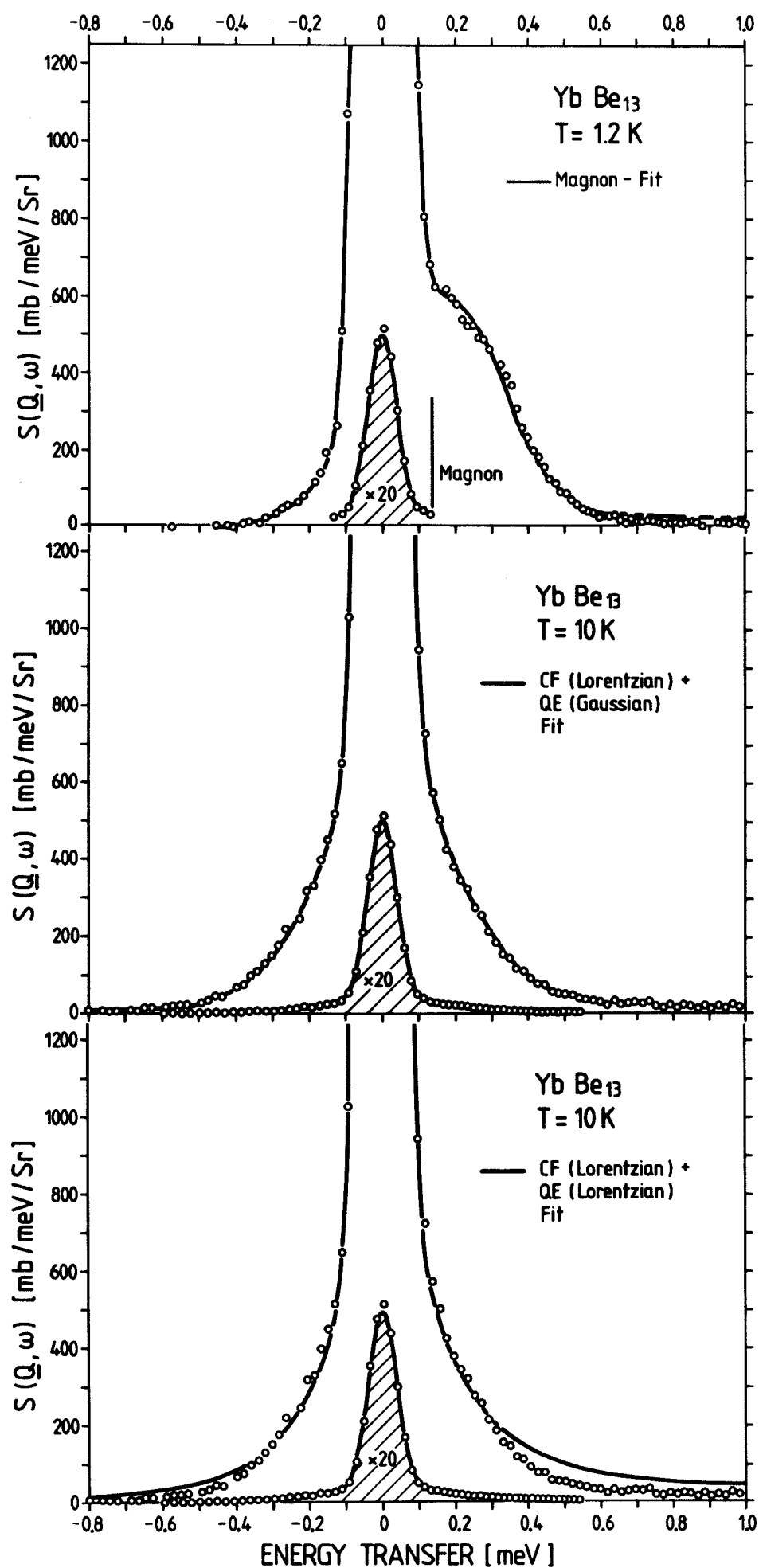
Fig. 3.11. Magnetisches Streuspektrum von YbBe 13 bei T = 1.2 K und 10 K. Die durchgezogene Linie ist bei T = 1.2 K ein Fit an das Spektrum mit einer inelastischen Linie (Magnon). Die beiden Abbildungen bei T = 10 K zeigen den qualitativen Unterschied bei Berücksichtigung einer QE-CF-Linie und einer zusätzlichen quasielastischen Lorentz- bzw. Gaußlinie als kritische Spinfluktuationen.
