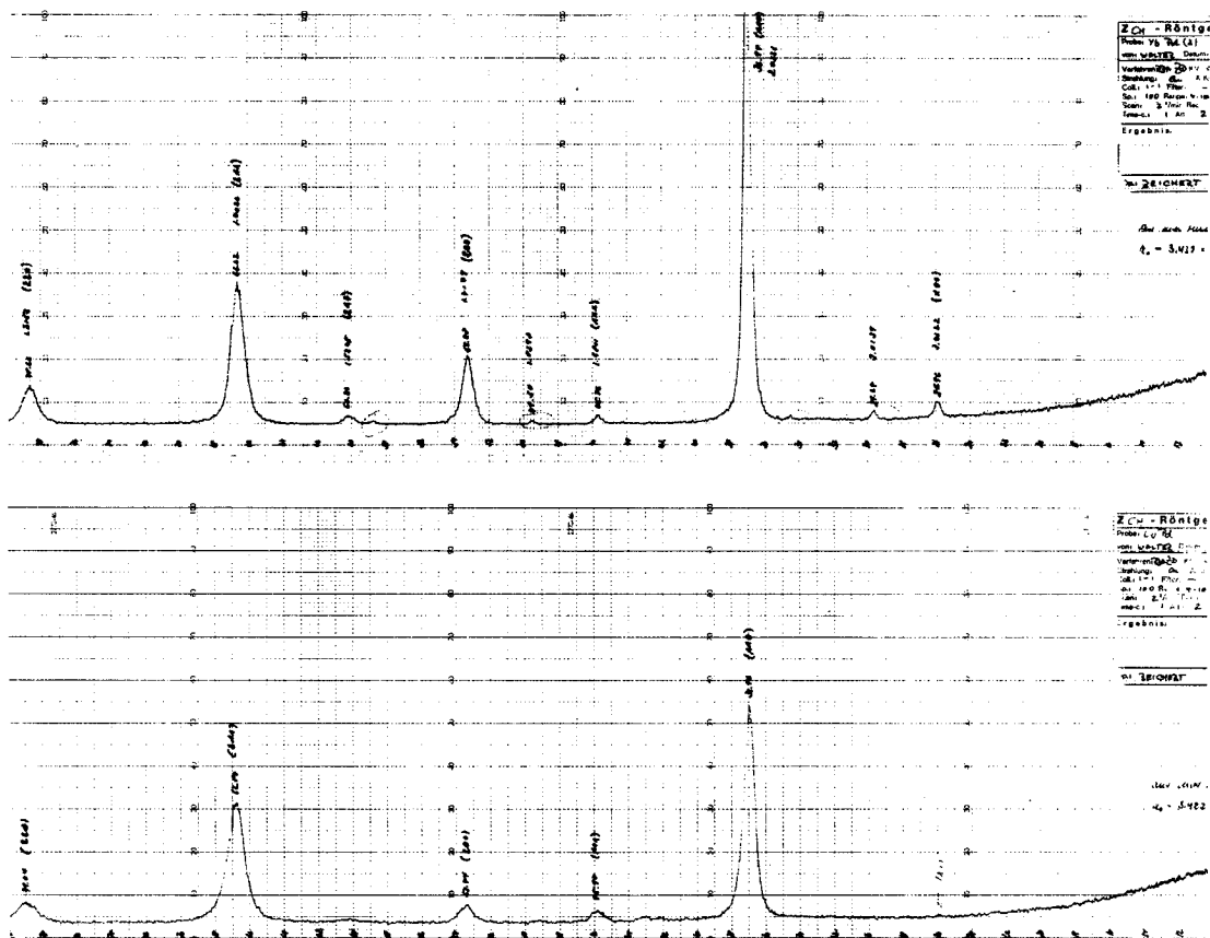
Fig. 3.17. Röntgendiffraktometrieaufnahmen von YbPd (oben) und LuPd (unten)
