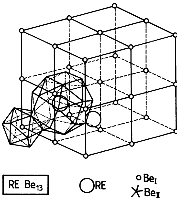
Fig. 3.5. Kristallstruktur von REBe 13
