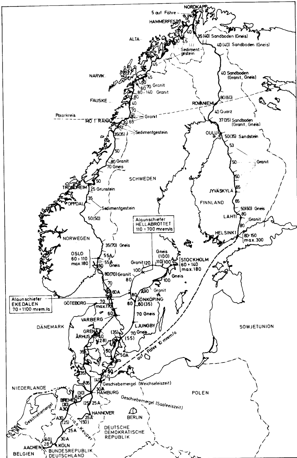
Abb. 3 : Ortsdosisleistung durch terrestrische Strahlung auf Straßen in Norddeutschland, Dänemark, Schweden, Norwegen, Finnland in mrem/a im Jahre 1979, Abschirmung durch das Auto etwa 10 % ( ) gemessene Werte abseits von der Straße A Autobahn
