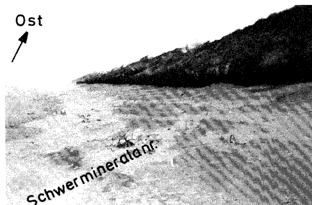
Abb. 11.6: wie Abb. 11.5, jedoch weiter westlich
