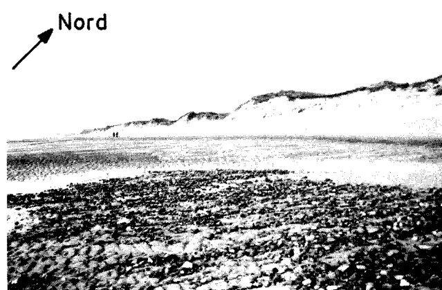
Abb. 19.29: Steine aus der Moräne der Südspitze von Sylt im Jahre 1980
