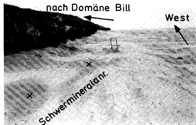
Abb. 11.7: etwa wie Abb. 11.6, jedoch westlich
