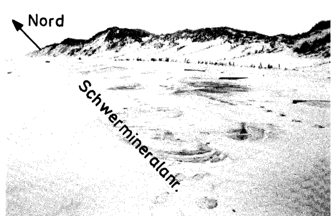
Abb. 19.7: wie Abb. 19.3, jedoch weiter nördlich
