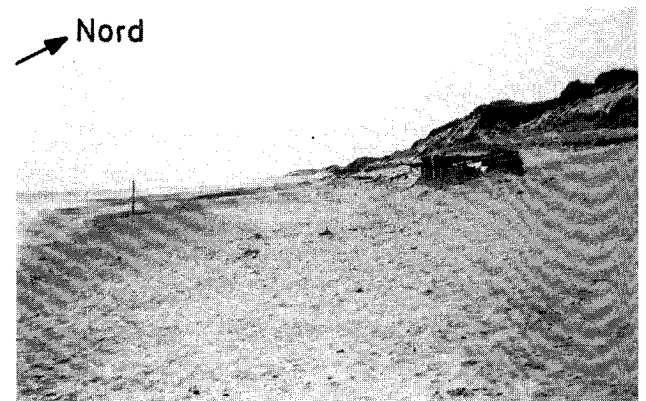
Abb. 19.25: wie Abb. 19.23, jedoch weiter nördlich
