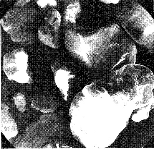
Abb. 40.1: Heller Sand Ke 2 in Tab. 3 unter einem Elektronenmikroskop
