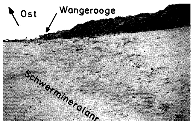
Abb. 16.7: wie Abb. 16.2, jedoch westlich des Ortes Wangerooge
