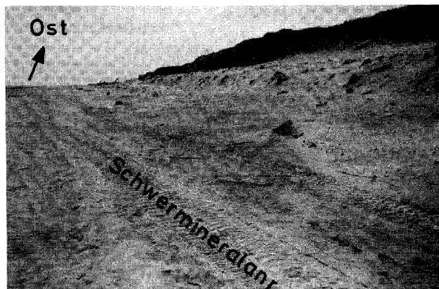
Abb. 16.9: wie Abb. 16.7, jedoch weiter westlich
