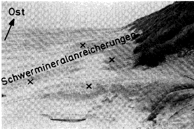
Abb. 11.2: Schwermineralanreicherungen am Weststrand von Juist im Jahre 1979
