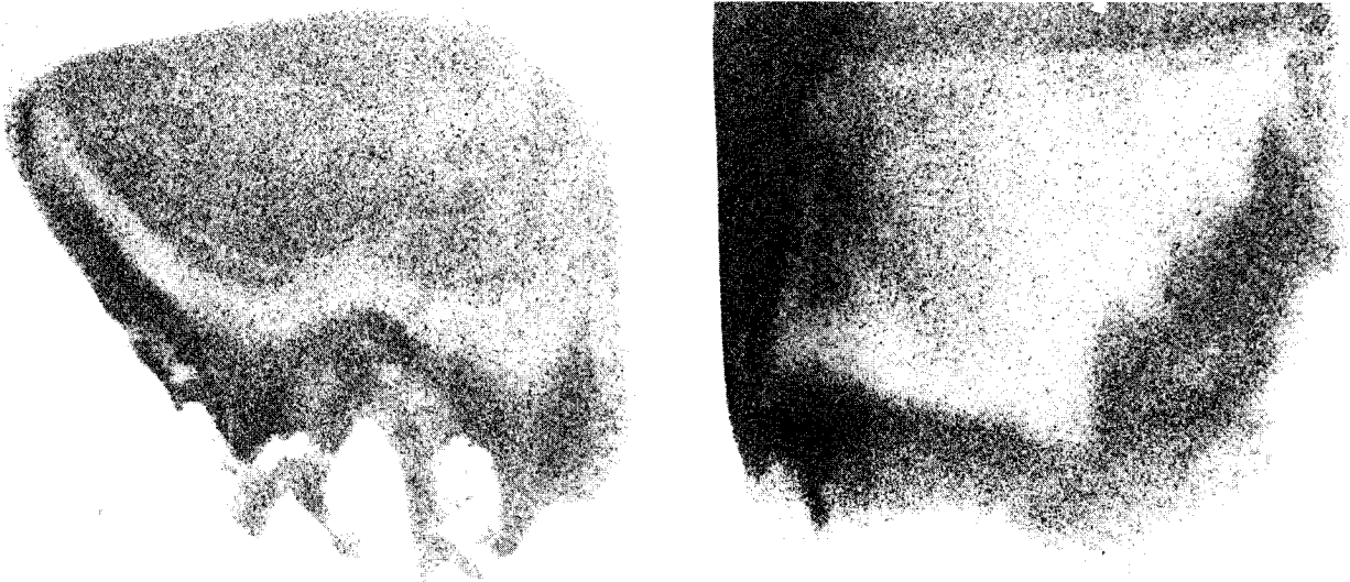
Abb. 31.2: Entmischung des dunklen Sandes bei ruckartiger Bewegung des Papierbodens
