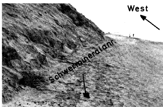
Abb. 12.11: wie Abb. 12.10, jedoch weiter östlich
