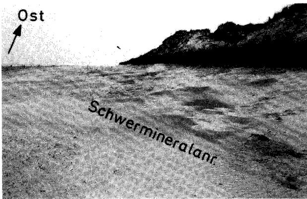
Abb. 12.3: Schwermineralanreicherungen am Stand von Norderney im Jahre 1978
