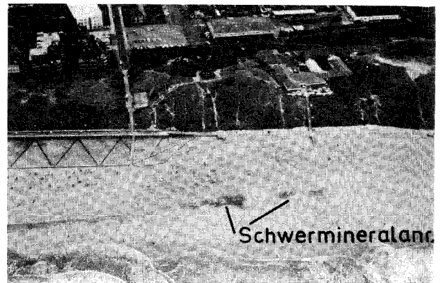
Abb. 19.9: wie Abb. 19.8 , jedoch weiter südlich Freigeg. v. Reg.Präs. Düsseldorf Nr. OL 850
