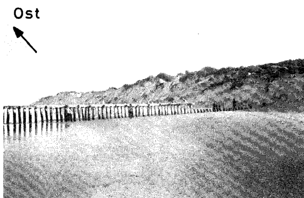
Abb. 12.13: wie Abb. 12.5 im Jahre 1980
