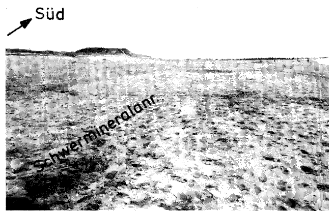
Abb. 19.33: wie Abb. 19.30, jedoch südlich des Dünenüberganges
