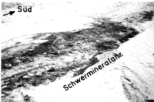
Abb. 19.4: Ausschnitt aus dem Bereich um Abb. 19.3
