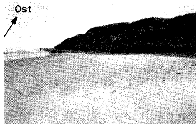
Abb. 12.6: wie Abb. 12.5, nach der Buhne
