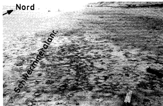
Abb. 19.17: Schwermineralanreicherungen südlich des Erholungsheims Klappholtal auf Sylt im Jahre 1980
