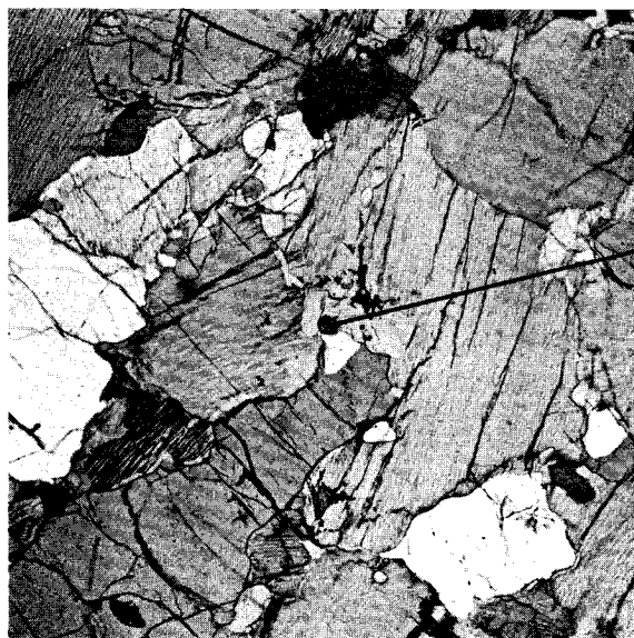
Abb. 30: Durchlichtaufnahme eines 30 \mu\text{m} dicken Granit-Scheibchens mit einem Zirkonsilicat-Kristall ( \text{ZrSiO}_4 ) in der Mitte nach /De 80/
