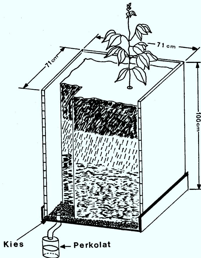
Abb. 3: Lysimeter mit eingefülltem Krümenboden.
