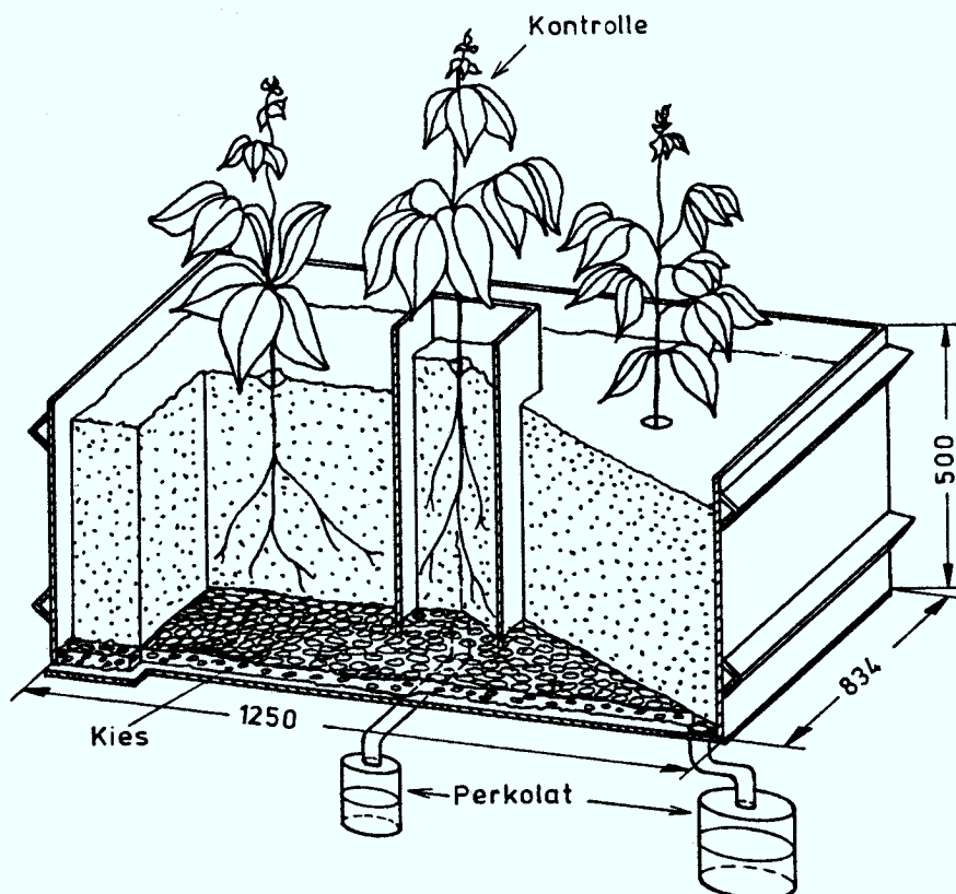
Abb. 3: Lysimeter mit eingefülltem Krümenboden.
