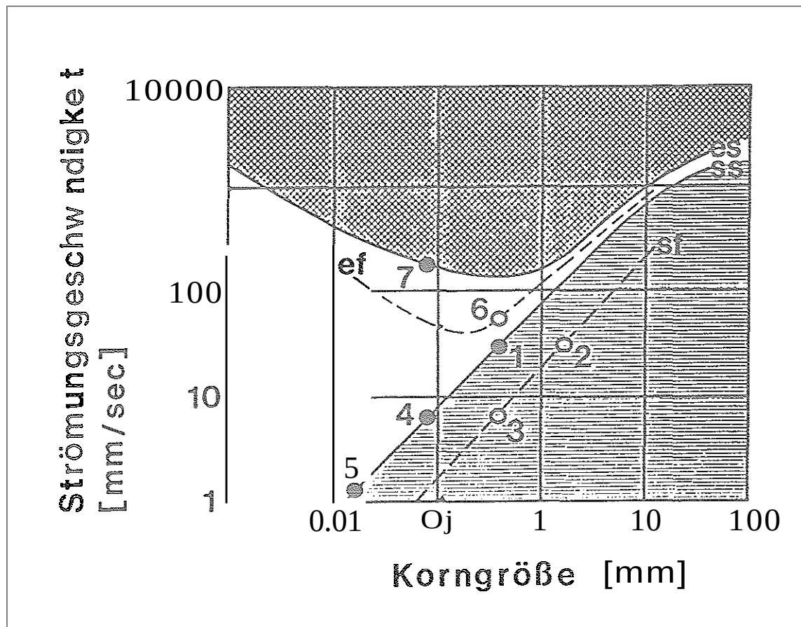
Abbildung 69. Erosions-Transport-Sedimentations-Diagramm
