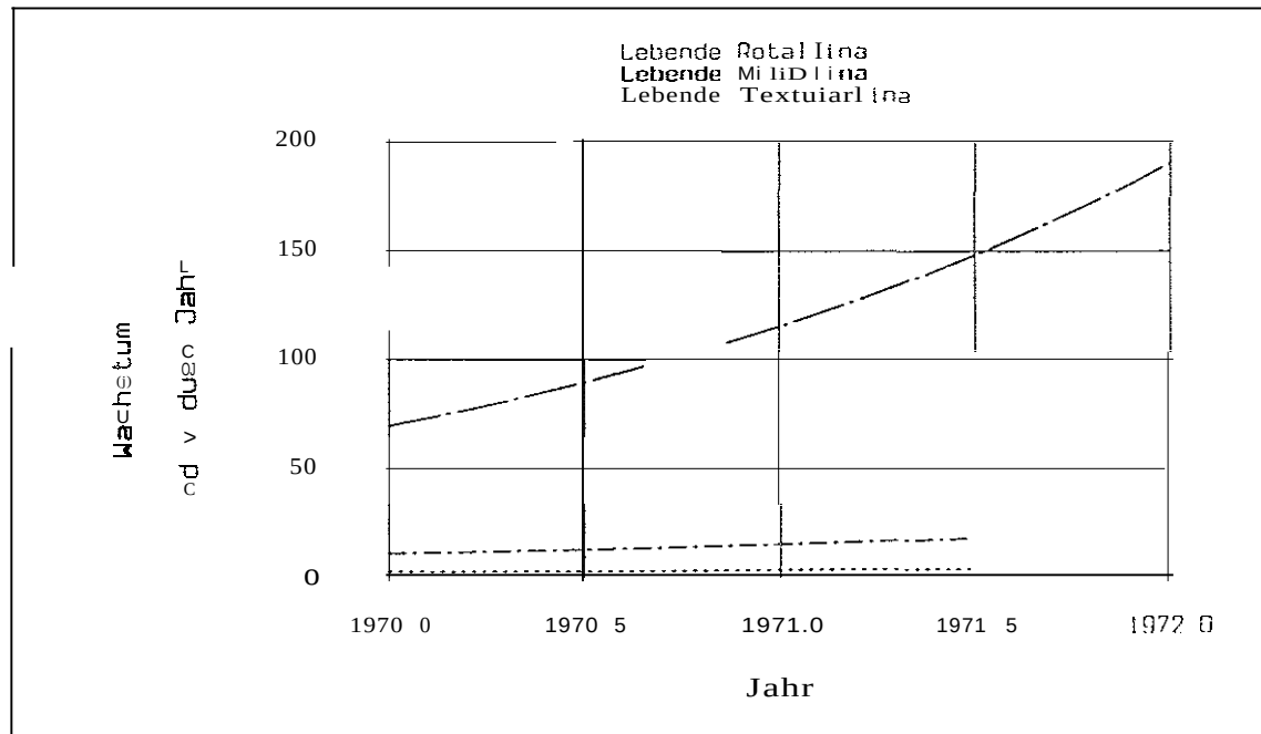
Abbildung 8. Wachstum der Populationen in Beispiel 2
