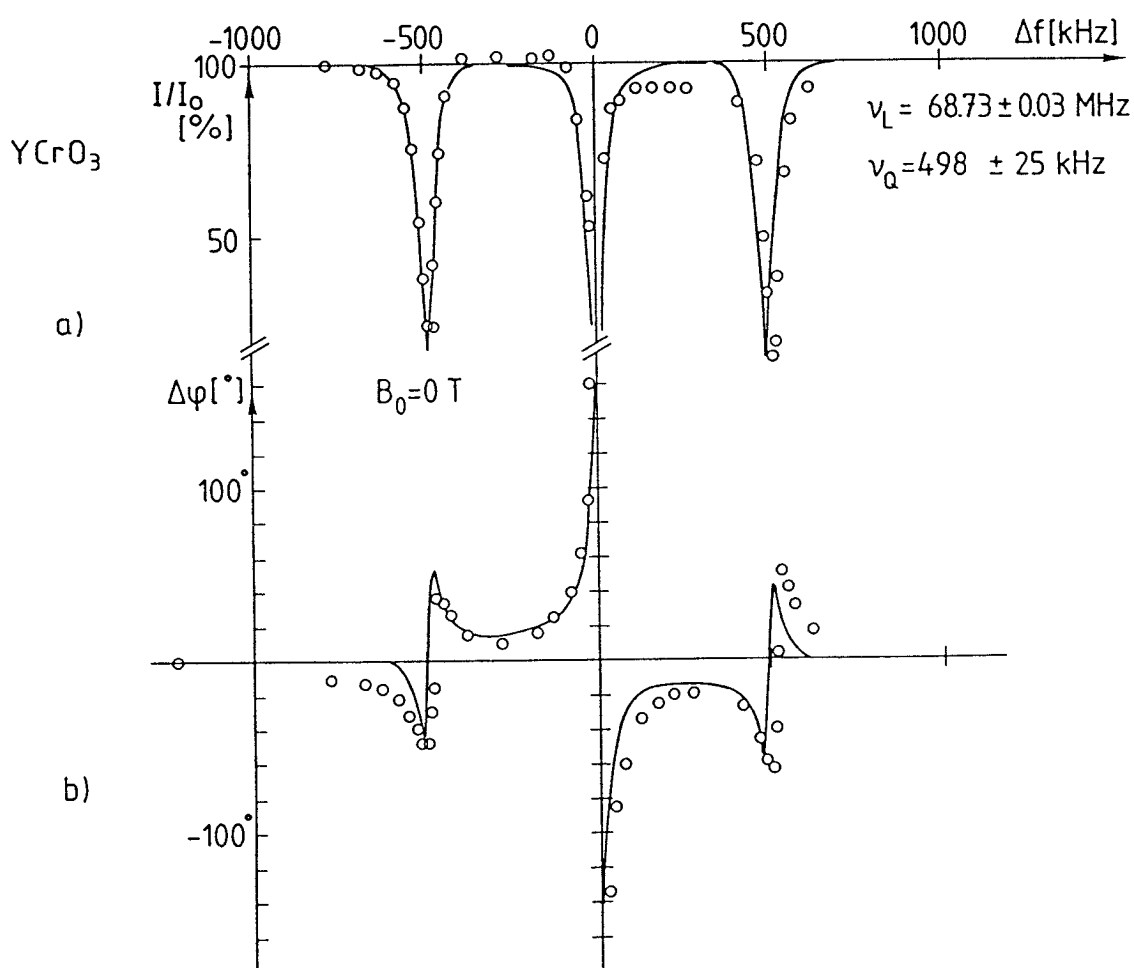
Abb. 3.4 : Amplitude (oben) und Phase (unten) der Zentralkomponente der Cr- Resonanz in \text{YCrO}_3 in einem Doppelresonanzexperiment nach dem zweiten Verfahren. Die Linien ergeben sich aus einer Simulation des Experiments.
