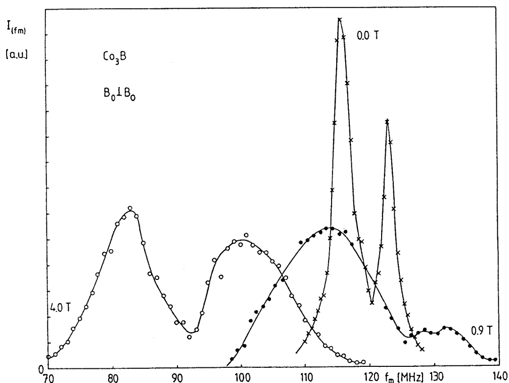
Abb. 2.7 : Co Spin- Echo Spektren in \text{Co}_3\text{B} ohne Feld (x), bei 0,9 T und bei 4,0 T (●) bzw (o) senkrecht zum Feld, mit dem die Pulvertextur erzeugt wurde.
