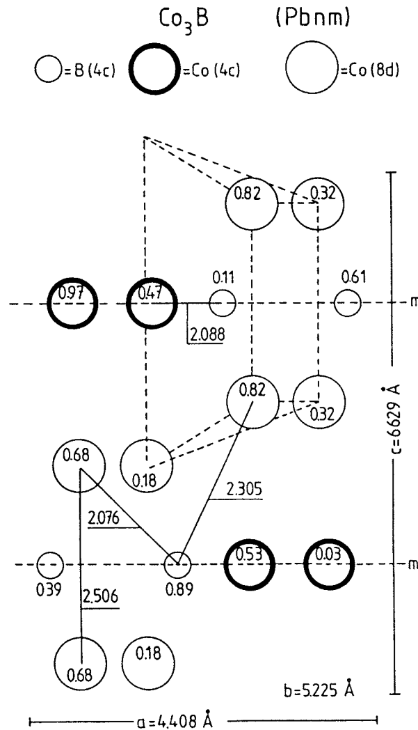
Abb. 2.5 : Projektion der \text{Co}_3\text{B} - Elementarzelle auf die b-Ebene. b- Komponenten in Gittereinheiten, Abstände unterstrichen in Å. Gestrichelt sind die beiden Spiegelebenen m durch die c- Plätze und das Prisma um das B- Atom bei 0,11·b eingetragen.
