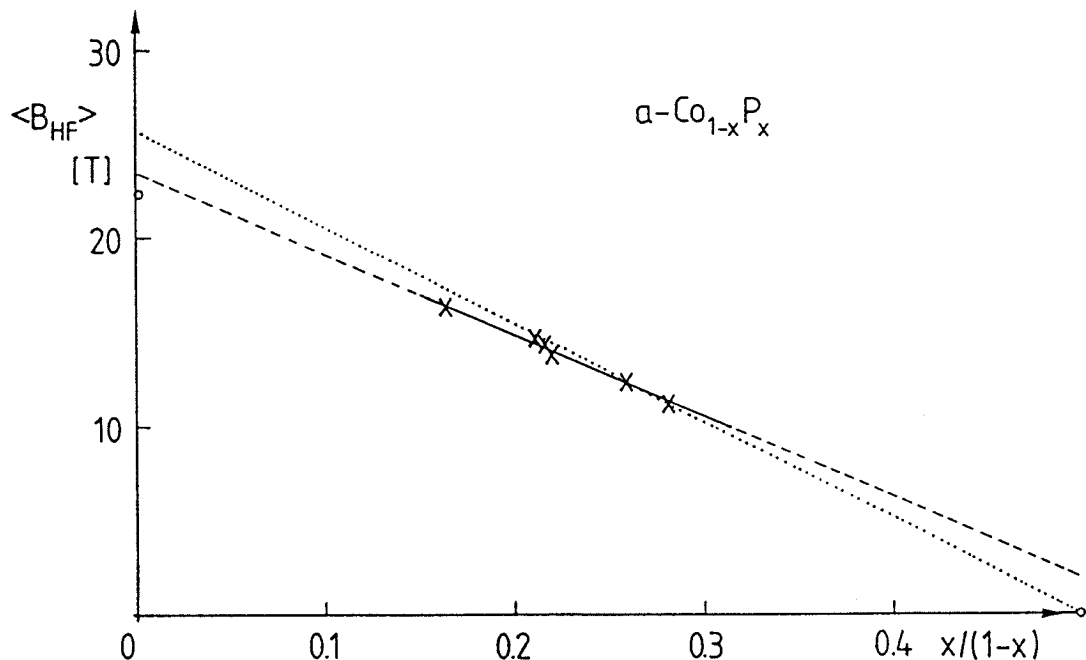
Abb. 2.10 : Mittleres Hyperfeinfeld \langle B_{\text{HF}} \rangle gegen x/(1-x) . Die Kreise entsprechen hcp-Co bzw. \text{Co}_2\text{P} . Die Gerade folgt aus der Anpassung nach Gl. 2.15, die punktierte Linie aus 2.19.
