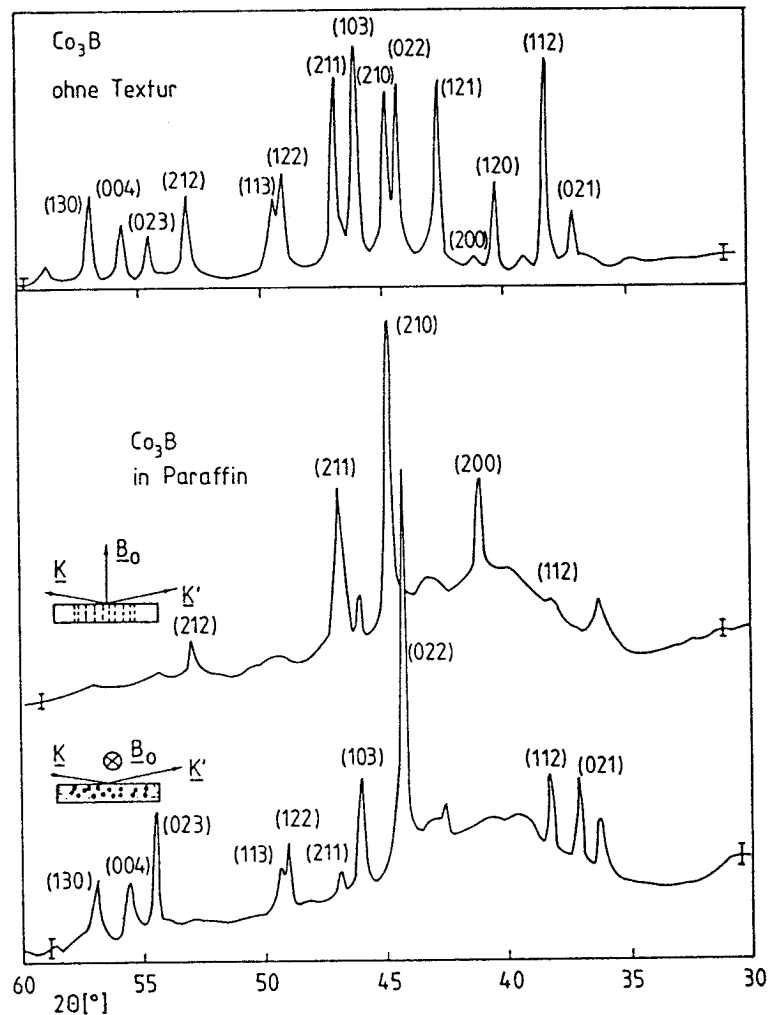
Abb. 2.6 : Röntgenbeugungsaufnahmen von \text{Co}_3\text{B} - Pulvern ohne Textur (oben) und mit Textur in Paraffin (unten). Die Balken am Rand geben Rauschamplituden an.
