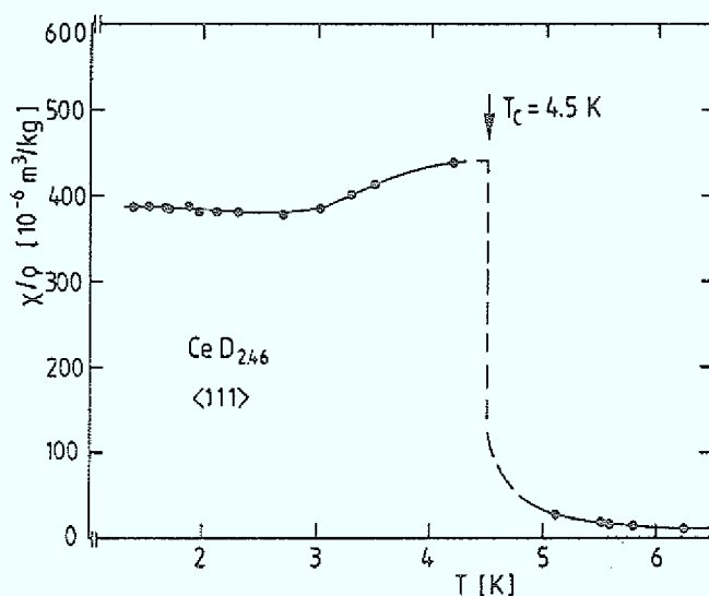
Abb. 4.12: Suszeptibilität von \text{CeD}_{2,46} , aufgetragen gegen die Temperatur.
