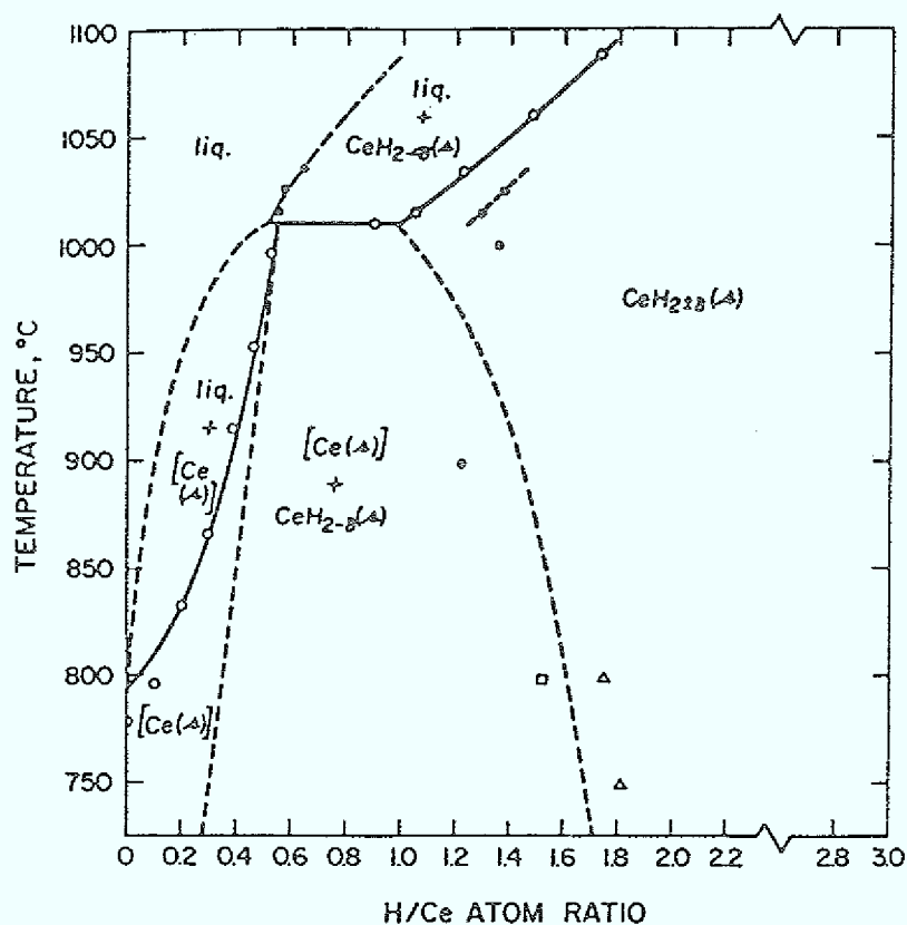
Abb. 2.1: Phasendiagramm von Ce Hydrid nach Libowitz [LP67]
