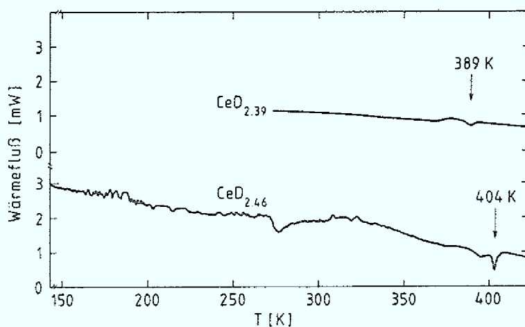
Abb. 4.24: DTA-Messung von \text{CeD}_{2,39} und \text{CeD}_{2,46} . Beide Proben zeigen einen Übergang bei 389 bzw. 404 K.
