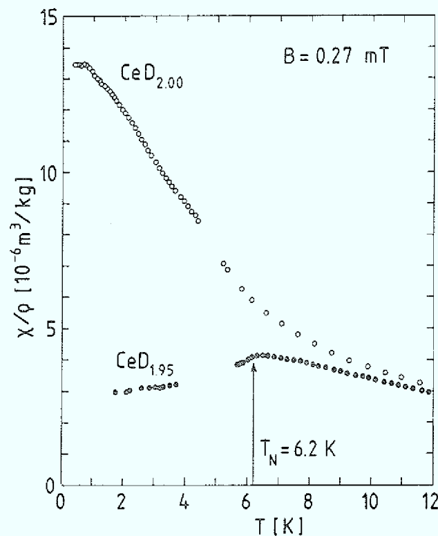
Abb. 4.1: Suszeptibilität von \text{CeD}_{1,95} bzw. \text{CeD}_{1,97} (●) und \text{CeD}_{2,00} (○), gemessen in B = 0,27 \text{ mT} und aufgetragen gegen die Temperatur. \text{CeD}_{1,95} zeigt bei T = 6,2 \text{ K} seine Neél-Temperatur, \text{CeD}_{2,00} ordnet bis hinab zu 0,7 \text{ K} nicht. Der flache Verlauf unterhalb von 0,7 \text{ K} wird in Abschnitt 5.1 diskutiert.
