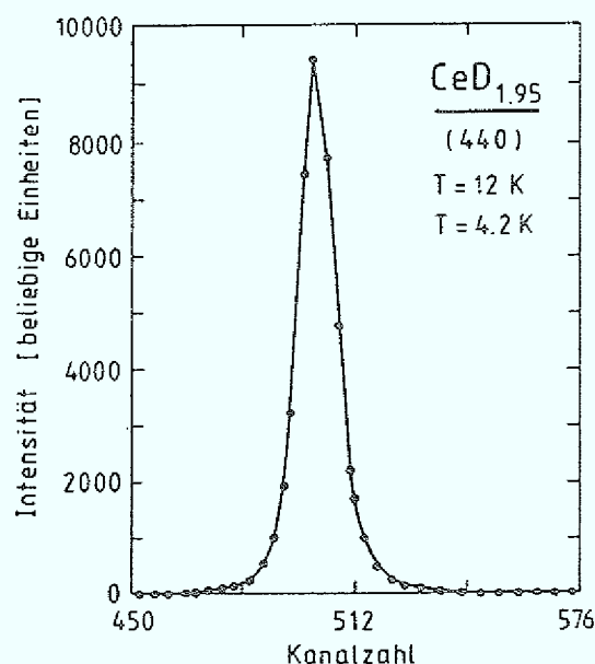
Abb. 4.27: (440)-Reflex von \text{CeD}_{1,95} , gemessen mit Röntgen-Diffraktometrie bei T = 12 und 4,2 \text{ K} . Der Reflex bleibt scharf und spaltet nicht auf, d.h. die Probe bleibt bis zur tiefsten Temperatur kubisch.
