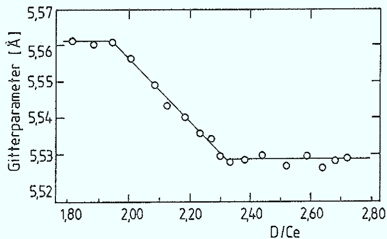
Abb. 4.2: Gitterparameter bei Raumtemperatur von Ce Deuterid als Funktion der Konzentration [KM82].
