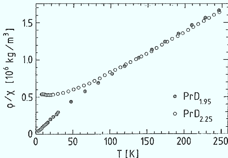
Abb. 4.20: Die reziproke Suszeptibilität von \text{PrD}_{1,95} (●) und \text{PrD}_{2,25} (○), gemessen in B = 1 \text{ T} , zeigt den Übergang von magnetischem Grundzustand in \text{PrD}_{1,95} zu dem Van Vleck-induzierten Paramagneten \text{PrD}_{2,25}
