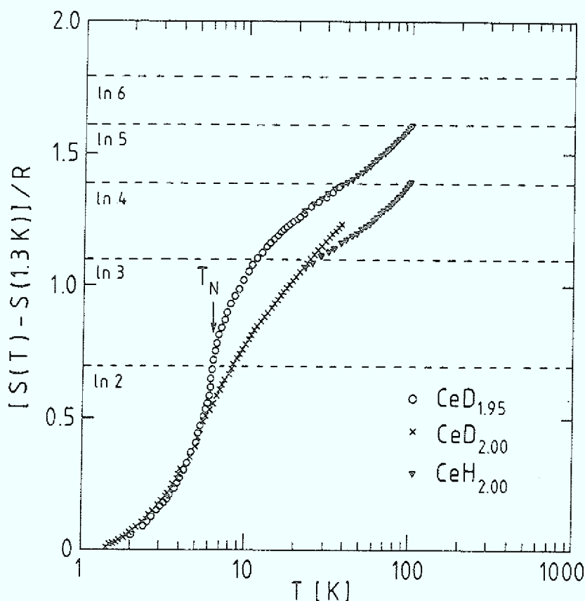
Abb. 5.16: Entropie von CeD_{1.95} ( \circ ) und CeD_{2.00} ( \times ) nach Abzug der spezifischen Wärme von LaH_{2.00} [B71].
