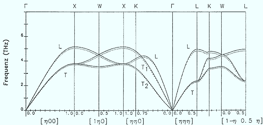
Abbildung 15. Phononendispersionskurven von kfcz-Kalzium bei T=100\text{K} (—) und T=293\text{K} (···)
