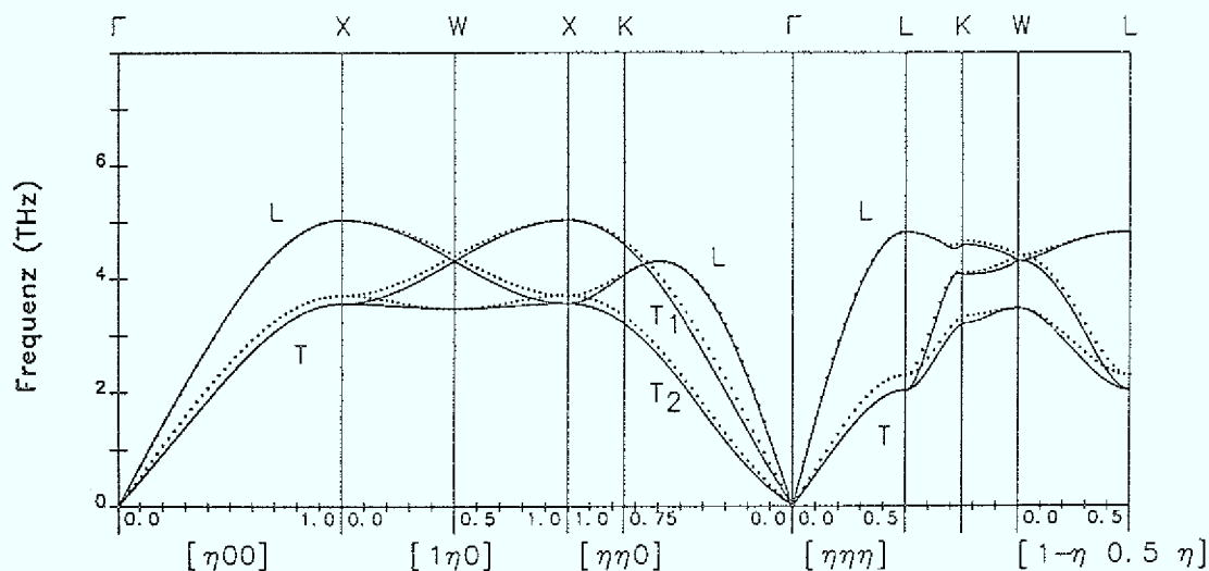
Abbildung 16. Phononendispersionskurven von kfcz-Kalzium bei T=705\text{K} (—) und T=293\text{K} (···)
