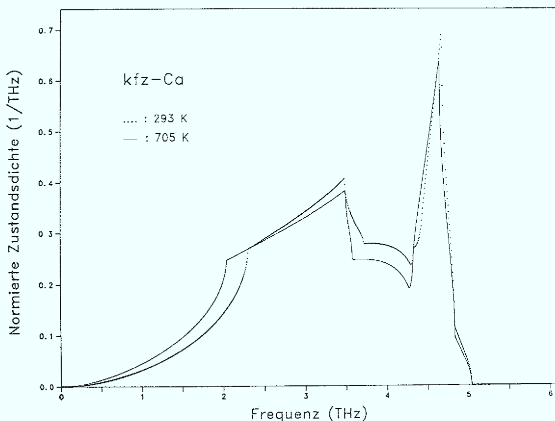
Abbildung 23. Normierte Phononenzustandsdichte von kfz-Kalzium, berechnet mit den BvK-Parametern aus Tabelle II. ( ... : T = 293 \text{ K} ; — : T = 705 \text{ K} )
