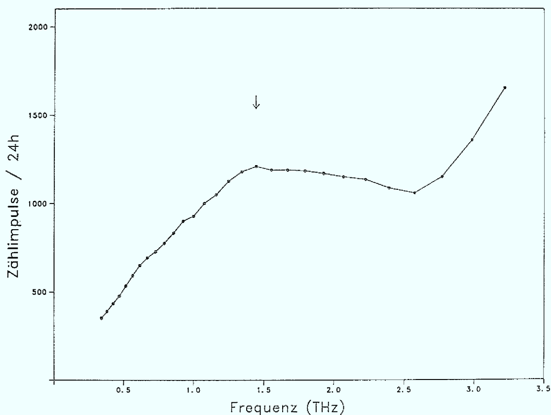
Abbildung 30. Inelastische Neutronenstreudaten von krx-Kalzium bei 726K (siehe Text)
