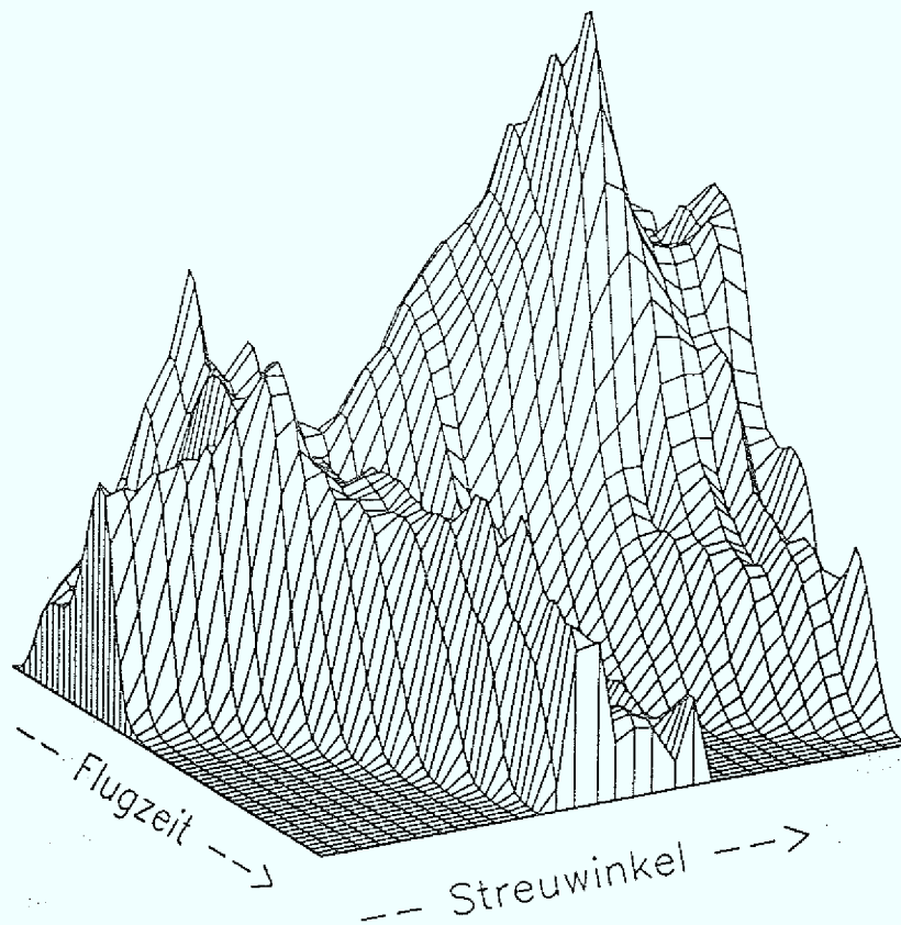
Abbildung 14. Gegenüberstellung der experimentellen (oben) und der theoretischen (unten) Neutronenstreudaten von kfz-Kalzium ( T = 705\text{K} )
