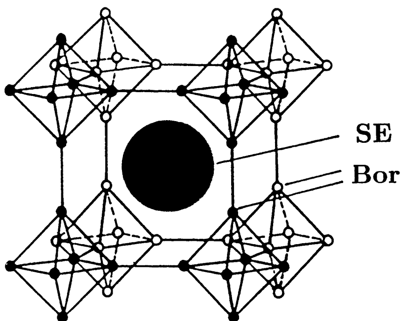
Abb. 2.1 : Die Gitterzelle der SE-Hexaboride
