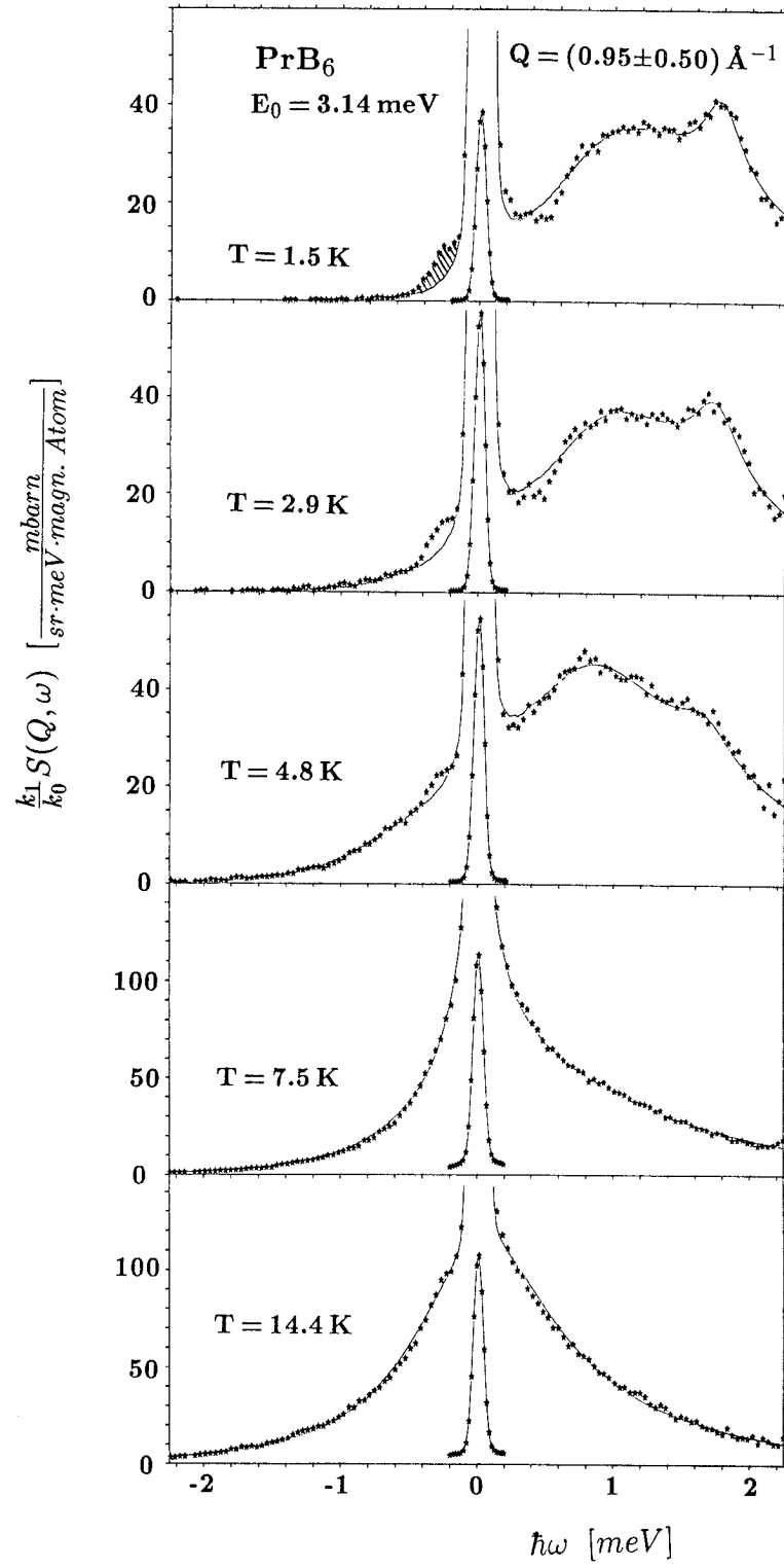
Abb. 4.8: Temperaturabhängigkeit des Anregungsspektrums von PrB 6
