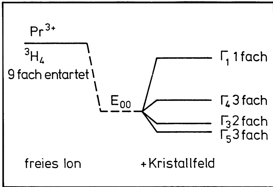
Abb. 2.5: Mögliche Aufspaltung des \text{Pr}^{3+} -Grundzustandes im Kristallfeld
