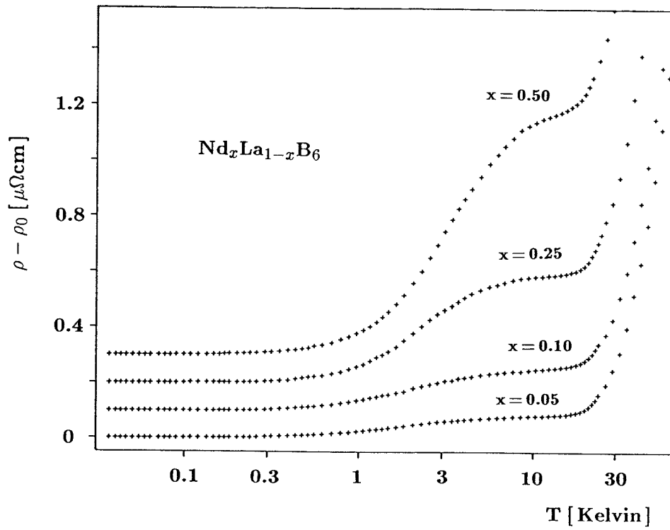
Abb. 4.12: Der spezifische Widerstand von \text{Pr}_x\text{La}_{1-x}\text{B}_6 und \text{Nd}_x\text{La}_{1-x}\text{B}_6 unter Abzug des Restwiderstands mit Nullpunktverschiebung für x \geq 0.10
