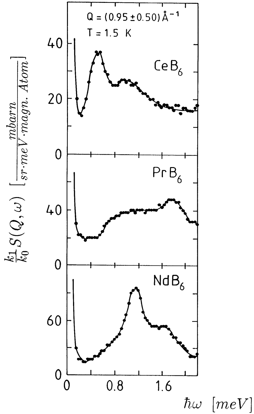
Abb. 4.3 : Niederenergetische Anregungsspektren in CeB 6 , PrB 6 und NdB 6
