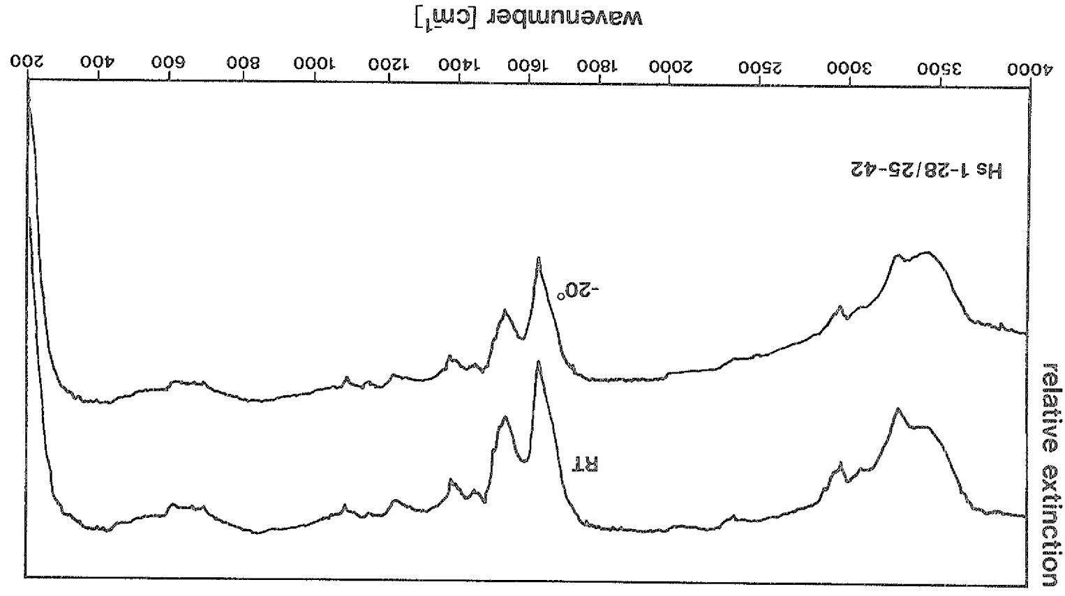
Bild 5.4.16: IR-Spektren der Aggregate 1-28 / 25-42
