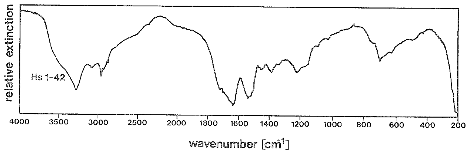
Bild 5.4.11: IR-Spektrum von 1-42
