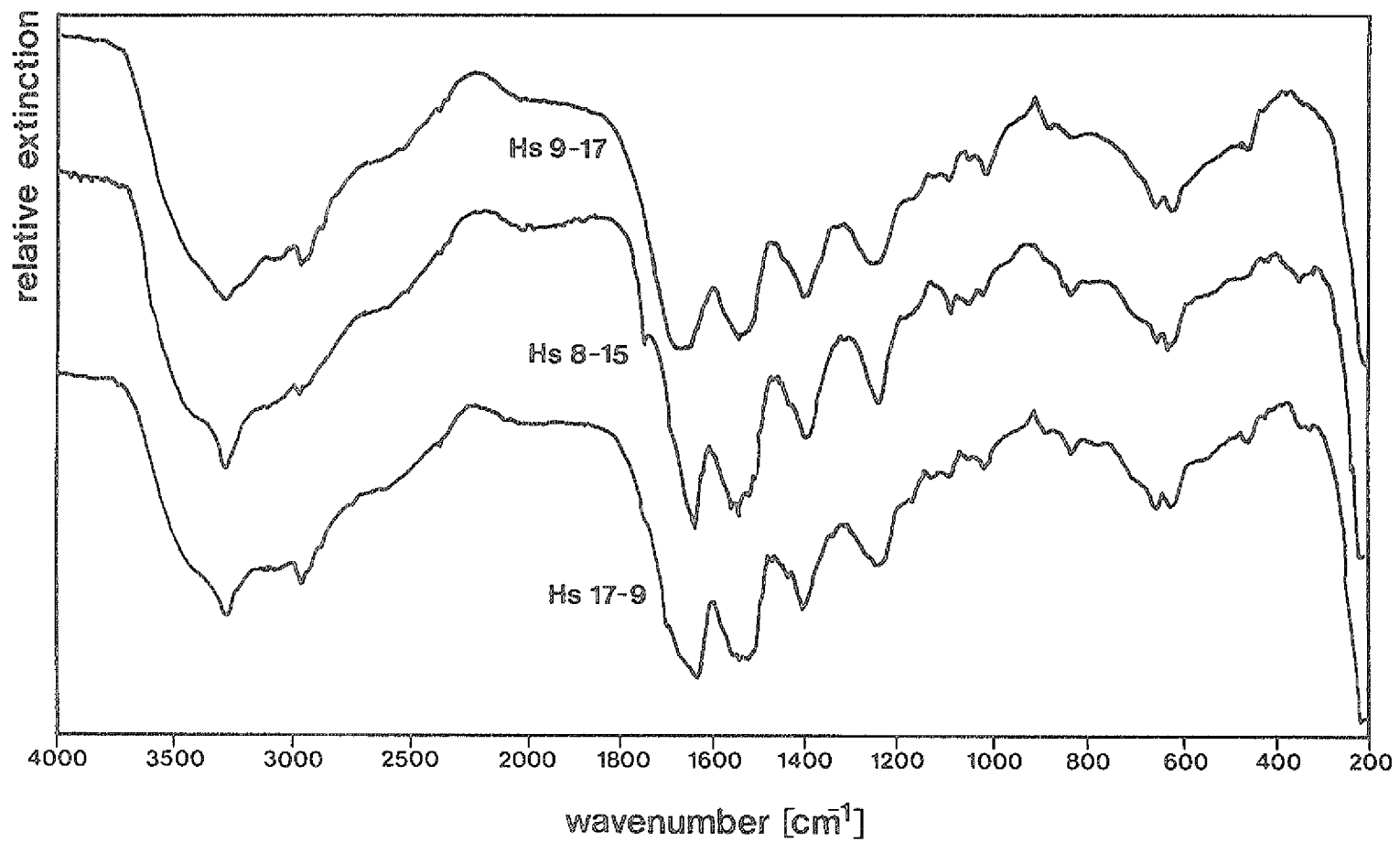
Bild 5.4.6: IR-Spektren von 9-17, 8-15 17-9
