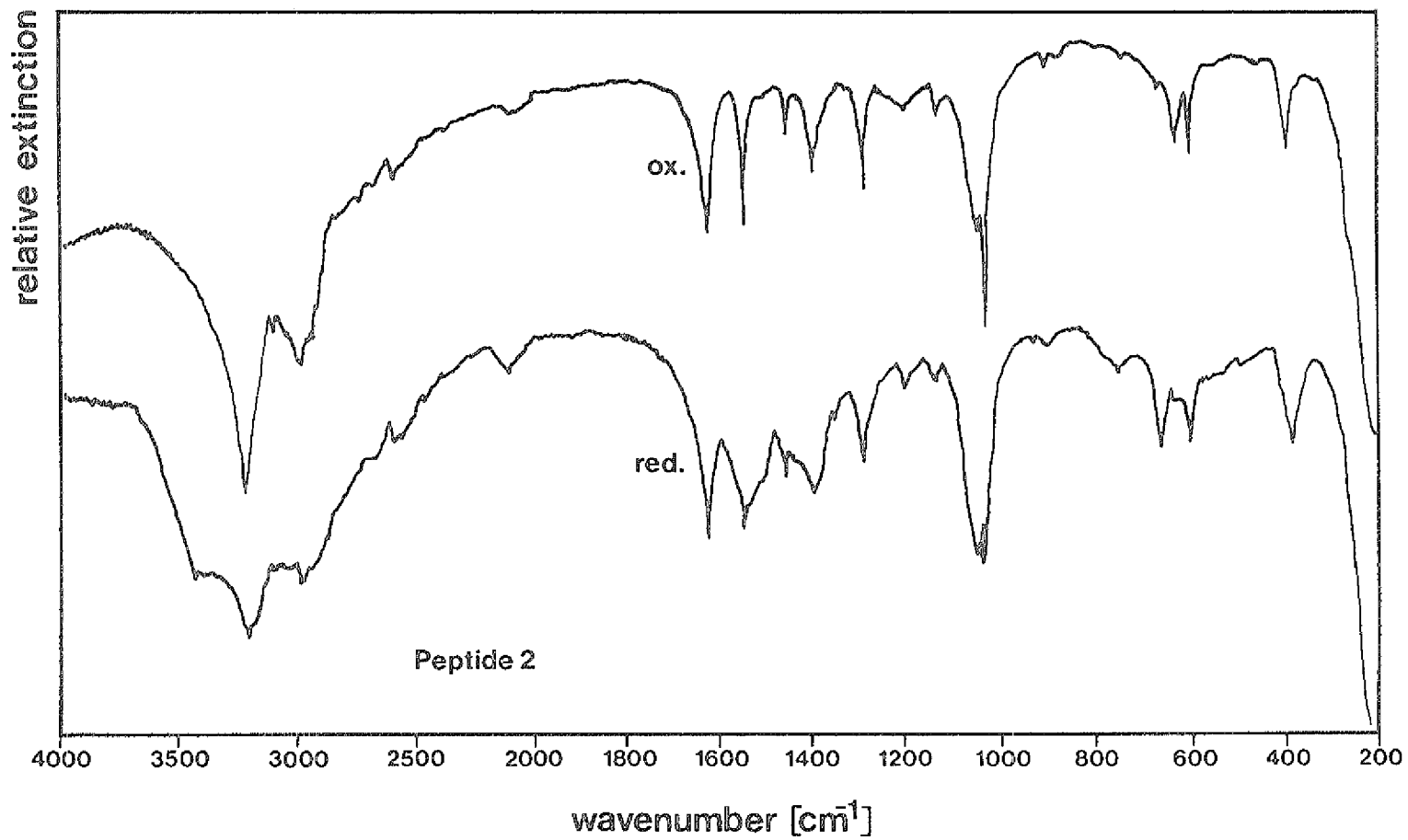
Bild 5.3.7: IR-Spektren des Peptid II a) oxidiert b) reduziert
