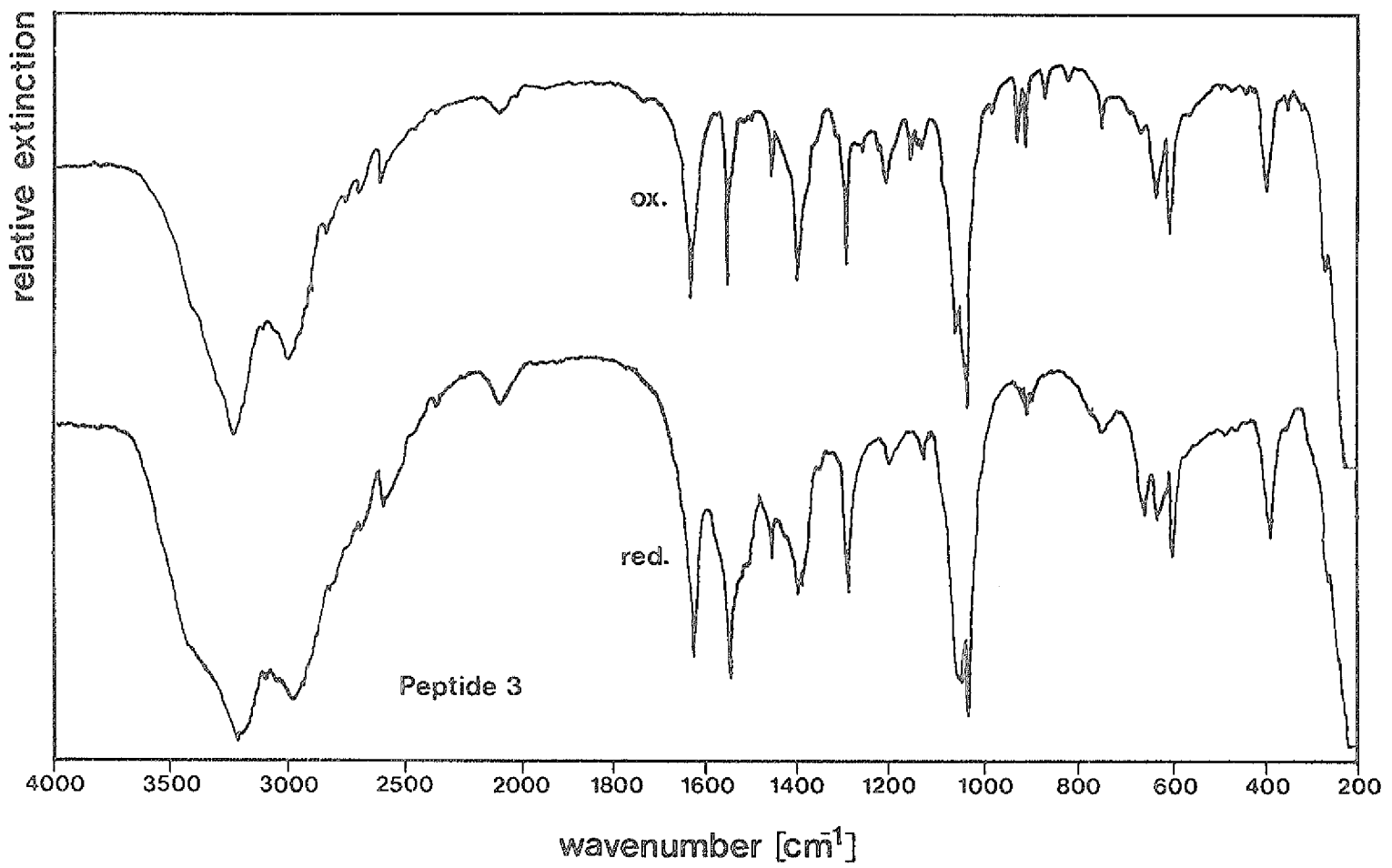
Bild 5.3.9: IR-Spektren des Peptid III
