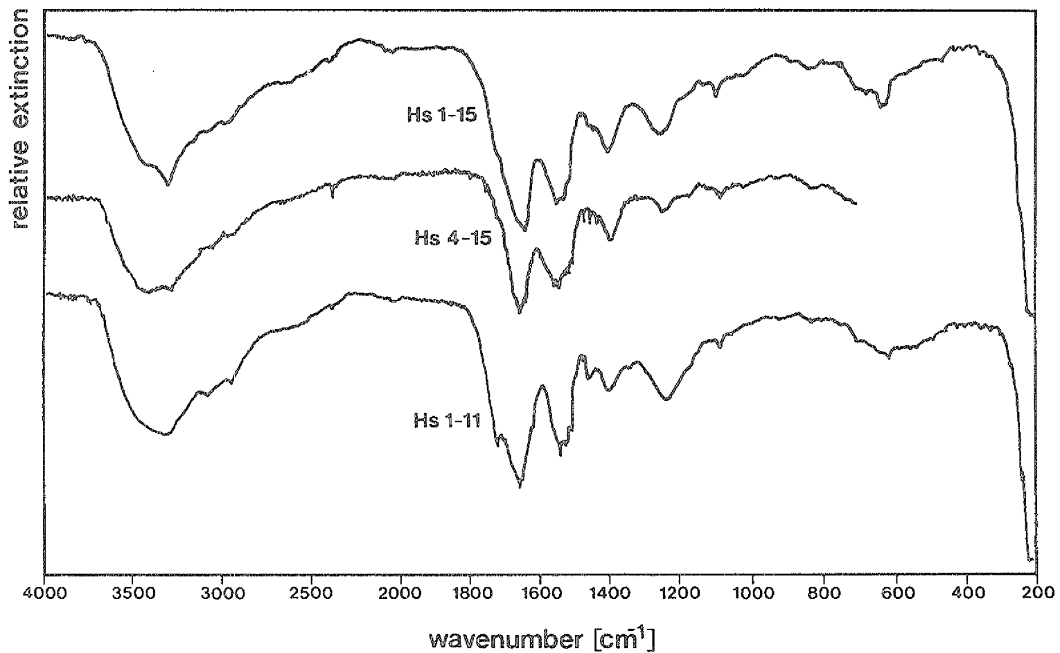
Bild 5.4.5: IR-Spektren von 1-15, 4-15, 1-11
