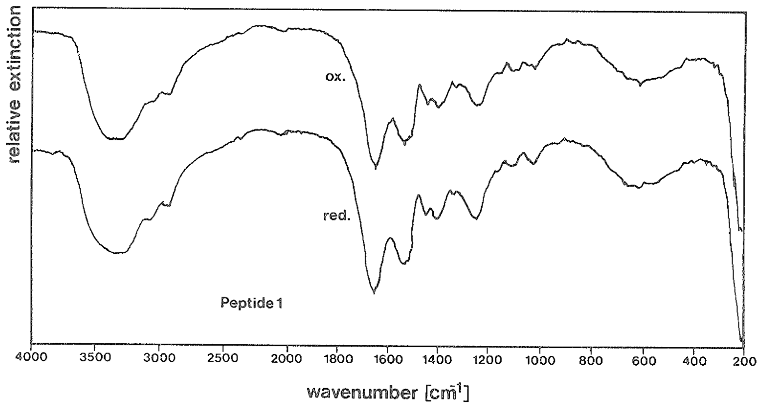
Bild 5.3.6: Vergleich der IR-Spektren des Peptid I a) oxidiert b) reduziert
