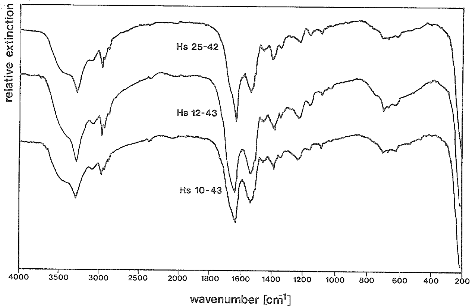
Bild 5.4.10: IR-Spektren von 25-42, 12-43, 10-43
