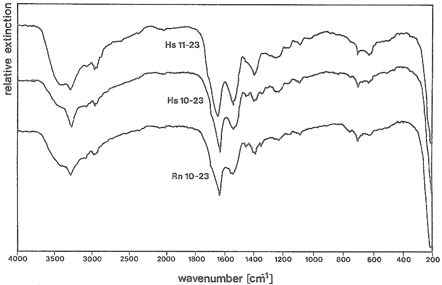
Bild 5.4.7: IR-Spektren von 11-23 (Homo s.), 10-23 \text{NH}_2 (Homo s.), 10-23 \text{NH}_2 (Rattus n.)
