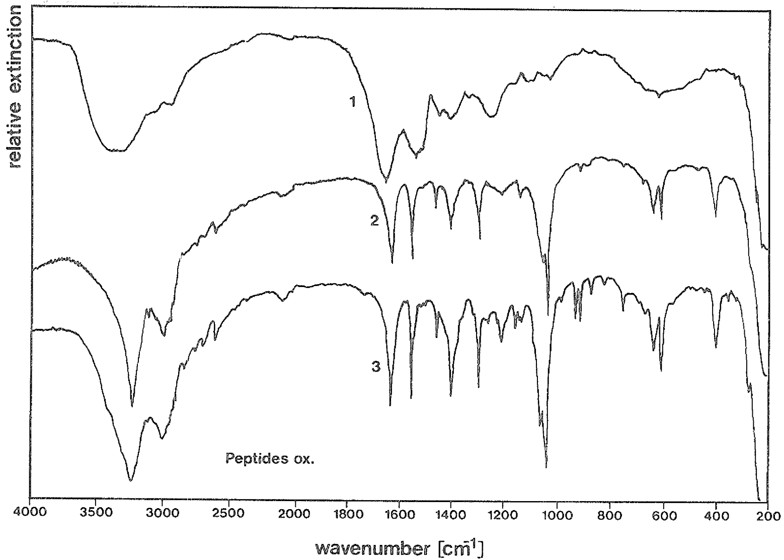
Bild 5.3.5 b): IR-Spektren der oxidierten Formen der Peptide I bis III
