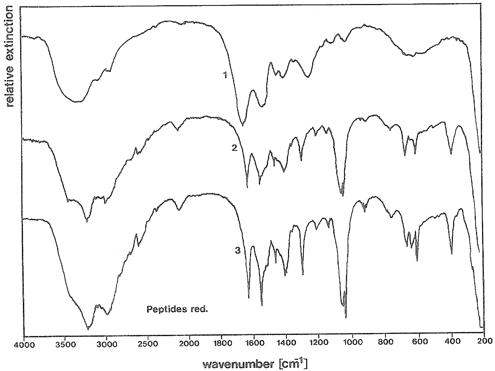
Bild 5.3.5 a): IR-Spektren der reduzierten Formen der Peptide I bis III
