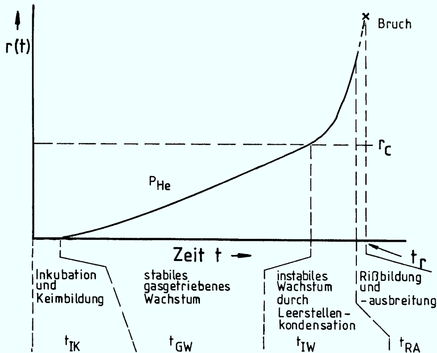
Abb. 32: Zeitabhängigkeit des mittleren Blasenradius während eines "in-beam" Versuchs mit konstanter Heliumimplantationsrate P_{\text{He}} (schematisch). r_c =kritischer Radius
