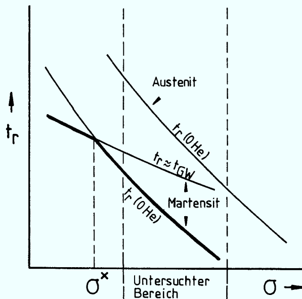
Abb. 34: Bruchzeit gegen Spannung bei Kriechversuchen mit martensitischen und austenitischen Stählen (schematisch). ( t_r(0\text{He}) : Bruchzeit von nicht implantierten Proben; t_{\text{GW}} : Zeitraum des gasgetriebenen stabilen Wachstums)
