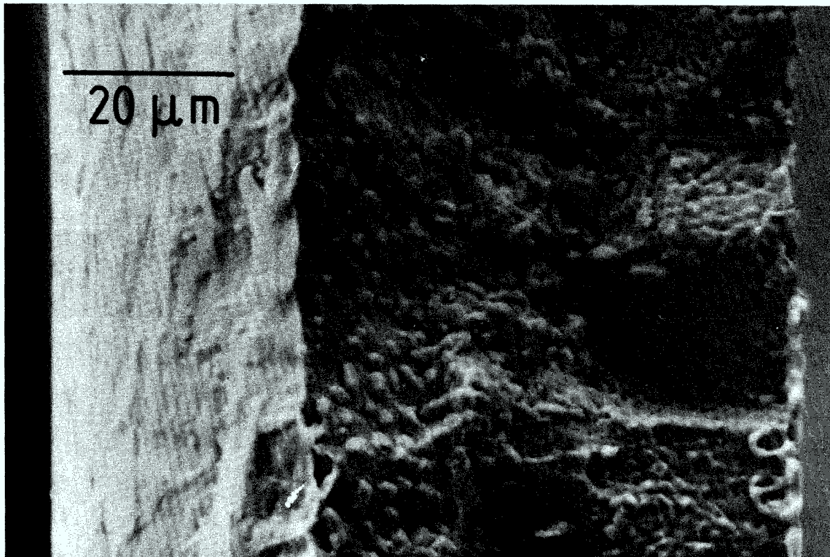
Abb. 22: Bruchfläche (REM-Aufnahme) einer bei Raumtemperatur mit 1000 appm Helium vorimplantierten und bei 873 K und 150 MPa konventionell getesteten Kriechprobe der Vorcharge. Auf einer Seite der Bruchfläche sind Korngrenzen sichtbar.
