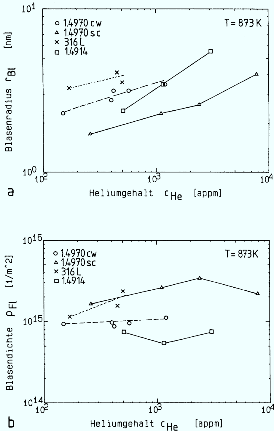
Abb. 33: Vergleich der Heliummikrostrukturdaten (auf Grenzflächen) des Stahls DIN 1.4914 mit denen austenitischer Stähle. "In-beam" Versuche bei 873 K. a) Blasenradien, b) Blasendichten
