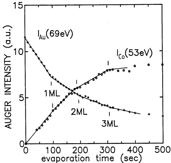
Abb. III.7: Intensität des Augersignals von Co-M_{23}VV und Au-N_{67}VV als Funktion der Aufdampfzeit.
