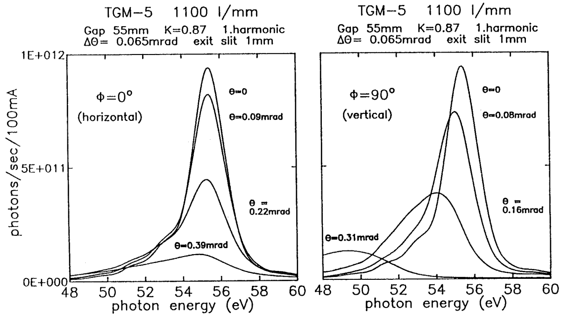
Abb. II.26: Fluß der 1. Harmonischen hinter einer Aperturblende (Öffnungswinkel \theta = 0.065 mrad) in Abhängigkeit vom Polarwinkel für zwei verschiedene Azimuthwinkel: a) \phi = 0^\circ (horizontal) , b) \phi = 90^\circ (vertikal)
