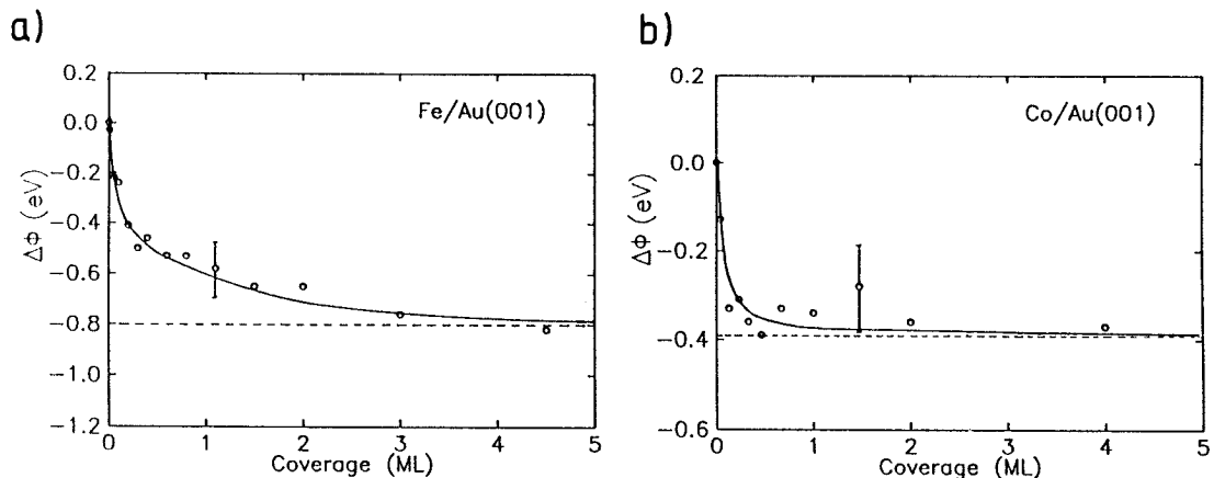
Abb. III.15: Änderung der Austrittsarbeit als Funktion der Schichtdicke für Fe bzw. Co auf Au(001). Die gestrichelte Linie entspricht dem Volumenwert /96,97/.
