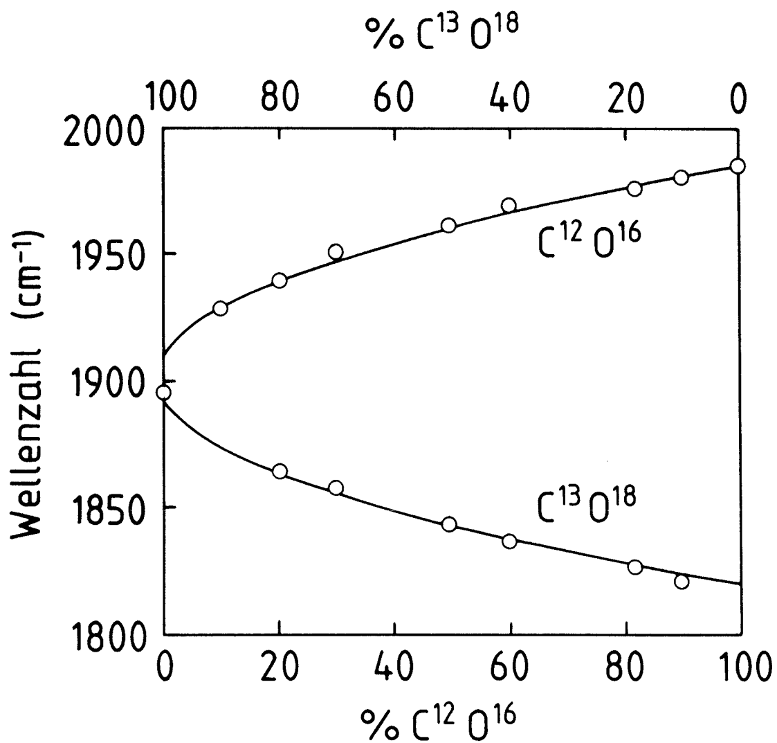
Abb. 6.6: Streckfrequenzen von C^{12}O^{16} und C^{13}O^{18} als Funktion der Isotopenzusammensetzung in der Ni(110)/CO(2x1)-Struktur.
