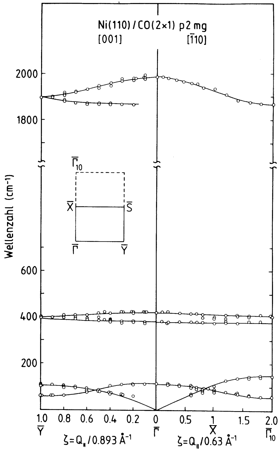
Abb. 6.2: Dispersionskurve der \text{Ni}(110)/\text{CO}(2 \times 1) -Struktur. In \bar{\Gamma}\bar{X} -Richtung ist die erste und zweite Brillouin-Zone der Überstruktur dargestellt. Entlang dieser Richtung werden die geraden Moden bezüglich der Gleitspiegelung nur in der ersten und die ungeraden nur in der zweiten Brillouin-Zone beobachtet.
