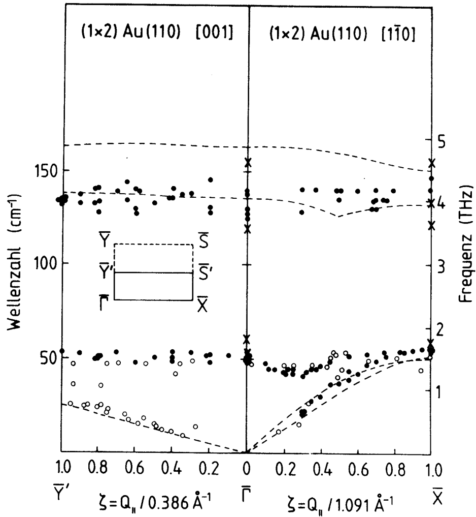
Abb. 8.4: Phonondispersion der (1x2)-rekonstruierten Oberfläche entlang der \overline{\Gamma X} - und der \overline{\Gamma Y} -Richtungen. Die EELS-Ergebnisse (geschlossene Kreise) werden mit Experimenten der He-Streuung (offene Kreise). „ab-initio“-Rechnungen (Kreuze bei \overline{\Gamma} und \overline{X} ) sowie mit „glue“-Modell Rechnungen (gestrichelte Linien) verglichen.
