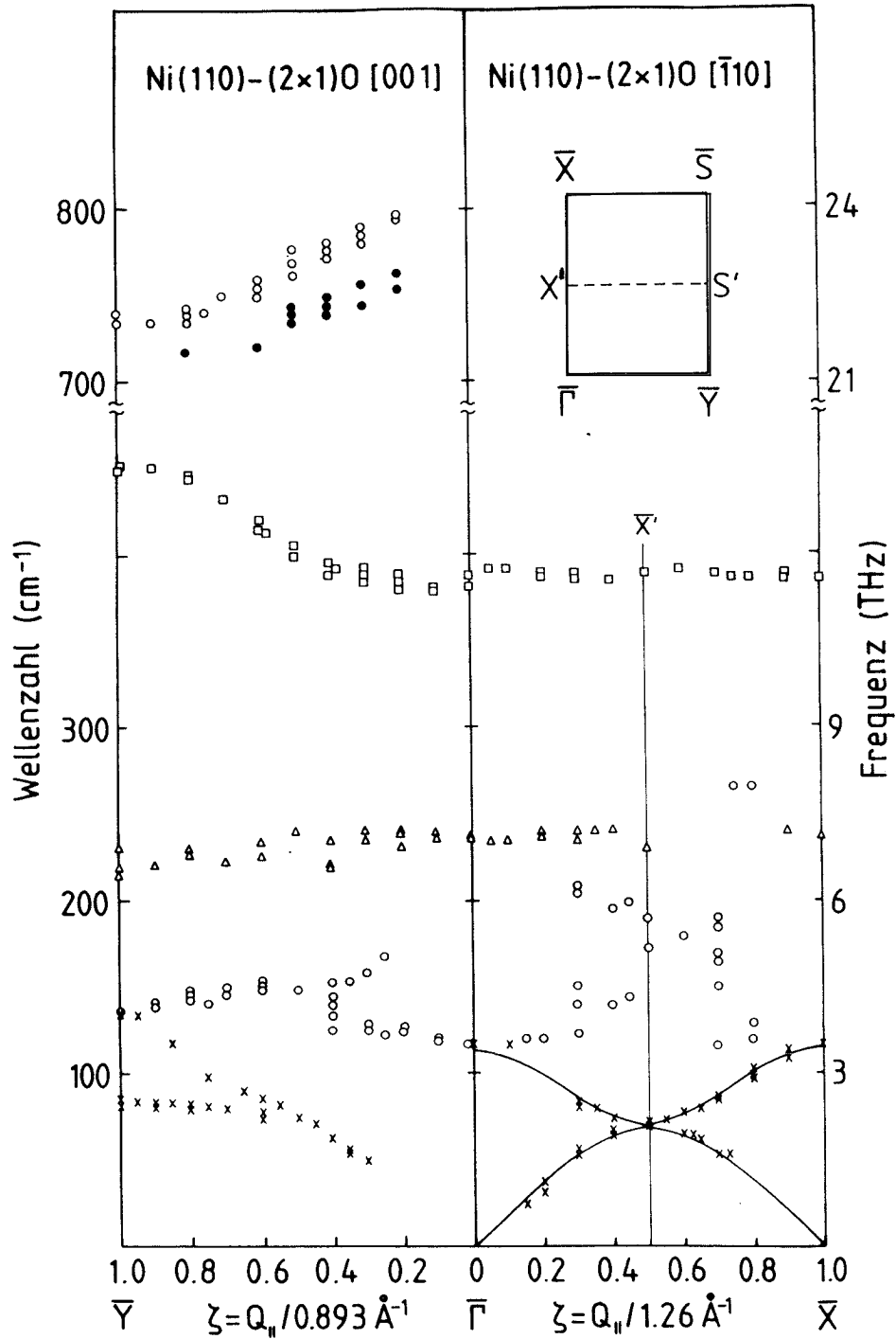
Abb. 7.7: Dispersionskurve der Phononen, die auf der Ni(110)-(2x1)O-Oberfläche entlang [001]- und [\bar{1}10] -Richtung gemessen wurden. Die dargestellte Brillouin-Zone ist die der reinen Fläche. Für die hochfrequente Sauerstoffmode oberhalb von 700\text{ cm}^{-1} ist die Dispersion für T = 100\text{ K} und T = 300\text{ K} (ausgefüllte Kreise) dargestellt. Bei allen anderen Verlusten war die Temperaturabhängigkeit unterhalb des experimentellen Fehlers von \sim 5\text{ cm}^{-1} .
