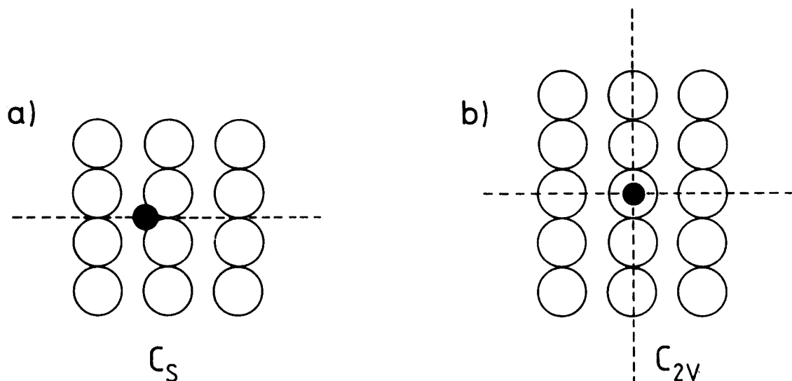
Abb. 2.1: Die Symmetrieeigenschaften der in (a) dargestellten Oberfläche können durch eine Spiegelung an der Horizontalen ( \sigma_x ) und die Drehung um 0^\circ ( E ) beschrieben werden ( C_S -Punktgruppe). Die Oberfläche in (b) wird durch folgende Symmetrieeoperationen beschrieben: Drehung um 180^\circ ( C_2 ), Spiegelung an der Horizontalen ( \sigma_x ), Spiegelung an der Vertikalen ( \sigma_y ) und die Drehung um 0^\circ ( E ) ( C_{2V} -Punktgruppe).
