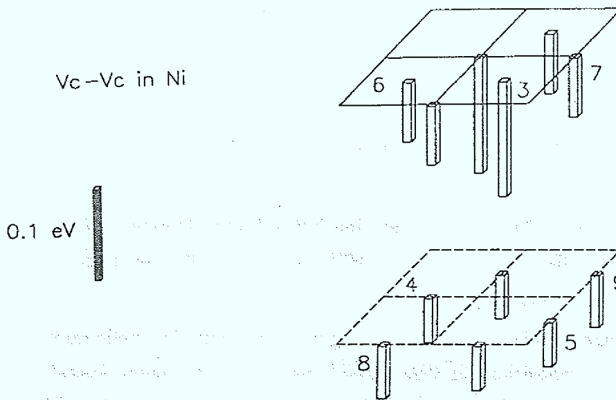
Abb. 4.16: In Ni von einer Doppelleerstelle (auf den Plätzen 1 und 2) hervorgerufene Änderungen des Madelungpotentials \Delta V_M^K an allen Plätzen des Clusters.
