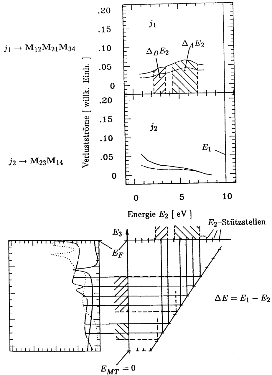
Bild 29 : Zur Erläuterung des Einflusses der k_{3//} -aufgelösten Oberflächenzustandsdichte (siehe Inset Bild 22–24) auf die Verluststromspektren. Links die Oberflächenzustandsdichte aus Bild 22–24 für k_{3//}^{sp=1} : (—), k_{3//}^{sp=2} : (---), k_{3//}^{sp=3} : ( \cdot \cdot \cdot ).
