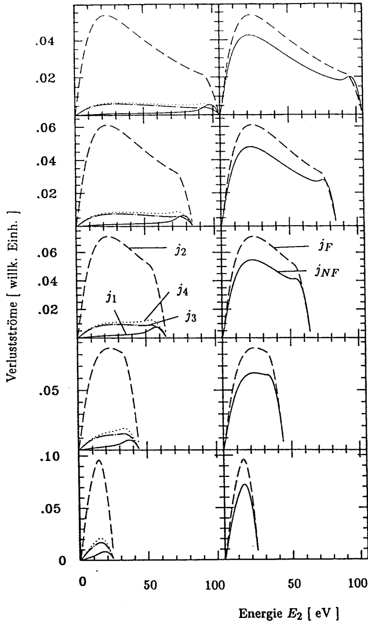
Bild 11 : Verlustströme für das homogene Elektronengas mit Oberflächenbarriere von Aluminium für die Primärenergien E_1 = 25, 45, 65, 85, 105 \text{ eV} mit \vartheta_1 = -45^\circ Einfalls- und \vartheta_2 = 45^\circ Austrittswinkel aus der "Kristalloberfläche". j_1 (—), j_2 (---), j_3 (-·-·-), j_4 (···) sind im linken Bildteil dargestellt, rechts die nach (3.35, 3.36) berechneten Non-Flip (—) und Flip (---) Verlustströme.
