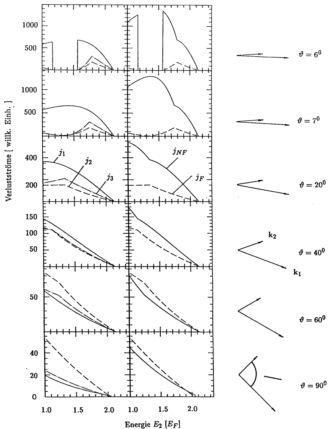
Bild 9: Non-Flip- und Flip-Verlustströme (3.35, 3.36) für Aluminium mit E_F = 11.7\text{eV} im Rahmen des Modells des homogenen Elektronengases mit konstanter Primärenergie E_1 = 2.14E_F \rightarrow 25\text{eV} , aber sich ändernden Einfallswinkel- und Ausfallswinkeln.
