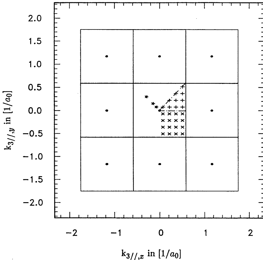
Bild 34: Drei erzeugende Punkte in der fcc(100) Oberflächenbrillouinzone sind mit ★ gekennzeichnet und in den ersten Quadranten geklappt zu denken. Die durch Symmetrietransformationen daraus erzeugten speziellen Punkte sind durch × dargestellt, sie sind ebenfalls in den ersten Quadranten transformiert vorzustellen. Die in den irreduziblen Teil der OBZ transformierten speziellen Punkte sind mit + symbolisiert.
