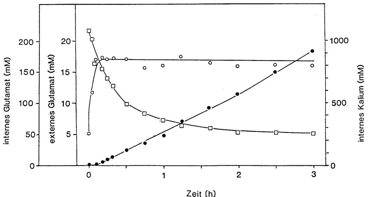
Abb. 6: Kurzzeitfermentation mit biotinlimitierten Produzenten-zellen. Die Verläufe der internen (offene Kreise) und der externen (geschlossene Kreise) Glutamatkonzentration, sowie der Verlauf der internen Kaliumkonzentration (offene Quadrate) sind angegeben.
