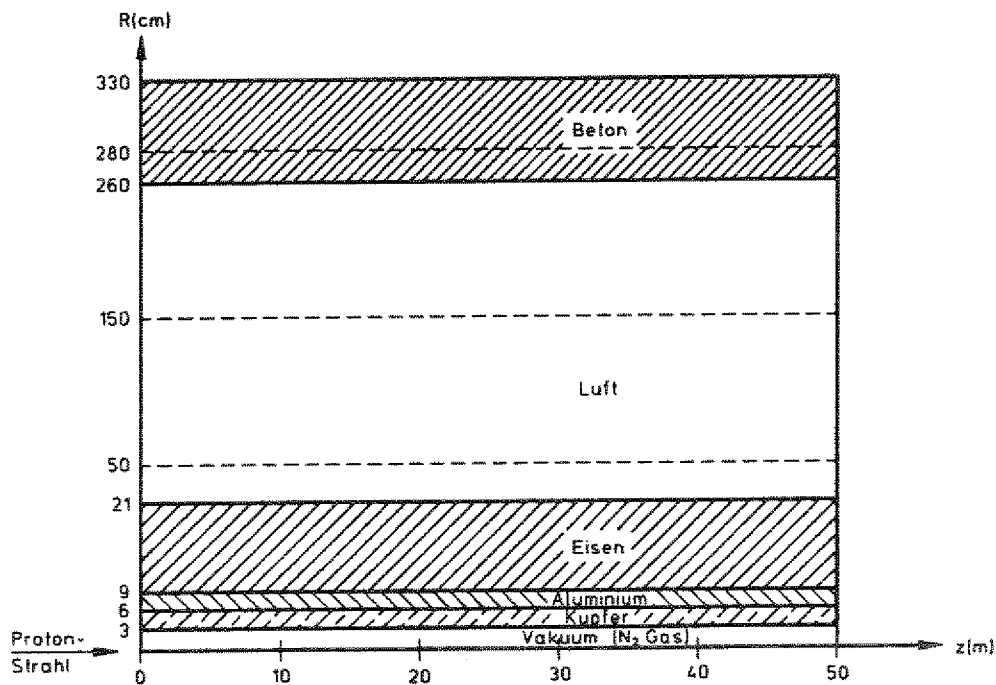
Abb. 5.49: Geometriemodell für die Simulation Magnet/Tunnel für den HERA-Beschleuniger
