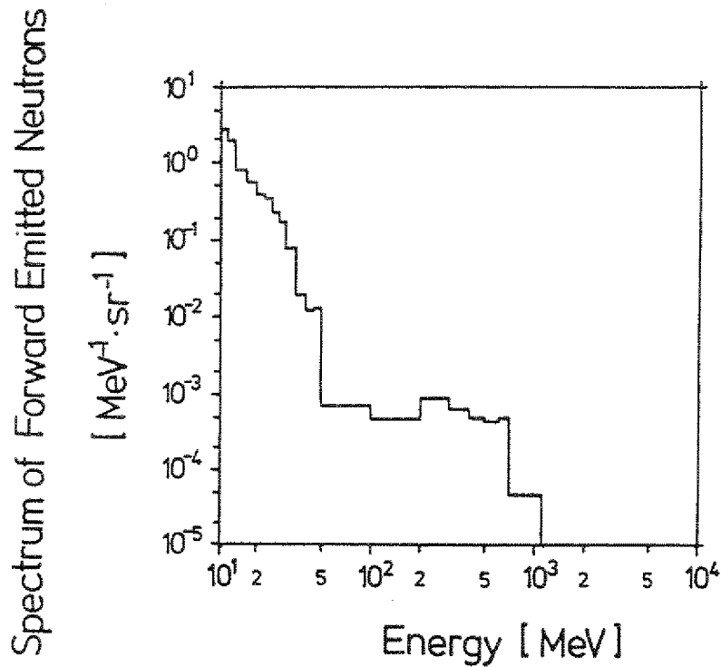
Abb. 5.29: Energiespektrum der im Target erzeugten Sekundärneutronen in Vorwärtsrichtung (0°) zum einfallenden Protonenstrahl von 1,1 GeV Energie
