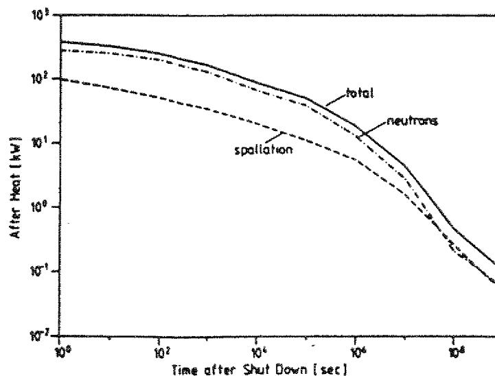
Abb. 6.8: Zeitlicher Verlauf der Nachwärmeabnahme in Uran nach 12000 Stunden Betrieb bei einer Protoneneinschussenergie von 1100 MeV und einem Strom von 5 mA nach Abschalten
