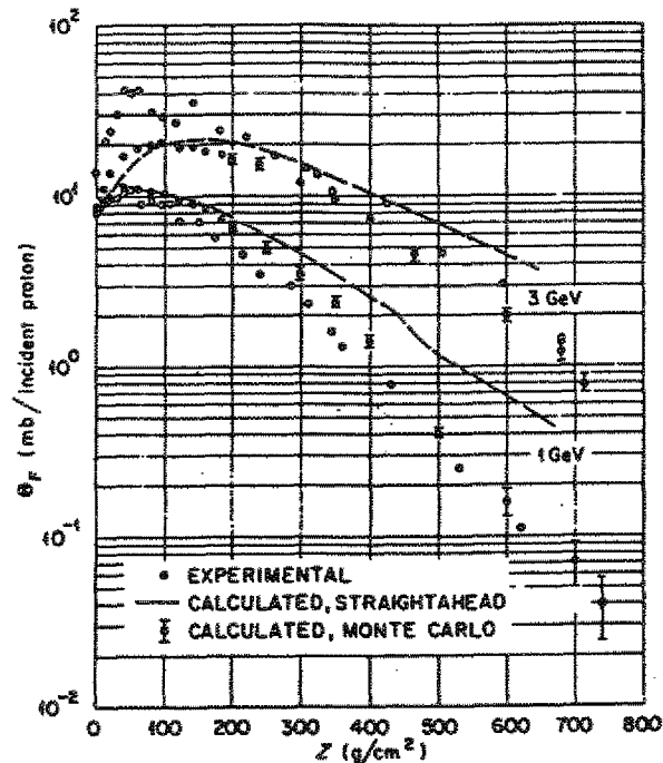
Abb. 5.3: Tiefenabhängigkeit (longitudinal) der Hochenergeteilchenkaskade in einer Eisenabschirmung für Protonenstrahlen von 1 GeV und 3 GeV. Die Ordinate ist proportional der ^{18}\text{F} -Produktion aus ^{27}\text{Al} -Folien mit einer Schwelle bei \approx 50 MeV. Der Beginn des Gleichgewichtsspektrums, d.h. exponentielle Abschwächung - liegt ca. bei 200\text{-}300\text{ g/cm}^2 (experimentelle Daten von S.P. Shen, Report BNL-8721, (1964))
