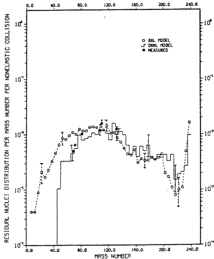
Abb. 4.13: Vergleich berechneter Restkernverteilungen HERMES-RAL Modell und ORNL Modell /4.43/ mit Messungen aus /4.44/ für 2,9 GeV Protonen auf Einschuß-Urantargets
