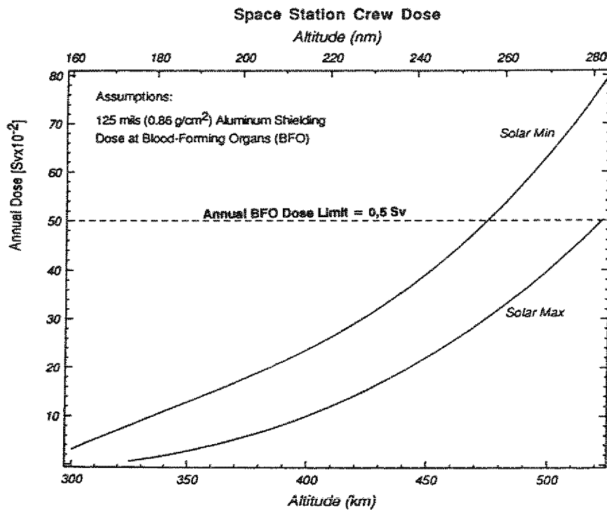
Abb. 7.15: Höhenabhängigkeit der Äquivalenzdosisrate im sog. LEO-Orbit (Low Earth Orbit)
