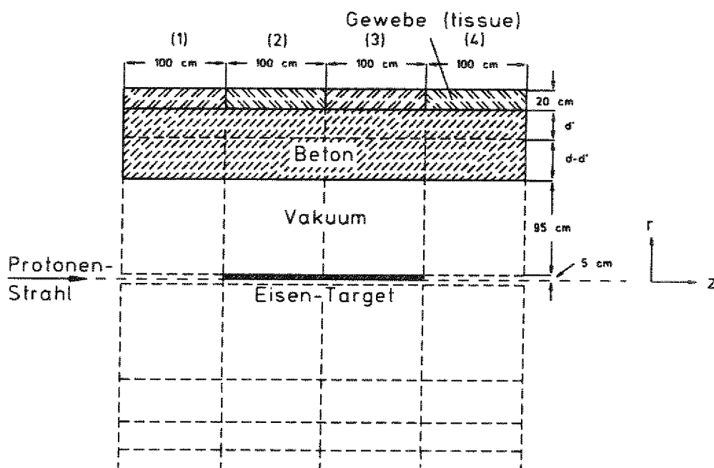
Abb. 5.45: Zylindrisches Geometriemodell für die Abschirmstudie (durchgezogene Linien sind Materialgrenzen; gestrichelte Linien stellen Zonengrenzen in der Geometrie dar)
