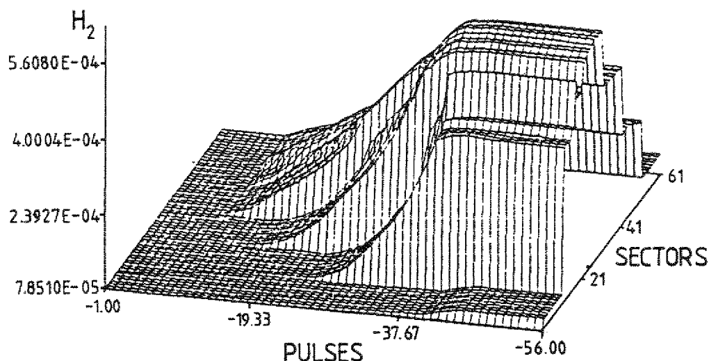
Abb. 6.11: H_2 -Konzentration in Mol pro Liter/Sektor und Zeitintervall
