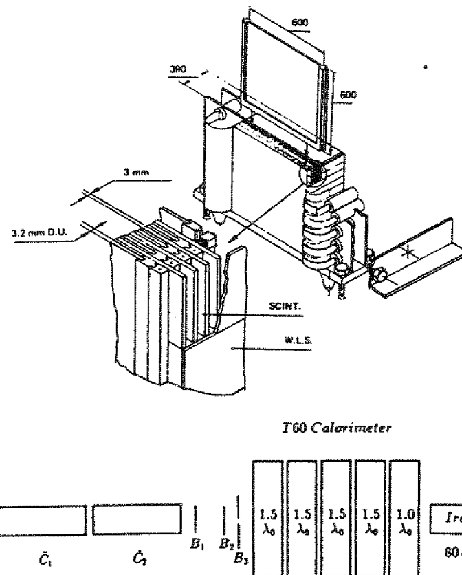
Abb. 5.9: Schematische Anordnung der Uran/Szintillator-Module des Test60B3 Experiments
