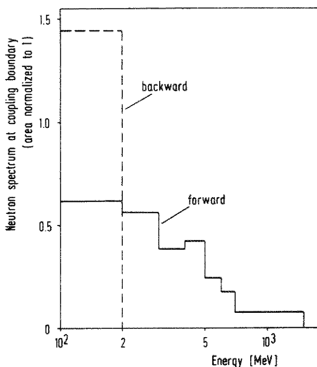
Abb. 5.26: Neutronenspektrum an der Kopplungsfläche von 1,1 GeV Protonen für das Targetsystem in Abb. 5.24 in Vorwärts- bzw. Rückwärtsrichtung ( 0^\circ/180^\circ ) (Kopplungsfläche bei R = 75 cm)
