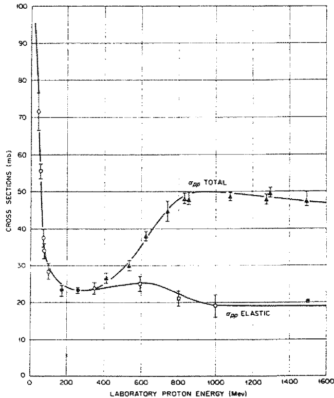
Abb. 4.1: Proton-Proton-Wechselwirkungsquerschnitt ( \sigma_{pp\text{-total}}/\sigma_{pp\text{-elastisch}} )
