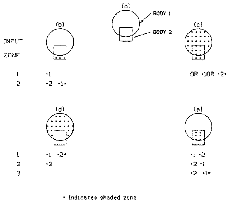
Abb. 2.17: Zonenbeschreibung für eine Kugel (SPH) und einen Zylinder (RCC) für eine Eingabe in CG (Schnittmenge)
