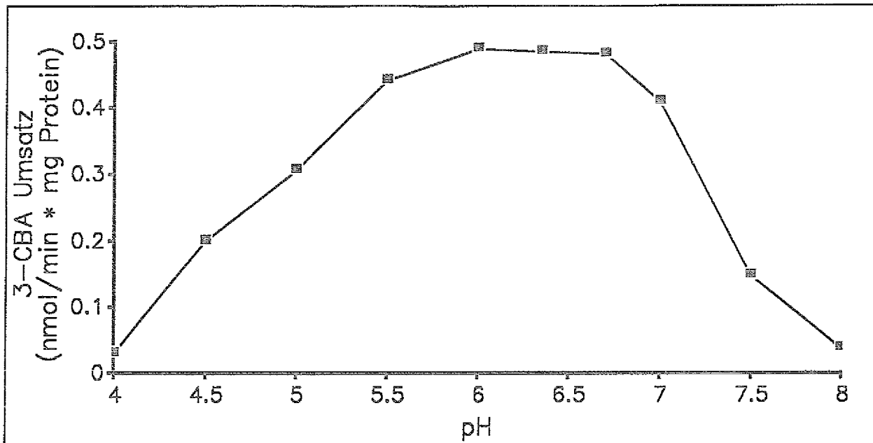
Abbildung 3.22: Einfluß des pH-Wertes auf die spezifische Aktivität in einem Rohextrakt aus D. vulgaris PY1 bei 37°C mit Wasserstoff als Elektronendonator und Methylviologen als Elektronenüberträger.
