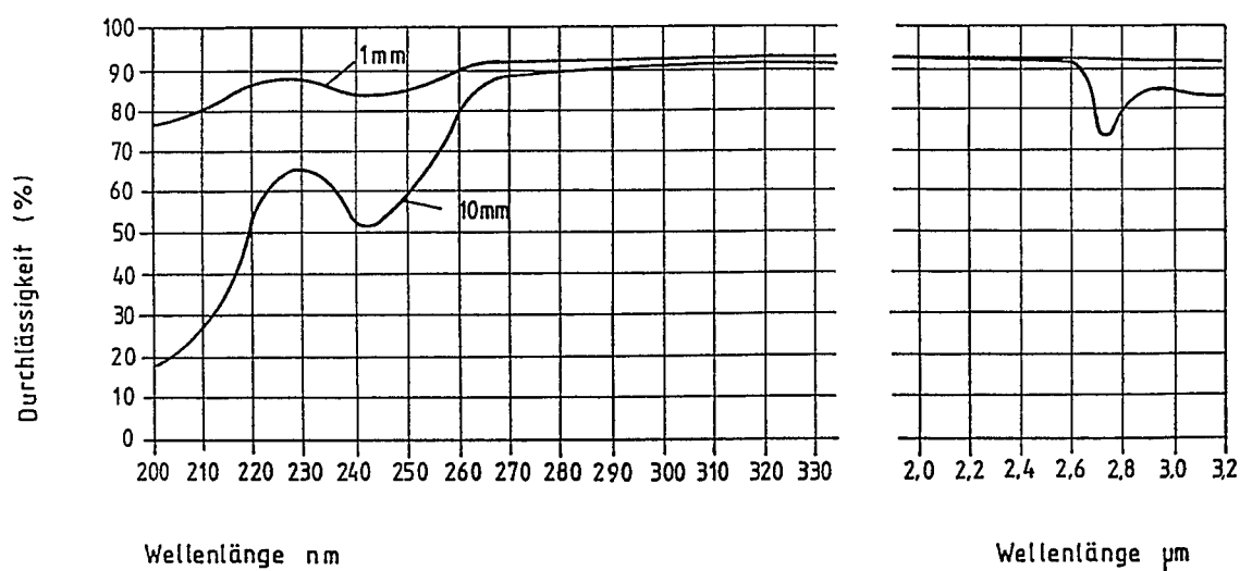
Abb. 3.9: Optische Durchlässigkeit von HSQ-Quarzglas (Heraeus Quarzschmelze 1988).
