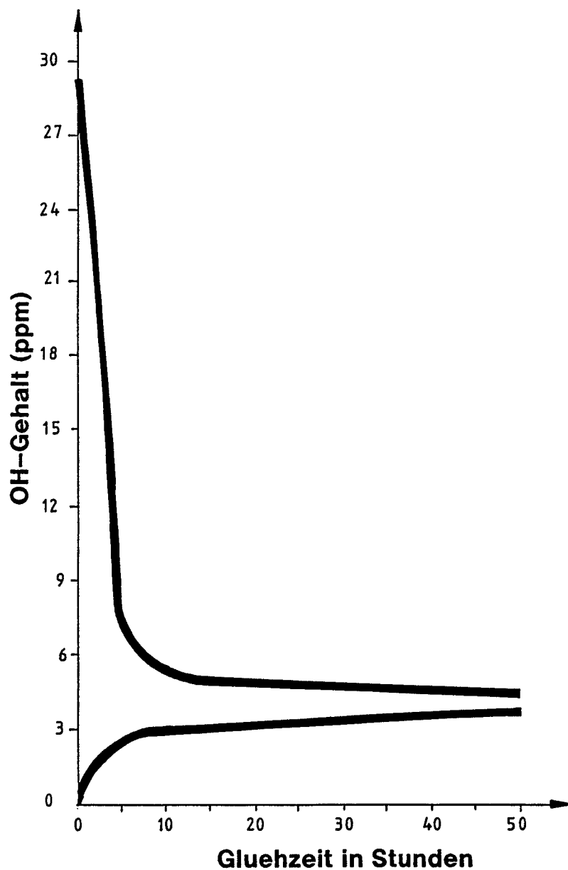
Abb. 3.10: OH-Gehalt in HSQ-Rohren an Luft (Heraeus Quarzschmelze 1988).
