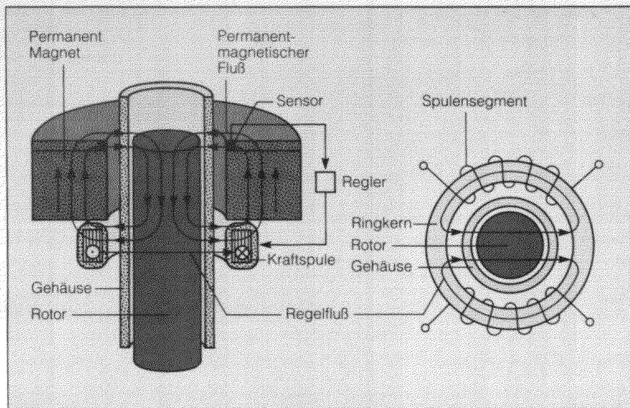
Abb. 3.3: Prinzip des berührungslosen Magnetlagers (K. Boden 1990).
