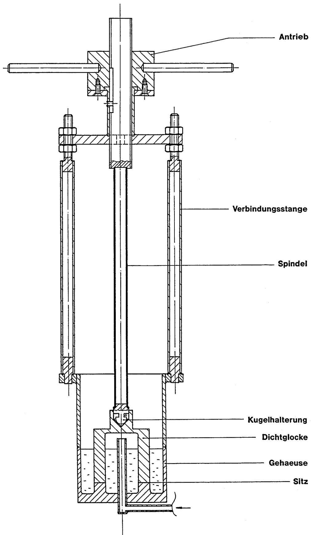
Abb. 6.16: Versuchsventil.
