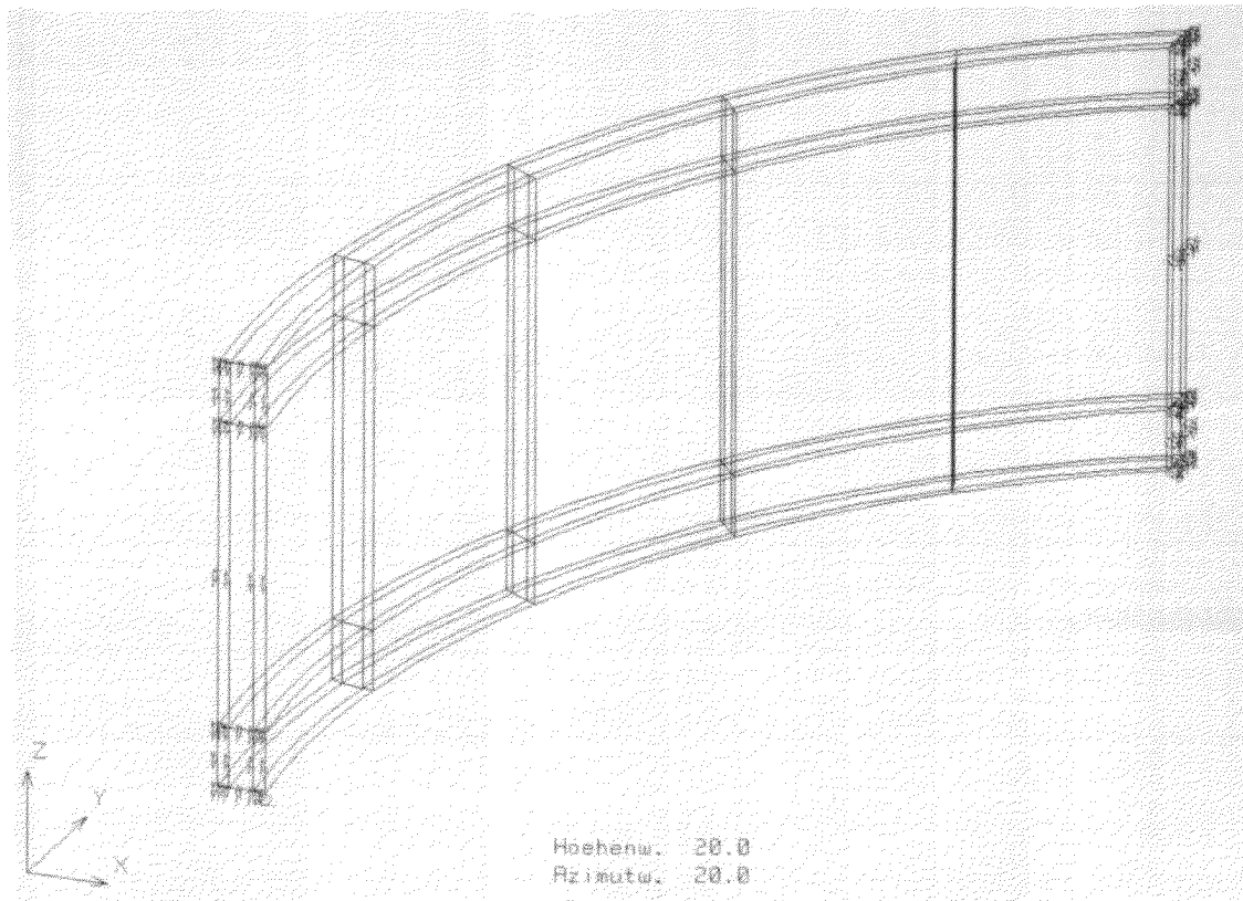
Abb. 4.13: Kühlkanal über den Winkelbereich von 90^\circ (H. Wyrwich 1989).
