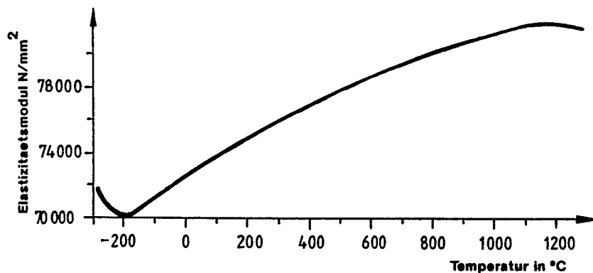
Abb. 3.8: Elastizitätsmodul von Quarzglas in Abhängigkeit von der Temperatur (Heraeus Quarzschmelze 1988).
