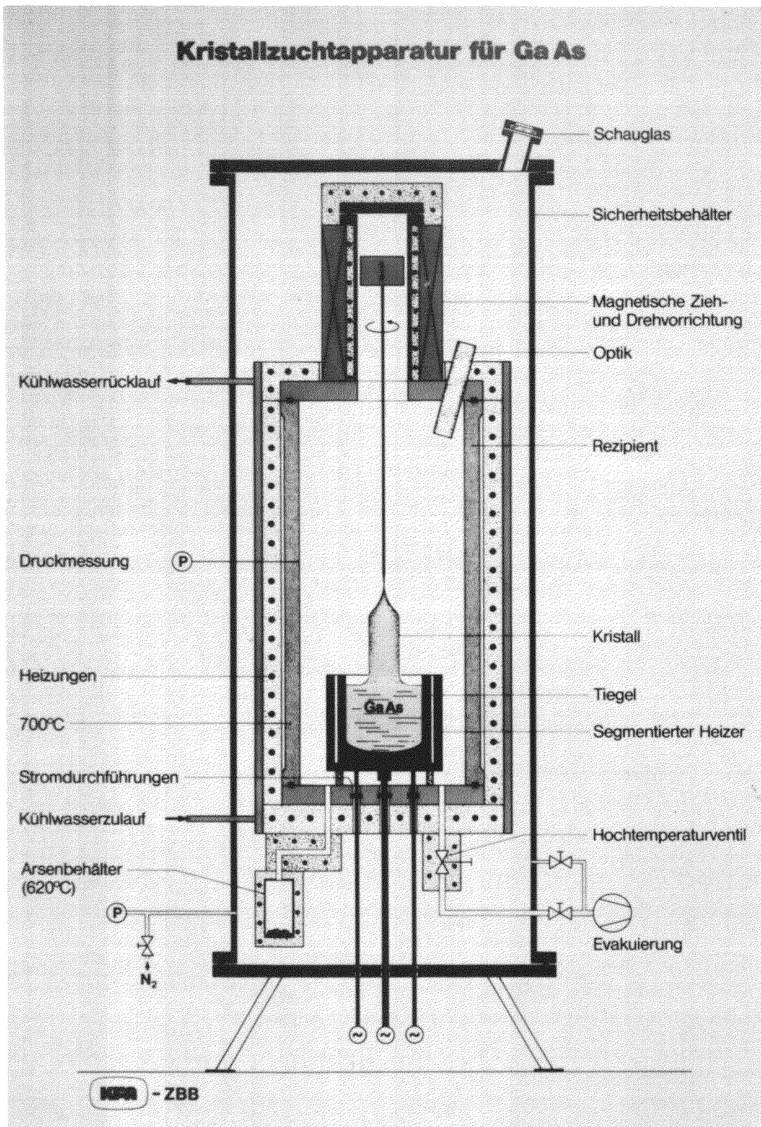
Abb. 6.1: Technisches Konzept einer metallischen GaAs-Kristallziehapparatur.
