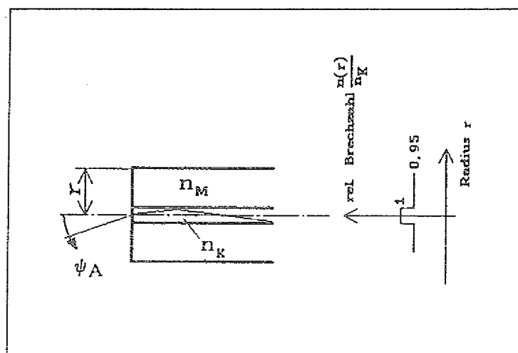
Abb. 5.1 Aufbau einer Monomodefaser und ideale Verteilung der Brechzahl über den Kernquerschnitt
