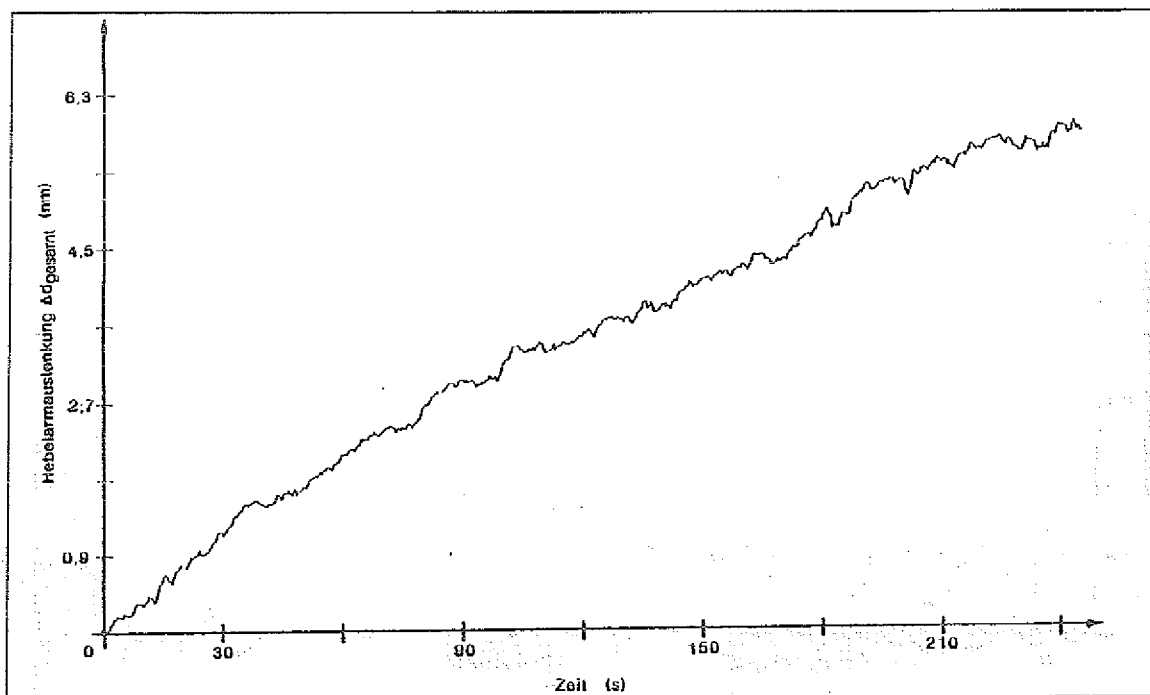
Abb. 6.6: Messung 4, Stabilität von d_{real} , i_{el} und \lambda durch messen von U_{\Delta d} U_{\Delta d} = U_{sig} (s. Gl. 5.6), \frac{d_{gesamt}}{t} = 2 \text{ nm/min}
