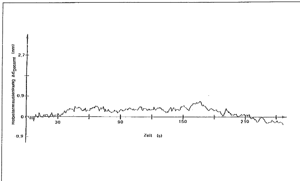
Abb. 6.5: Messung 3, Stabilität von d_{real} , i_{el} und \lambda durch messen von U_{\Delta d} U_{\Delta d} = U_{sig} (s. Gl. 5.6), \frac{d_{gesamt}}{t} = 0,2 \text{ nm/min}
