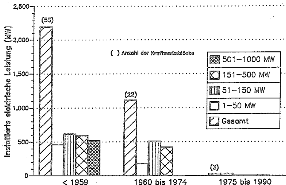
Bild 15a: Altersstruktur (Inbetriebnahmejahr) der industriellen Kraftwerke in den neuen Bundesländern, unterteilt nach Leistungsklassen
