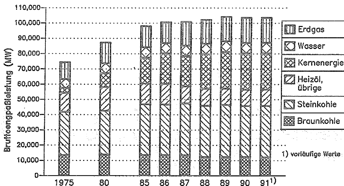
Bild 2: Installierte Bruttoengpaßleistung nach Energieträgern in den alten Bundesländern /BMWi 1990/, /VIK-Statistik 1991/, /SCHIFFER 1992/
