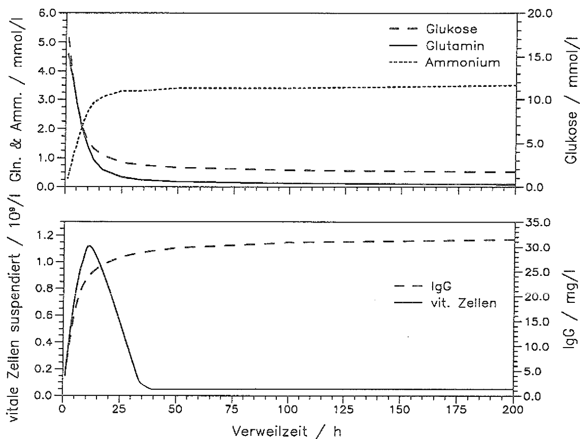
Abb. 5.5.7: Simulation eines X/D-Diagramms in einem Wirbelschichtreaktor; 200 ml Carrier, 1 l Gesamtvolumen, [Glk.]_{ein} 20 mM, [Gln.]_{ein} 5 mM
