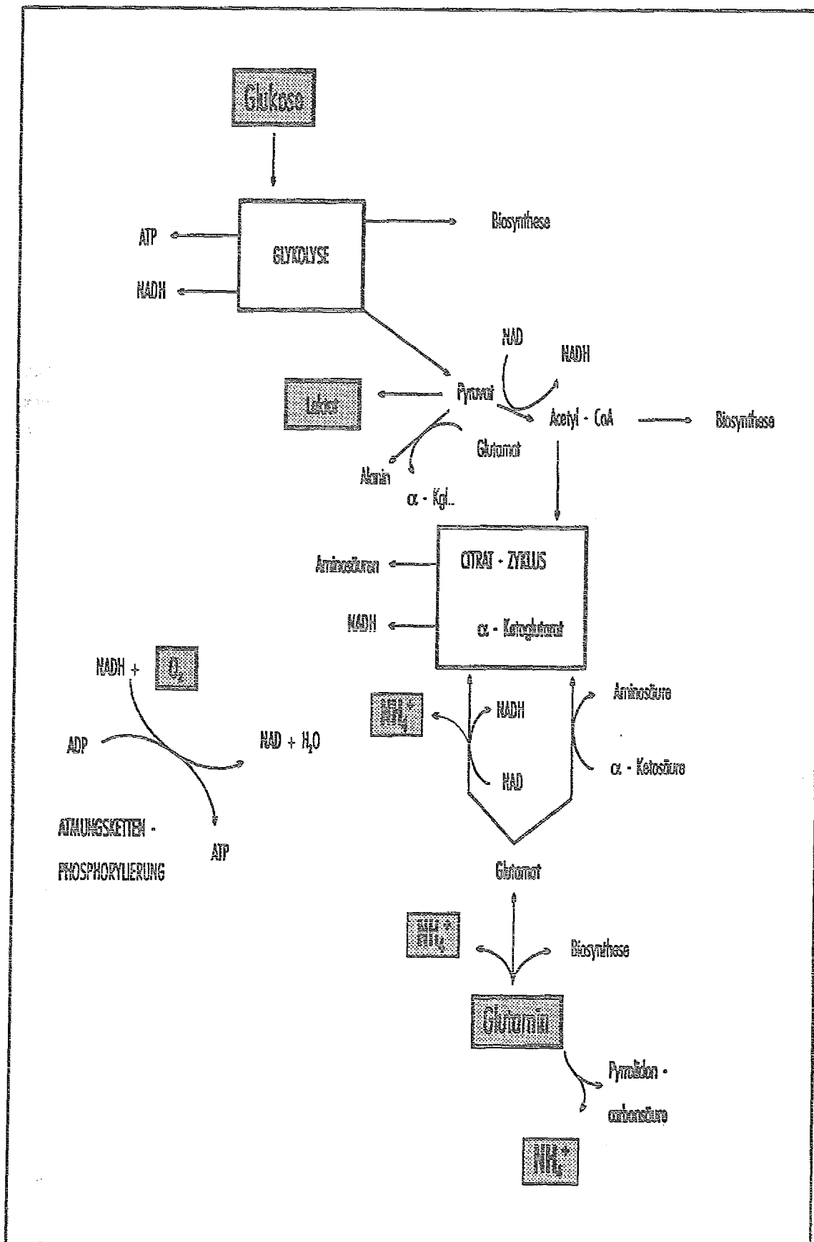
Abb. 3.1.1: Vereinfachte Darstellung der wichtigsten Wege des Hybridomastoffwechsels
