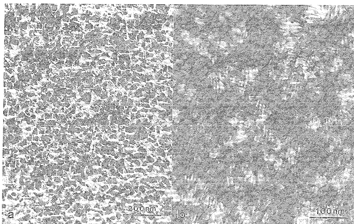
Abb. 6.5: (a) Fehlpassungsversetzungen an der Substrat-Puffer-Grenzfläche unter verschiedenen WBDF-Abbildungsbedingungen in der [001]-Projektion (Probe B2099, \vec{g} = (220) ). (b) Zweidimensionales Moiré-Kontrastmuster in einer [001]-Hellfeldabbildung (Probe B2099, \vec{g} = (220) ).
