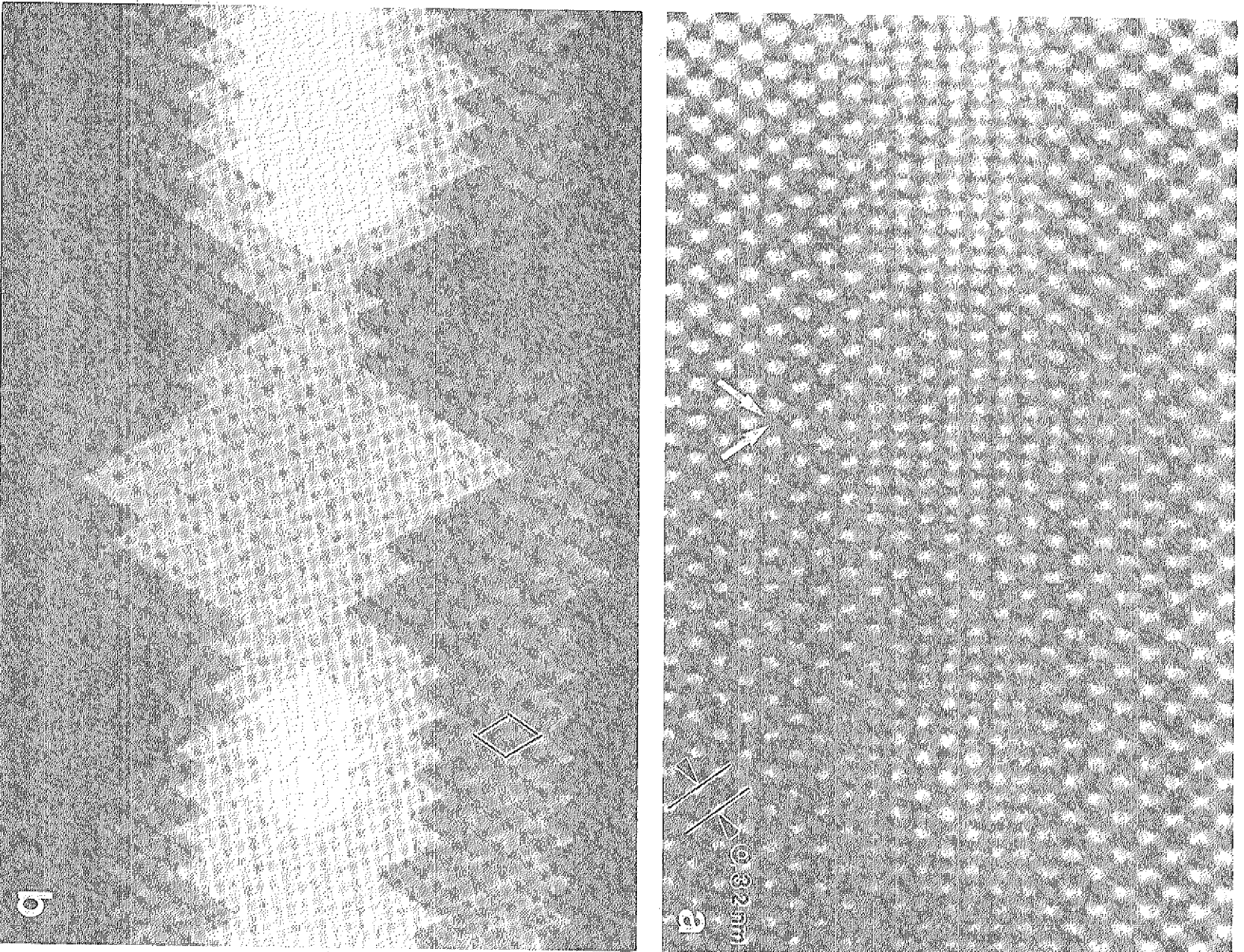
Abb. 6.13: (a) Experimentelle hochaufgelöste 7-Strahl-Gitterabbildung eines in Si eingebetteten \text{Si}_x\text{Ge}_{1-x} -Quantentopfes (nominal x = 0.3 ) in der [110]-Projektion. (b) Quantitative Graustufenrepräsentation der durch Anwendung der Methode bestimmten lokalen Komposition x_{\text{loc}} . Die unterschiedlichen Graustufen repräsentieren Kompositionen von x = 0.40 - 0.55 (hellgrau), von x = 0.55 - 0.70 (hell-/mittelgrau), von x = 0.70 - 0.85 (mittel-/dunkelgrau) sowie von x = 0.85 - 1.0 (dunkelgrau).
