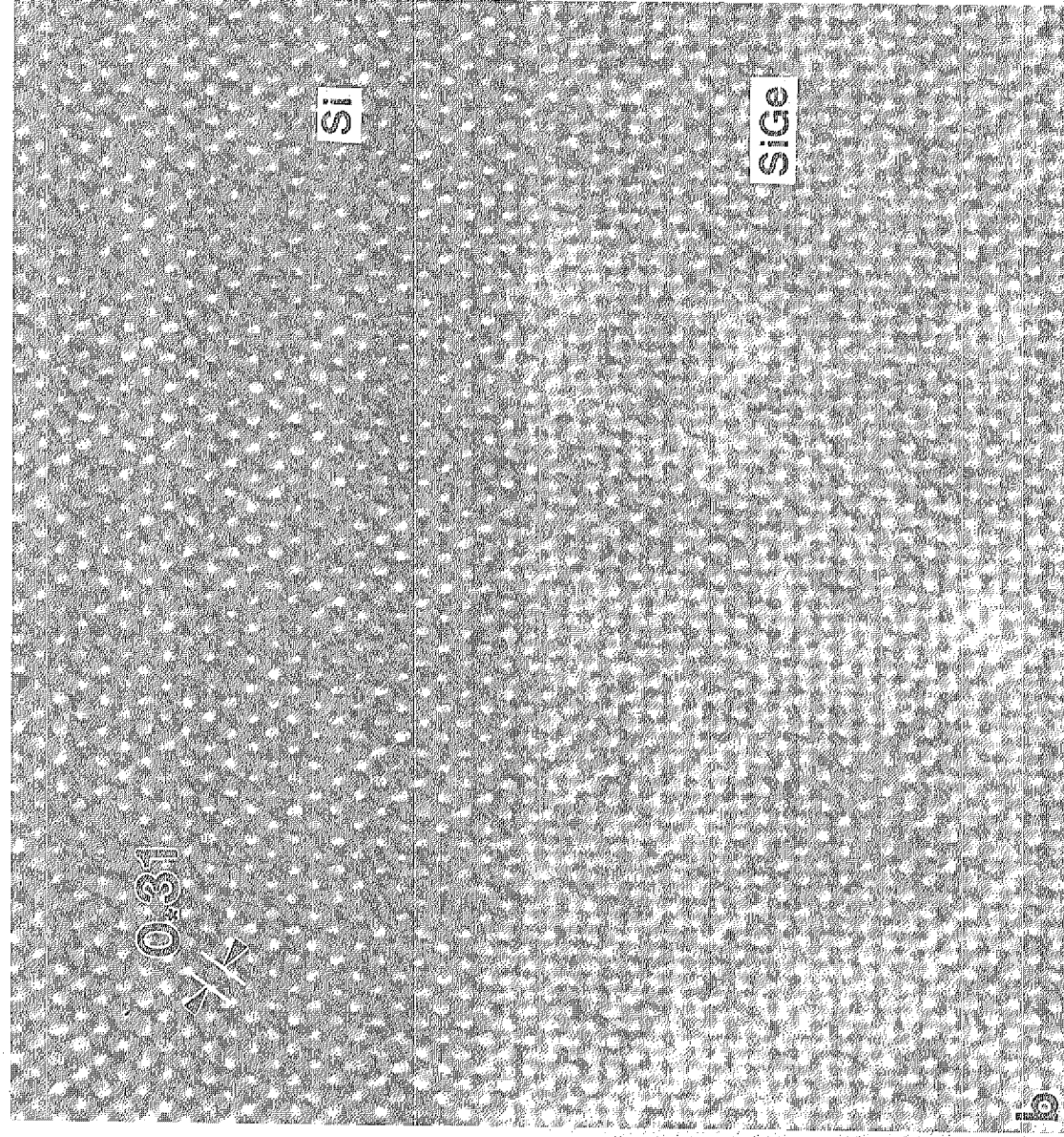
Abb. 6.15: (a) Übersichts-Hellfeldabbildung und (b) hochaufgelöste Gitterabbildung einer langperiodischen Si/Si 0,73 Ge 0,27 -Übergitterstruktur (Probe H1) vor der Temperbehandlung.
