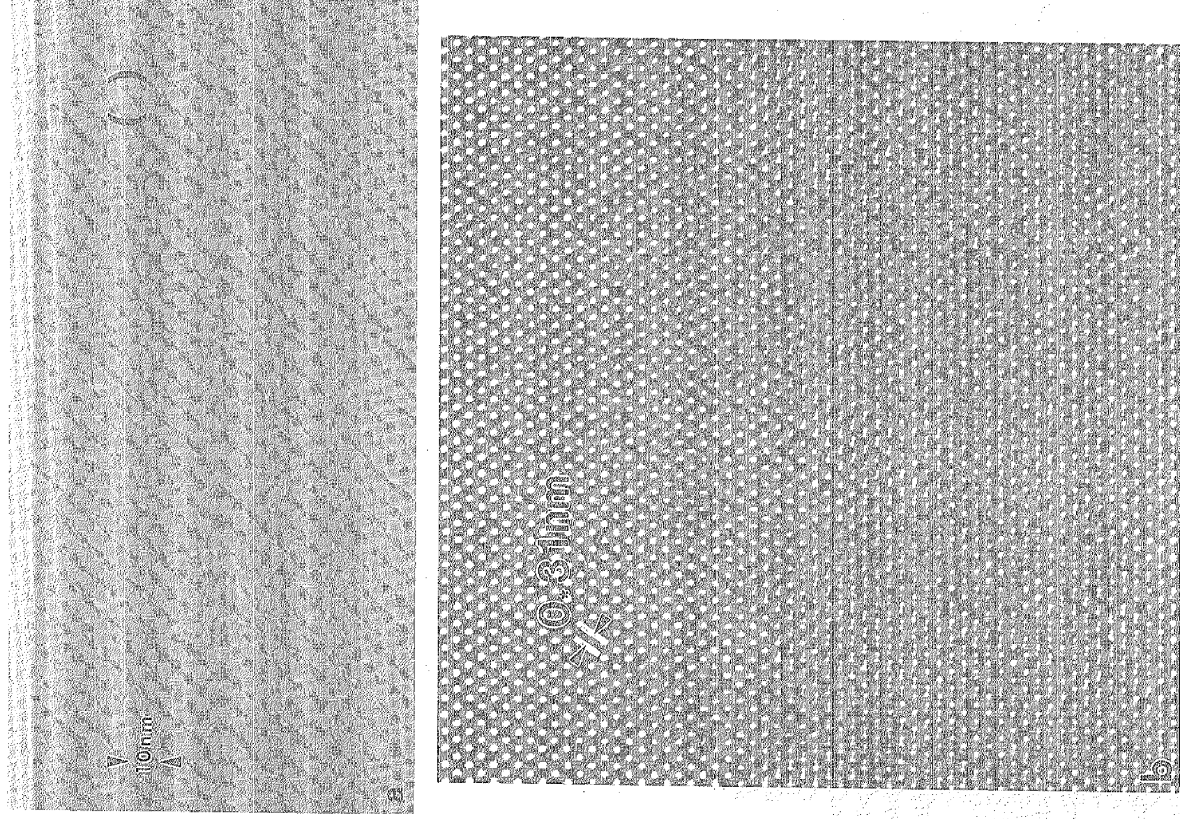
Abb. 6.16: (a) Übersichts-Hellfeldabbildung und (b) hochaufgelöste Gitterabbildung einer langperiodischen Si/Si 0.73 Ge 0.27 -Übergitterstruktur (Probe H1) nach der Temperbehandlung.
