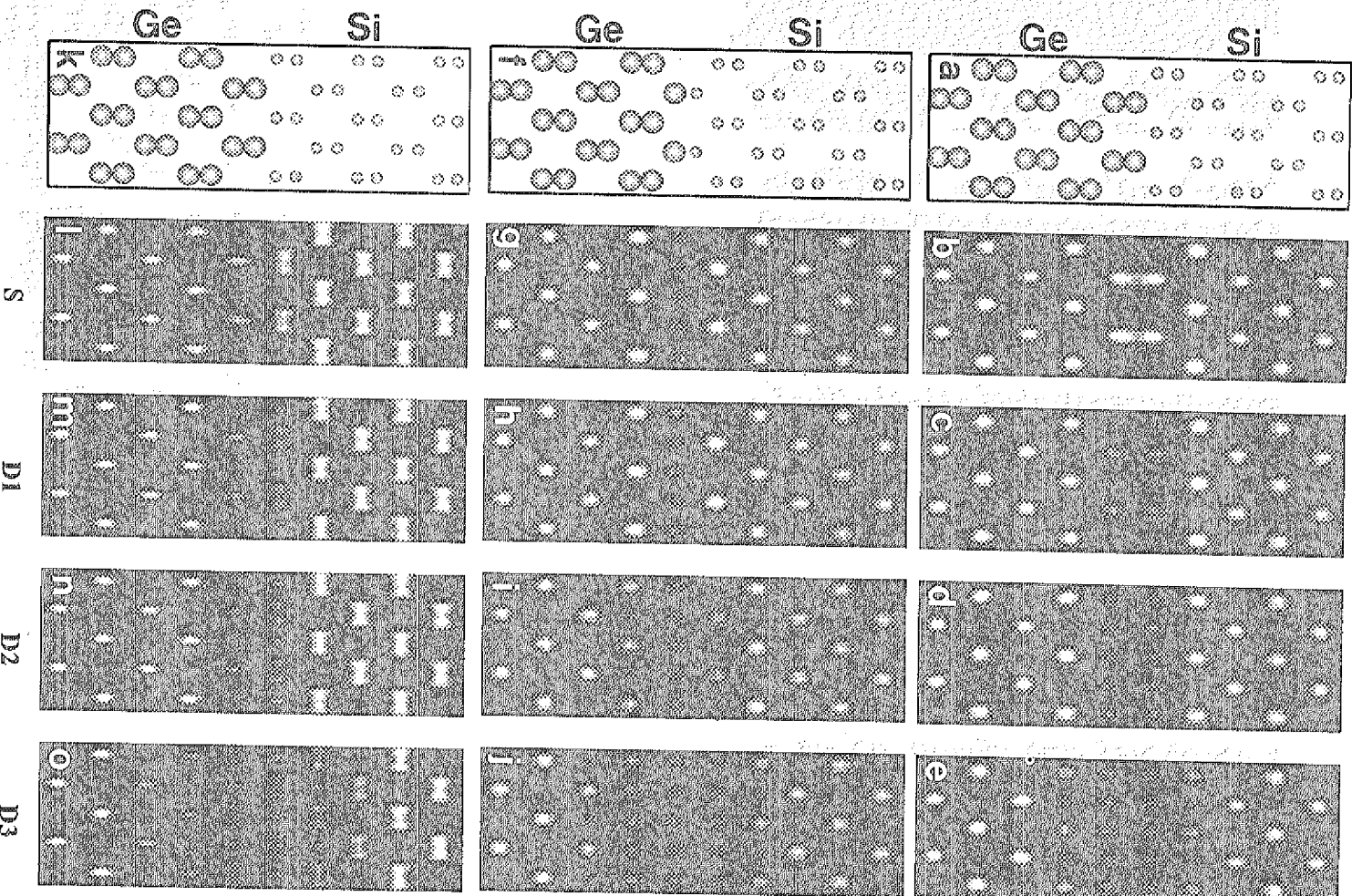
Abb. 4.1 : (b-e, g-j) Simulierte Gitterabbildungen unterschiedlicher Si/Si 2 Ge 1-x -Grenzflächentypen in der [110]-Projektion. (a, f, k) Projizierte atomare Grenzflächenstruktur für abrupte Grenzflächen vom Typ (S-a), (S-b) und (S-a). (b, g) 5-Strahl-Gitterabbildungen abrupter Grenzflächen vom Typ (S-a) und (S-b). (l) 9-Strahl-Gitterabbildungen einer abrupten Grenzfläche vom Typ (S-a). (c-e, h-j) 5-Strahl-Gitterabbildungen diffuser Grenzflächen vom Typ (D1-a), (D2-a) und (D3-a) bzw. (D1-b), (D2-b) und (D3-b) mit jeweils unterschiedlich breiten Si-Ge-Durchmischungszone(n). (m-o) 9-Strahl-Gitterabbildungen diffuser Grenzflächen vom Typ (D1-a), (D2-a) und (D3-a).
