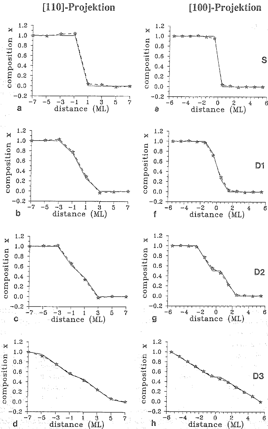
Abb. 5.4: Kompositionsprofile für abrupte (a,e) und diffuse (b-d, f-h) Si/Si x Ge 1-x -Grenzflächen in der [110]- und [100]-Projektion. Nominelle Komposition x_{\text{nom}} (—), ermittelte Komposition x_{\text{det}} (---).
