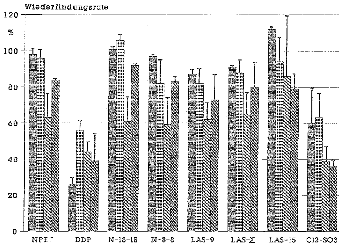
Abb. 3-8. Vergleich der Leistungsfähigkeit verschiedener Lösemittel und Verfahren bei der Extraktion feststoffgebundener Tenside. - Probe: Tensidgemisch nach Tab. 3-1 (S. 19), direkt auf die Filter dotiert. Wartezeit nach Dotierung: 1 h. Extraktionsmittel und Extraktionsverfahren: ■ Salzsäure/Methanol & Heißeextraktion; ▨ Salzsäure/Methanol & Kochen; ▤ Methanol & Heißeextraktion; ▦ Methanol & Kochen. Extraktionsdauer: 4 h. Mittelwert und Standardabweichung aus 2 Messungen bzw. 4 Messungen ( ▨ ). Experimentelle Details siehe Abschnitt 5.3.3.
