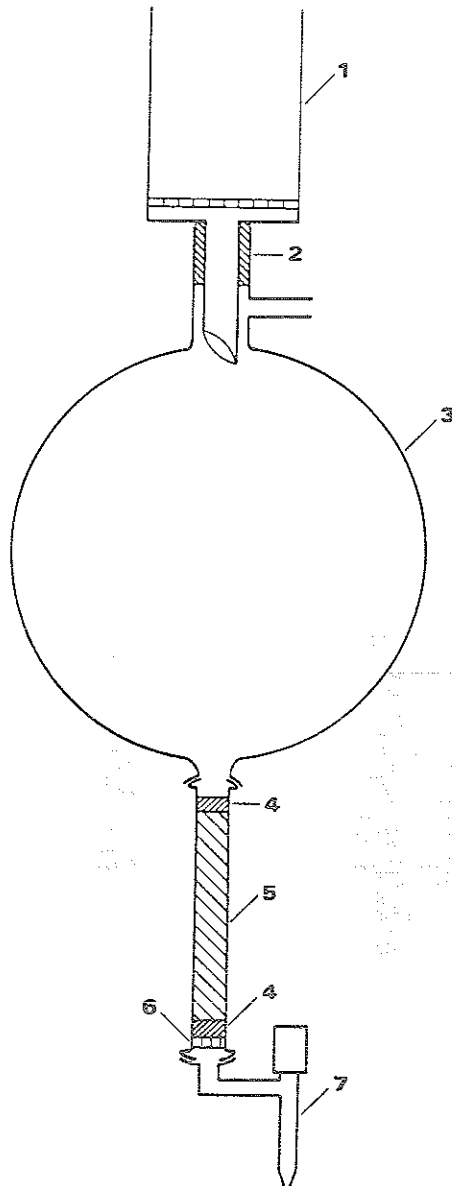
Abb. 3-2. Apparatur zur Filtration und Festphasenextraktion wäßriger Tensidlösungen. - 1 Filtrationsaufsatz; 2 Gummidichtung; 3 Kolbenaufsatz mit Vakuumstutzen; 4 Glaswatte/-wolle; 5 Adsorbersäule; 6 Glasfritte; 7 Bürettenhahn.
