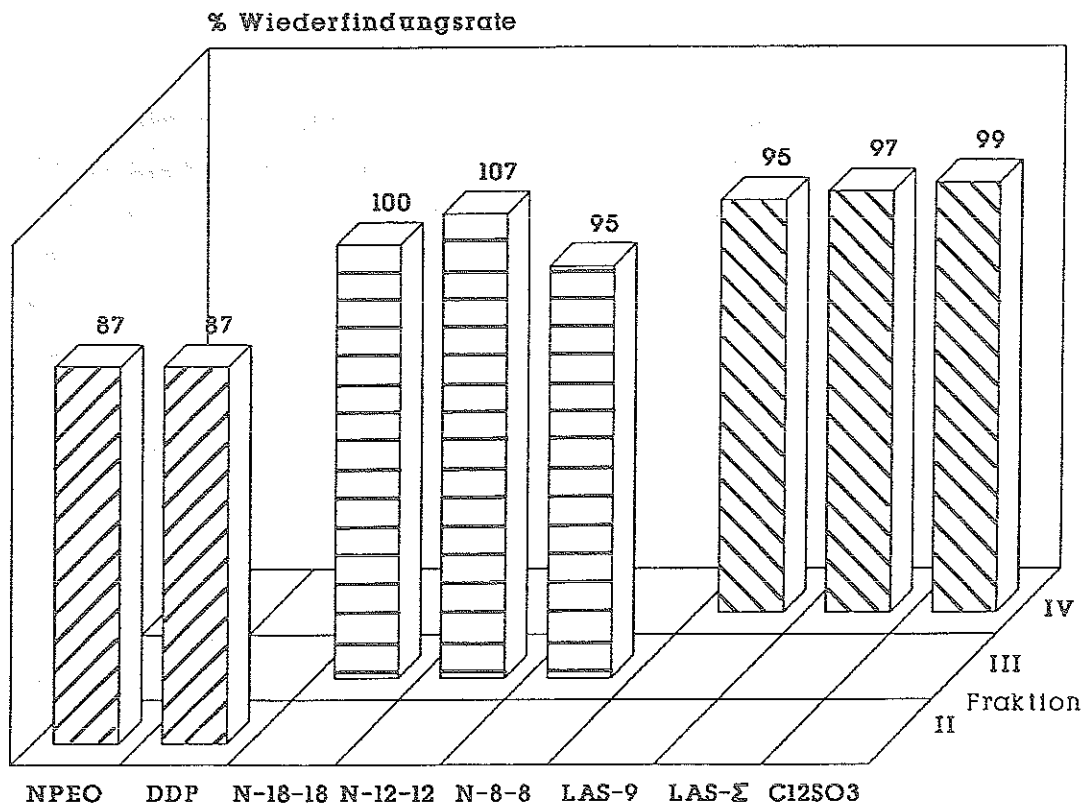
Abb. 3-12. Wiederfindung von Modellschubstanzen im Trennungsgang und Verteilung auf die einzelnen Fraktionen. - Erläuterungen siehe Tab. 3-7.
