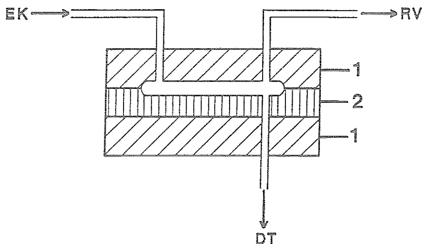
Abb. 3-15. Aufbau des Phasenseparators. - 1 Edelstahl; 2 PTFE; EK Extraktionskapillare; DT Fluoreszenzdetektor; RV Regulierventil.
