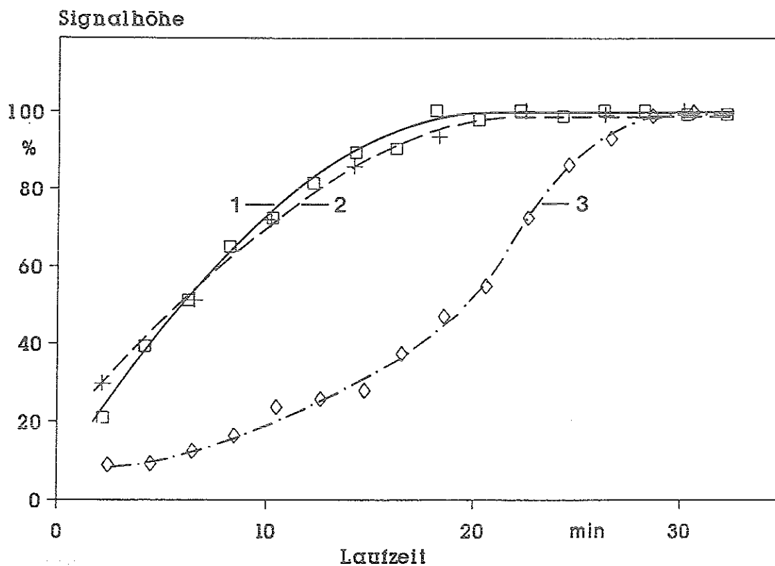
Abb. 3-19. Zeit- und Tensidmengenabhängigkeit des Detektorsignals bei verschiedenen Materialien der Mischkapillare.
