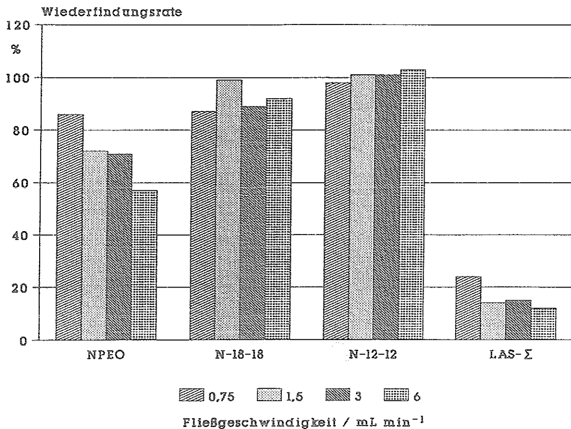
Abb. 3-3. Einfluß der Fließgeschwindigkeit der Probelösung auf die Wiederfindung von Tensiden. - Probe: Tensidgemisch nach Tab. 3-1 (S. 19), gelöst in 1000 mL destilliertem Wasser. Säule: 120 mm x 10 mm i.D. (innerer Durchmesser) XAD-2. Manuelle Mehrstufenelution. Einfachbestimmungen. Experimentelle Details siehe Abschnitt 5.3.2.
