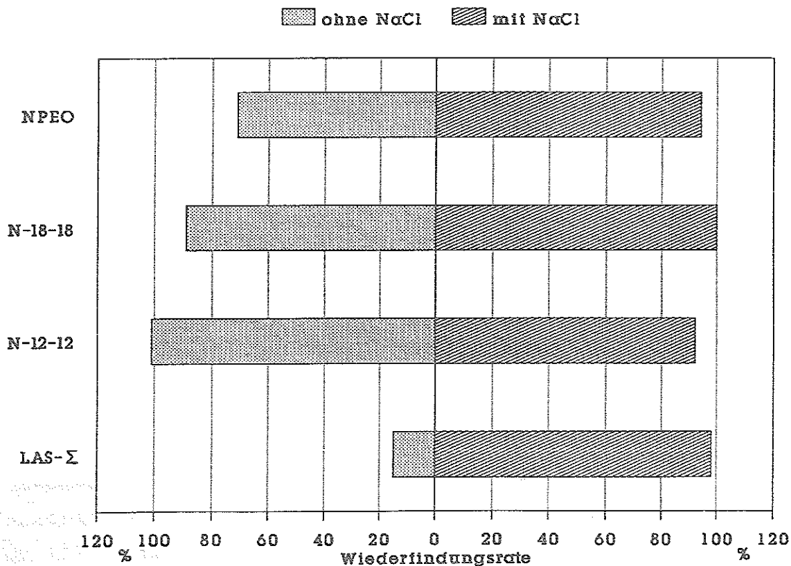
Abb. 3-4. Einfluß des Salzzusatzes zur Probelösung auf die Wiederfindung von Tensiden. - Probe: Tensidgemisch nach Tab. 3-1 (S. 19), gelöst in 1000 mL destilliertem Wasser bzw. Natriumchloridlösung ( 10 \text{ gL}^{-1} ). Säule: 120 mm x 10 mm i.D. XAD-2. Manuelle Mehrstufenelution. Einfachbestimmungen. Experimentelle Details siehe Abschnitt 5.3.2.
