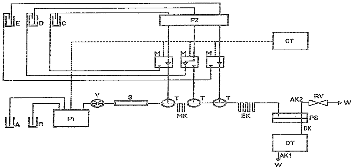
Abb. 3-22. Aufbau des Systems. - A Fließmittel A; AK1 Abfallkapillare; AK2 Abfallkapillare; B Fließmittel B; C Reagenzlösung; D Methanol; DK Detektorkapillare; DT Fluoreszenzdetektor; E Chloroform; EK Extraktionskapillare; M Magnetventil; MK Mischkapillare; P1 HPLC-Gradientenpumpe; P2 3-Kanal-Reagenzpumpe; PS Phasenseparator; RV Regulierventil; S HPLC-Trennsäule; T T-Verbindungs-Stück; V Injektionsventil; W Abfall.
