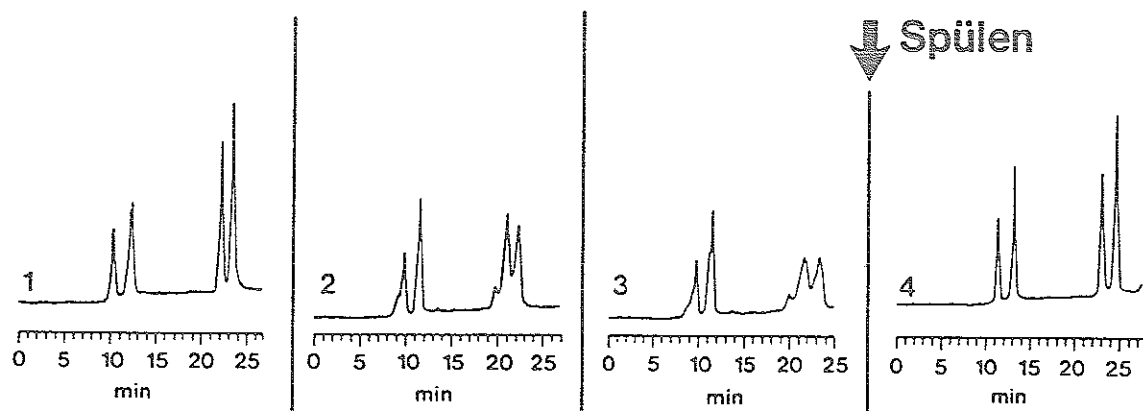
Abb. 3-17. Wirkung der integrierten Spülfunktion.
