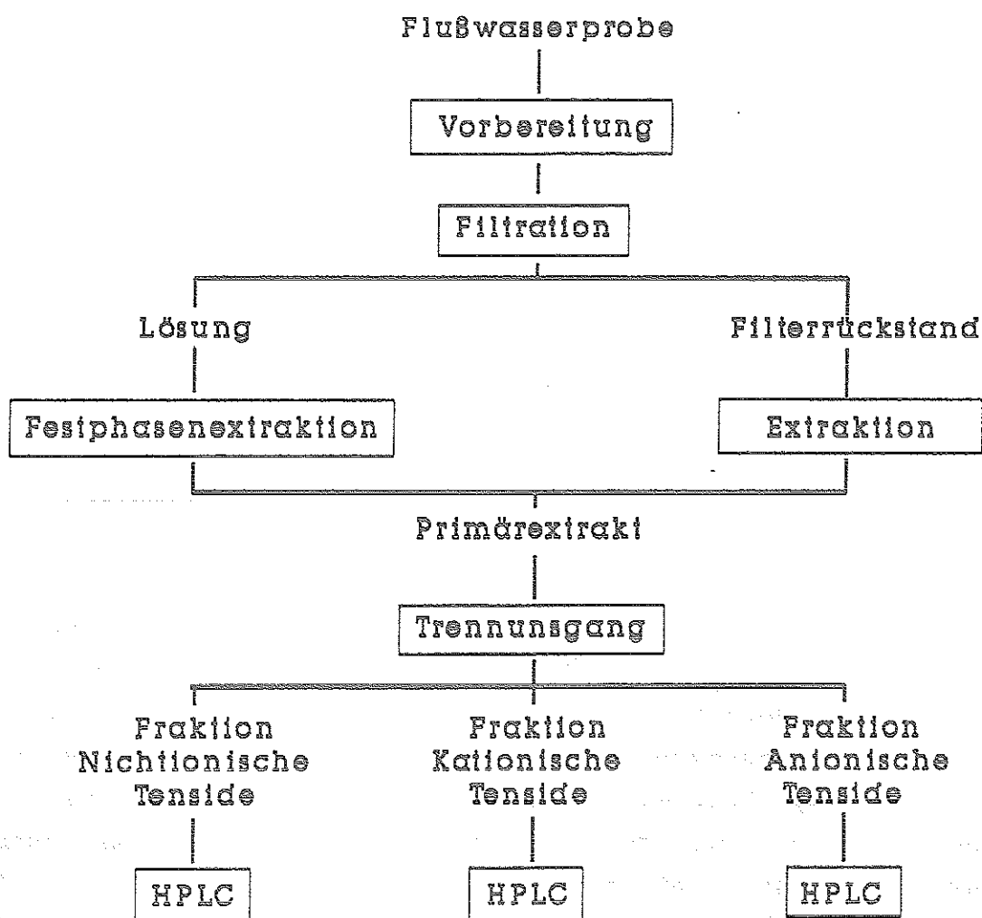
Abb. 3-1. Arbeitsablauf der Bestimmung von Tensiden in Flußwasser.
