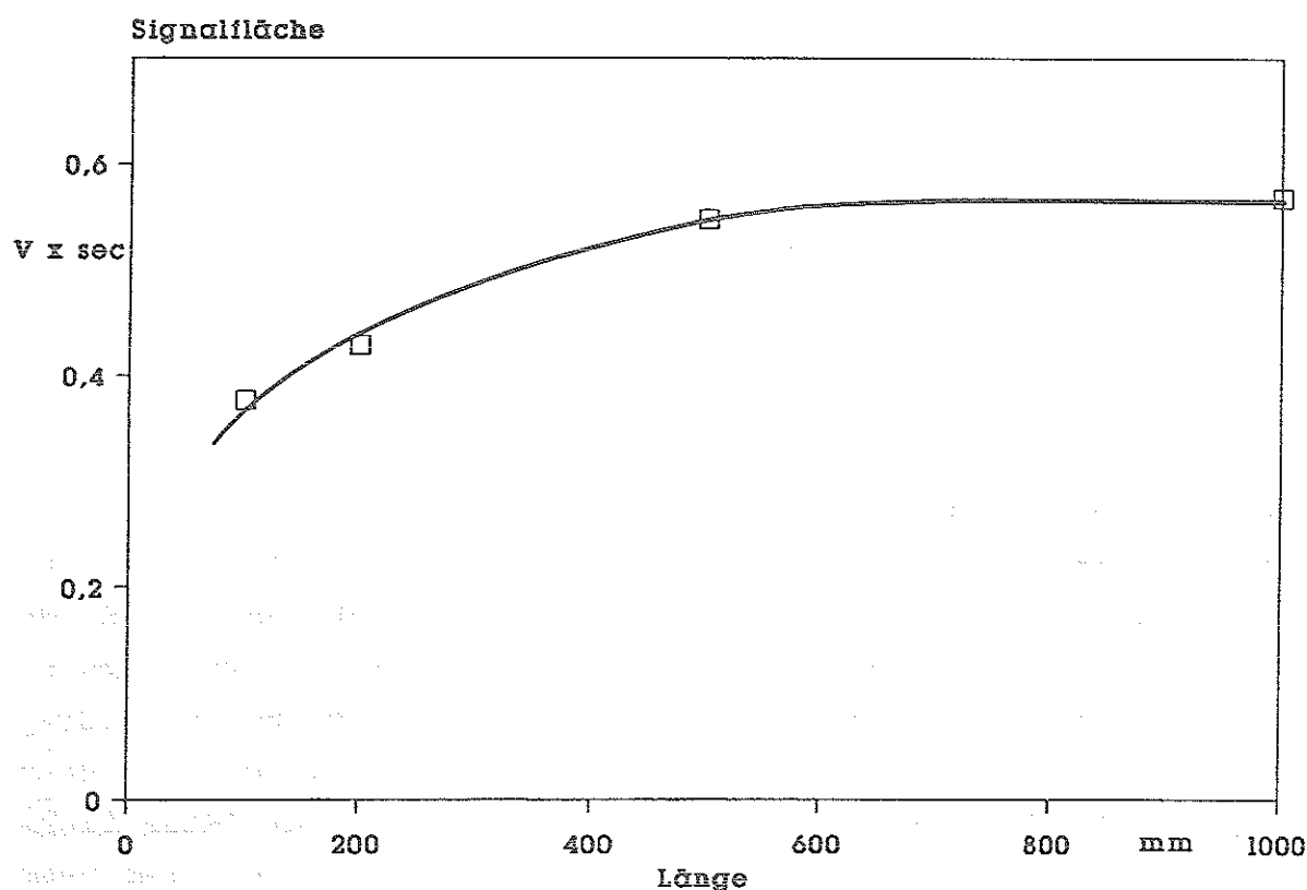
Abb. 3-26. Signalfläche als Funktion der Länge der Extraktionskapillare. - Injektionsmenge: 100 ng C10-SO3. Extraktionskapillare: Tefzel 0,5 mm i.D.. Einfachbestimmungen.
