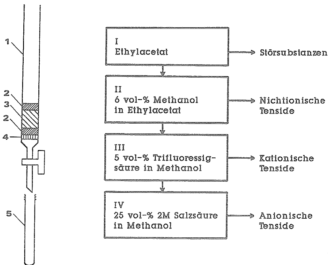
Abb. 3-11. Aufbau der Trennsäule und Arbeitsablauf des optimierten Trennungsganges. - 1 Chromatographiesäule; 2 Glasfaserwatte; 3 Aluminiumoxid; 4 Glasfritte; 5 Schraubgläschen. Elutionsmittelvolumina: je 6 mL. Experimentelle Details in Abschnitt 5.2.1.
