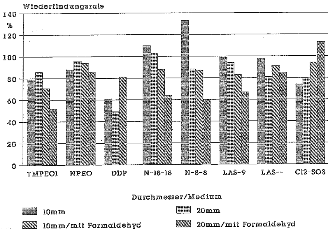
Abb. 3-5. Einfluß der Säulendimensionierung und des Formaldehydgehaltes der Probelösung auf die Wiederfindung von Modellsubstanzen. - Probe: Tensidgemisch nach Tab. 3-1 (S. 19), gelöst in 1000 mL Natriumchlorid/Citratpuffer mit bzw. ohne 0,36 vol-% Formaldehyd. Säule: 120 mm x 10 mm bzw. 20 mm i.D. XAD-2. Destillative Zweistufenelution. Einfachbestimmungen. Experimentelle Details siehe Abschnitt 5.3.2.
