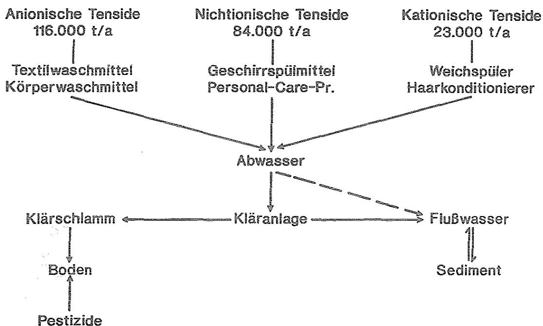
Abb. 2-2. Eintrag und Verteilung von Tensiden in der Umwelt.
