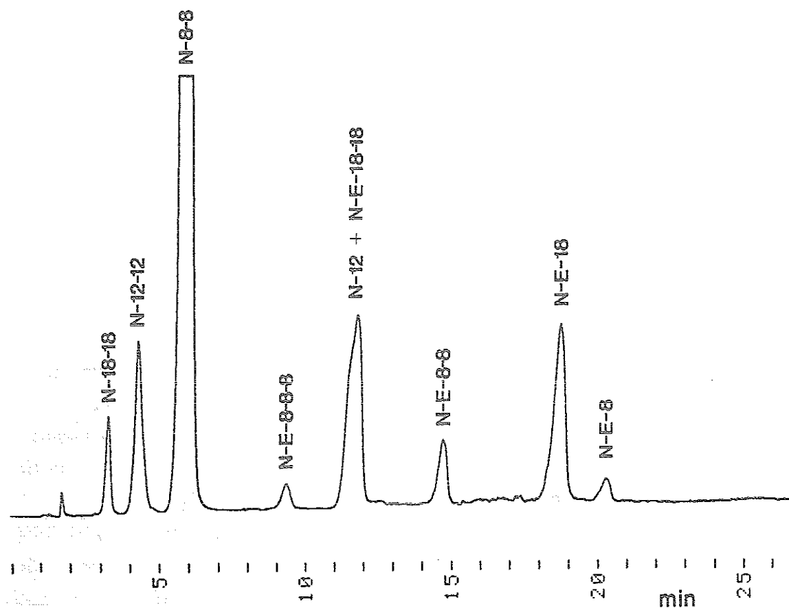
Abb. 3-16. Chromatogramm eines Standardgemisches von Alkylammoniumverbindungen und Esterquats. - Injektionsmengen: Alkylammoniumverbindungen jeweils 100 ng; N-E-8-E 200 ng; N-E-18-E 1000 ng. HPLC-Bedingungen: siehe Abschnitt 5.2.3.
