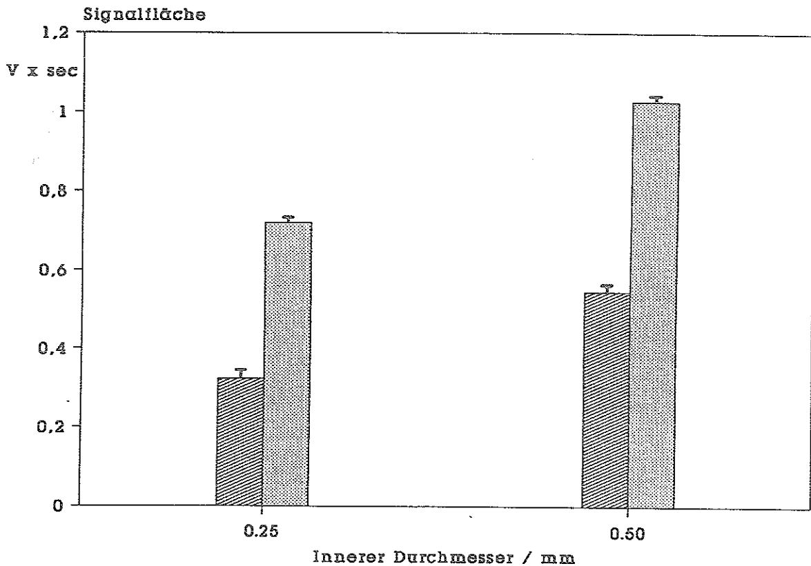
Abb. 3-27. Signalfläche bei unterschiedlichen inneren Durchmessern der Extraktionskapillare und verschiedenen Injektionsmengen. - Injektionsmenge C10-SO3: ▨ 100 ng; ▩ 1000 ng. Extraktionskapillare: Tefzel, Länge 500 mm, i.D.: 0,25 bzw. 0,5 mm. Vierfachbestimmungen.
