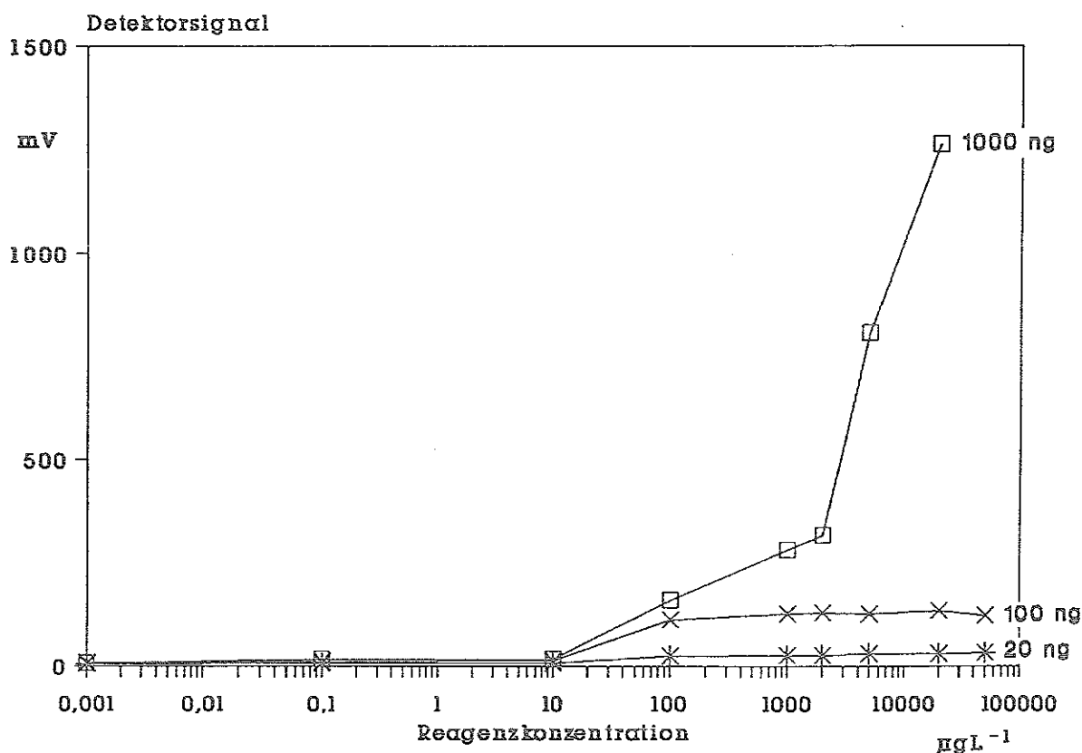
Abb. 3-18. Einfluß der Reagenzkonzentration auf die Signalhöhe. -Injektion: 3 verschiedene Mengen N-18-18. Jeweils Einfachbestimmungen. HPLC-Bedingungen: siehe Abschnitt 5.3.5.
