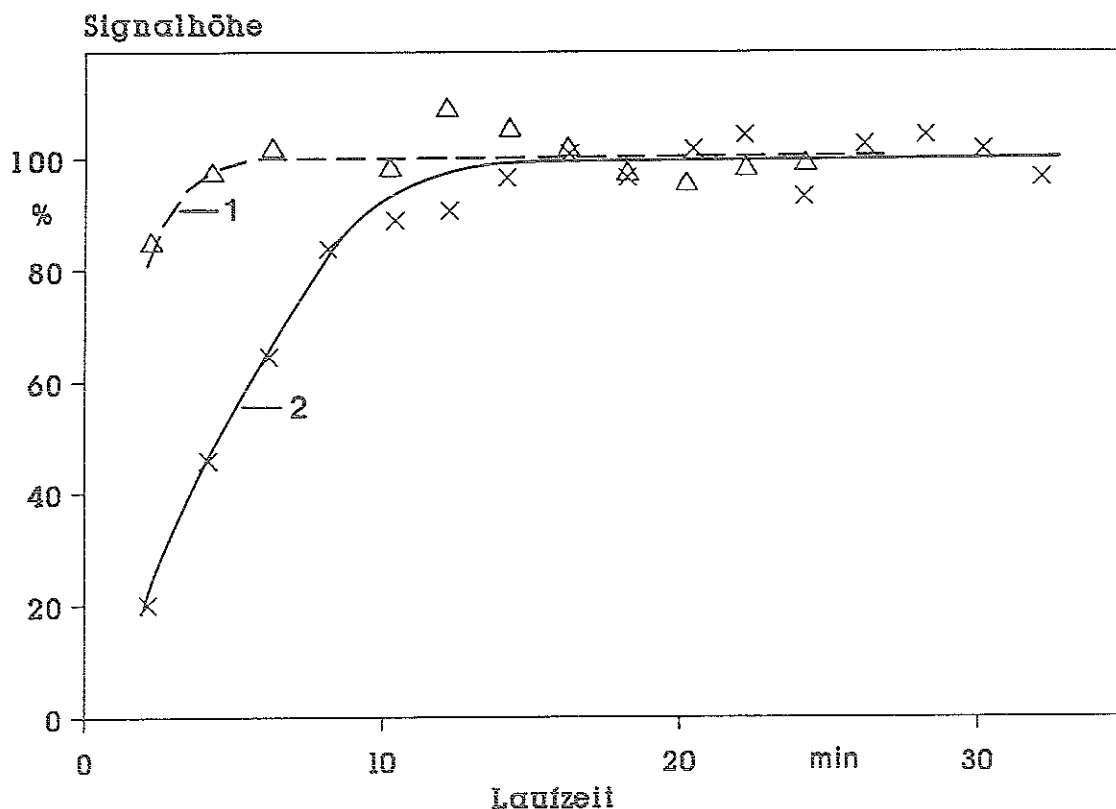
Abb. 3-20. Zeit- und Tensidmengenabhängigkeit des Detektorsignals bei verschiedenen Materialien der Detektorkapillare.
