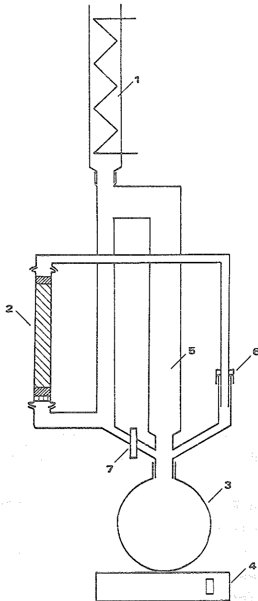
Abb. 3-6. Apparatur zur destillativen Elution von Tensiden von XAD-Säulen. - 1 Rückflußkühler; 2 Adsorbersäule; 3 Rundkolben; 4 Heizgerät; 5 Elutionsaufsatz; 6 Verschraubung; 7 Dreiwegehahn.
