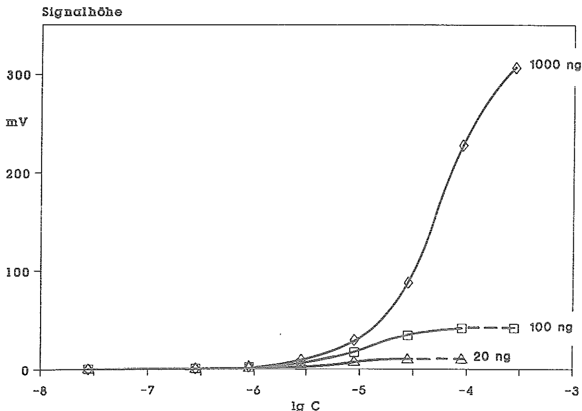
Abb. 3-25. Einfluß der Reagenzkonzentration auf die Signalhöhe. - Injektion: 3 verschiedene Mengen Natrium-decylsulfonat (C10-SO 3 ). Einfachbestimmungen. C Reagenzkonzentration.
