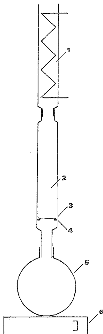
Abb. 3-7. Apparatur zur destillativen Heiextraktion von Tensiden aus Fluwasser-Filtrerrückstnden. - 1 Rckflukhler; 2 Extraktor; 3 Filter mit Rckstand; 4 Glaseinbuchtungen; 5 Vorlagekolben; 6 Heizgert.
