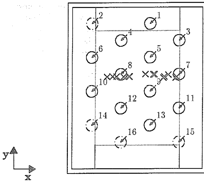
Abbildung 4.3: Projektion rekonstruierter Positionen des Schwerpunktes des Strahlflecks (x) auf die Matrix des Testmoduls (der Rand der Szintillatorfläche ist punktiert, bei der Testmessung nicht ausgelesene Photosensoren sind gestrichelt dargestellt)
