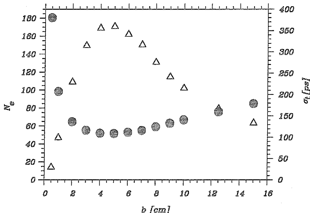
Abbildung 2.18: Ausbaustufe 2: Nachgewiesene Photoelektronenzahl der drei "günstigsten" Photomultiplier ( \triangle ) und resultierende Zeitauflösung ( \bullet ) als Funktion des Abstandes zwischen Szintillator (5 cm) und PM-Matrix
