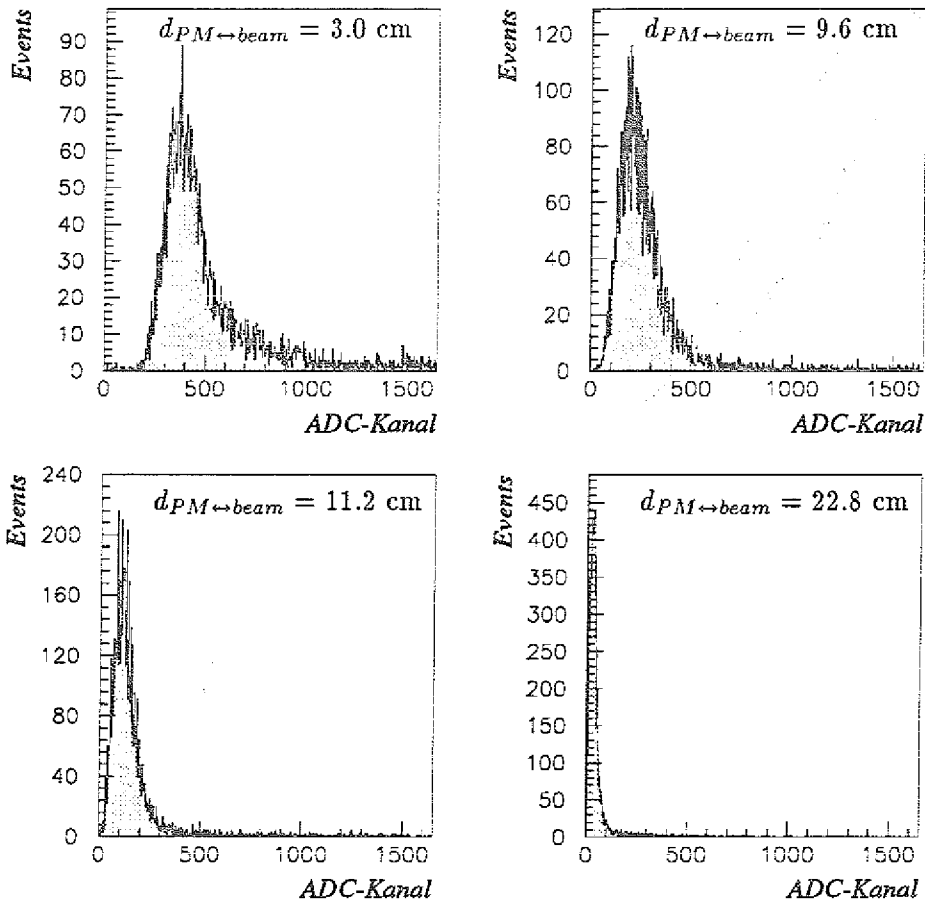
Abbildung 4.5: ADC-Spektren für unterschiedliche Photomultiplier bei einer Meßposition ( \pi^+ )
