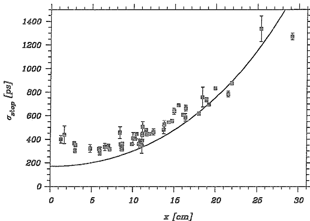
Abbildung 4.7: Zeitauflösung des Testmoduls für minimal ionisierende Pionen bei Auswertung eines Photomultipliers (■) im Vergleich mit Erwartungen gemäß der Monte-Carlo-Simulation (—). Im Falle nicht dargestellter Fehlerbalken liegt die Meßunsicherheit unterhalb der Symbolgröße.
