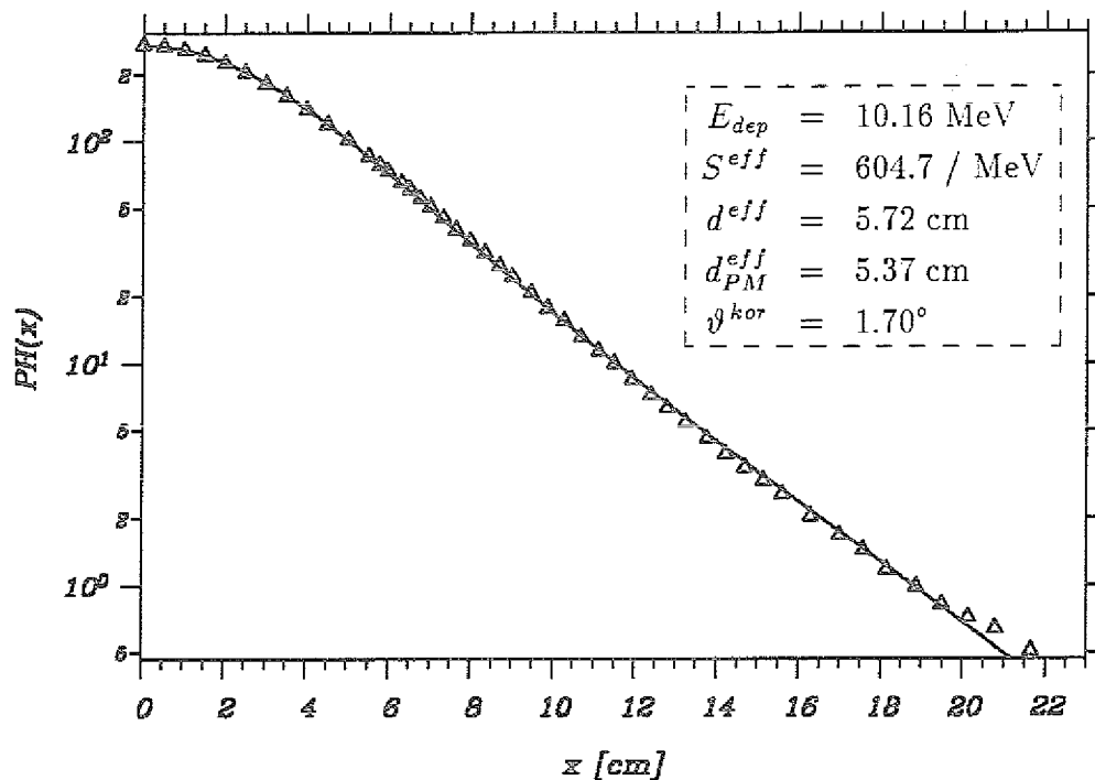
Abbildung 2.6: Pulshöhenfunktion für minimal ionisierende Protonen (Szintillatordicke d_{\text{zzi}} = 5 cm, Abstand zwischen Szintillator und PM-Matrix b = 4 cm). Die Ergebnisse der Monte-Carlo-Simulation sind durch Dreiecke repräsentiert, die durchgezogene Linie zeigt die Anpassung mit der Fit-Funktion.
