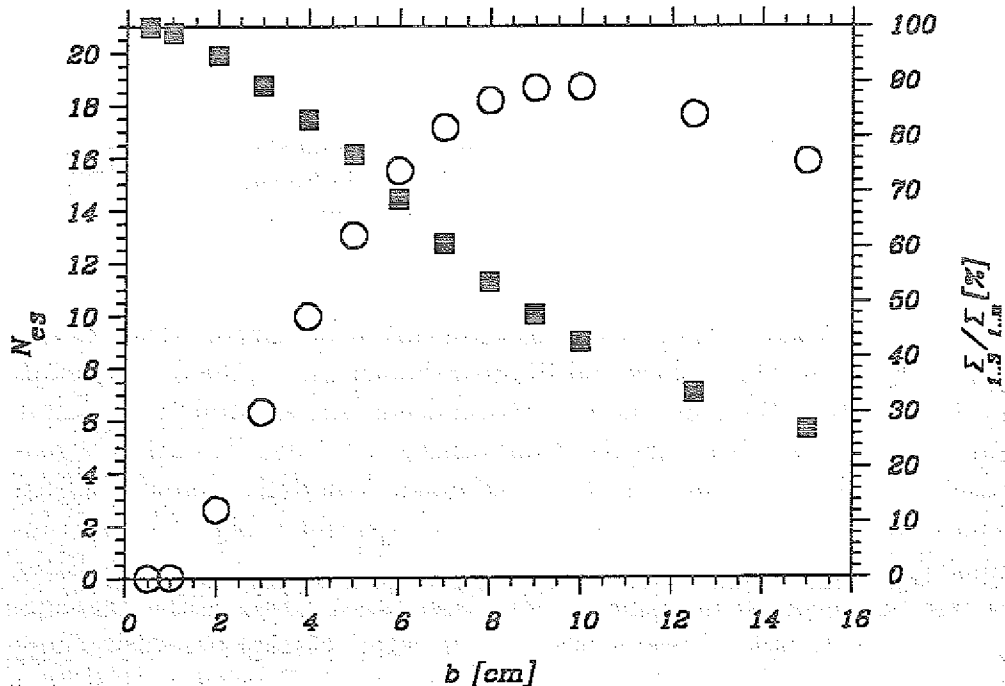
Abbildung 2.17: Ausbaustufe 2: Photoelektronenzahl in "drittbestem" PM ( \circ ) und Anteil der drei Photomultiplier mit höchstem Signal an der Pulshöhensumme ( \blacksquare ) als Funktion des Abstandes zwischen Szintillator (5 cm) und PM-Matrix
