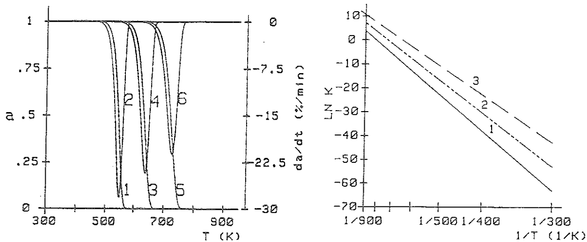
Abb. 4.6 und Abb. 4.7 Abhängigkeit der Zersetzungskinetik von der Aktivierungsenergie A = 1,5 \cdot 10^5 , Kurve 1 E = 180 kJ/mol, Kurve 2 E = 210 kJ/mol, Kurve 3 E = 240 kJ/mol Kurven 4,5,6 Geschwindigkeit der Massenabnahme
