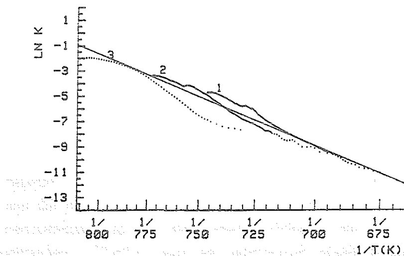
Abb. 6.2 Pyrolyse von PE, Kurve 1 HR=2°C/min, Kurve 2 HR=10°C/min, Kurve 3 HR=50°C/min, — Berechnung A=3,15E21 1/s, E=340 kJ/mol
