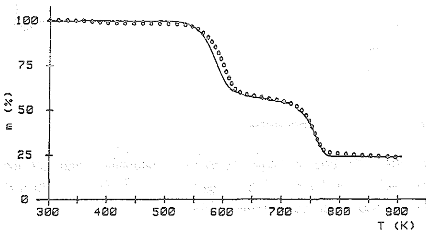
Abb. 6.18 Pyrolyse eines Zellulose-Aluminium-PE-Verbundes, HR=10°C/min, aus 64,6% Zellulose, 28,2% PE u. 7,2 % Aluminium, o Messung, — Berechnung
