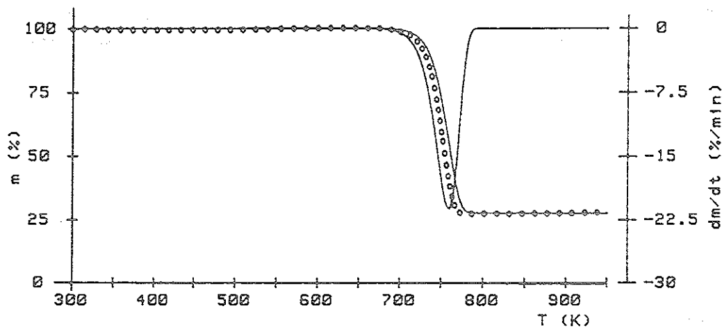
Abb. 6.5 Pyrolyse eines PE-Aluminium Verbunds, HR=10^{\circ}\text{C}/\text{min} , o PE-Aluminium-mit 72,5% PE u. 27,5% Al, — Berechnung A=3,15E21 1/s, E=340 kJ/mol
