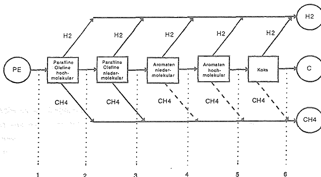
Abb. 6.34 Pyrolyse von PE
