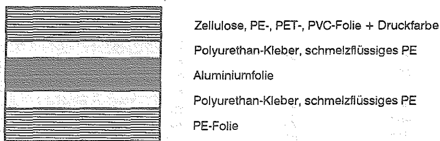
Abb. 1.1 Aufbau von Verbundverpackungen
