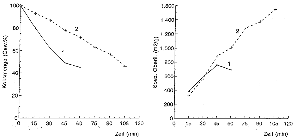
Abb. 7.1 Wasserdampfaktivierung von Zellulosekoks und PET-Koks bei 900°C links: Aktivkohsmenge, 1 Zellulosekoks, 2 PET-Koks rechts: spezifische Oberfläche (BET), 1 Zellulosekoks, 2 PET-Koks
