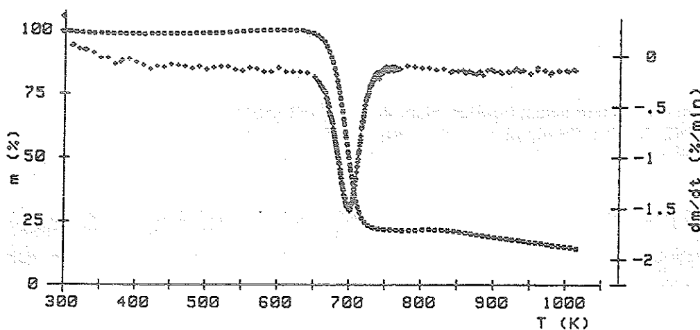
Abb. 6.6 Pyrolyse von PET, HR=30^{\circ}\text{C}/\text{min}
