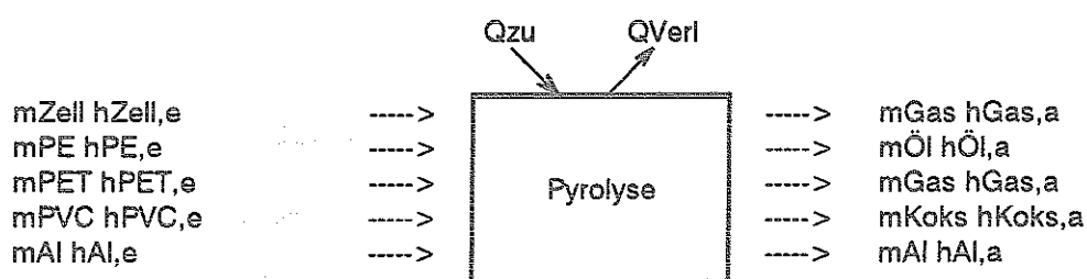
Abb. 5.2 Energiebilanz
