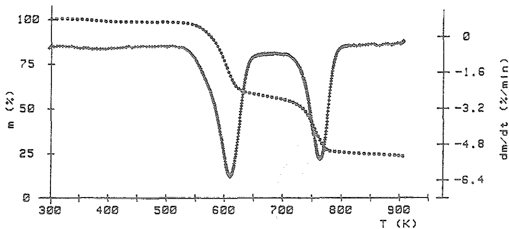
Abb. 6.17 Pyrolyse eines Zellulose-Aluminium-PE-Verbundes, HR=10°C/min, mit 64,6% Zellulose, 28,2% PE u. 7,2 % Aluminium
