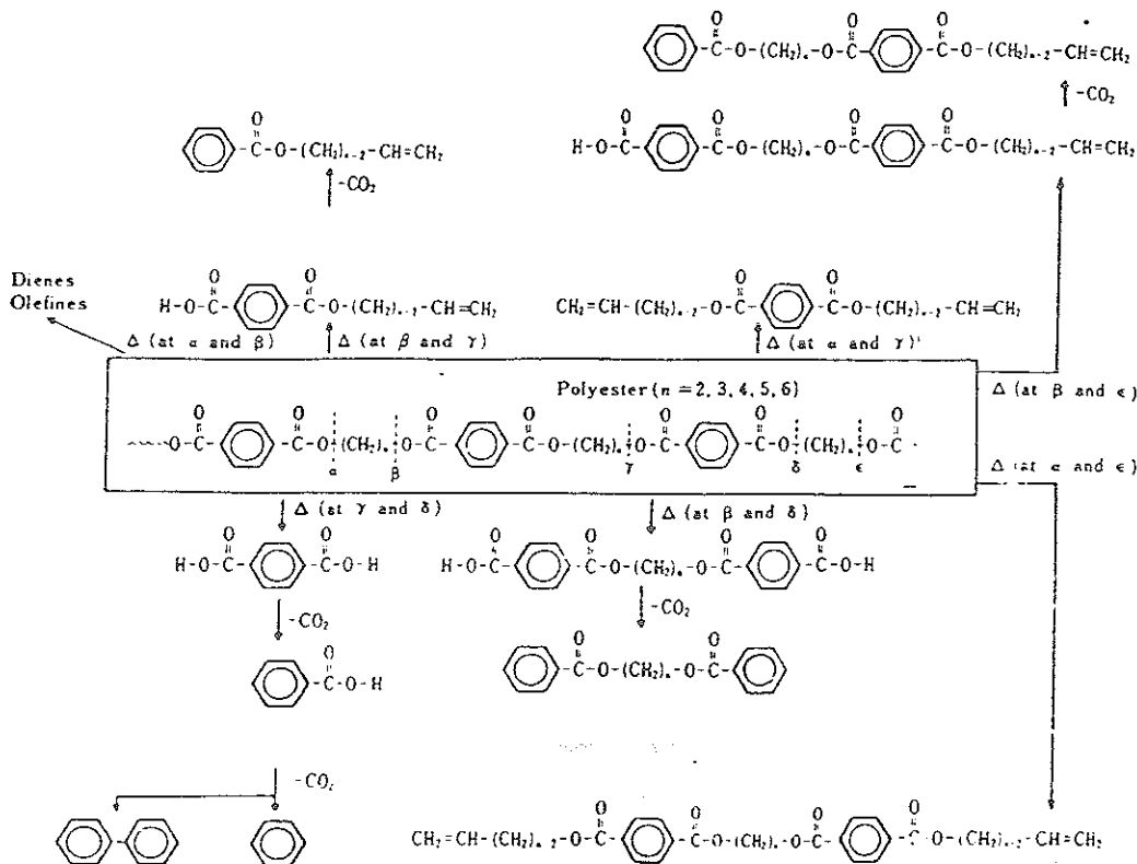
Abb. 3.1 Thermische Zersetzung von PET, nach Ohtani, Kimura und Tsuge /36/
