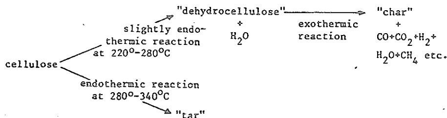
Abb. 6.15 Pyrolyse von Zellulose, Reaktionsschema nach Kilzer und Broido /78/
