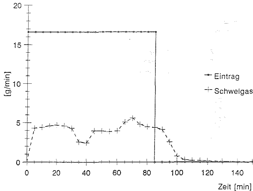
Abb. 6.28 Pyrolyseverlauf für einen PE-Aluminium-Verbund 620°C, mit 23% PE, 74% Al, 3% PU
