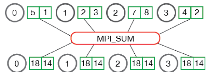
MPI_Allreduce
