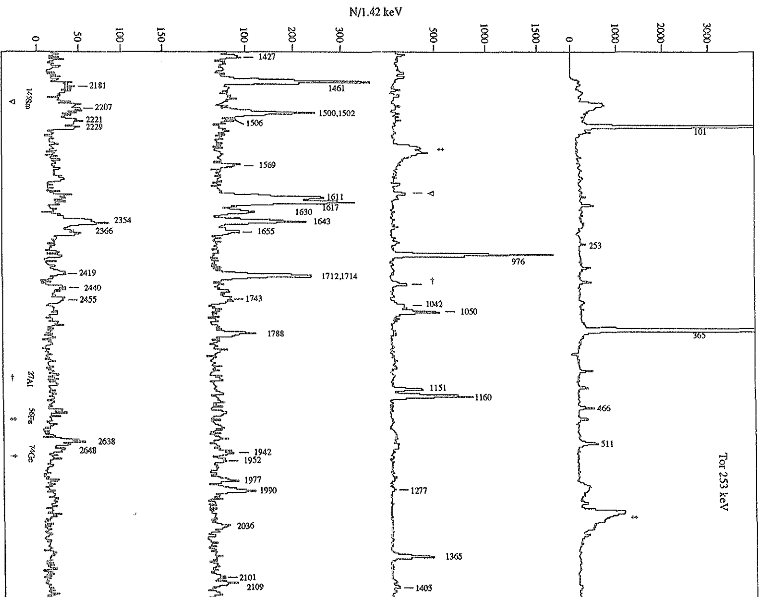
Fig. 16: \gamma\gamma -Koinzidenzen gemessen unter 90 Grad aus der Reaktion ^{144}\text{Sm}(^6\text{Li},3n)^{147}\text{Tb}
