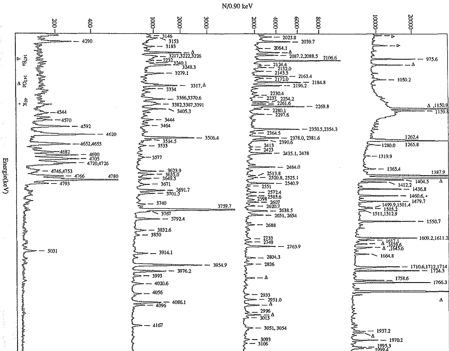
Fig. 25: Compton-unterdrücktes Gammaspektrum für Masse A=147 gemessen an Isolde mit 40 Sekunden Sammel- und 64 Sekunden Meßzeit. Die Gammaenergien sind bei den ^{147}\text{Tb} -Übergängen angegeben. Die Messung dauerte 8 Stunden.
