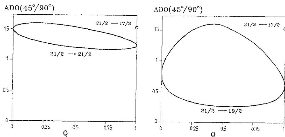
Fig. 18: Berechnete ADO-Winkelverteilungsverhältnisse als Funktion der Quadrupolbeimischung Q bei den Winkeln 45 Grad und 90 Grad für nicht- abgeschwächte Übergänge 21/2 \rightarrow 21/2 und 21/2 \rightarrow 19/2 , sowie für den reinen Quadrupolzerfall 21/2 \rightarrow 17/2 .
