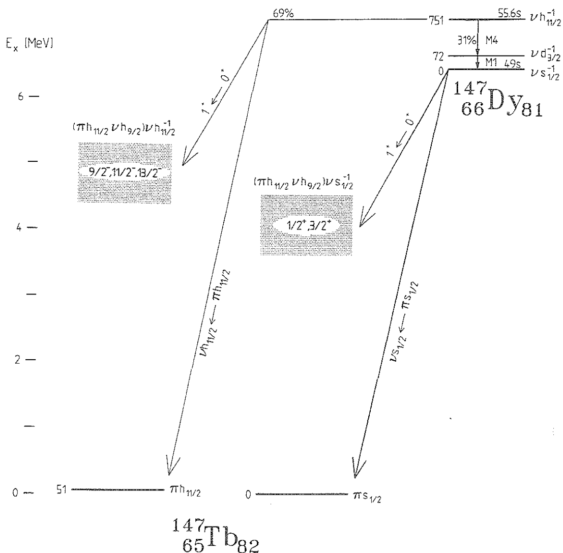
Fig. 24: Die \beta -Zerfälle beider ^{147}\text{Dy} -Isomere
