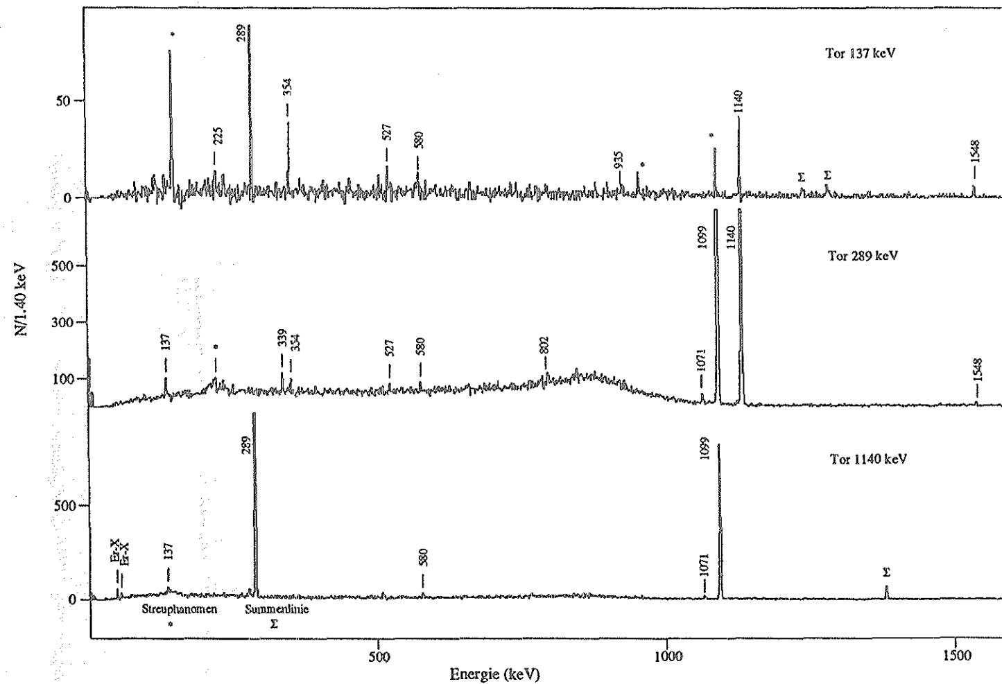
Fig. 46: \gamma\gamma -Koinzidenzspektren von Übergängen aus dem ^{151}\text{Er} -E3-Isomerzerfall
