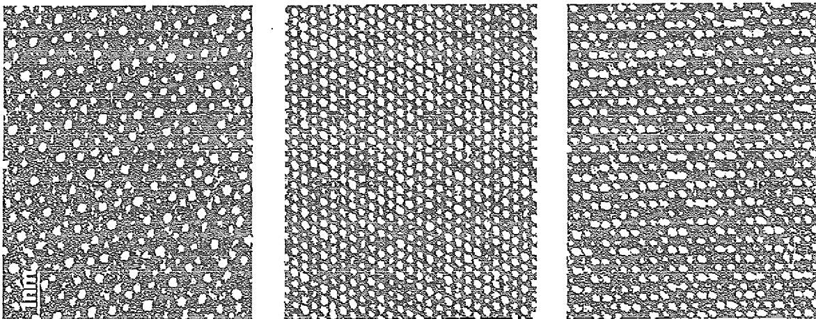
Abb. 2.10: Elektronenmikroskopische Hochauflösungsaufnahmen, gewonnen an \text{Al}_{86}\text{Mn}_{14} (aus [37]).
