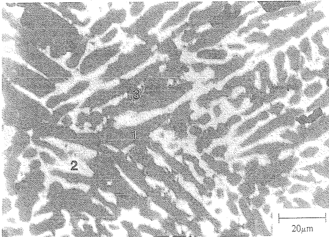
Abb. 5.30 REM-Bild des Gefüges der maximal unterkühlten \text{Al}_{64}\text{Cu}_{22}\text{Co}_{14} -Probe, deren Temperatur-Zeit-Profil in Abb. 5.27c gezeigt wurde.
