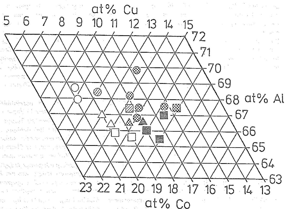
Abb. 5.40 Mittlere Zusammensetzung der D-Phase in Abhängigkeit von der Nukleations- temperatur. Die verwendeten Symbole repräsentieren dabei die Probenzusammensetzung, die Füllung die Nukleationstemperatur T_N , wie nachfolgender Tabelle zu entnehmen ist.
