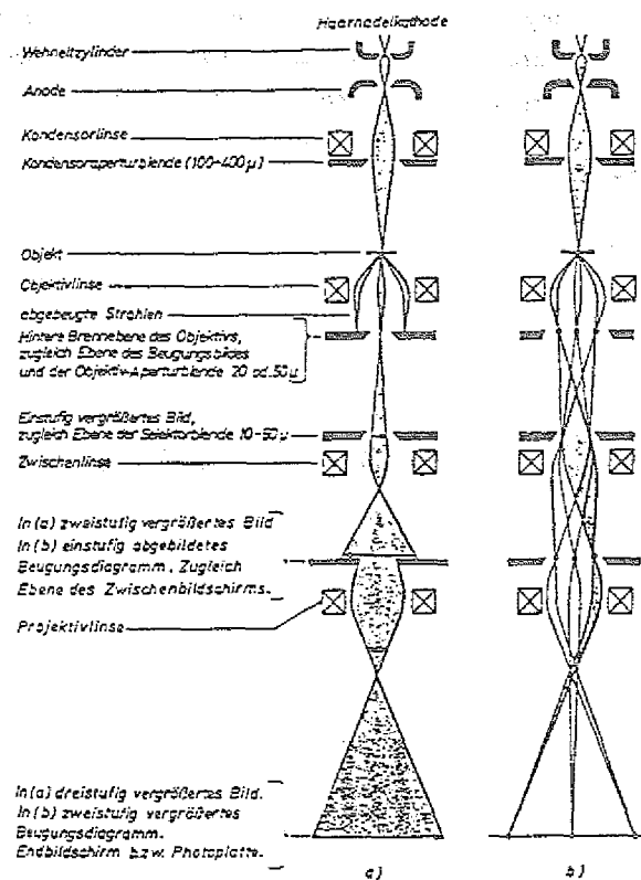
Abb. 4.9 Schematische Darstellung des Strahlengangs eines Transmissionselektronenmikroskops bei einer Hellfeldabbildung (a) und bei Elektronenbeugung (b) (aus [24]).
