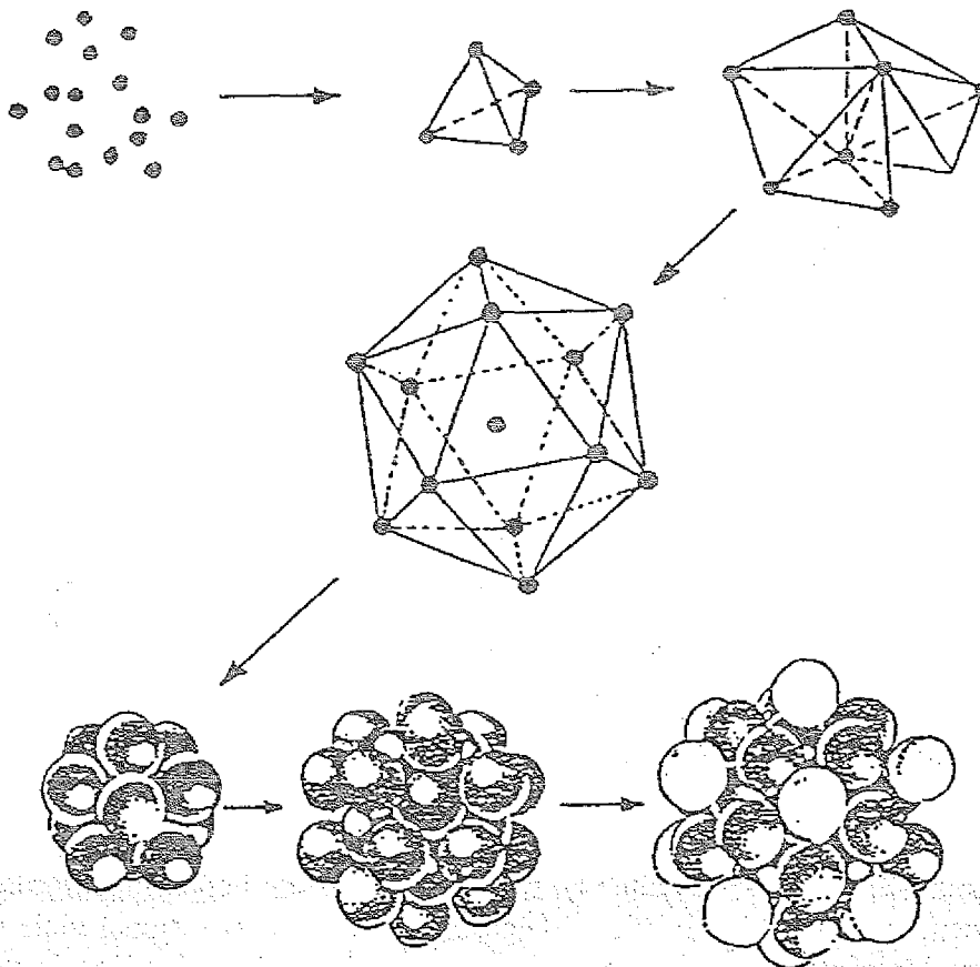
Abb. 3.5: Bildung von Clustern mit ikosaedrischer Symmetrie.
