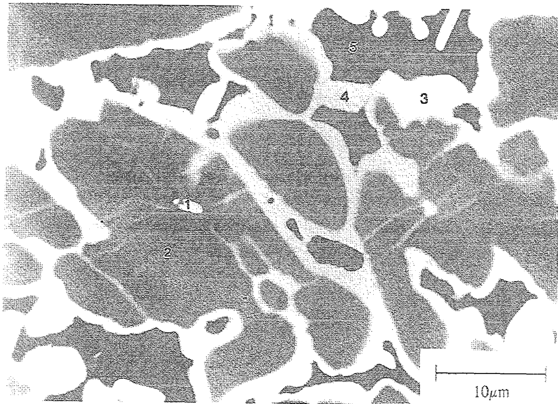
Abb. 5.6: REM-Aufnahme einer \text{Al}_{62.5}\text{Cu}_{27}\text{Co}_{10.5} -Probe, die in der Levitationsanlage auf Grund von Probenkontamination nicht signifikant unterkühlt hat.
