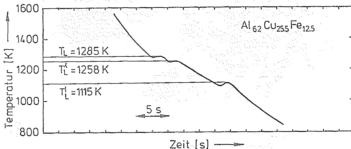
Abb. 5.22 Temperatur-Zeit-Profil einer kaum unterkühlten \text{Al}_{62}\text{Cu}_{25.5}\text{Fe}_{12.5} -Probe.
