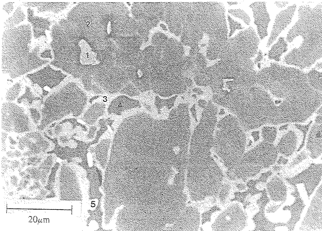
Abb. 5.39 REM-Aufnahme einer kaum unterkühlten \text{Al}_{64}\text{Cu}_{22}\text{Co}_{14} -Probe.
