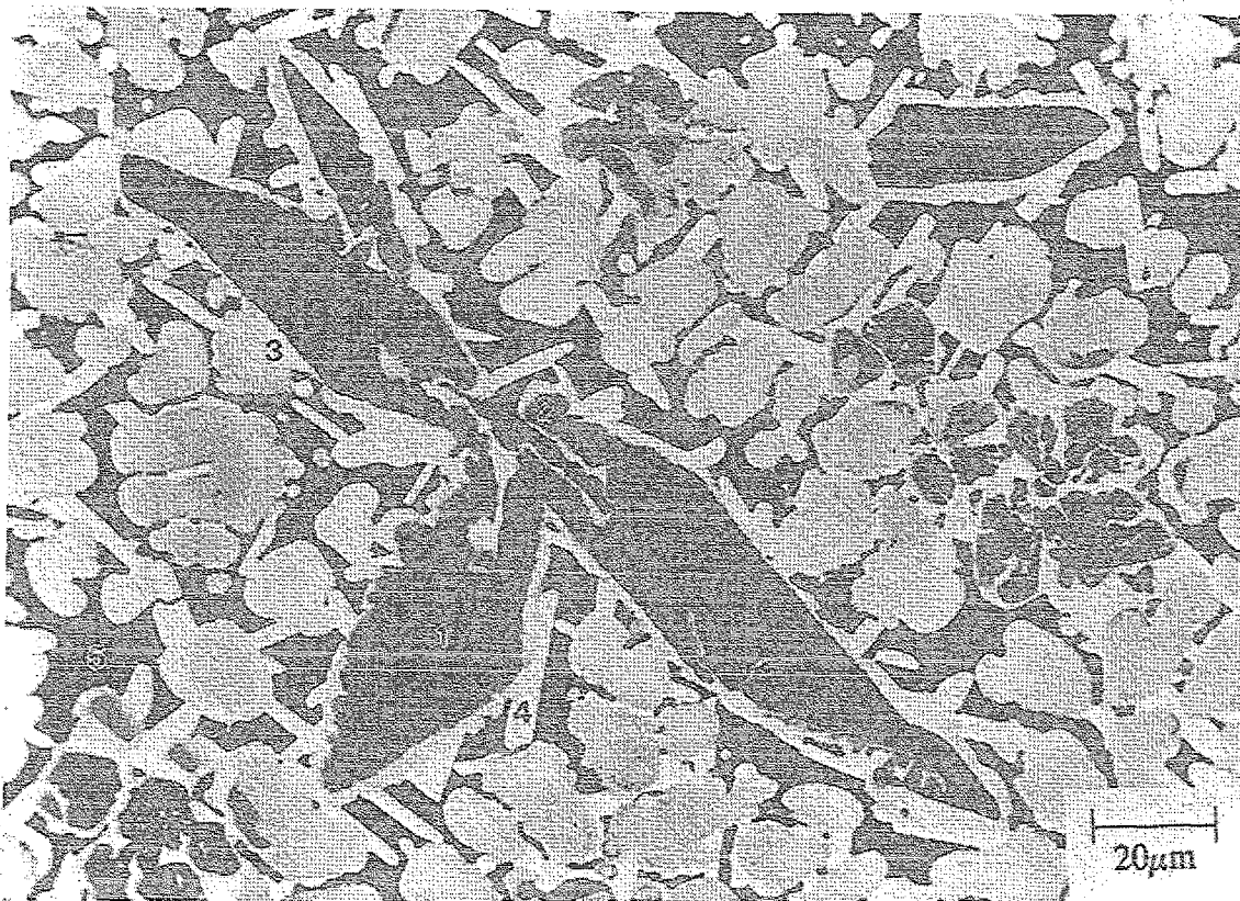
Abb. 5.20 REM-Aufnahme der zum Temperatur-Zeit-Profil (Abb. 5.19) gehörigen, kaum unterkühlten, \text{Al}_{60}\text{Cu}_{34}\text{Fe}_6 -Probe.
