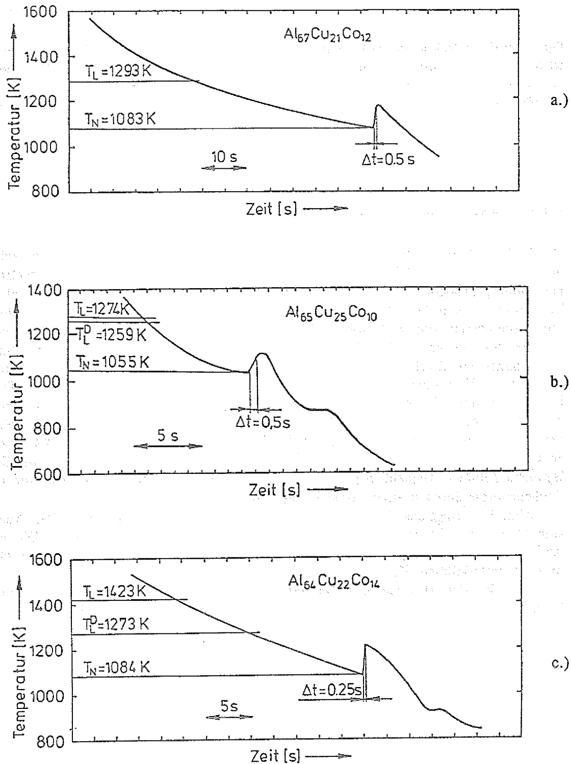
Abb. 5.27 Temperatur-Zeit-Profile von Levitationsexperimenten, in denen maximale Unterkühlungen an Al-Cu-Co-Proben unterschiedlicher Zusammensetzung erreicht wurden.
