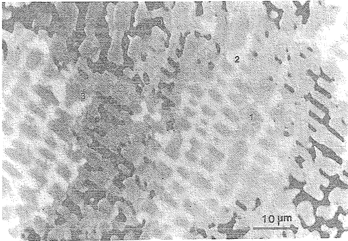
Abb. 5.28 REM-Bild des Gefüges der maximal unterkühlten \text{Al}_{67}\text{Cu}_{21}\text{Co}_{12} -Probe, deren Temperatur-Zeit-Profil in Abb. 5.27a gezeigt wurde.
