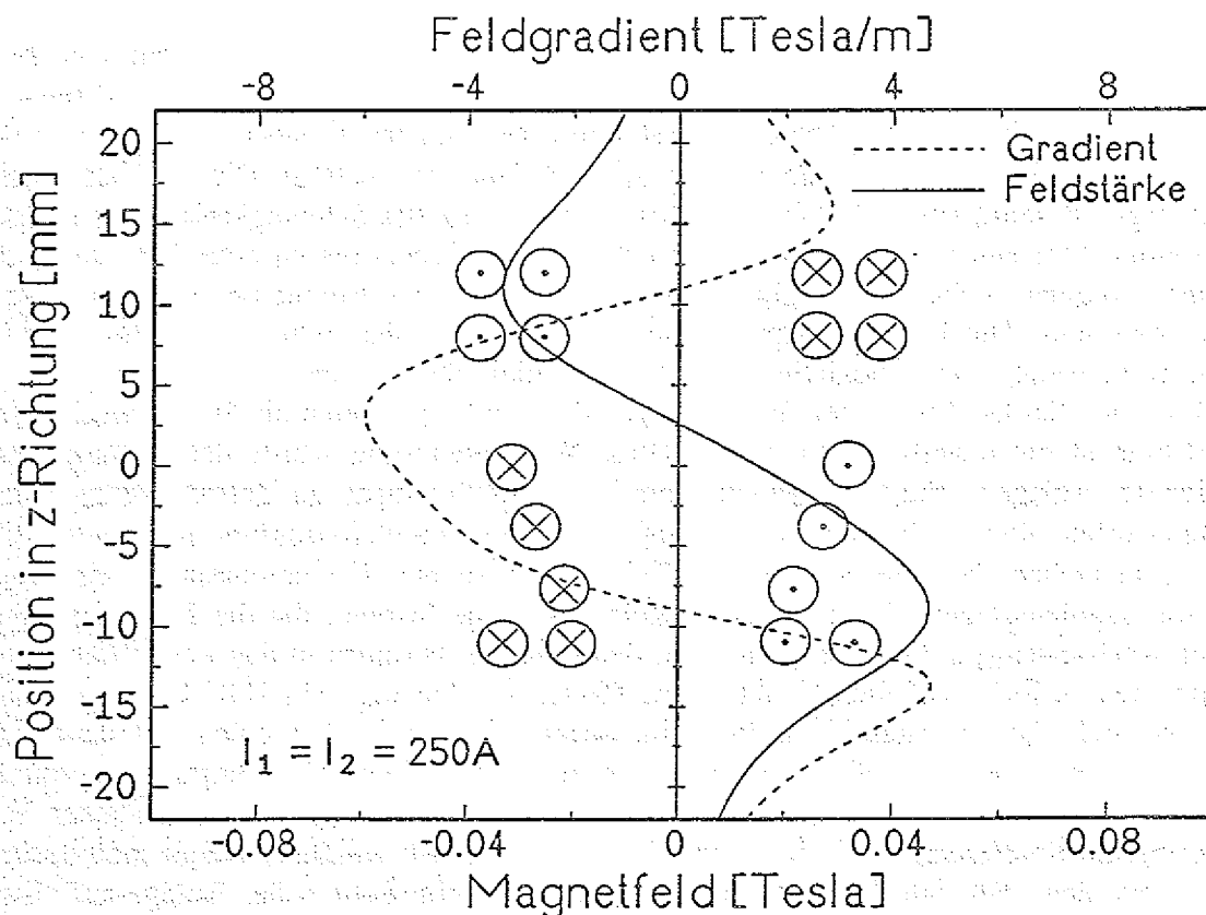
Abb. 4.5 Maßstabsgerechte Darstellung des für die Unterkuhlungsexperimente an quasikristallbildenden Legierungen entwickelten Spulensystems, sowie berechnete magnetische Feldstärke B(z) und Feldgradient dB(z)/dz als Funktion des Ortes z (Spulenströme I_1 = I_2 = 250 A).
