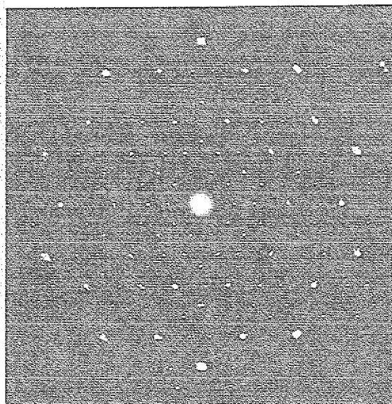
Abb. 5.48 Elektronenbeugungsbilder, gewonnen an einem dekadagonalen Quasikristall ([00001]-Orientierung) der splatgekühlten \text{Al}_{64}\text{Cu}_{22}\text{Co}_{14} -Probe.
