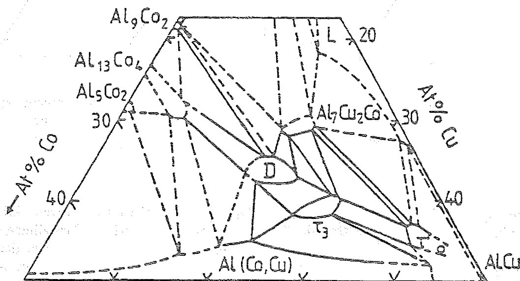
Abb. 4.14 Ausschnitt aus dem Phasendiagramm von Al-Cu-Co bei 873 K (aus [181]).
