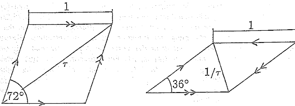
Abb. 2.3: Die Elemente des Penrose-Musters, die "dicke" und die "dünne" Raute.
