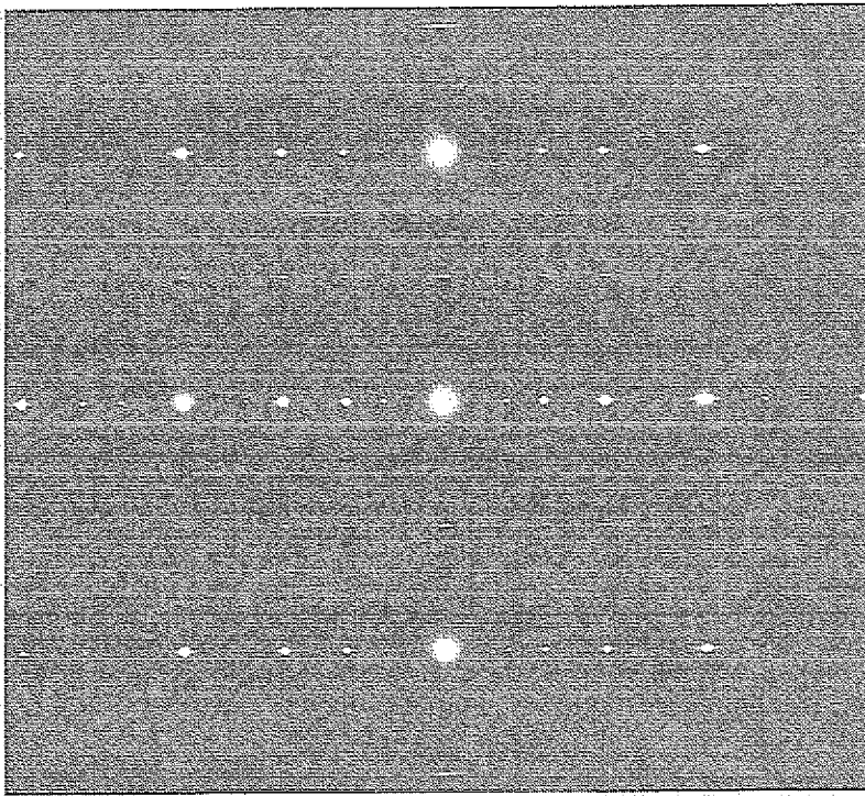
Abb. 5.34 TEM-Beugungsbild der [1\bar{2}100] -Zonenachse der maximal unterkühlten \text{Al}_{64}\text{Cu}_{22}\text{Co}_{14} -Probe.
