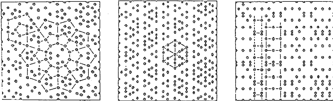
Abb. 2.9: Unterschiedliche Projektionen eines dreidimensionalen quasiperiodischen Gitters (aus [37]).
