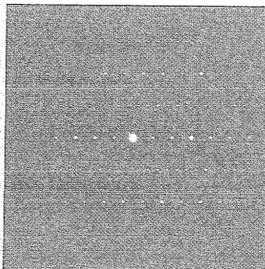
Abb. 5.16 Elektronenbeugungsbild der [1\bar{1}0] -Zonenachse der \lambda -Phase, welches an einer maximal unterkühlten \text{Al}_{62}\text{Cu}_{25.5}\text{Fe}_{12.5} -Probe gewonnen wurde.
