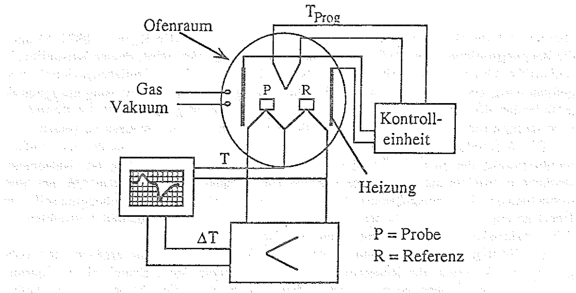
Abb. 4.12 Schematische Darstellung einer DTA-Anlage (aus [166]).
