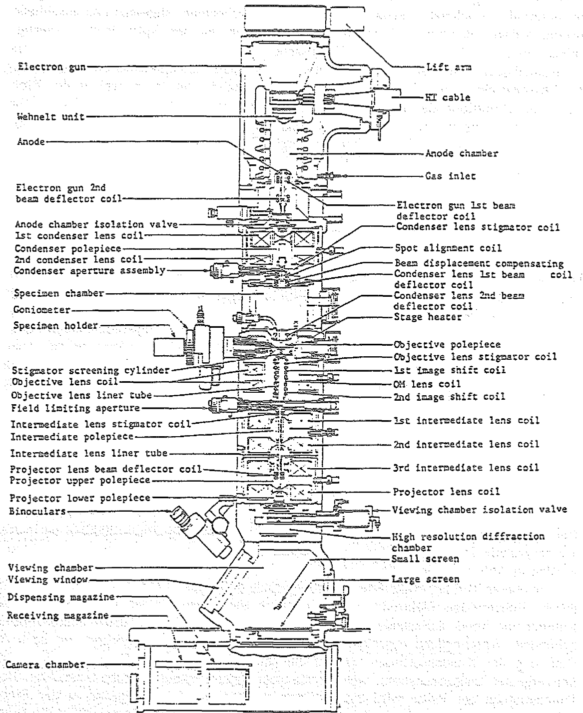
Abb. 4.8 Aufbau des Transmissionselektronenmikroskops JEOL 2000EX (aus [156]).
