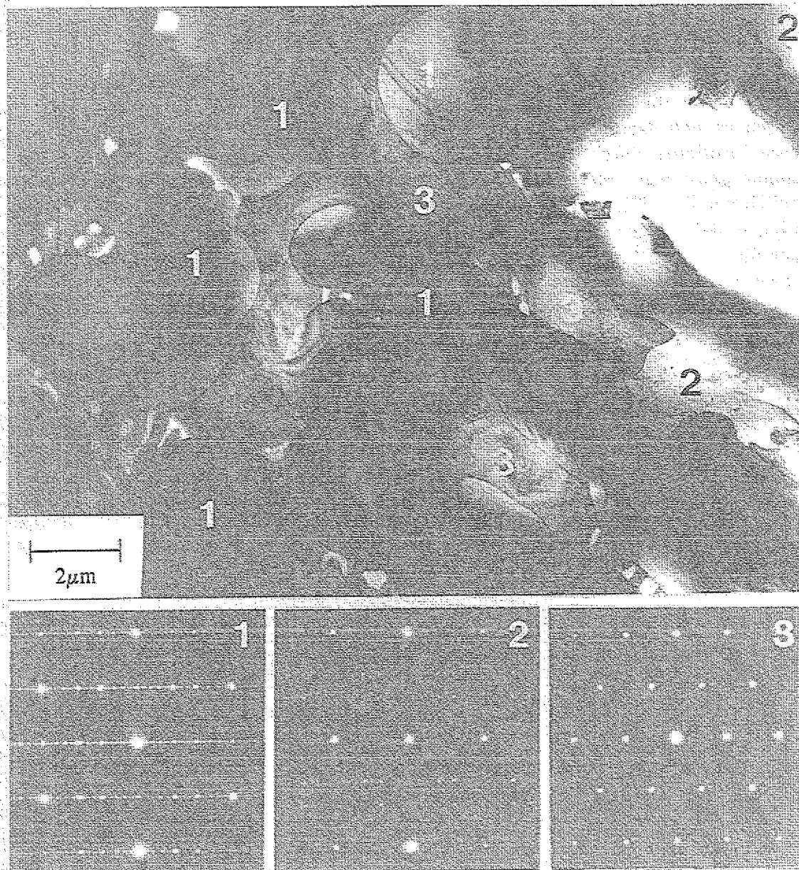
Abb. 5.32 TEM-Hellfeldbild gewonnen an einer maximal unterkühlten \text{Al}_{67}\text{Cu}_{21}\text{Co}_{12} -Probe. Die Nebenbilder zeigen Elektronenbeugungsbilder, die an verschiedenen Bereichen der Probe beobachtet wurden.
