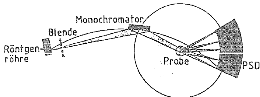
Abb. 4.11 Strahlengang des Röntgenpulverdiffraktometers (aus [163]).
