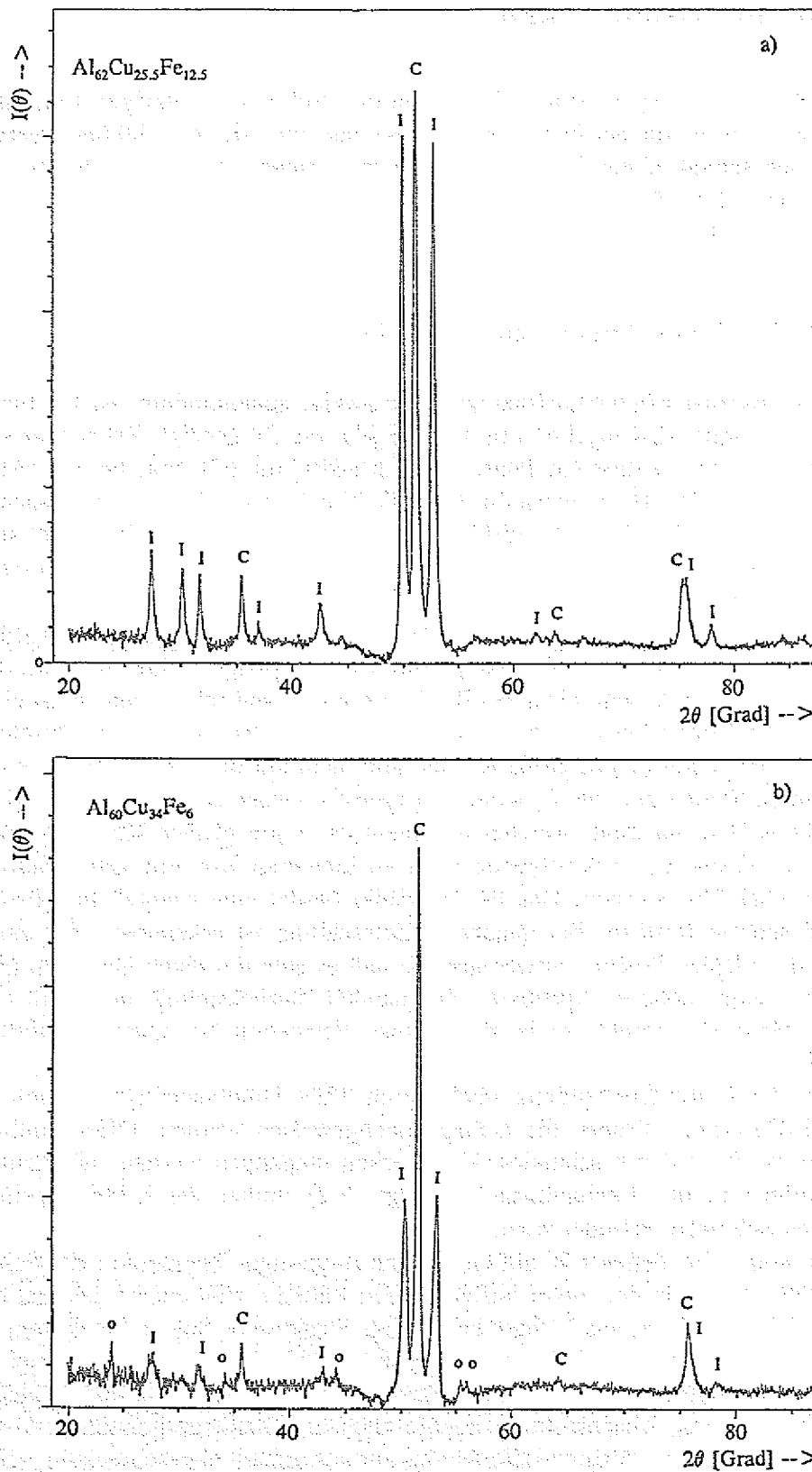
Abb. 5.41 Röntgendiffraktogramme splatgekühlter Al-Cu-Fe-Proben.
