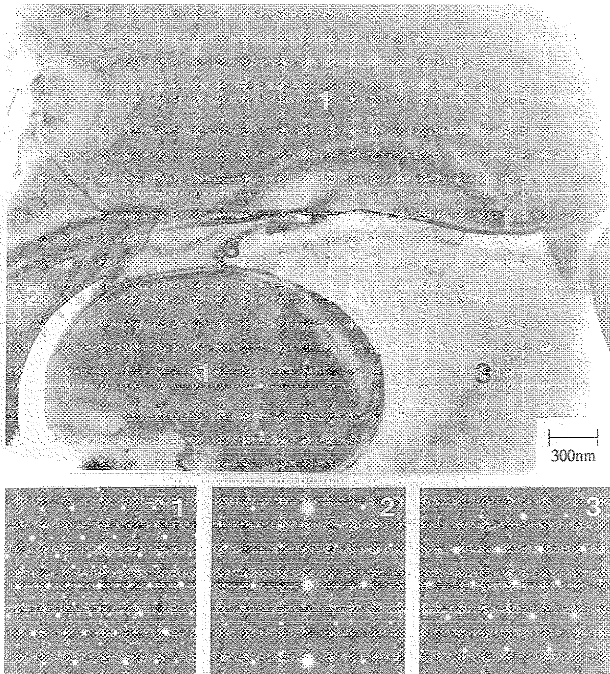
Abb. 5.15: TEM-Hellfeldbild, gewonnen an der maximal unterkühlten \text{Al}_{60}\text{Cu}_{34}\text{Fe}_6 -Probe. Die Nebensbilder zeigen Elektronenbeugungsbilder, die an den gekennzeichneten Bereichen des Hellfeldbilds gewonnen wurden: (1) I-Phase (5-zählige Achse), (2) \tau -Phase ([110]-Zonenachse), (3) \text{Al}_2\text{Cu} ([111]-Zonenachse).
