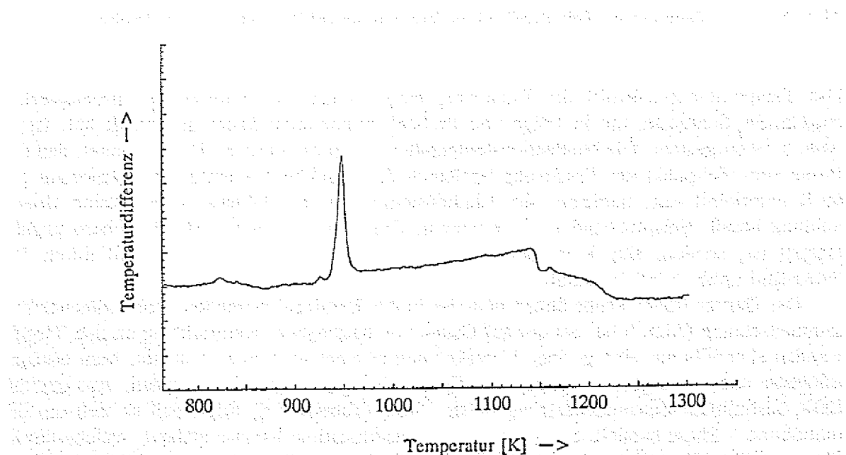
Abb. 5.18 DTA-Aufheizkurve, gewonnen an der maximal unterkühlten \text{Al}_{58}\text{Cu}_{34}\text{Fe}_8 -Probe, deren Temperatur-Zeit-Profil in Abb. 5.10b gezeigt wurde.
