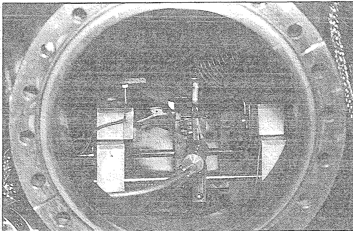
Abb. 9.1: Foto der Vorrichtungen zum Bedampfen der Proben mit Kupfer und zum Ausschleusen der Proben
