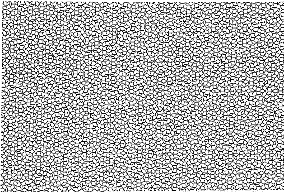
Abb. 2.4: Penrose-Muster
