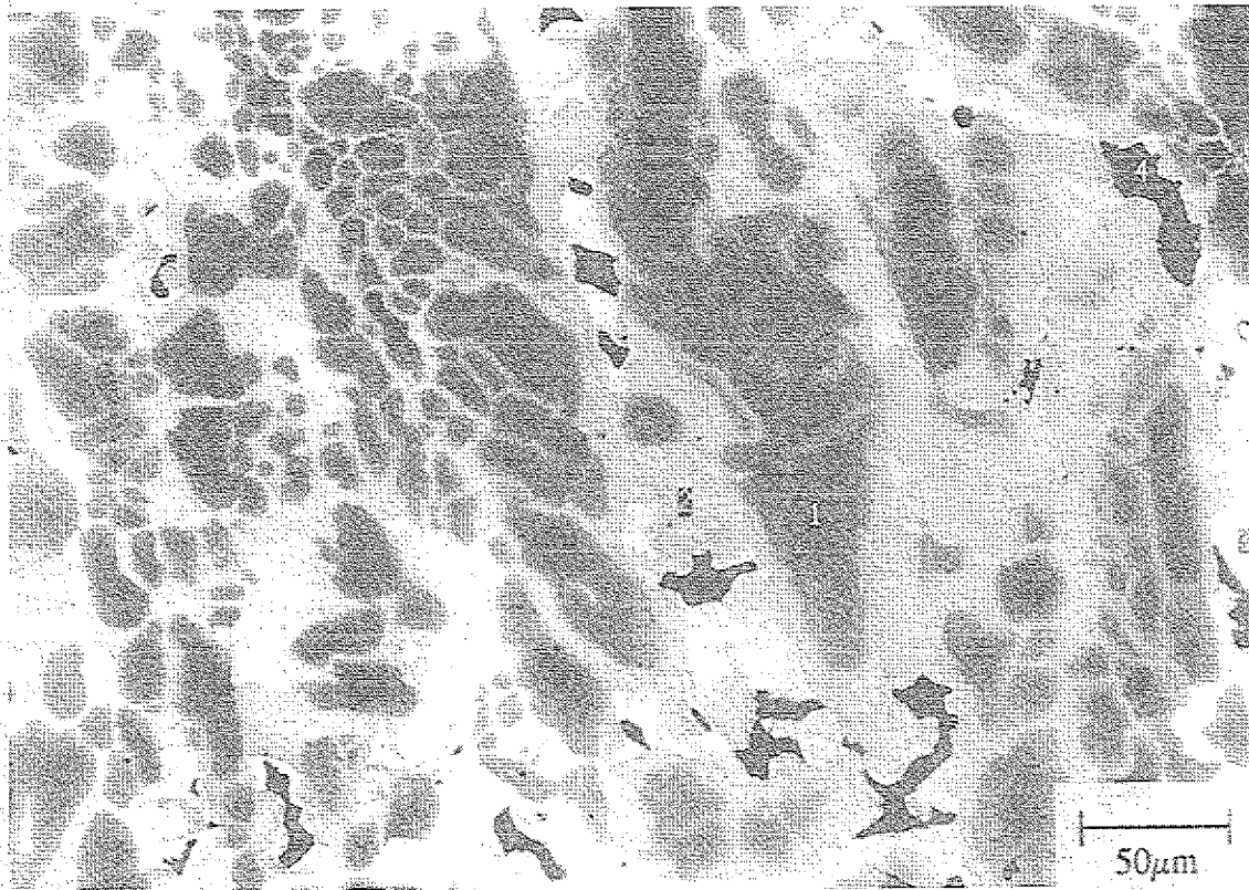
Abb. 5.4 REM-Aufnahme der in der DTA-Anlage erstarrten \text{Al}_{60}\text{Cu}_{34}\text{Fe}_6 -Probe. Die Zusammensetzungen der einzelnen Phasen sind Tabelle 5.2 zu entnehmen.
