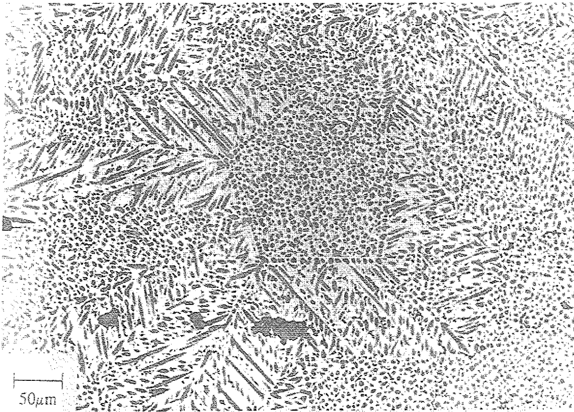
Abb. 5.25 REM-Aufnahme einer bei T_N=1055\text{ K} ( \Delta T^I=45\text{ K} ) erstarrten \text{Al}_{60}\text{Cu}_{34}\text{Fe}_6 -Probe. Die 5-zählige Symmetrie der I-Phase schlägt sich in der Wachstumsrichtung der Dendriten nieder.
