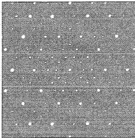
Abb. 2.1: Elektronenbeugungsbild mit 10-zähliger Symmetrie, gewonnen an einer \text{Al}_{60}\text{Cu}_{34}\text{Fe}_6 -Probe (Ikosaedrische Phase).
