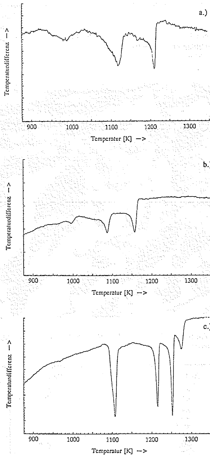
Abb. 5.1 DTA Abkühlkurven von Al-Cu-Fe-Proben unterschiedlicher Zusammensetzung. a.) \text{Al}_{58}\text{Cu}_{34}\text{Fe}_8 , b.) \text{Al}_{60}\text{Cu}_{34}\text{Fe}_6 , c.) \text{Al}_{62}\text{Cu}_{25.5}\text{Fe}_{12.5}
