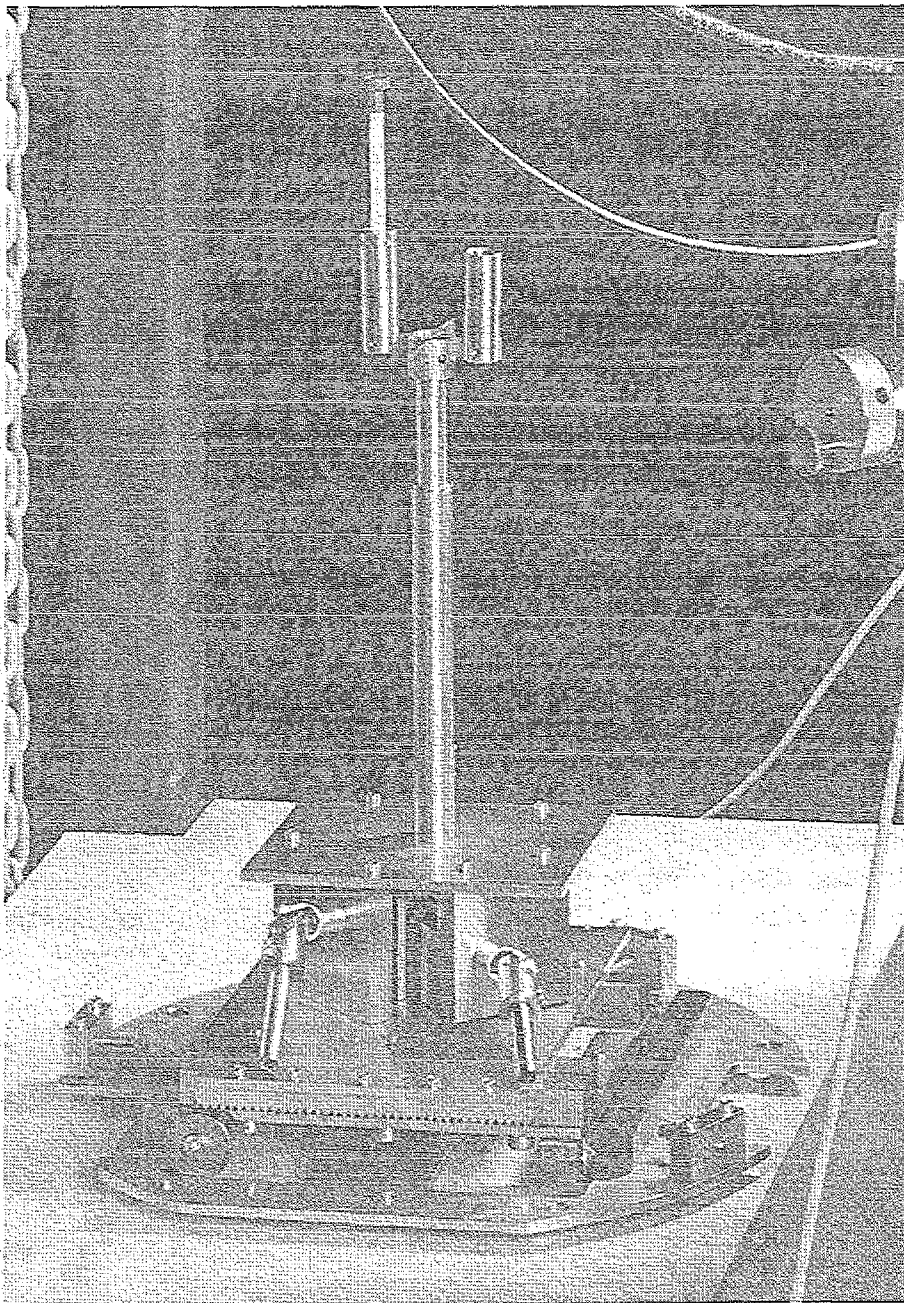
Abb. 4.4: Der Probenmanipulator.
