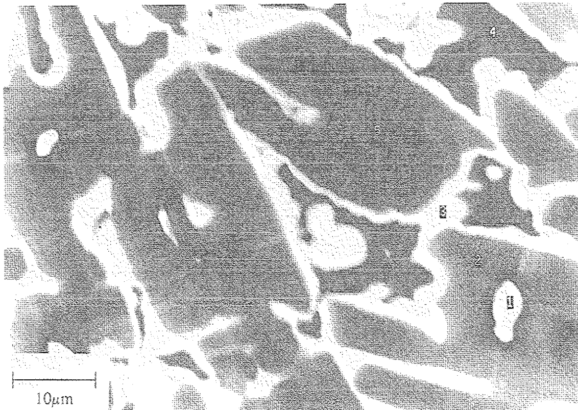
Abb. 5.38 REM-Aufnahme einer kaum unterkühlten \text{Al}_{65}\text{Cu}_{25}\text{Co}_{10} -Probe.
