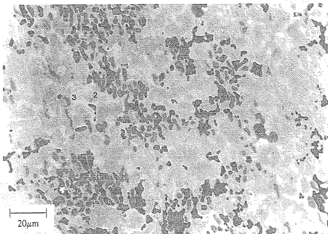
Abb. 5.13 REM-Bild des Gefüges der maximal unterkühlten \text{Al}_{62}\text{Cu}_{25.5}\text{Fe}_{12.5} -Probe, deren Temperatur-Zeit-Profil in Abb. 5.10c gezeigt wurde.
