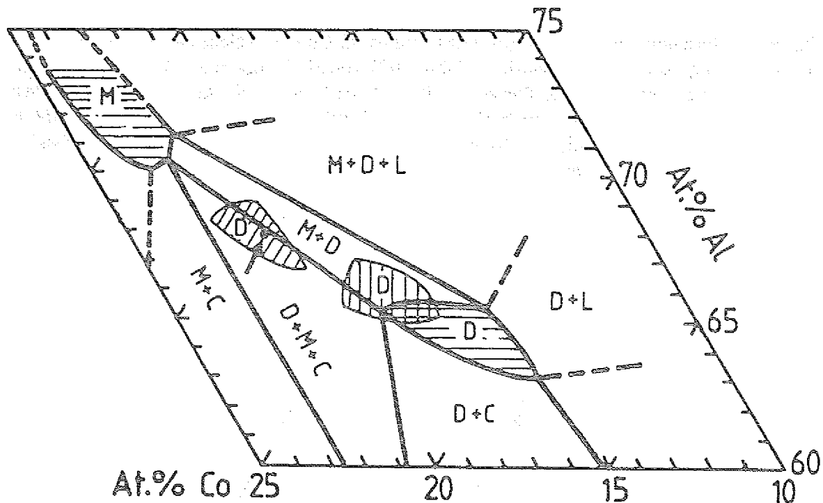
Abb. 4.15 Lage des Einphasengebiets der dekalonalen Phase bei Temperaturen von 1073 K (waagrecht schraffiert), von 1173 K (senkrecht schraffiert) und von 1273 K (schräg schraffiert). Außerdem: Lage der monoklinen Phase M sowie der Mehrphasengebiete bei 1073 K (aus [49]).
