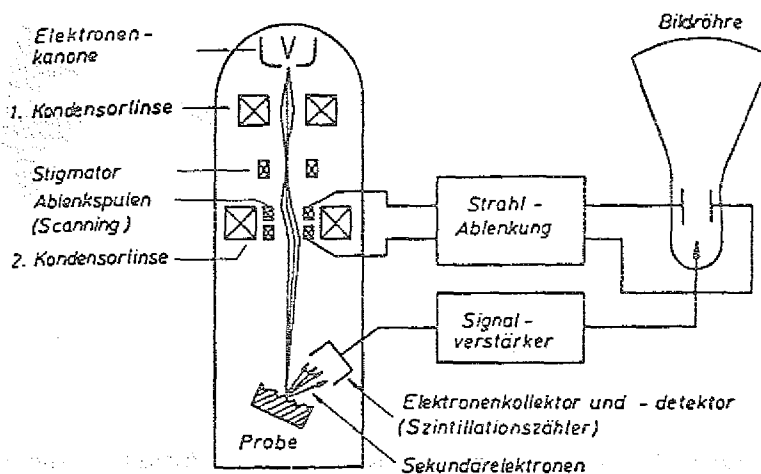
Abb. 4.10 Schematische Darstellung eines Rasterelektronenmikroskops (aus [24]).
