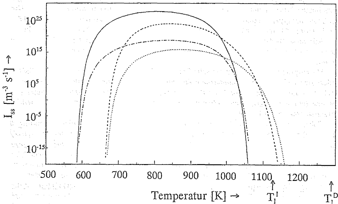
Abb. 6.1 Nukleationsrate I_{ss} als Funktion der Temperatur berechnet für die I-Phase in Al-Cu-Fe und die D-Phase in Al-Cu-Co.
