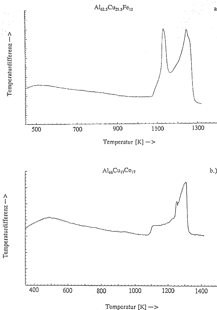
Abb. 5.8 DTA-Meßkurven beim ersten Aufschmelzen. a.) einphasig ikosaedrische \text{Al}_{62.5}\text{Cu}_{25.5}\text{Fe}_{12} -Probe b.) einphasig dekadonale \text{Al}_{66}\text{Cu}_{17}\text{Co}_{17} -Probe
