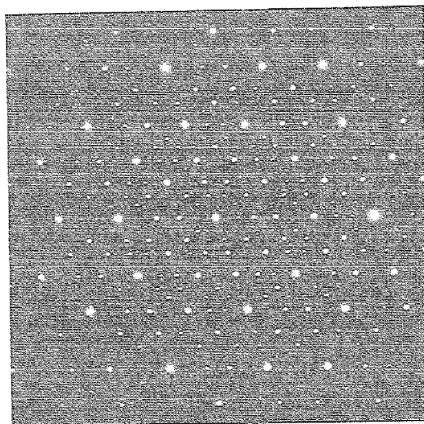
Abb. 5.43 TEM-Beugungsbild eines quasikristallinen Korns in fünfzähliger Orientierung.
