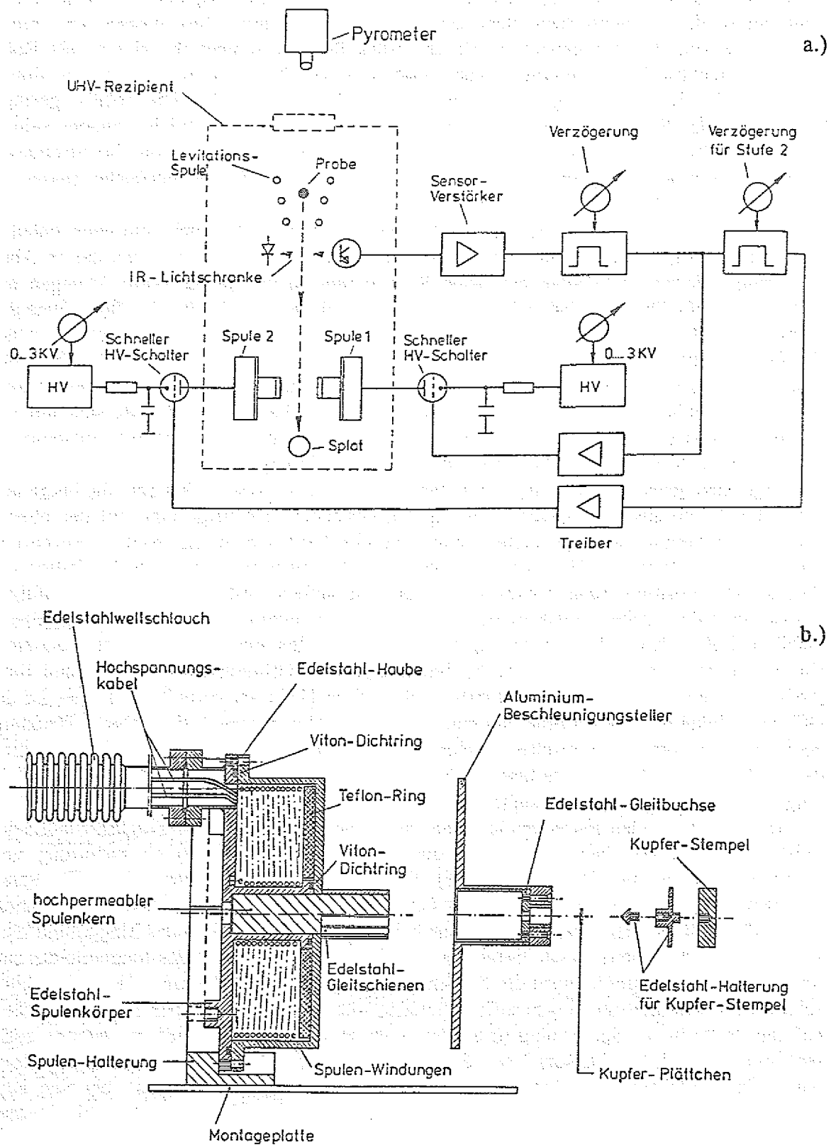
Abb. 4.6 Schematische Darstellung des Splatkühlers. a.) Funktionsschema b.) Aufbau des Schlagbolzensystems
