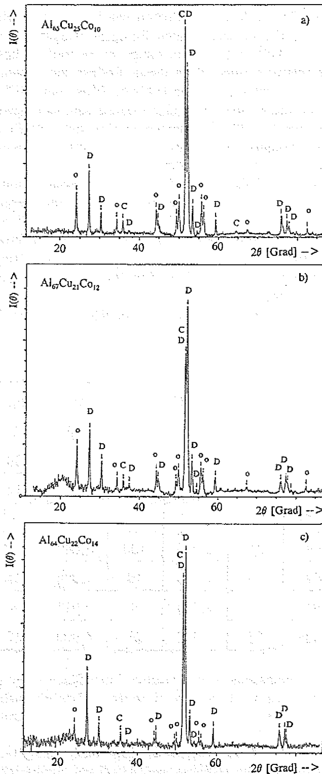
Abb. 5.35 Röntgenbeugungsbilder der maximal unterkühlten Al-Cu-Co-Proben a.) \text{Al}_{65}\text{Cu}_{25}\text{Co}_{10} , b.) \text{Al}_{67}\text{Cu}_{21}\text{Co}_{12} und c.) \text{Al}_{64}\text{Cu}_{22}\text{Co}_{14} D: D-Phase, C: kubische Phase (CsCl-Typ) und o: \text{Al}_2\text{Cu} .
