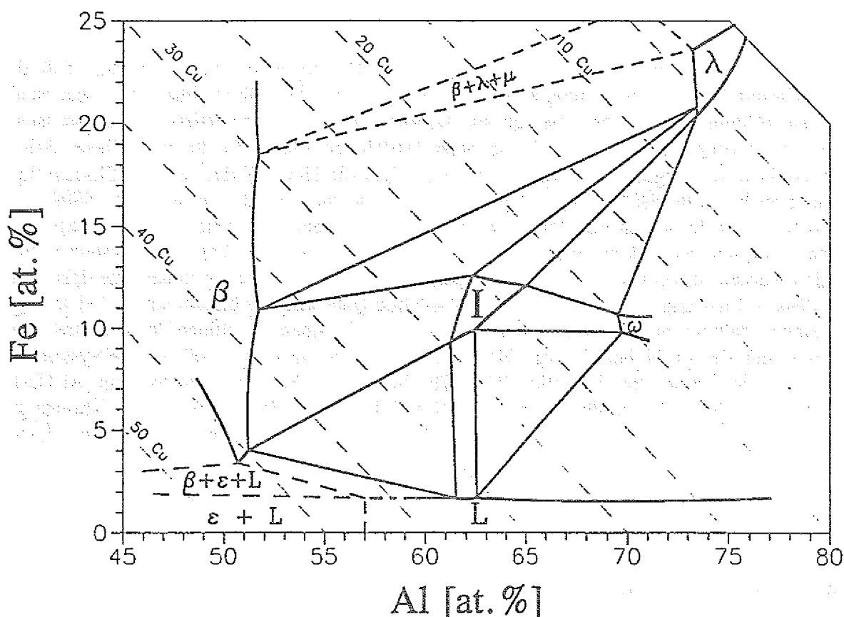
Abb. 4.13 Ausschnitt aus dem Phasendiagramm des Systems Al-Cu-Fe bei 973 K (nach [169]).
