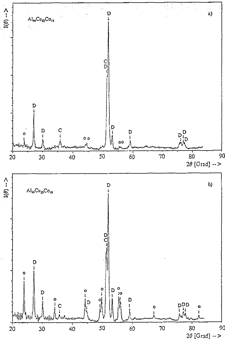
Abb. 5.45 Röntgendiffraktogramme von splatgekühlten Al-Cu-Co-Proben.
