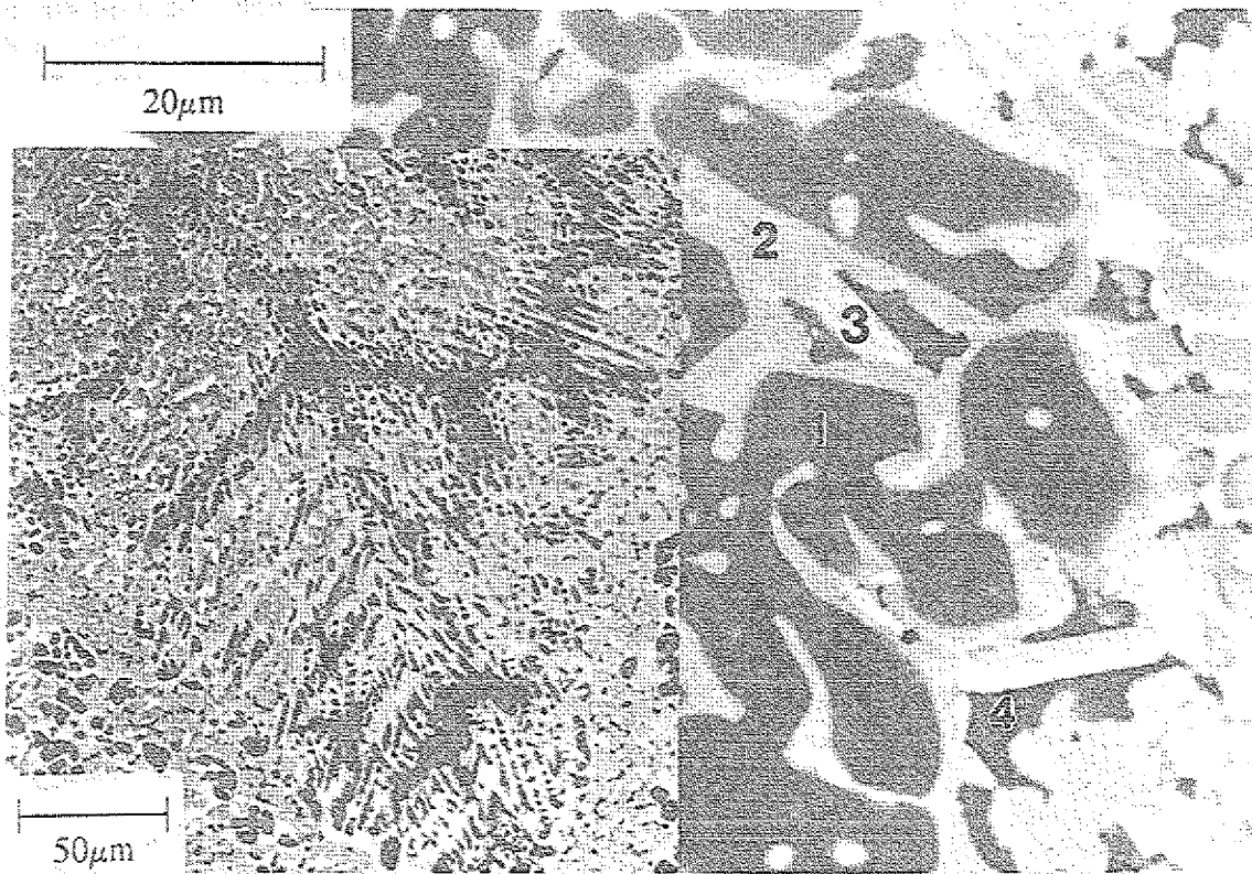
Abb. 5.12 REM-Bild des Gefüges der maximal unterkühlten \text{Al}_{58}\text{Cu}_{34}\text{Fe}_8 -Probe, deren Temperatur-Zeit-Profil in Abb. 5.10b gezeigt wurde. Das Nebenbild zeigt in geringerer Vergrößerung einen ausgedehnten, aus der I-Phase bestehenden Dendriten.
