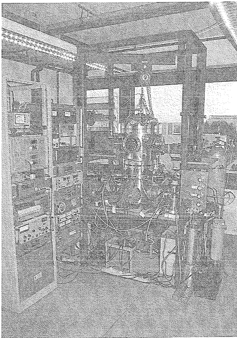
Abb. 4.2 Die Levitationsanlage.
