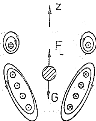
Abb. 4.1 Schematische Darstellung der Funktionsweise einer elektromagnetischen Levitationsanlage.
