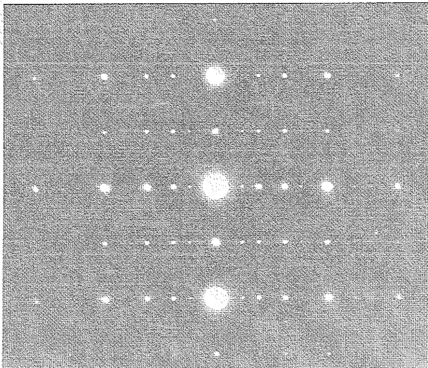
Abb. 5.49 TEM-Beugungsbild der [\bar{1}\bar{2}100] -Zonenachse einer aus der unterkühlten Schmelze splatgekühlten \text{Al}_{65}\text{Cu}_{25}\text{Co}_{10} -Probe.
