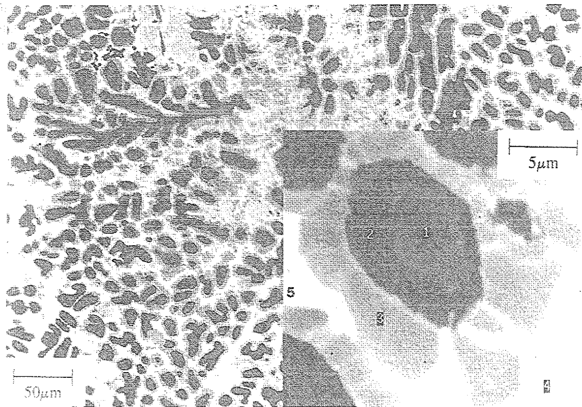
Abb. 5.23 REM-Aufnahme der kaum unterkühlten \text{Al}_{62}\text{Cu}_{25.5}\text{Fe}_{12.5} -Probe, deren Temperatur-Zeit-Profil in Abb. 5.22 gezeigt wurde. Das Nebenbild zeigt ein stärker vergrößertes Bild der Probe.
