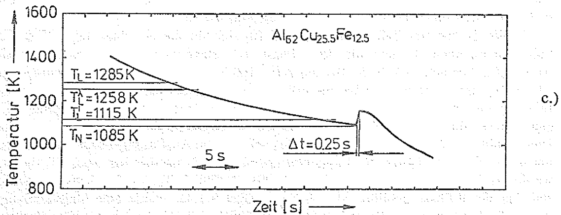
Abb. 5.10 Temperatur-Zeit-Profile von Levitationsexperimenten an Al-Cu-Fe-Proben unterschiedlicher Zusammensetzung, in denen maximale Unterkühlungen erreicht wurden.
