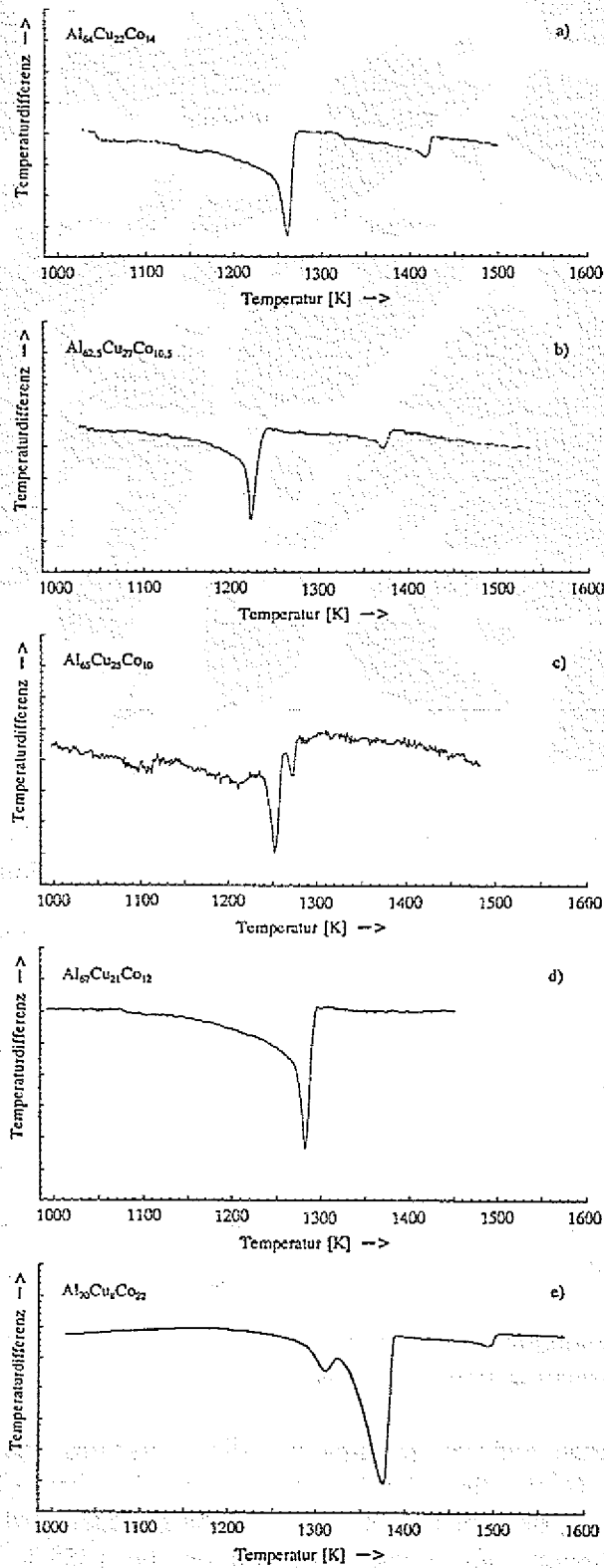
Abb. 5.5 DTA-Abkühlkurven von Al-Cu-Co-Proben unterschiedlicher Zusammensetzung.
