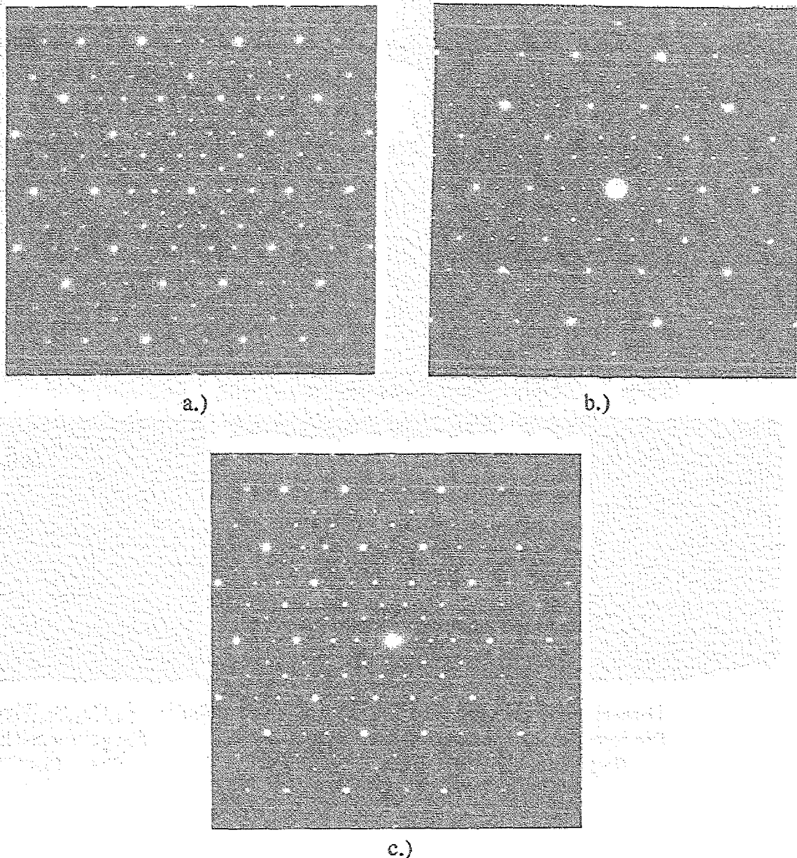
Abb. 5.14 TEM-Beugungsbilder der 5-zähligen Achse der I-Phase, gewonnen an den maximal unterkühlten Proben, deren Temperatur-Zeit-Profile in Abb. 5.10 gezeigt wurden. a.) \text{Al}_{60}\text{Cu}_{34}\text{Fe}_6 , b.) \text{Al}_{58}\text{Cu}_{34}\text{Fe}_8 und c.) \text{Al}_{62}\text{Cu}_{25.5}\text{Fe}_{12.5} .
