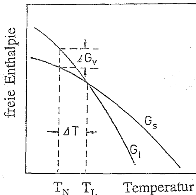
Abb. 3.1 Schematische Darstellung der freien Enthalpie G für Schmelze ( G_L ) und Festkörper ( G_S ) als Funktion der Temperatur T .
