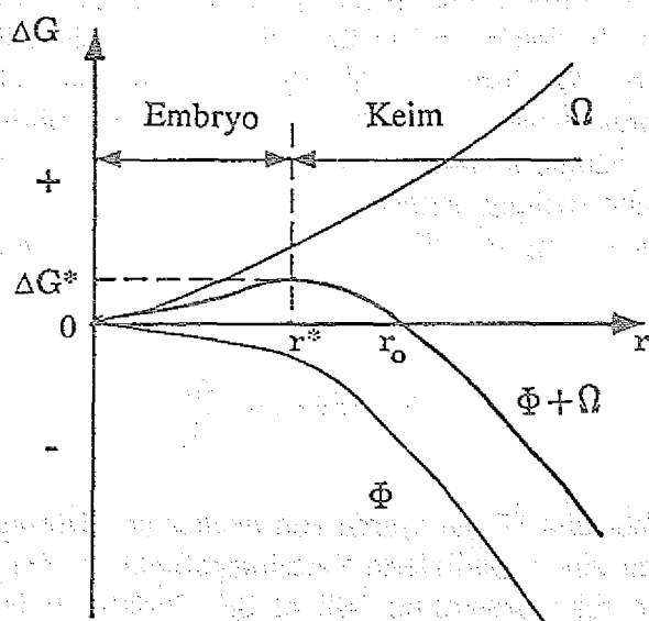
Abb. 3.2 Schematische Darstellung des Grenzflächen- ( \Omega ) und Volumenterms ( \Phi ) eines Clusters, sowie deren Summe ( \Delta G ), als Funktion des Clusterradius r .
