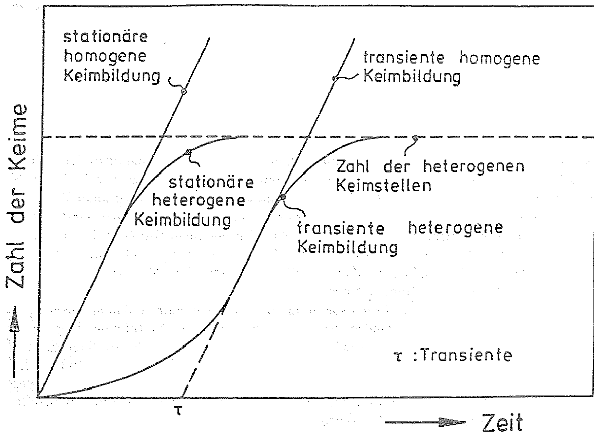
Abb. 3.4 Zeitliche Entwicklung der Zahl der Keime für homogene und heterogene Keimbildung mit und ohne Berücksichtigung transienter Effekte (aus [21]).
