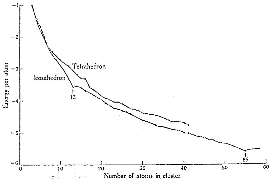
Abb. 3.6: Energie pro Clusteratom als Funktion der Clustergröße aus [115].
