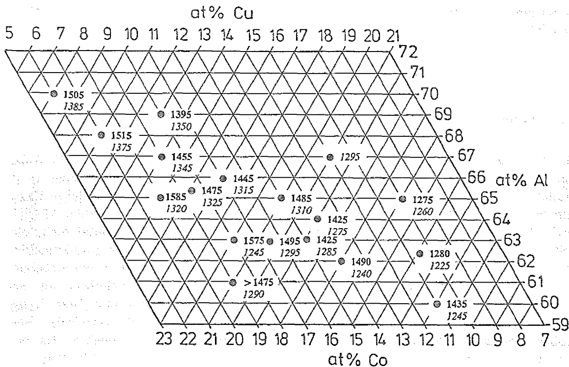
Abb. 5.7 Liquidustemperaturen T_L der Legierungen (Fettdruck) und der D-Phase T_L^D (kursiv) in K als Funktion der Legierungszusammensetzung.
