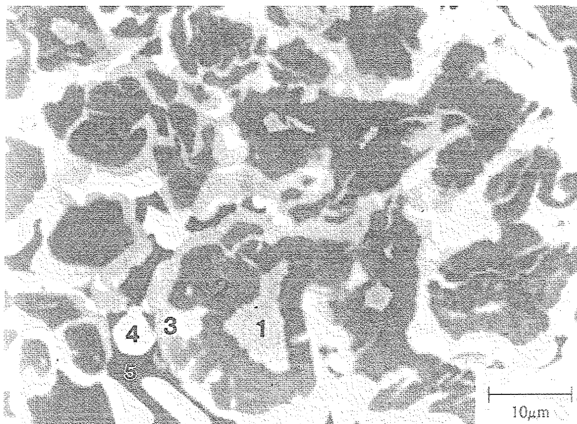
Abb. 5.21 REM-Aufnahme einer kaum unterkühlten \text{Al}_{58}\text{Cu}_{34}\text{Fe}_8 -Probe ( \Delta T=50 K).
