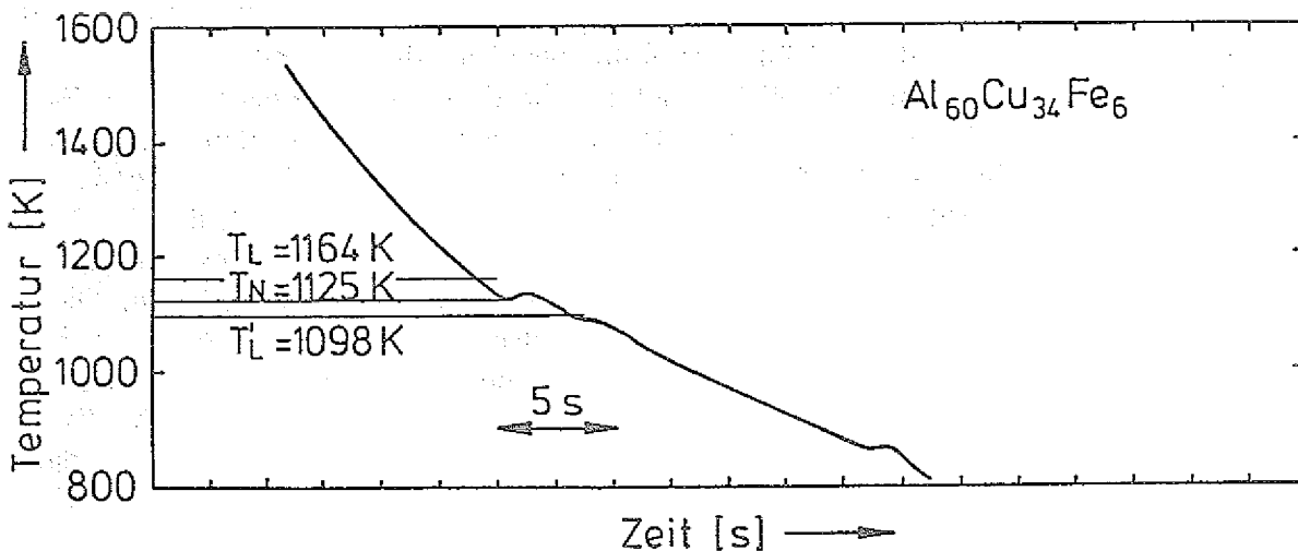
Abb. 5.19 Temperatur-Zeit-Profil einer kaum unterkühlten \text{Al}_{60}\text{Cu}_{34}\text{Fe}_6 -Probe.
