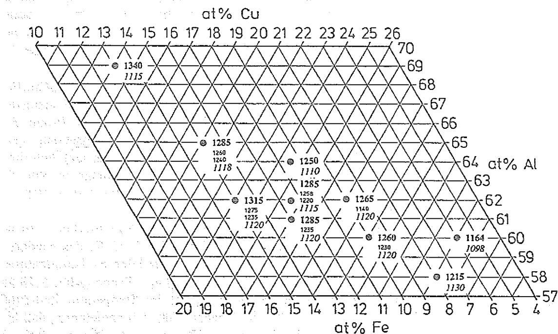
Abb. 5.3 Liquidustemperaturen T_L der Legierungen (Fettdruck) und der I-Phase T_L' (kursiv) als Funktion der Legierungszusammensetzung. Die klein gedruckten Temperaturen entsprechen weiteren Phasenumwandlungen (siehe Text). Alle Temperaturen sind in K angegeben.
