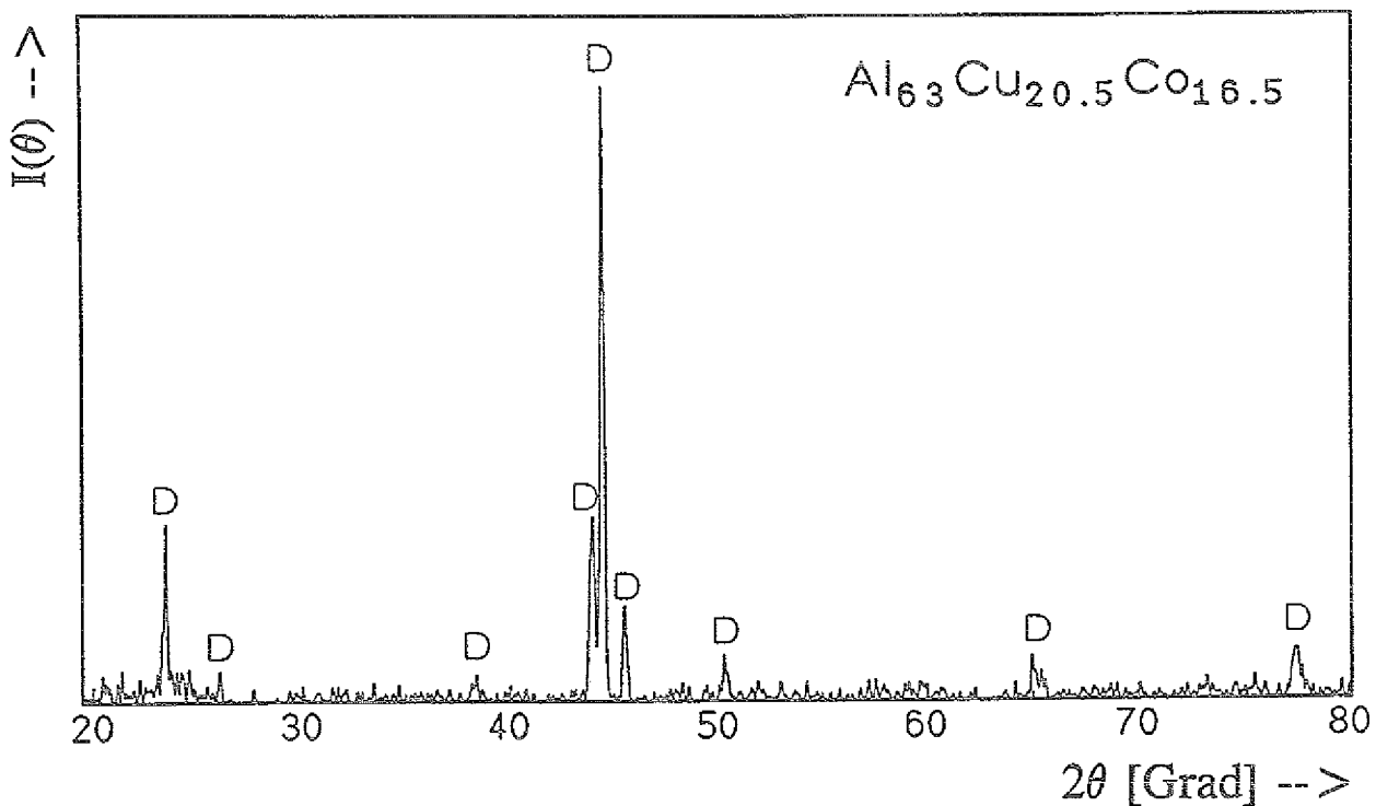
Abb. 5.46 Röntgendiffraktogramm einer \text{Al}_{63}\text{Cu}_{20.5}\text{Co}_{16.5} . Bei dieser Messung wurde \text{Cu-K}_\alpha -Strahlung verwendet!
