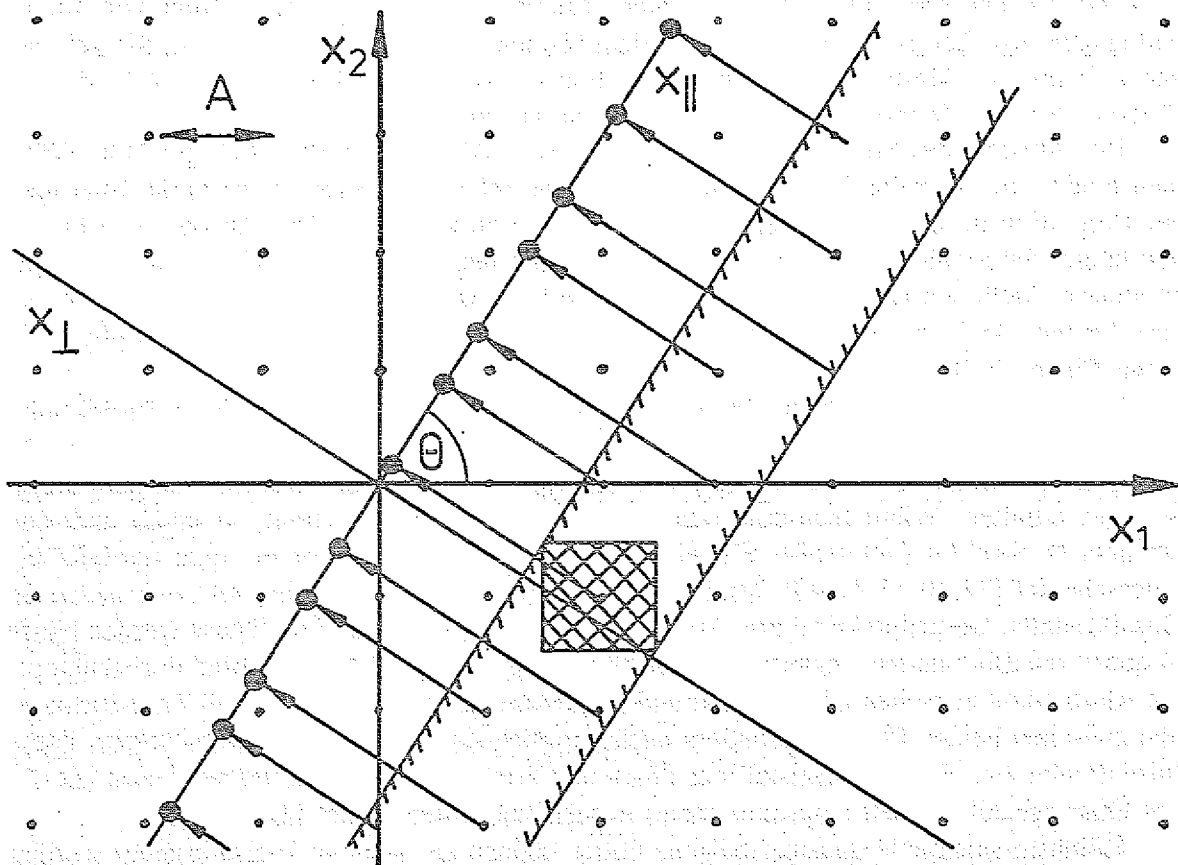
Abb. 2.11: Erzeugung eines eindimensionalen Quasigitters durch eine Projektion (nach [38]).
