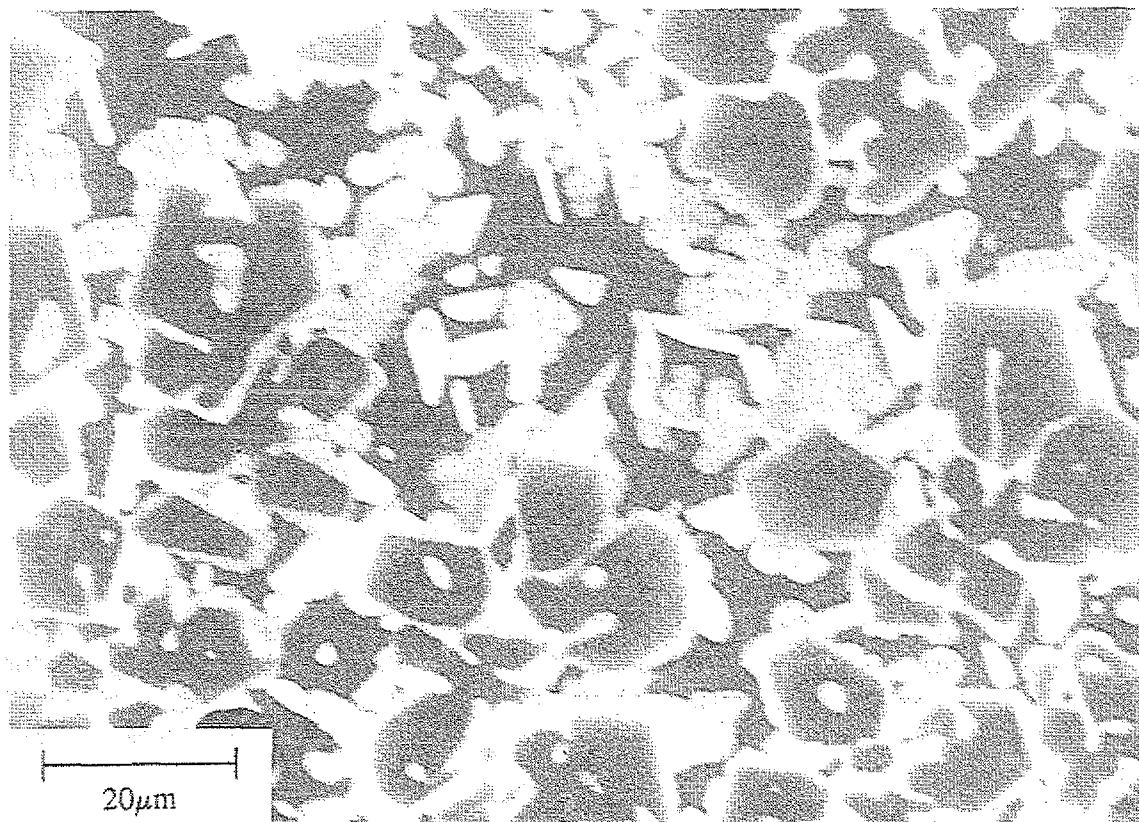
Abb. 5.26 REM-Aufnahme einer bei ca. 1090 K ( \Delta T_L^I = 10 K) erstarrten \text{Al}_{60}\text{Cu}_{34}\text{Fe}_6 -Probe. Die aus I-Phasen bestehenden Dendriten zeigen eine Facettierung.
