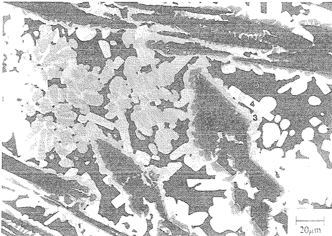
Abb. 5.2 REM-Aufnahme der in der Kalttiegel-Anlage erstarrten \text{Al}_{60}\text{Cu}_{34}\text{Fe}_6 -Probe. Die Zusammensetzungen der einzelnen Phasen sind Tabelle 5.1 zu entnehmen.
