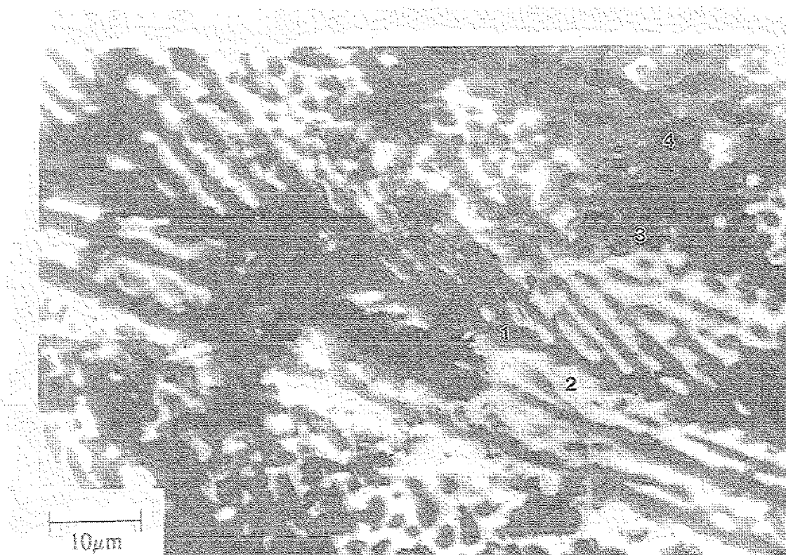
Abb. 5.29 REM-Bild des Gefüges der maximal unterkühlten \text{Al}_{65}\text{Cu}_{25}\text{Co}_{10} -Probe, deren Temperatur-Zeit-Profil in Abb. 5.27b gezeigt wurde.
