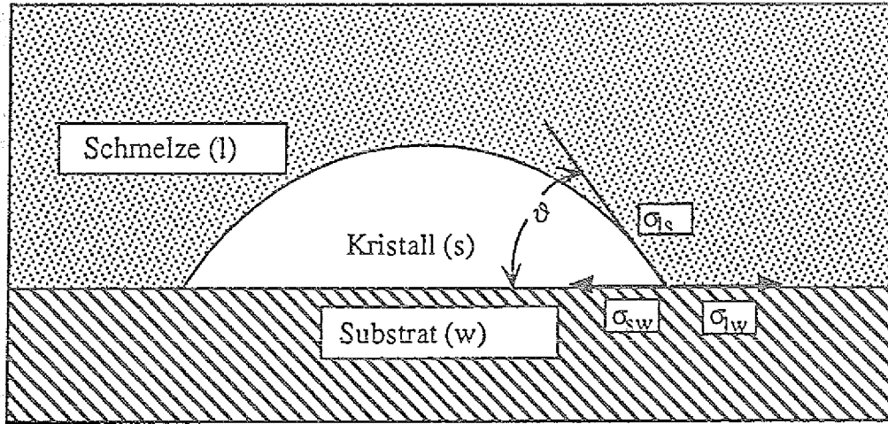
Abb. 3.3 Wachstum eines heterogenen Keims (s) auf einem Substrat (w).
