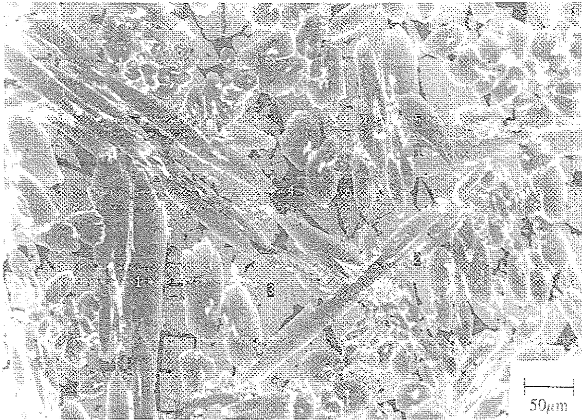
Abb. 5.37 REM-Aufnahme einer in der Kalttiegel-Anlage erstarrten \text{Al}_{67}\text{Cu}_{21}\text{Co}_{12} -Probe.
