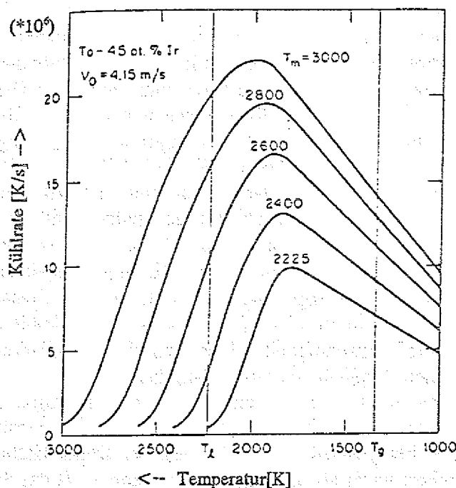
Abb. 4.7 Kühlrate als Funktion der Probestemperatur, berechnet für das Splatkühlen einer Ta 55 Ir 45 -Schmelze mit einer Stempelgeschwindigkeit von 4.15 m/s bei unterschiedlichen Ausgangstemperaturen (aus [153]).
