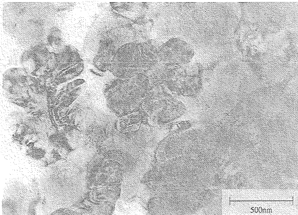
Abb. 5.44 TEM-Hellfeldbild einer splatgekühlten Al 60 Cu 34 Fe 6 -Probe, bei der auf Grund von zu geringem Aufheizen keine optimale Kühlrate erreicht wurde.
