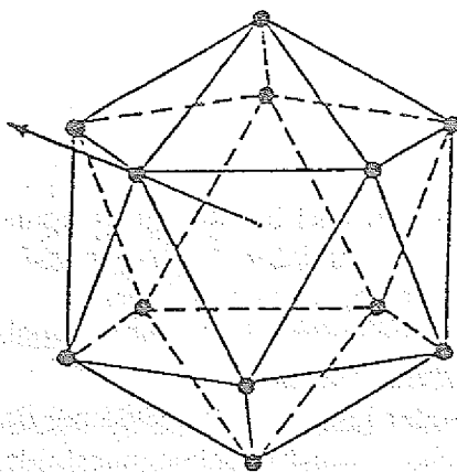
Abb. 2.2: Ikosaeder.
