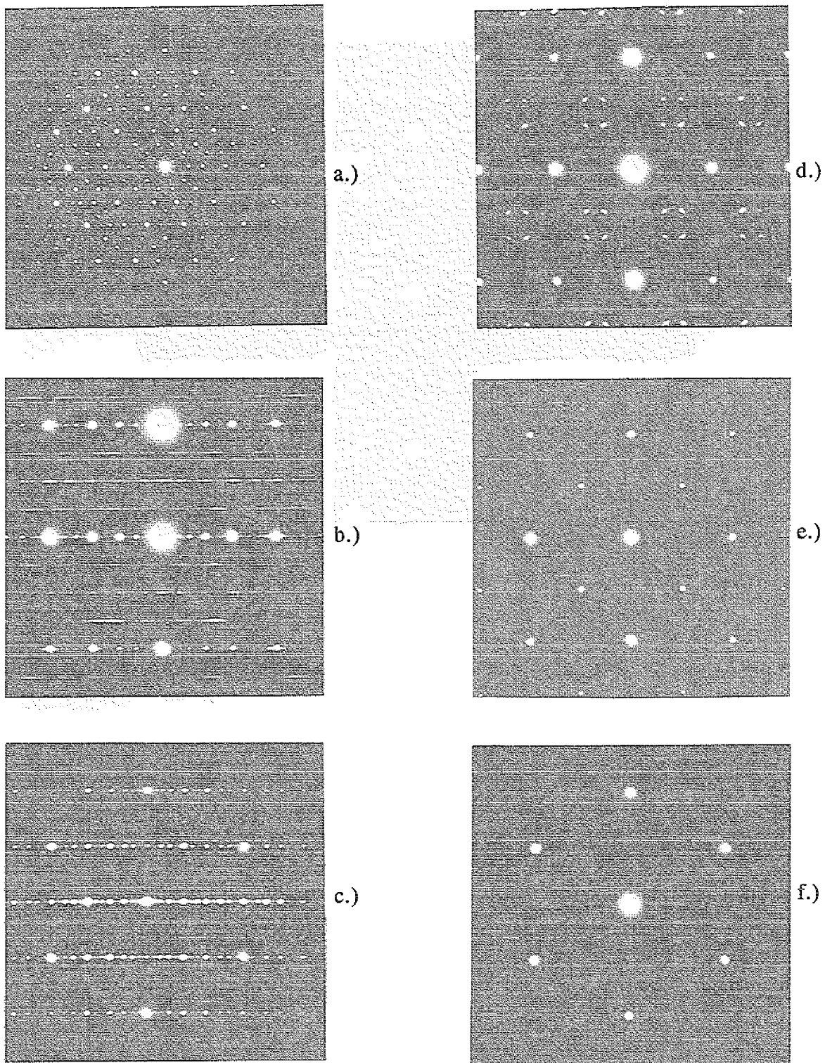
Abb. 5.33 Beugungsbilder der [00001] - (a), [\bar{1}2100] - (b) und [001\bar{1}0] -Zonenachse (c) der D-Phase in der \text{Al}_{65}\text{Cu}_{25}\text{Co}_{10} -Probe und unter gleichen Kippwinkeln an der angrenzenden \tau_{13} -Phase aufgenommene Beugungsbilder der [110] - (d), [001] - (e) und [111] -Zonenachse (f).
