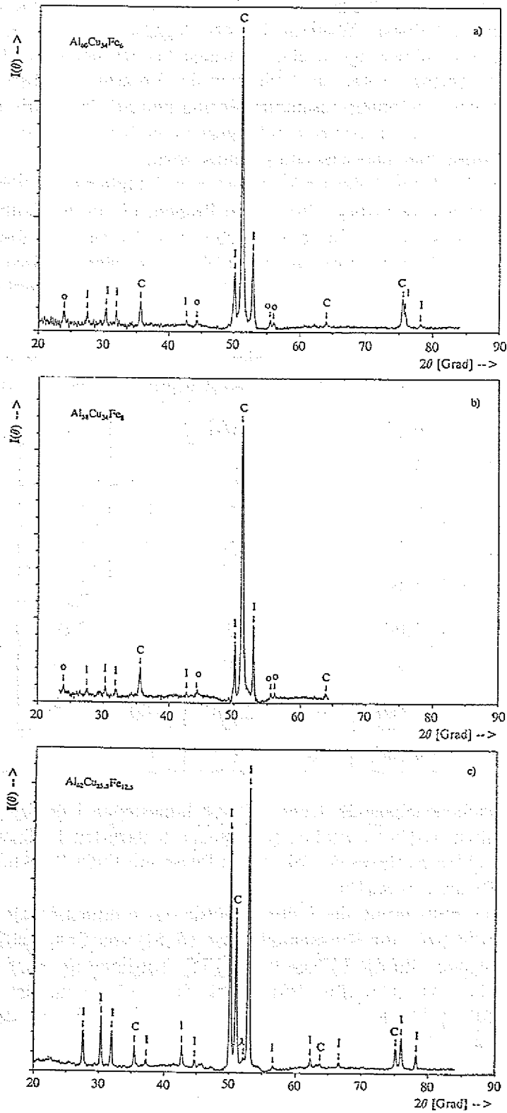
Abb. 5.17 Röntgendiffraktogramme, gewonnen an den maximal unterkühlten Al-Cu-Fe-Proben: a.) \text{Al}_{60}\text{Cu}_{34}\text{Fe}_6 , b.) \text{Al}_{58}\text{Cu}_{34}\text{Fe}_8 und c.) \text{Al}_{62}\text{Cu}_{25.5}\text{Fe}_{12.5} I: I-Phase, C: kubische Phase (CsCl-Typ), o: \text{Al}_2\text{Cu} , \lambda : \lambda -Phase.
