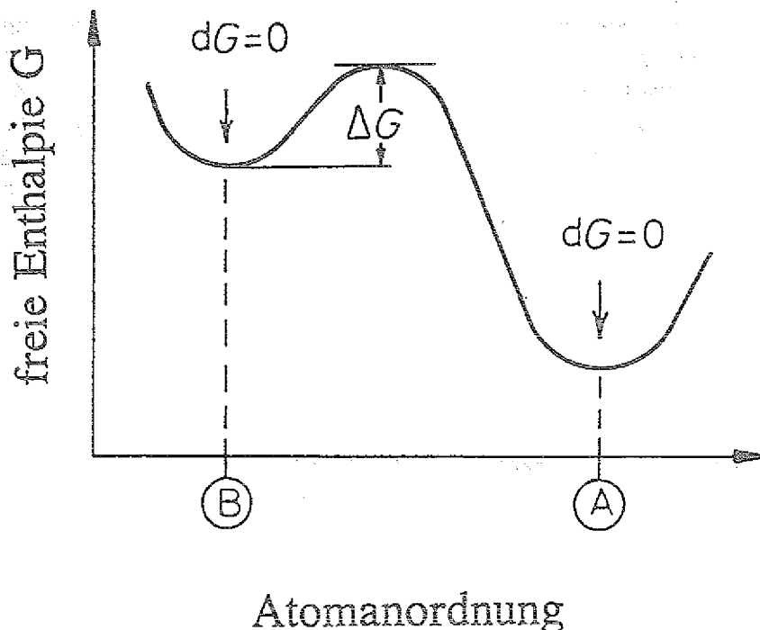
Abb. 2.12 Schematische Darstellung der Gibbs'schen freien Energie als Funktion der Atomanordnung (Anordnung A: stabile Phase, Anordnung B: metastabile Phase).
