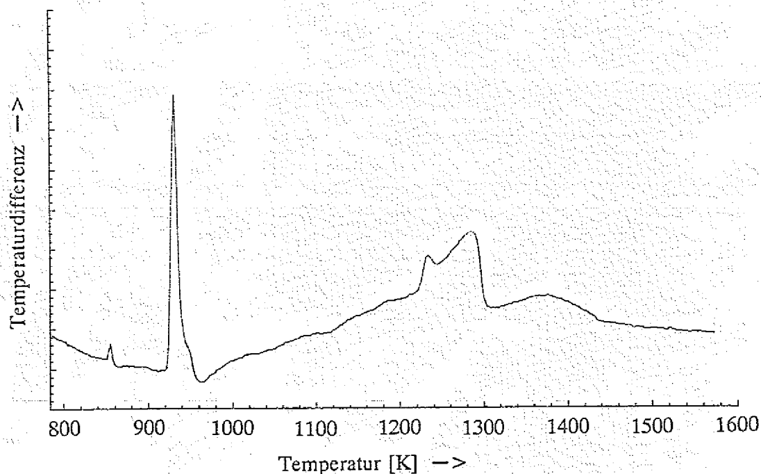
Abb. 5.36 DTA-Aufheizkurve gewonnen an der maximal unterkühlten \text{Al}_{64}\text{Cu}_{22}\text{Co}_{14} -Probe, deren Temperatur-Zeit-Profil in Abb. 5.27c gezeigt wurde.
