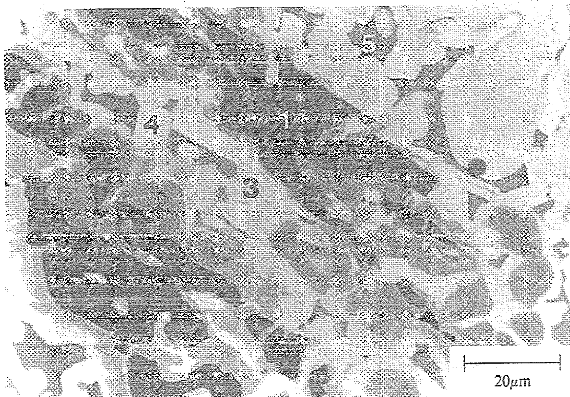
Abb. 5.24 REM-Aufnahme einer ca. 40 K bezüglich T_L unterkühlten \text{Al}_{62}\text{Cu}_{25.5}\text{Fe}_{12.5} -Probe.
