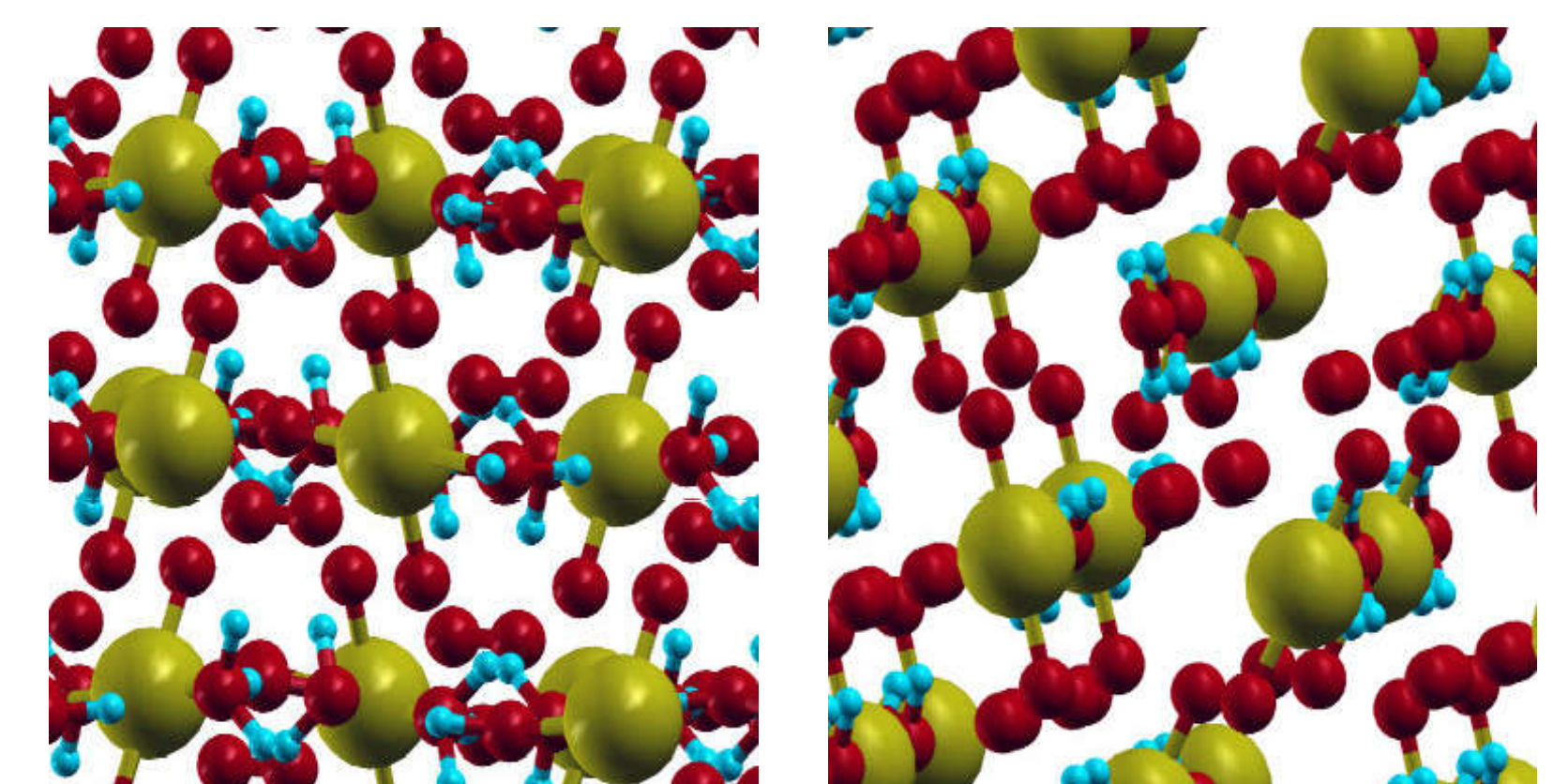
( UO_2 ) O_2 ( H_2O ) _4 (ST) ( UO_2 ) O_2 ( H_2O ) _2 (MST)
