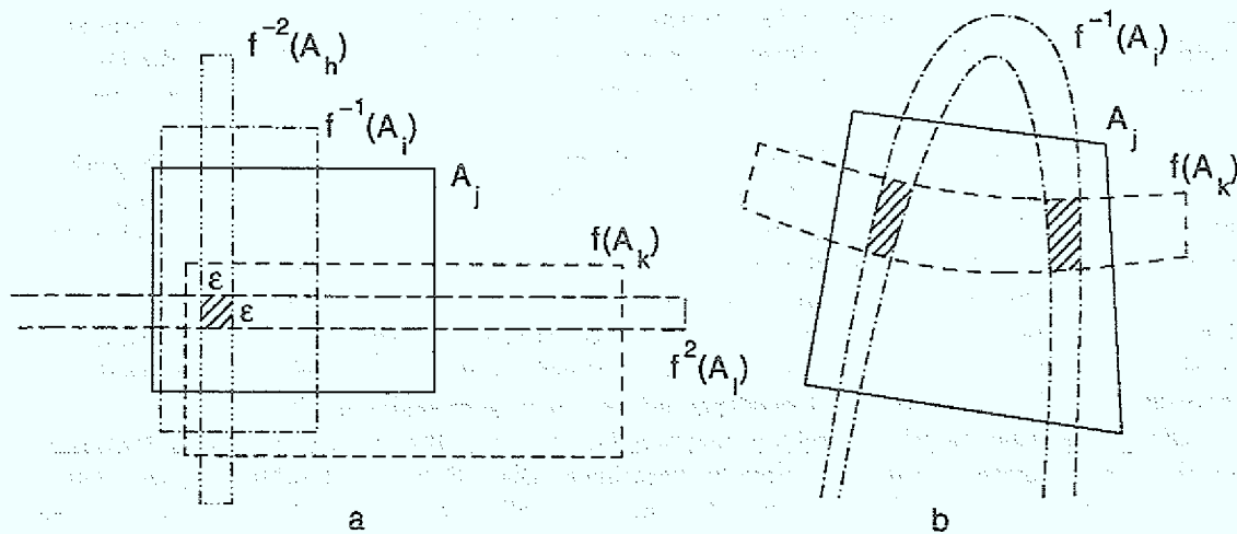
Abbildung 2.1: Abb. a zeigt ein Beispiel für eine günstige Wahl Symbolischer Gebiete. Ein Orbit schneidet bei aufeinanderfolgenden Zeitschritten die Symbolischen Gebiete, A_l , A_k , A_j , A_i und A_h . Seine möglichen Lagen werden durch den Schnitt von Abbildern und Urbildern dieser Symbolischen Gebiete auf ein schraffiertes Gebiet beschränkt, das viel kleiner als die Symbolischen Gebiete selbst ist. Abb. b illustriert ebenso schematisch, warum bei einer ungünstigen Wahl der Symbolischen Gebiete, das heißt bei einer nicht generierenden Partition, die Lage des Orbits nur sehr ungenau bestimmt sein kann.
