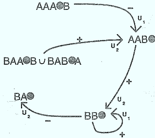
Abbildung 8.10: Die senkrechte Ordnung, nachdem die Orientierung im Gebiet BB\odot umgedreht wurde. Nur ein Ausschnitt des Graphen 8.9 wird gezeigt. Geändert hat sich die Beschriftung „+“ oder „-“ nur auf den Übergängen, die entweder zu BB\odot hin oder von BB\odot weg führen, und außerdem die Beschriftung U_i der Übergänge, die zu BB\odot hin führen.
