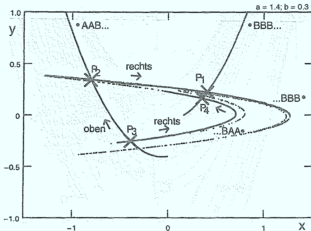
Abbildung 8.6: Die AB -Partiton des Hénon Attraktors bei Standardparameterwerten erzeugt keine selbstkonsistente räumliche Ordnung. Die Attraktorpunkte sind wie in Abb. 4.2 eingetragen. Die vier Attraktorpunkte P_1 , P_2 , P_3 und P_4 liegen jeweils paarweise auf kontrahierenden und expandierenden Blättern (dicke durchgezogene Linien), die von der AB -Partiton erzeugt werden. Wenn P_2 als oberhalb von P_3 definiert wird, dann liegt P_1 rechts von P_2 und P_4 rechts von P_3 . Auf dem kontrahierenden Blatt von P_1 und P_4 kann dann aber keine Richtung „oben“ gewählt werden, die mit diesen beiden Richtungen „rechts“ in Einklang wäre.
