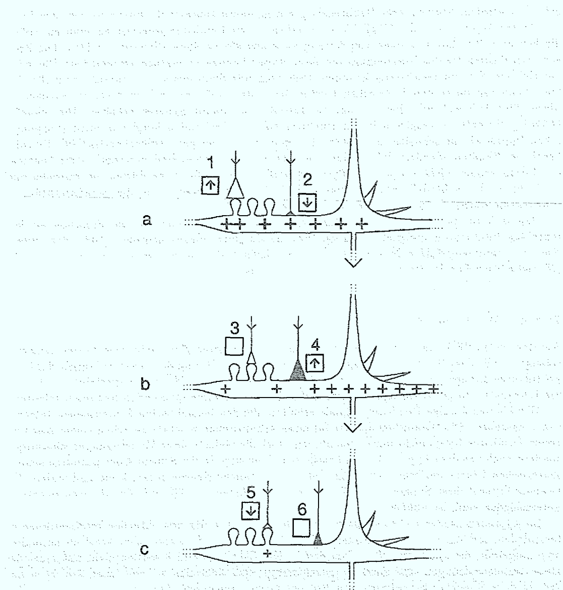
Abbildung D.3: Die drei idealen Erregungszustände eines Basaldendriten dieses Modells. Der Dendrit ist entweder stark erregt (a), geshunter (b) oder passiv (c). Depolarisierung des Dendriten oder des Zellkörpers wird durch Pluszeichen symbolisiert. In (a) und (b) feuert die Pyramidenzelle. Nur aktive Synapsen sind eingezeichnet. Die ideale Stärke einer aktiven erregenden Synapse (offenes Dreieck auf Dorn) und einer aktiven Shunt-Synapse (schwarzes Dreieck auf Schaft) sind durch die Größe (groß-mittel-klein) der Dreiecke angedeutet. Die Richtung der Lernprozesse, die solche synaptischen Stärken erzeugen, wird durch den eingerahmten Pfeil symbolisiert: Pfeil nach oben bedeutet Stärkung, Pfeil nach unten Schwächung, ein leeres Kästchen geringe Änderung der Synapse.
