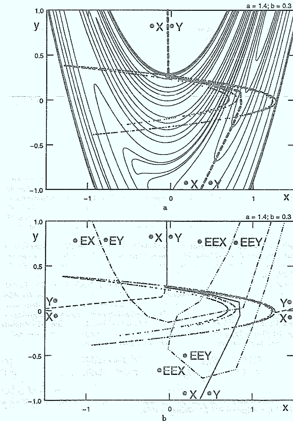
Abbildung 7.1: Die XY -Partition des Hénon Attraktors bei Standardparameterwerten. Sie ist anders, aber nicht unbedingt komplizierter als die 01 -Partition in Abb. 2.4 und verwechselt auch nicht mehr Orbits als diese. In Abb. a sind die Attraktorpunkte und die Abschnitte der stabilen Mannigfaltigkeit wie in Abb. 2.4 eingetragen. Abb. b zeigt die Partitions Grenzen bei drei aufeinanderfolgenden Zeiten. Sie trennen \circ EX von \circ EY , \circ X von \circ Y , bzw. X \circ von Y \circ .
