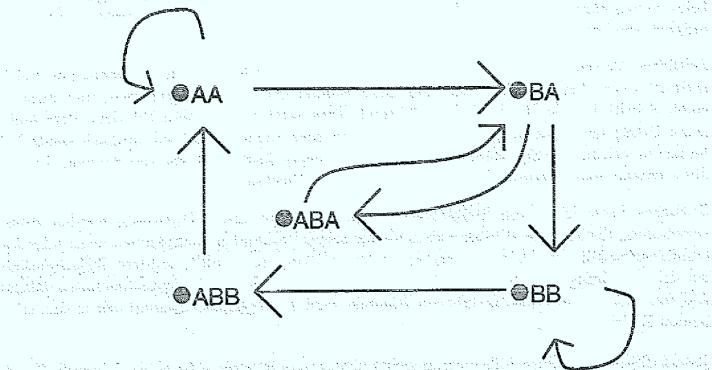
Abbildung 5.7: Die Partition, die beschreibt, welche kontrahierenden Blätter unter der inversen Abbildung f^{-1} geteilt werden. Diese Partition erzeugt dieselben kontrahierenden Blätter wie die Partition in Abb. 5.6. Das kontrahierende Bündel \{\bullet AB(A \sqcup B)^{+\infty}\} wurde in seine Teilmengen \{\bullet ABA(A \sqcup B)^{+\infty}\} und \{\bullet ABB(A \sqcup B)^{+\infty}\} zerlegt. Keines der darin enthaltenen kontrahierenden Blätter unter der inversen Abbildung f^{-1} geteilt. Denn von \bullet ABA und \bullet ABB geht wegen der grammatikalischen Regel A \bullet ABA = B \bullet ABB = \emptyset nur jeweils ein Übergang aus.
