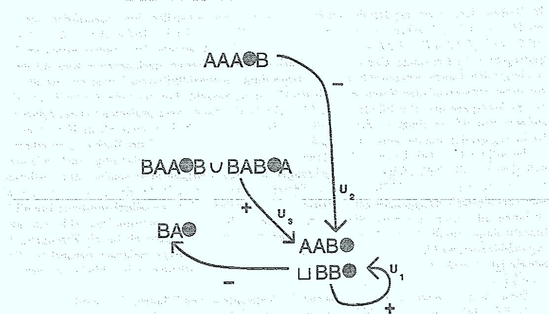
Abbildung 8.11: Die senkrechte Ordnung, nachdem die beiden expandierenden Bündel \{(A \sqcup B)^{-\infty} AAB \circ\} und \{(A \sqcup B)^{-\infty} BB \circ\} aus Abb. 8.10 zu \{(A \sqcup B)^{-\infty} (AAB \sqcup (A \sqcup B)BB) \circ\} vereinigt wurden. Zu diesem neuen expandierenden Bündel führen drei Übergänge. Weil in Abb. 8.10 der Übergang AAB \circ \rightarrow BB \circ die senkrechte Orientierung erhält, liegen auch in dem neuen Graphen die expandierenden Blätter, die von BAA \circ B \cup BAB \circ A her stammen, oberhalb der Blätter, die von AAA \circ B her stammen: U_3 > U_2 .
