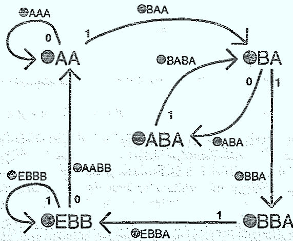
Abbildung 6.3: Die Rekonstruktion von 01-Symbolen in der Partition, die die kontrahierenden Bündel beschreibt. Der gerichtete Graph ist derselbe wie in Abb. 5.12. Doch jeder Übergang \circ \alpha \rightarrow \circ \beta trägt zwei zusätzliche Beschriftungen. Die Beschriftung \circ E \alpha \cap \circ \beta bezeichnet das Gebiet im Phasenraum, das diesem Übergang entspricht. Und die Beschriftung mit dem Symbol 0 oder 1 kennzeichnet, ob dieses Gebiet nach der Rekonstruktion der 01-Partition in dem Symbolischen Gebiet \circ 0 oder in \circ 1 enthalten ist.
