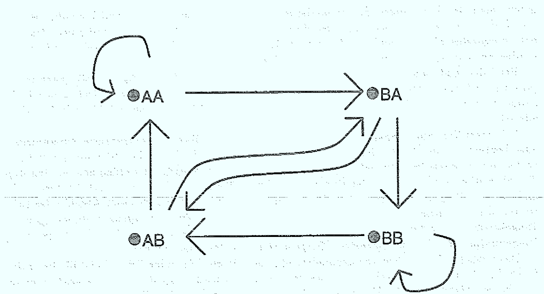
Abbildung 5.6: Die Übergänge zwischen den Symbolischen Gebieten der Partition \{\bullet AA, \bullet AB, \bullet BA, \bullet BB\} unter der inversen Abbildung f^{-1} . Am Beginn der Beispielrechnung werden die kontrahierenden Bündel \{\bullet B_j (\bigsqcup_{i=1}^m B_i)^{+\infty}\} durch diese Partition erzeugt. Ein Übergang von \bullet B_i nach \bullet B_j existiert dann, wenn f^{-1}(\bullet B_i) \cap \bullet B_j = \bullet B_j B_i \neq \emptyset .
