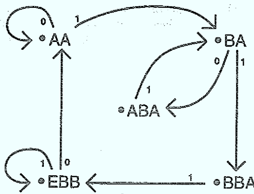
Abbildung 6.4: Zusammenfassung der Abbildungen 6.2 und 6.3. Die zeitlichen Übergänge zwischen den Symbolischen Gebieten der zwiefachen Partition sind mit den Symbolen C_1 = 0 und C_2 = 1 beschriftet.
